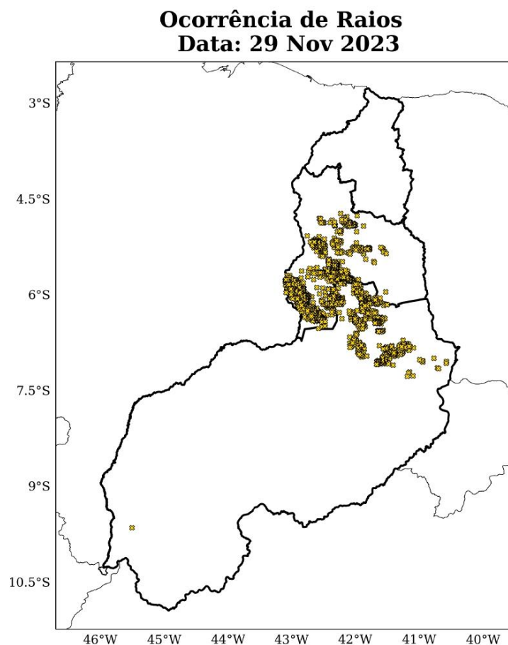
Figura 6: Densidade de descargas atmosféricas nuvem-solo detectadas pelo sistema Earth Networks para o dia 29 de Novembro sobre a área de concessão da Equatorial-PI.
