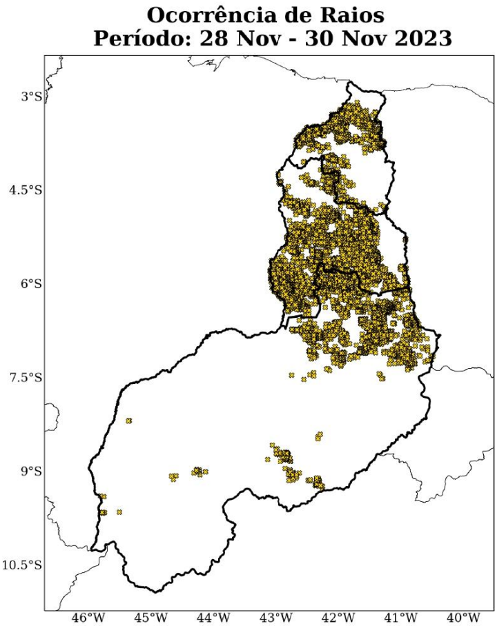
Figura 7: Total de descargas atmosféricas nuvem-solo detectadas pelo sistema Earth Networks durante o período de 28 a 30 de Novembro de 2023 sobre a área de concessão da Equatorial-PI.
