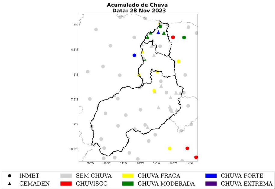
Figura 8: Acumulado diário de precipitação sobre a área de concessão da Equatorial-PI para o dia 28 de Novembro, baseado nas estações meteorológicas do INMET e CEMADEN.
