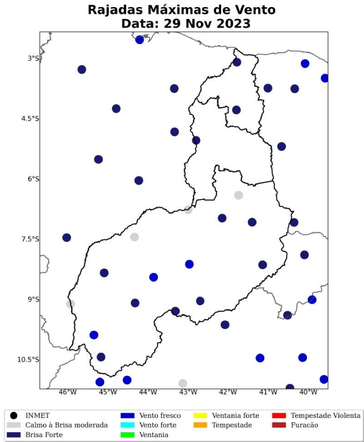
Figura 13: Máxima rajada de vento diária sobre a área de concessão da Equatorial-PI para o dia 29 de Novembro, baseado nas estações meteorológicas do INMET.
