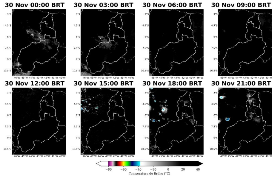
Figura 4: Imagens realçadas do satélite GOES-16 das 00 BRT até 21 BRT (a cada 3 horas) para o dia 30 de Novembro.
