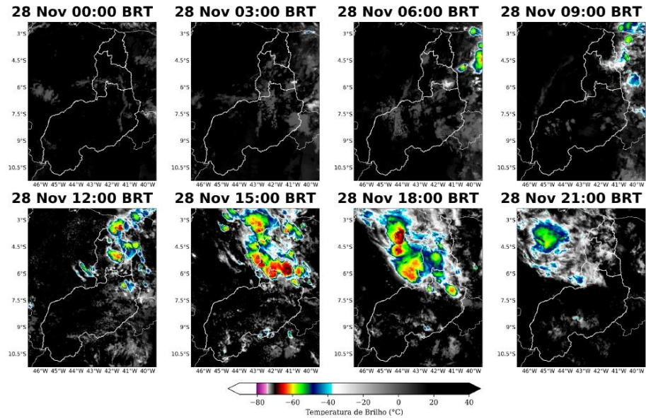
Figura 2: Imagens realçadas do satélite GOES-16 das 00 BRT até 21 BRT (a cada 3 horas) para o dia 28 de Novembro.
