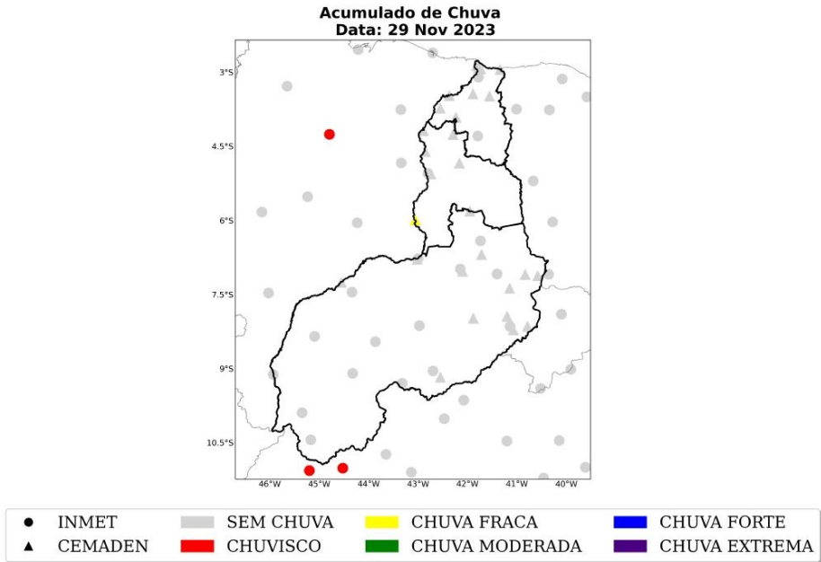
Figura 9: Acumulado diário de precipitação sobre a área de concessão da Equatorial-PI para o dia 29 de Novembro, baseado nas estações meteorológicas do INMET e CEMADEN.
