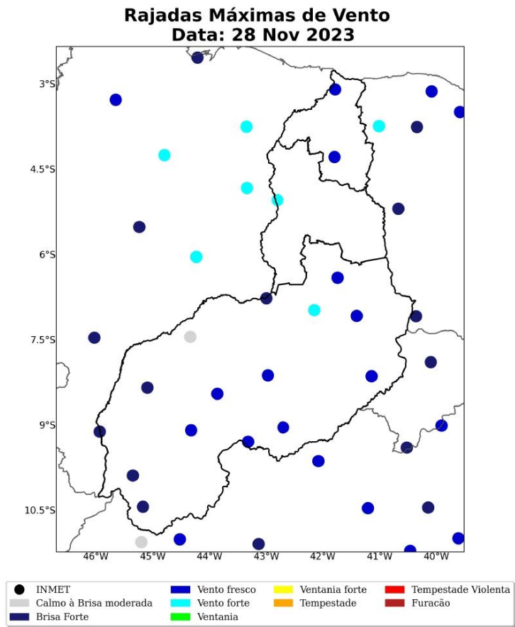
Figura 12: Máxima rajada de vento diária sobre a área de concessão da Equatorial-PI para o dia 28 de Novembro, baseado nas estações meteorológicas do INMET.
