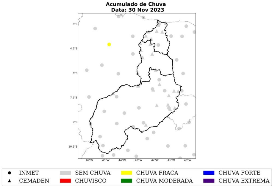
Figura 10: Acumulado diário de precipitação sobre a área de concessão da Equatorial-PI para o dia 30 de Novembro, baseado nas estações meteorológicas do INMET e CEMADEN.
