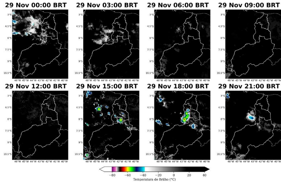
Figura 3: Imagens realçadas do satélite GOES-16 das 00 BRT até 21 BRT (a cada 3 horas) para o dia 29 de Novembro.
