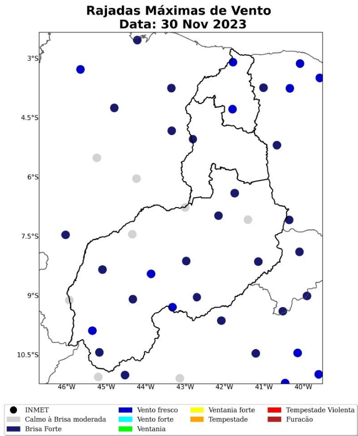
Figura 14: Máxima rajada de vento diária sobre a área de concessão da Equatorial-PI para o dia 30 de Novembro, baseado nas estações meteorológicas do INMET.
