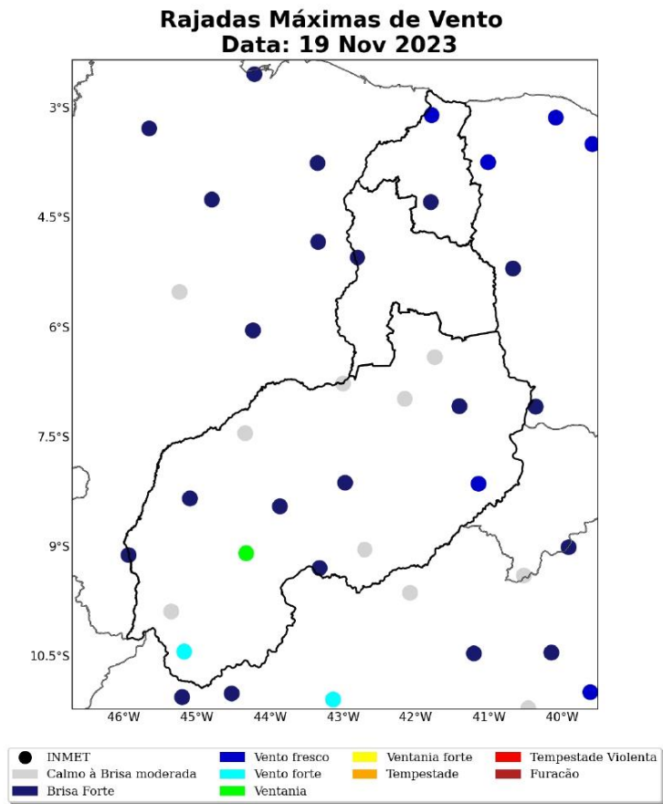
Figura 16: Máxima rajada de vento diária sobre a área de concessão da Equatorial-PI para o dia 19 de Novembro, baseado nas estações meteorológicas do INMET.
