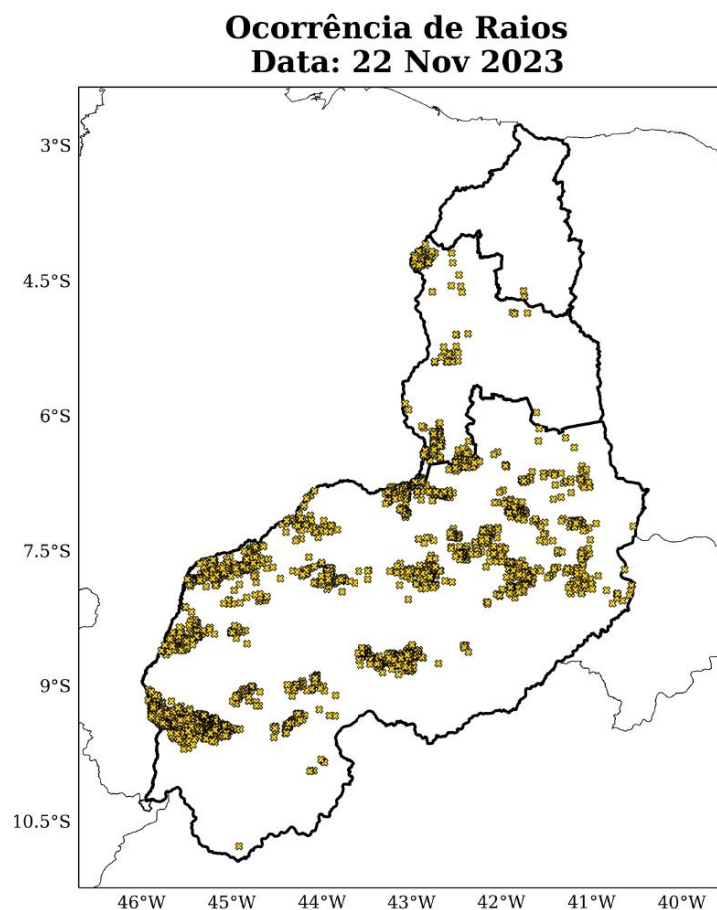
Figura 9: Densidade de descargas atmosféricas nuvem-solo detectadas pelo sistema Earth Networks para o dia 22 de Novembro sobre a área de concessão da Equatorial-PI.
