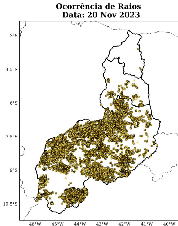
Figura 7: Densidade de descargas atmosféricas nuvem-solo detectadas pelo sistema Earth Networks para o dia 20 de Novembro sobre a área de concessão da Equatorial-PI.
