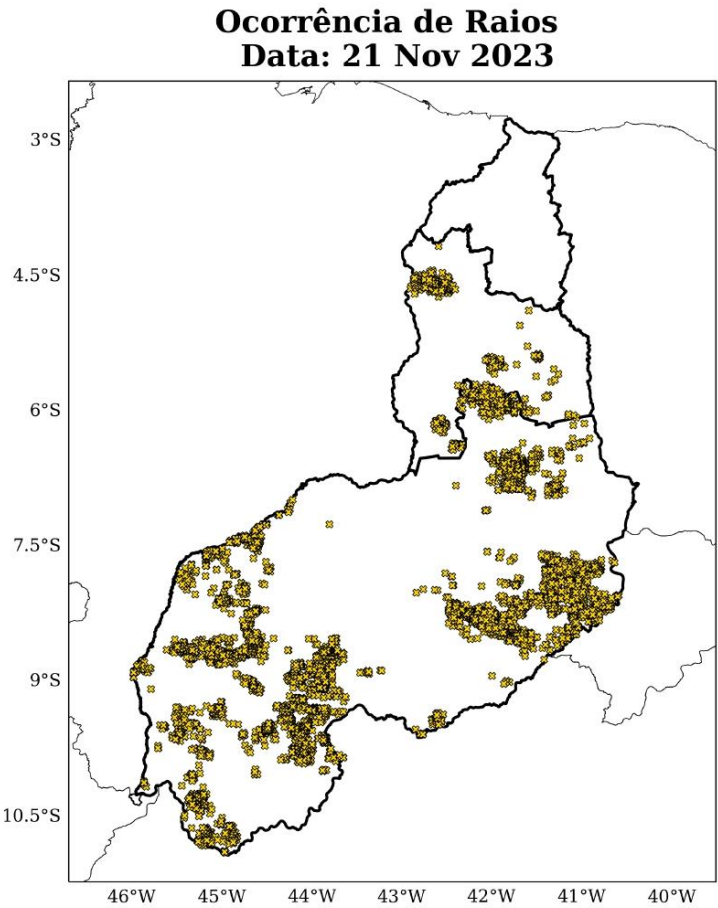
Figura 8: Densidade de descargas atmosféricas nuvem-solo detectadas pelo sistema Earth Networks para o dia 21 de Novembro sobre a área de concessão da Equatorial-PI.
