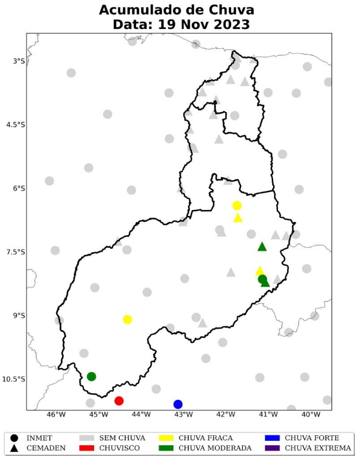
Figura 11: Acumulado diário de precipitação sobre a área de concessão da Equatorial-PI para o dia 19 de Novembro, baseado nas estações meteorológicas do INMET e CEMADEN.
