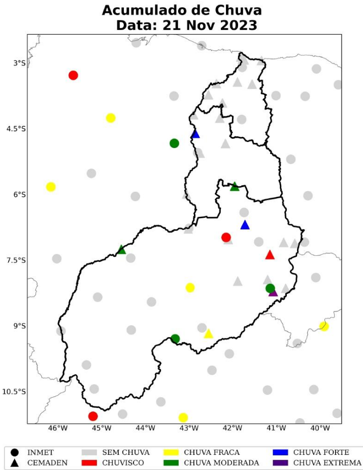
Figura 13: Acumulado diário de precipitação sobre a área de concessão da Equatorial-PI para o dia 21 de Novembro, baseado nas estações meteorológicas do INMET e CEMADEN.
