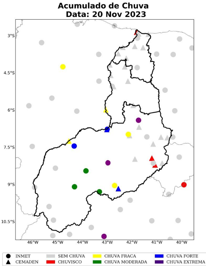
Figura 12: Acumulado diário de precipitação sobre a área de concessão da Equatorial-PI para o dia 20 de Novembro, baseado nas estações meteorológicas do INMET e CEMADEN.
