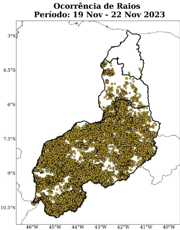
Figura 10: Total de descargas atmosféricas nuvem-solo detectadas pelo sistema Earth Networks durante o período de 19 a 22 de Novembro de 2023 sobre a área de concessão da Equatorial-PI.
