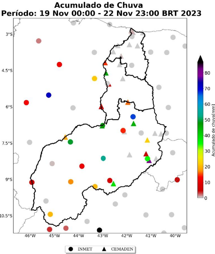
Figura 15: Acumulado de precipitação sobre o estado do Piauí para o período do evento (dias 19 a 22 de Novembro de 2023), baseado nas estações meteorológicas do INMET e CEMADEN.
