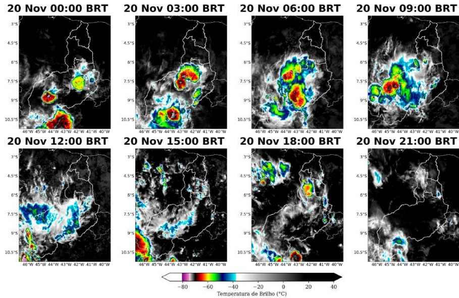
Figura 3: Imagens realçadas do satélite GOES-16 das 00 BRT até 21 BRT (a cada 3 horas) para o dia 20 de Novembro.
