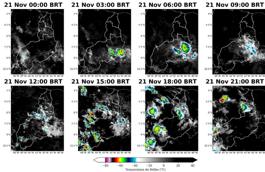
Figura 4: Imagens realçadas do satélite GOES-16 das 00 BRT até 21 BRT (a cada 3 horas) para o dia 21 de Novembro.
