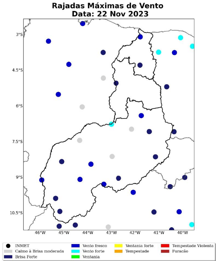
Figura 19: Máxima rajada de vento diária sobre a área de concessão da Equatorial-PI para o dia 22 de Novembro, baseado nas estações meteorológicas do INMET.
