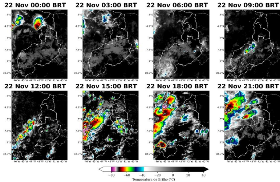
Figura 5: Imagens realçadas do satélite GOES-16 das 00 BRT até 21 BRT (a cada 3 horas) para o dia 22 de Novembro.
