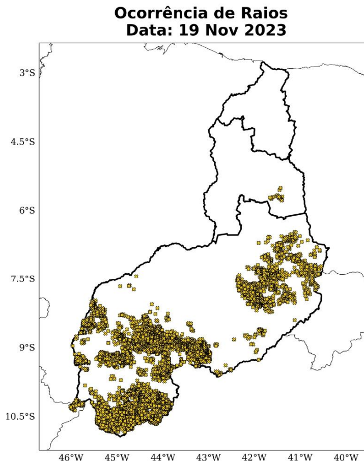
Figura 6: Densidade de descargas atmosféricas nuvem-solo detectadas pelo sistema Earth Networks para o dia 19 de Novembro sobre a área de concessão da Equatorial-PI.
