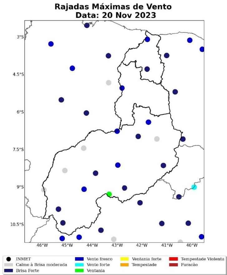
Figura 17: Máxima rajada de vento diária sobre a área de concessão da Equatorial-PI para o dia 20 de Novembro, baseado nas estações meteorológicas do INMET.
