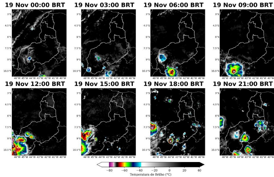
Figura 2: Imagens realçadas do satélite GOES-16 das 00 BRT até 21 BRT (a cada 3 horas) para o dia 19 de Novembro.
