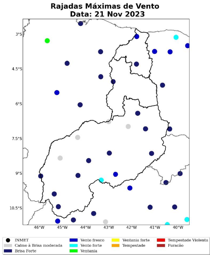
Figura 18: Máxima rajada de vento diária sobre a área de concessão da Equatorial-PI para o dia 21 de Novembro, baseado nas estações meteorológicas do INMET.
