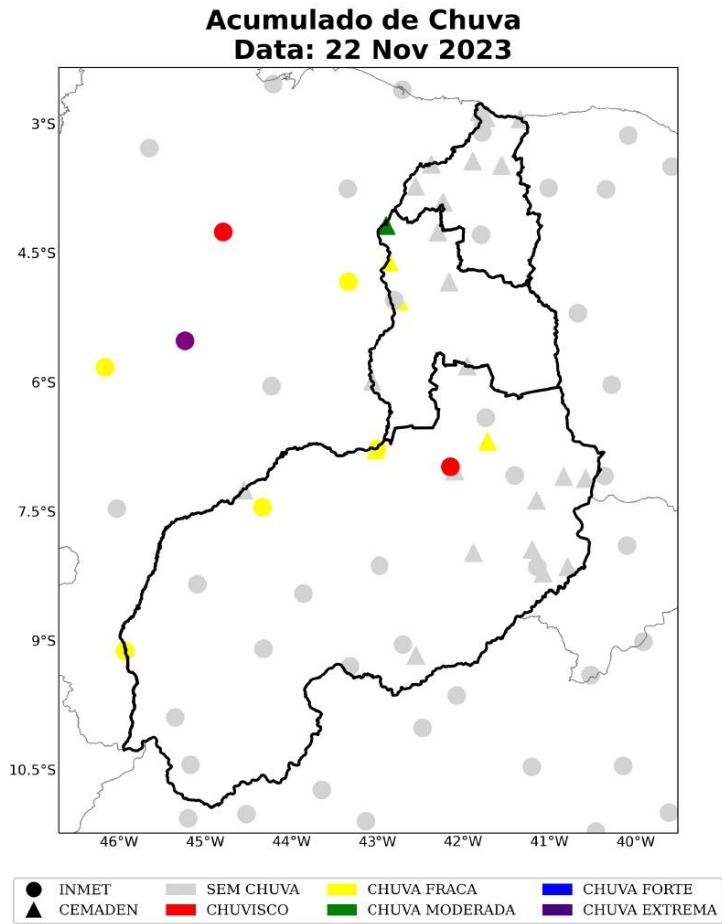
Figura 14: Acumulado diário de precipitação sobre a área de concessão da Equatorial-PI para o dia 22 de Novembro, baseado nas estações meteorológicas do INMET e CEMADEN.
