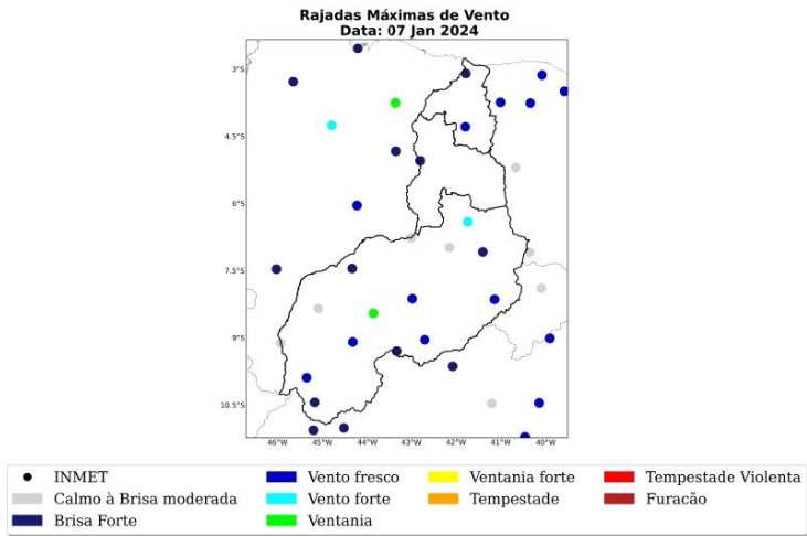
Figura 10: Máxima rajada de vento diária sobre a área de concessão da Equatorial-PI para o dia 07 de janeiro, baseado nas estações meteorológicas do INMET.
