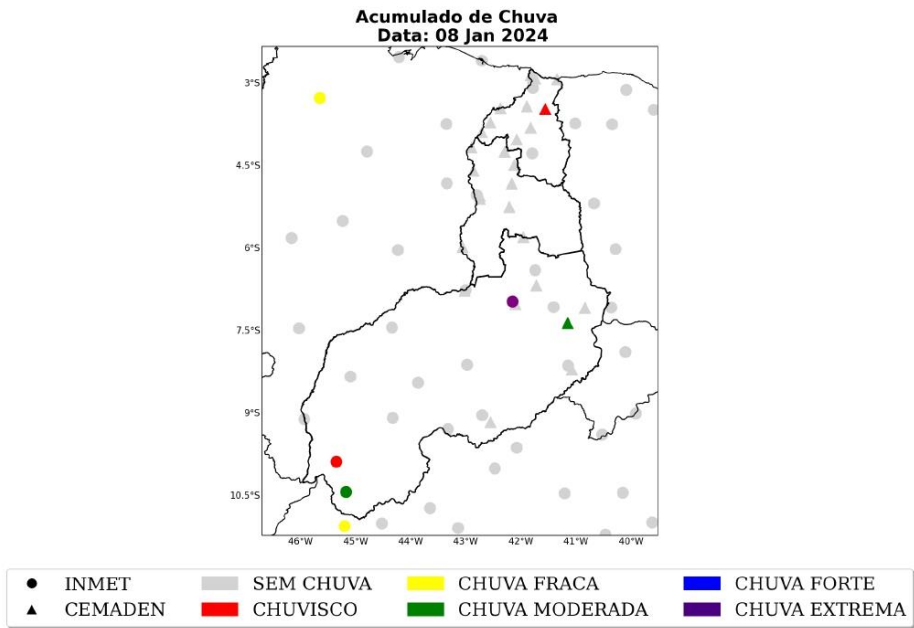
Figura 8: Acumulado diário de precipitação sobre a área de concessão da Equatorial-PI para o dia 08 de janeiro, baseado nas estações meteorológicas do INMET e CEMADEN.
