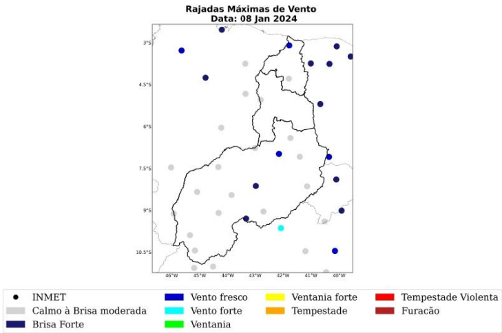
Figura 11: Máxima rajada de vento diária sobre a área de concessão da Equatorial-PI para o dia 08 de janeiro, baseado nas estações meteorológicas do INMET.
