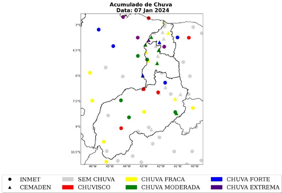
Figura 7: Acumulado diário de precipitação sobre a área de concessão da Equatorial-PI para o dia 07 de janeiro, baseado nas estações meteorológicas do INMET e CEMADEN.
