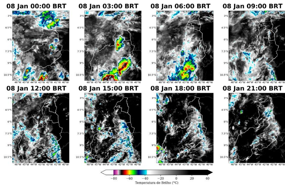
Figura 3: Imagens realçadas do satélite GOES-16 das 00 BRT até 21 BRT (a cada 3 horas) para o dia 08 de janeiro.
