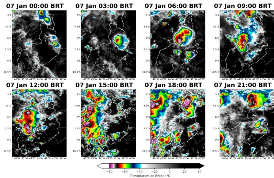
Figura 2: Imagens realçadas do satélite GOES-16 das 00 BRT até 21 BRT (a cada 3 horas) para o dia 07 de janeiro.
