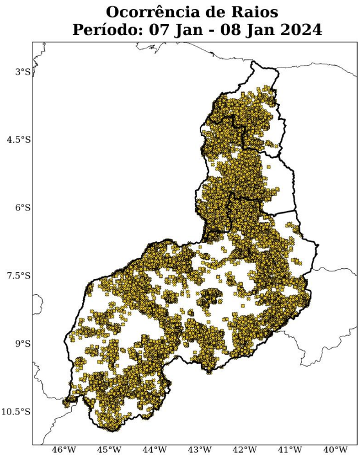
Figura 6: Total de descargas atmosféricas nuvem-solo detectadas pelo sistema Earth Networks durante o período de 07 a 08 de janeiro de 2024 sobre a área de concessão da Equatorial-PI.
