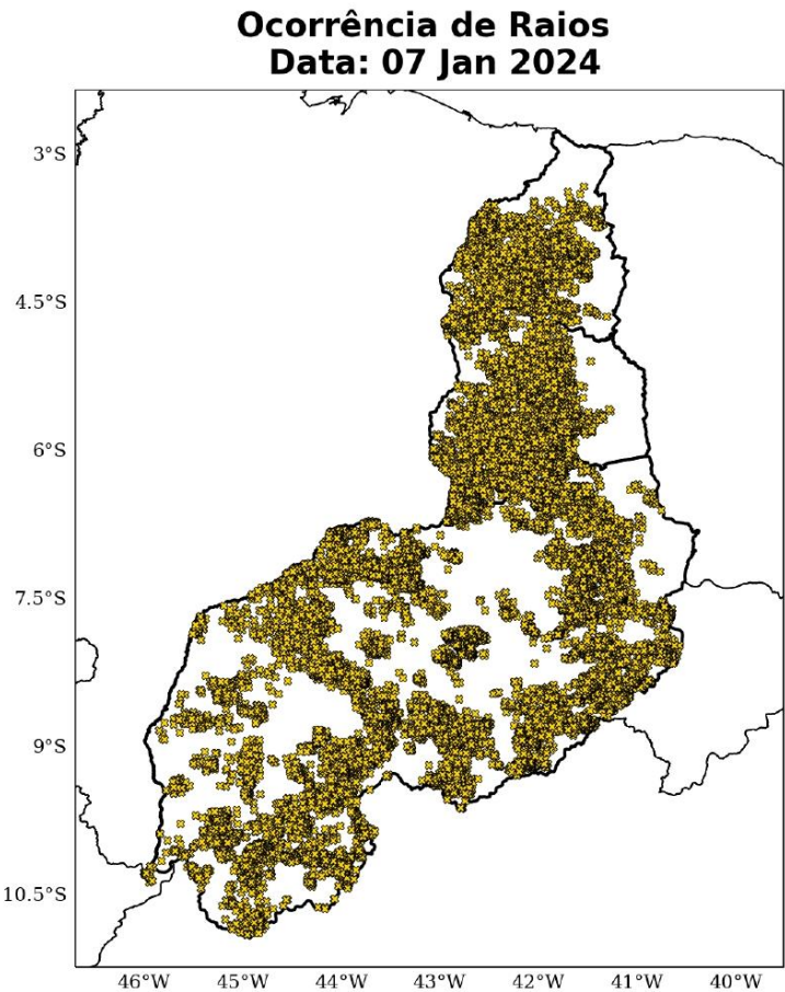
Figura 4: Densidade de descargas atmosféricas nuvem-solo detectadas pelo sistema Earth Networks para o dia 07 de janeiro sobre a área de concessão da Equatorial-PI.
