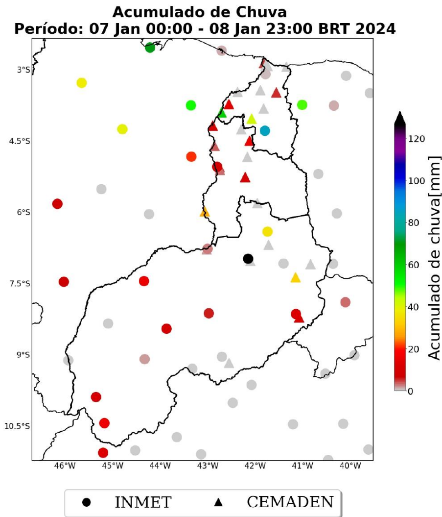
Figura 9: Acumulado de precipitação sobre o estado do Piauí para o período do evento (dias 07 a 08 de janeiro de 2024), baseado nas estações meteorológicas do INMET e CEMADEN.
