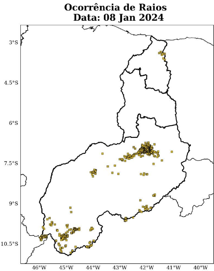
Figura 5: Densidade de descargas atmosféricas nuvem-solo detectadas pelo sistema Earth Networks para o dia 08 de janeiro sobre a área de concessão da Equatorial-PI.
