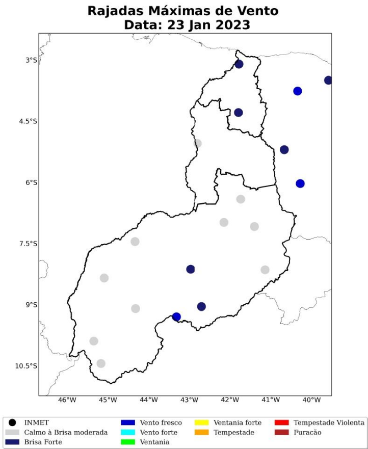
Figura 23: Máxima rajada de vento diária sobre a área de concessão da Equatorial-PI para o dia 23 de janeiro, baseado nas estações meteorológicas do INMET.
