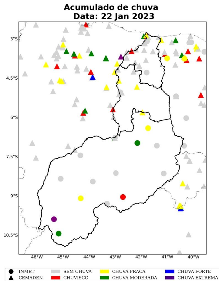
Figura 15: Acumulado diário de precipitação sobre a área de concessão da Equatorial-PI para o dia 22 de janeiro, baseado nas estações meteorológicas do INMET e CEMADEN.
