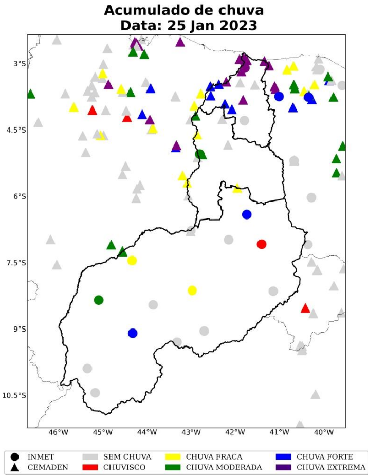
Figura 18: Acumulado diário de precipitação sobre a área de concessão da Equatorial-PI para o dia 25 de janeiro, baseado nas estações meteorológicas do INMET e CEMADEN.
