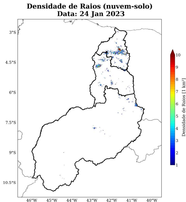
Figura 10: Densidade de descargas atmosféricas nuvem-solo detectadas pelo sistema Earth Networks para o dia 24 de janeiro sobre a área de concessão da Equatorial-PI.
