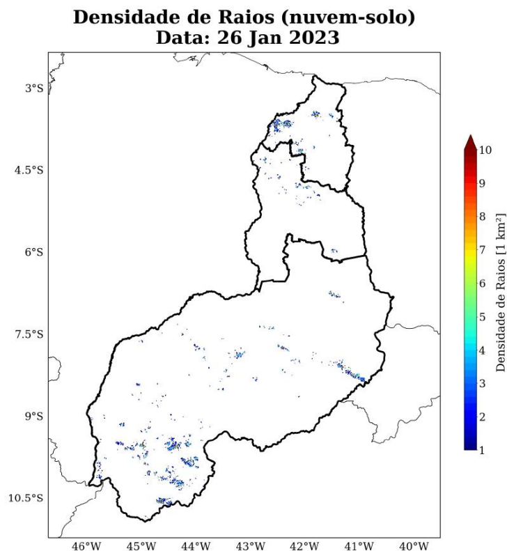
Figura 12: Densidade de descargas atmosféricas nuvem-solo detectadas pelo sistema Earth Networks para o dia 26 de janeiro sobre a área de concessão da Equatorial-PI.
