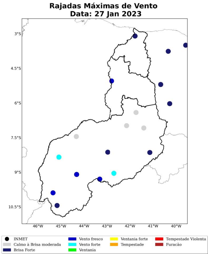
Figura 27: Máxima rajada de vento diária sobre a área de concessão da Equatorial-PI para o dia 27 de janeiro, baseado nas estações meteorológicas do INMET.
