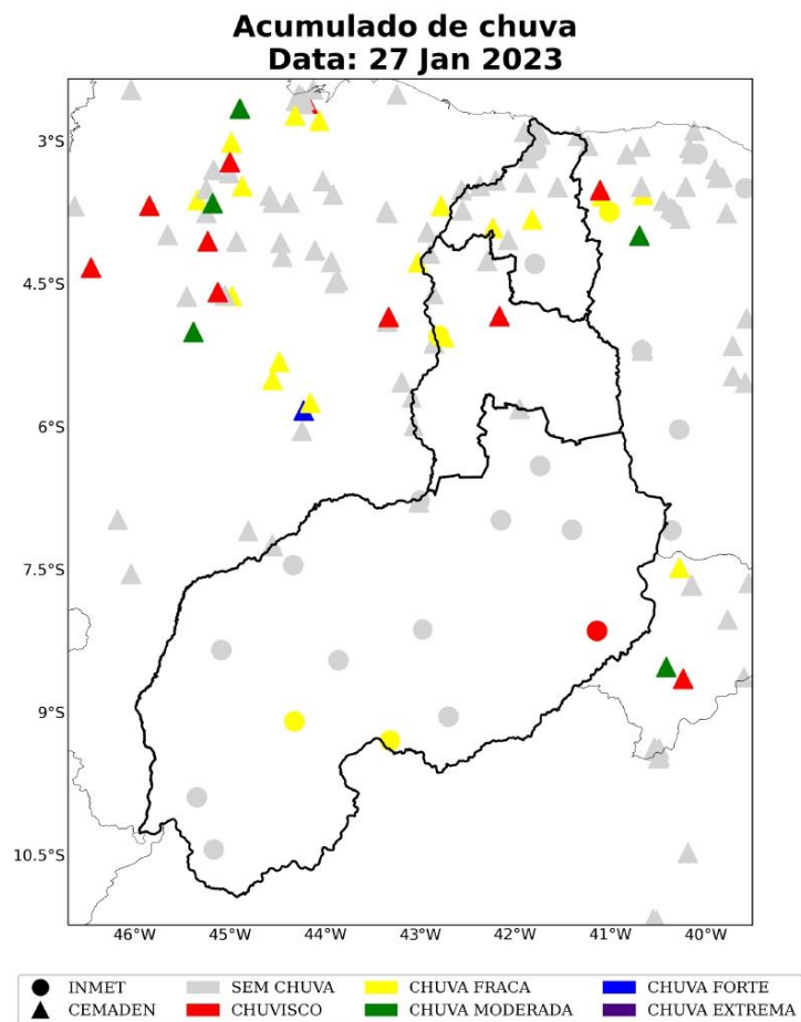
Figura 20: Acumulado diário de precipitação sobre a área de concessão da Equatorial-PI para o dia 27 de janeiro, baseado nas estações meteorológicas do INMET e CEMADEN.
