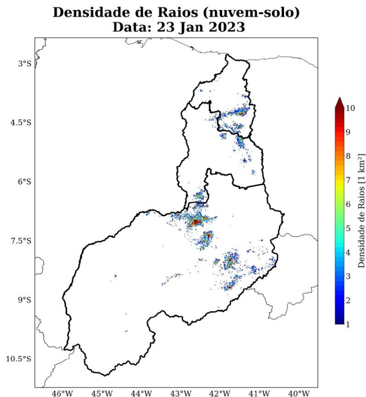
Figura 9: Densidade de descargas atmosféricas nuvem-solo detectadas pelo sistema Earth Networks para o dia 23 de janeiro sobre a área de concessão da Equatorial-PI.
