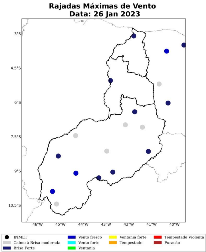
Figura 26: Máxima rajada de vento diária sobre a área de concessão da Equatorial-PI para o dia 26 de janeiro, baseado nas estações meteorológicas do INMET.
