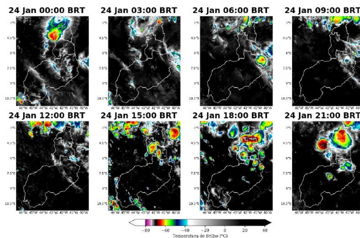
Figura 4: Imagens realçadas do satélite GOES-16 das 00 BRT até 21 BRT (a cada 3 horas) para o dia 24 de janeiro.
