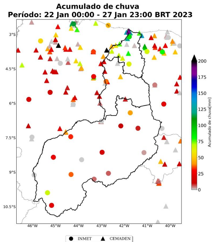
Figura 21: Acumulado de precipitação para o período 22 a 27 de janeiro de 2023 sobre a área de concessão da Equatorial-PI, baseado nas estações meteorológicas do INMET e CEMADEN.
