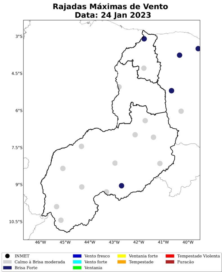
Figura 24: Máxima rajada de vento diária sobre a área de concessão da Equatorial-PI para o dia 24 de janeiro, baseado nas estações meteorológicas do INMET.
