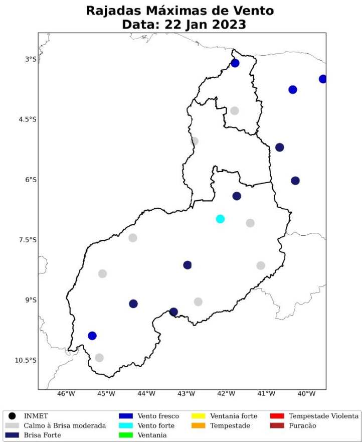
Figura 22: Máxima rajada de vento diária sobre a área de concessão da Equatorial-PI para o dia 22 de janeiro, baseado nas estações meteorológicas do INMET.
