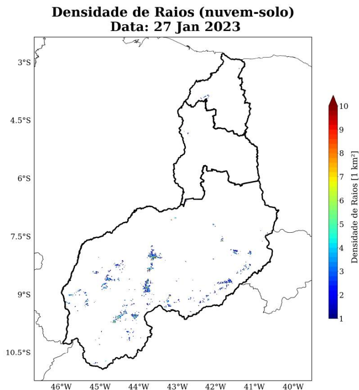
Figura 13: Densidade de descargas atmosféricas nuvem-solo detectadas pelo sistema Earth Networks para o dia 27 de janeiro sobre a área de concessão da Equatorial-PI.
