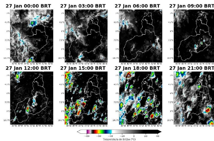
Figura 7: Imagens realçadas do satélite GOES-16 das 00 BRT até 21 BRT (a cada 3 horas) para o dia 27 de janeiro.
