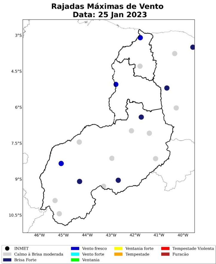
Figura 25: Máxima rajada de vento diária sobre a área de concessão da Equatorial-PI para o dia 25 de janeiro, baseado nas estações meteorológicas do INMET.
