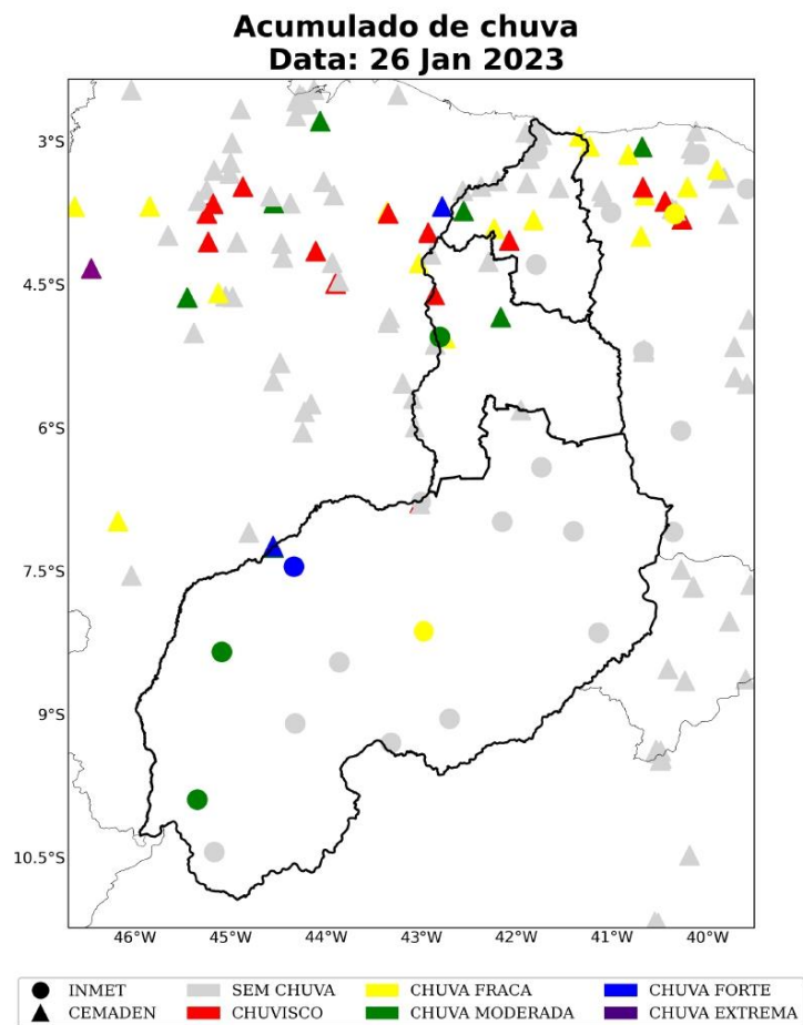
Figura 19: Acumulado diário de precipitação sobre a área de concessão da Equatorial-PI para o dia 26 de janeiro, baseado nas estações meteorológicas do INMET e CEMADEN.
