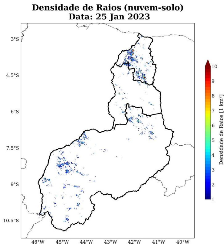
Figura 11: Densidade de descargas atmosféricas nuvem-solo detectadas pelo sistema Earth Networks para o dia 25 de janeiro sobre a área de concessão da Equatorial-PI.
