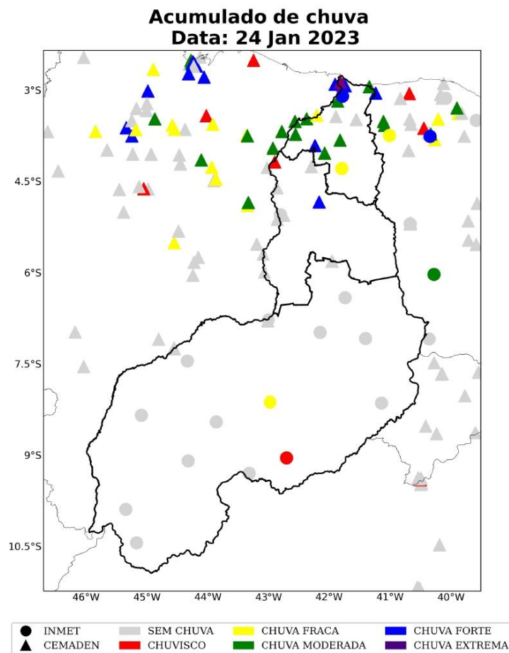
Figura 17: Acumulado diário de precipitação sobre a área de concessão da Equatorial-PI para o dia 24 de janeiro, baseado nas estações meteorológicas do INMET e CEMADEN.
