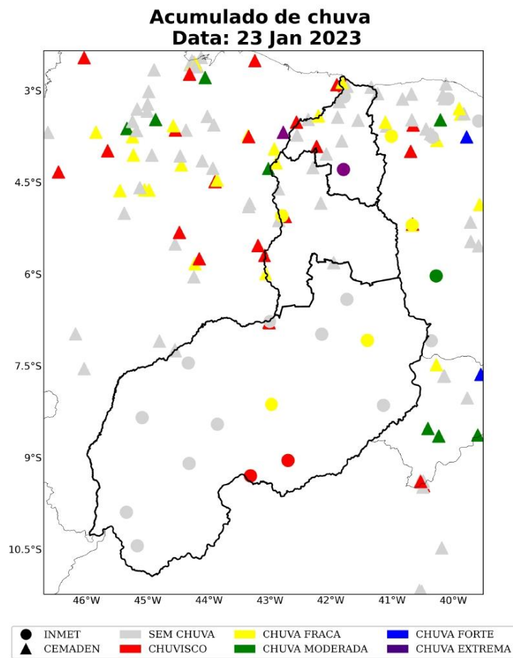
Figura 16: Acumulado diário de precipitação sobre a área de concessão da Equatorial-PI para o dia 23 de janeiro, baseado nas estações meteorológicas do INMET e CEMADEN.
