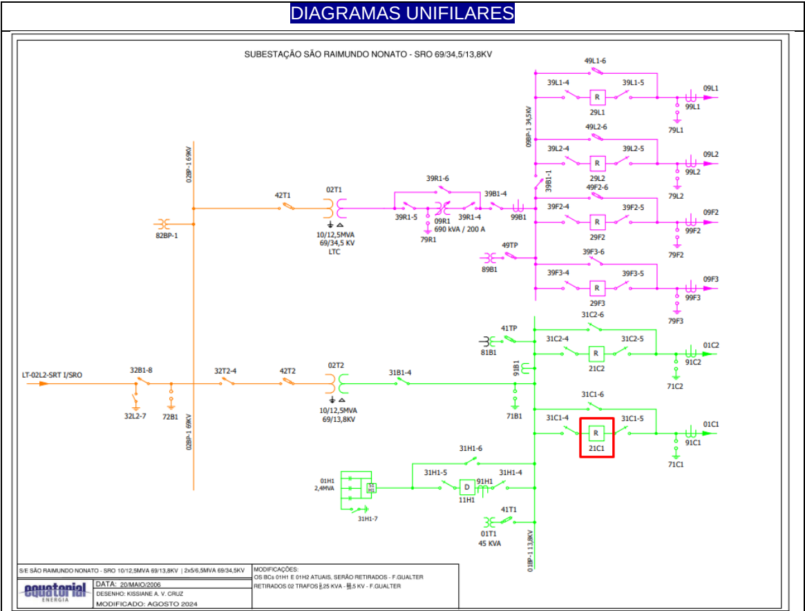
Figura 1 - Diagrama unifilar da subestação de São Raimundo Nonato
