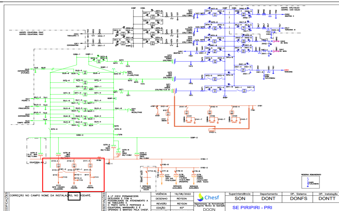
Figura 4 - Diagrama unifilar do sistema de distribuição da SE PRI
