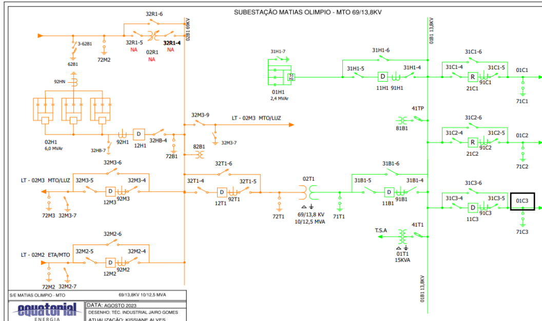
Figura 2 - Diagrama unifilar do sistema de distribuição da SE MTO
