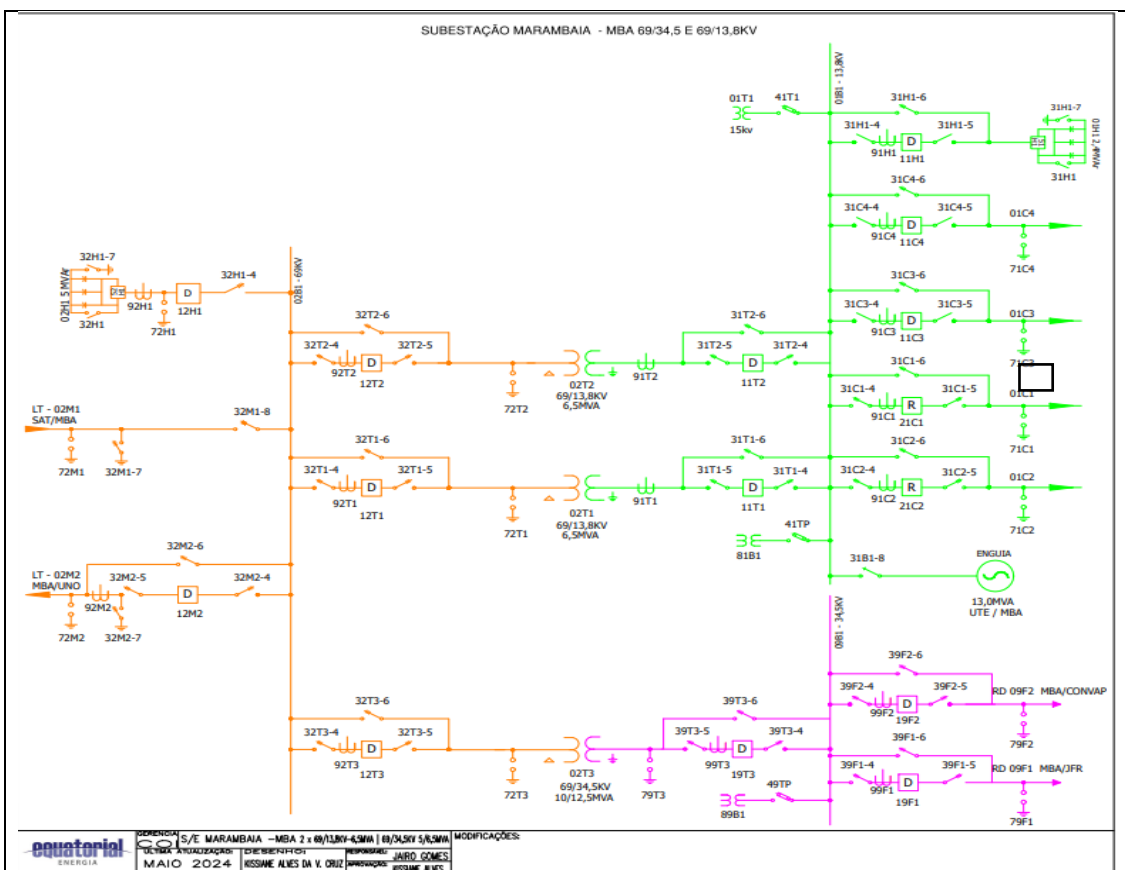
Figura 2 - Diagrama unifilar do sistema de distribuição da SE MBA
