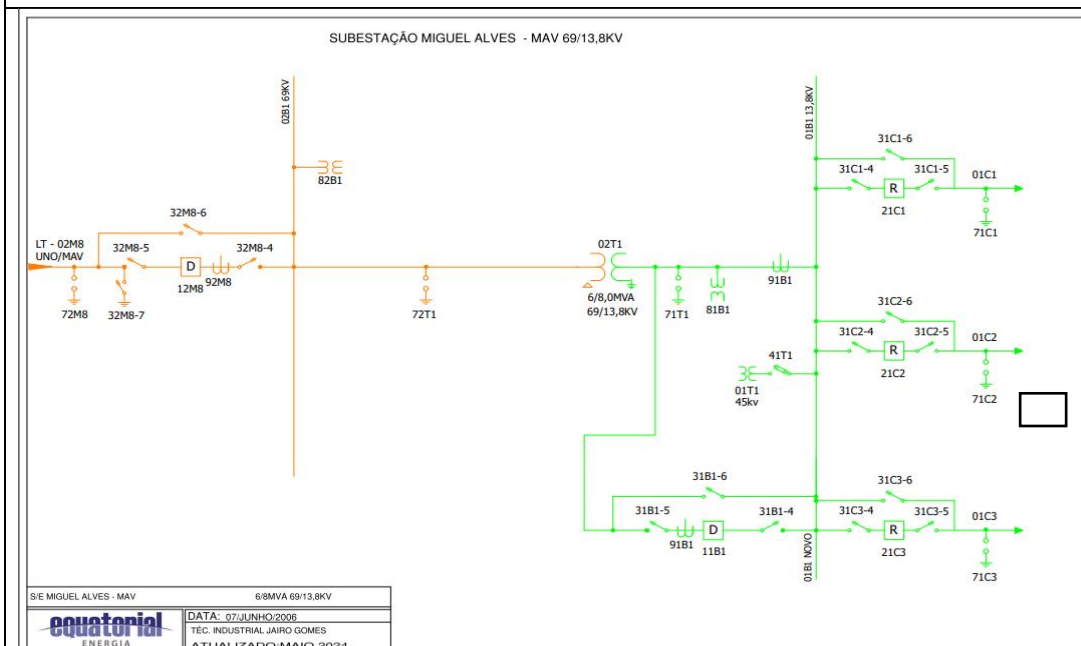
Figura 3 - Diagrama unifilar do sistema de distribuição da SE MAV
