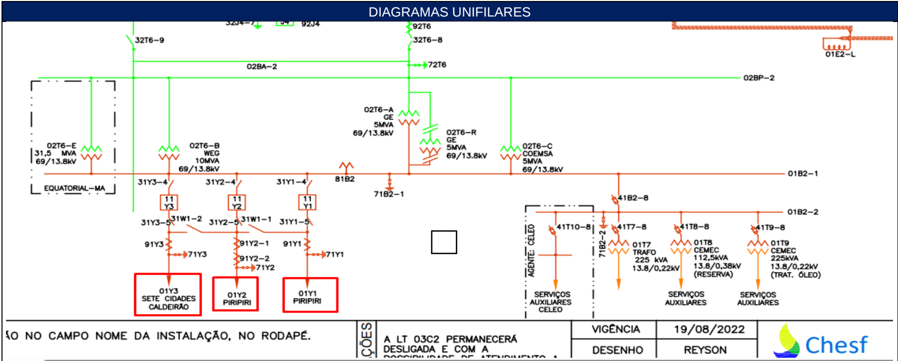
Figura 1 - Diagrama unifilar do sistema de distribuição da SE PRI
