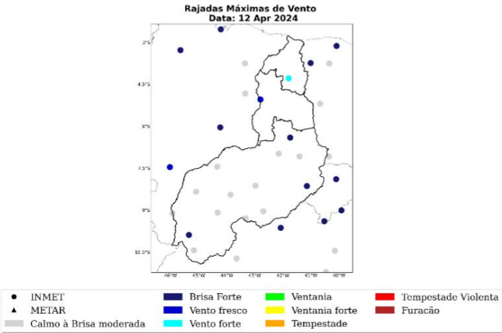
Figura 13: Máxima rajada de vento diária sobre a área de concessão da Equatorial-PI para o dia 12 de abril, baseado nas estações meteorológicas do INMET.
