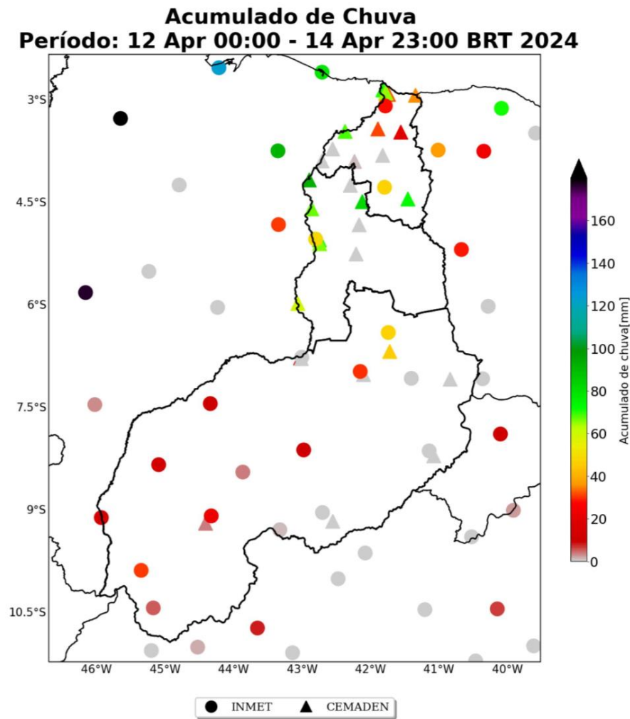
Figura 12: Acumulado de precipitação sobre o estado do Piauí para o período do evento (dias 12 a 14 de abril de 2024), baseado nas estações meteorológicas do INMET e CEMADEN.
