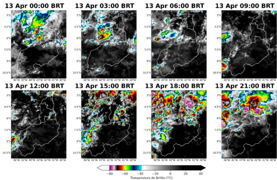
Figura 3: Imagens realçadas do satélite GOES-16 das 00 BRT até 21 BRT (a cada 3 horas) para o dia 13 de abril.
