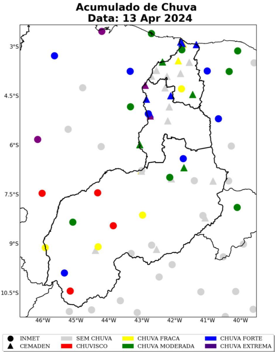
Figura 10: Acumulado diário de precipitação sobre a área de concessão da Equatorial-PI para o dia 13 de abril, baseado nas estações meteorológicas do INMET e CEMADEN.
