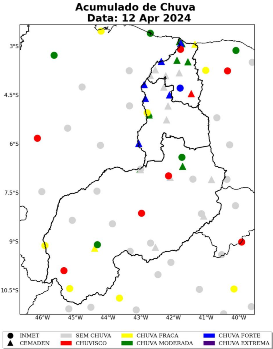
Figura 9: Acumulado diário de precipitação sobre a área de concessão da Equatorial-PI para o dia 12 de abril, baseado nas estações meteorológicas do INMET e CEMADEN.
