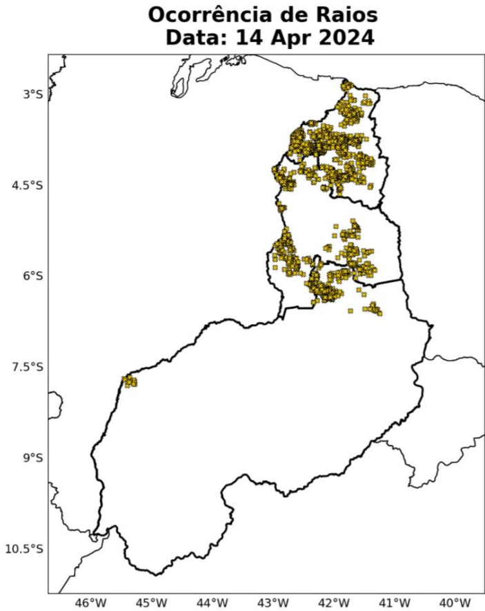
Figura 7: Ocorrências de descargas atmosféricas nuvem-solo detectadas pelo sistema Earth Networks para o dia 14 de abril sobre a área de concessão da Equatorial-PI.
