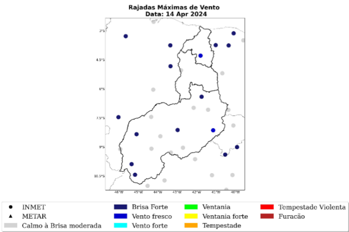
Figura 15: Máxima rajada de vento diária sobre a área de concessão da Equatorial-PI para o dia 14 de abril, baseado nas estações meteorológicas do INMET.
