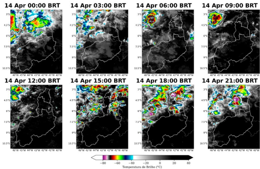
Figura 4: Imagens realçadas do satélite GOES-16 das 00 BRT até 21 BRT (a cada 3 horas) para o dia 14 de abril.
