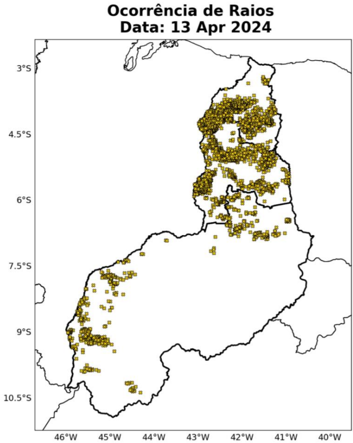
Figura 6: Ocorrências de descargas atmosféricas nuvem-solo detectadas pelo sistema Earth Networks para o dia 13 de abril sobre a área de concessão da Equatorial-PI.
