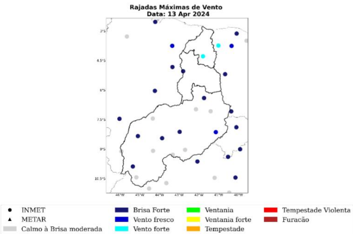
Figura 14: Máxima rajada de vento diária sobre a área de concessão da Equatorial-PI para o dia 13 de abril, baseado nas estações meteorológicas do INMET.
