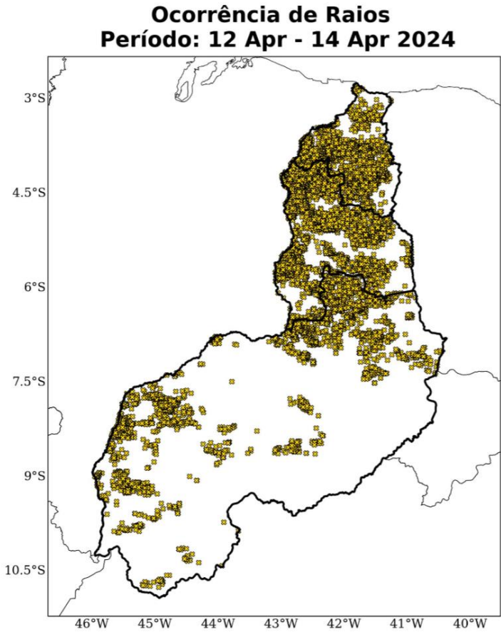
Figura 8: Total de descargas atmosféricas nuvem-solo detectadas pelo sistema Earth Networks durante o período de 12 a 14 de abril de 2024 sobre a área de concessão da Equatorial-PI.
