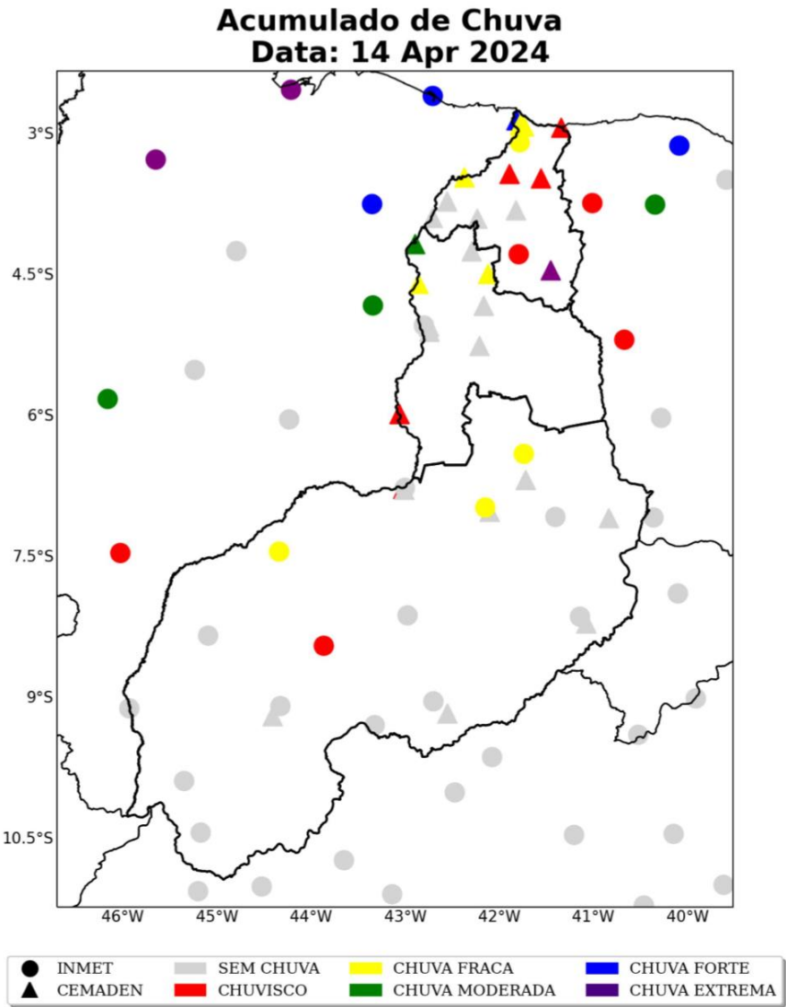
Figura 11: Acumulado diário de precipitação sobre a área de concessão da Equatorial-PI para o dia 14 de abril, baseado nas estações meteorológicas do INMET e CEMADEN.
