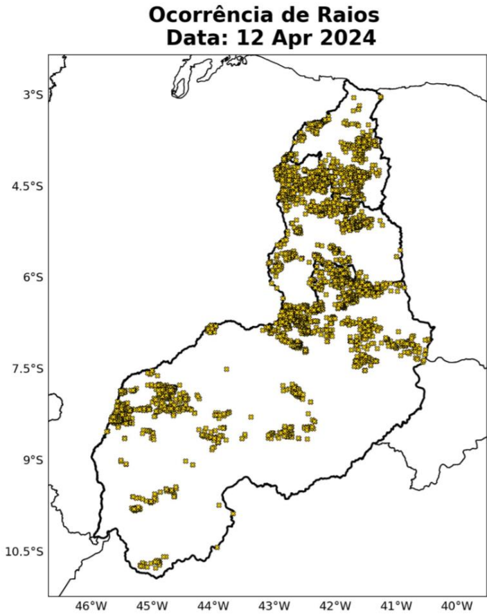
Figura 5: Ocorrências de descargas atmosféricas nuvem-solo detectadas pelo sistema Earth Networks para o dia 12 de abril sobre a área de concessão da Equatorial-PI.
