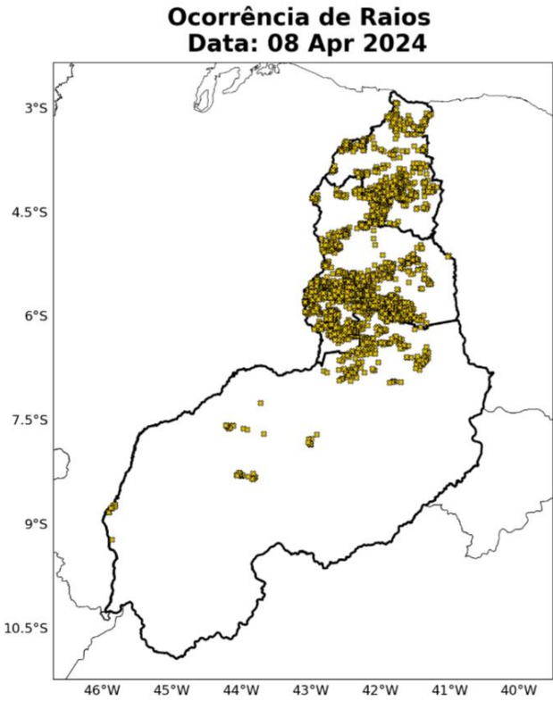
Figura 8: Ocorrências de descargas atmosféricas nuvem-solo detectadas pelo sistema Earth Networks para o dia 08 de abril sobre a área de concessão da Equatorial-PI.
