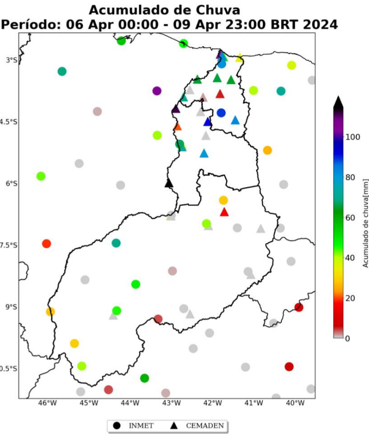
Figura 15: Acumulado de precipitação sobre o estado do Piauí para o período do evento (dias 06 a 09 de abril de 2024), baseado nas estações meteorológicas do INMET e CEMADEN.
