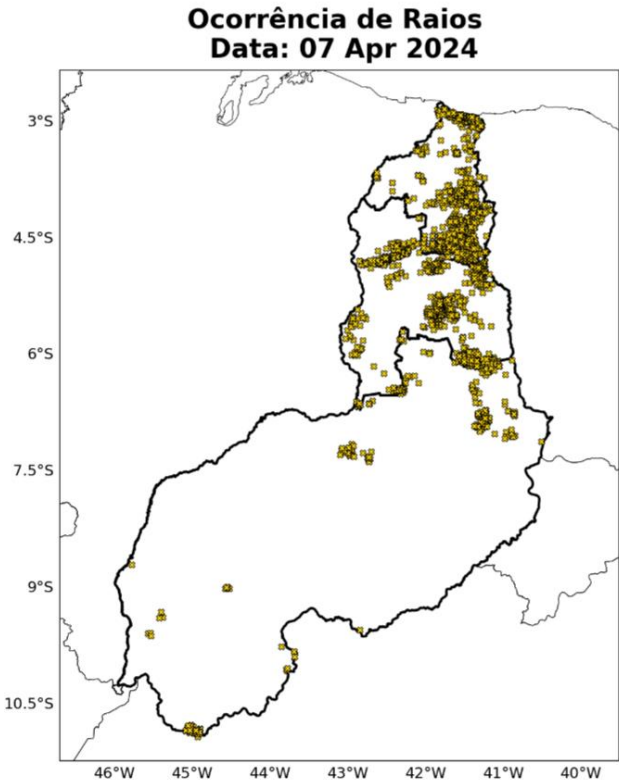
Figura 7: Ocorrências de descargas atmosféricas nuvem-solo detectadas pelo sistema Earth Networks para o dia 07 de abril sobre a área de concessão da Equatorial-PI.
