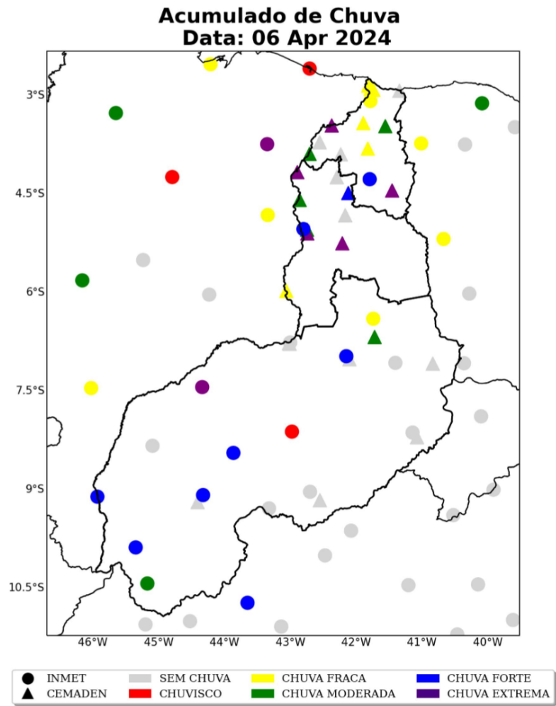
Figura 11: Acumulado diário de precipitação sobre a área de concessão da Equatorial-PI para o dia 06 de abril, baseado nas estações meteorológicas do INMET e CEMADEN.
