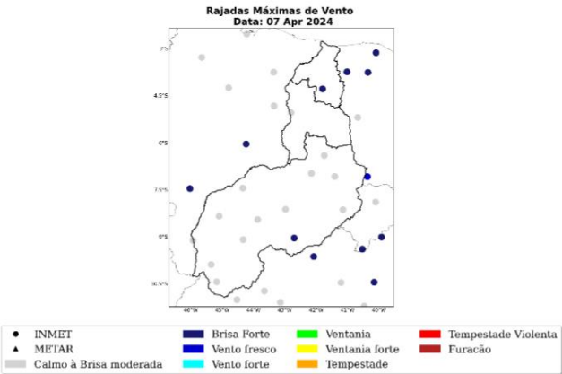
Figura 17: Máxima rajada de vento diária sobre a área de concessão da Equatorial-PI para o dia 07 de abril, baseado nas estações meteorológicas do INMET.
