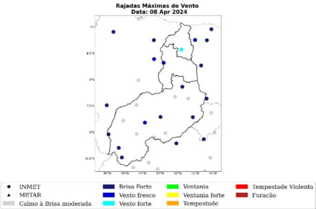
Figura 18: Máxima rajada de vento diária sobre a área de concessão da Equatorial-PI para o dia 08 de abril, baseado nas estações meteorológicas do INMET.
