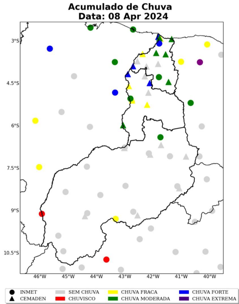
Figura 13: Acumulado diário de precipitação sobre a área de concessão da Equatorial-PI para o dia 08 de abril, baseado nas estações meteorológicas do INMET e CEMADEN.
