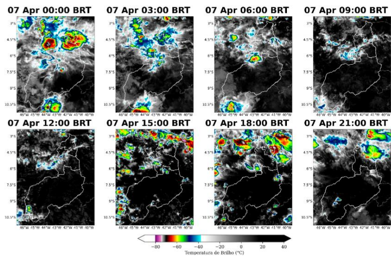
Figura 3: Imagens realçadas do satélite GOES-16 das 00 BRT até 21 BRT (a cada 3 horas) para o dia 07 de abril.
