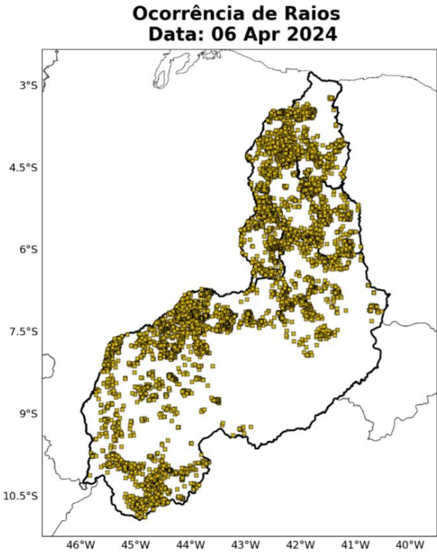
Figura 6: Ocorrências de descargas atmosféricas nuvem-solo detectadas pelo sistema Earth Networks para o dia 06 de abril sobre a área de concessão da Equatorial-PI.
