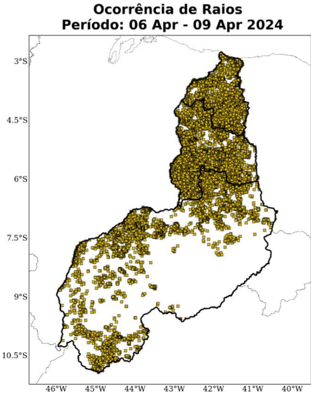
Figura 10: Total de descargas atmosféricas nuvem-solo detectadas pelo sistema Earth Networks durante o período de 06 a 09 de abril de 2024 sobre a área de concessão da Equatorial-PI.
