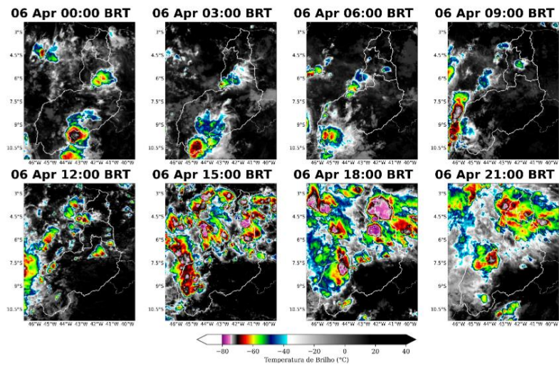
Figura 2: Imagens realçadas do satélite GOES-16 das 00 BRT até 21 BRT (a cada 3 horas) para o dia 06 de abril.
