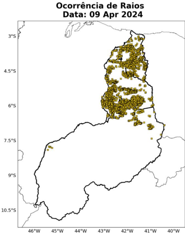
Figura 9: Ocorrências de descargas atmosféricas nuvem-solo detectadas pelo sistema Earth Networks para o dia 09 de abril sobre a área de concessão da Equatorial-PI.
