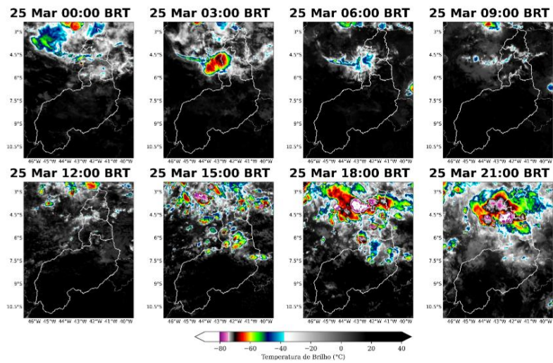
Figura 2: Imagens realçadas do satélite GOES-16 das 00 BRT até 21 BRT (a cada 3 horas) para o dia 25 de março.
