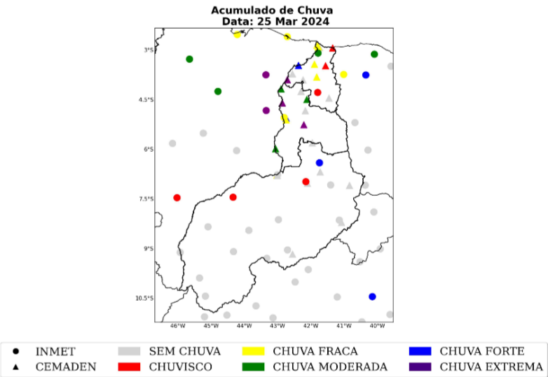
Figura 9: Acumulado diário de precipitação sobre a área de concessão da Equatorial-PI para o dia 25 de março, baseado nas estações meteorológicas do INMET e CEMADEN.
