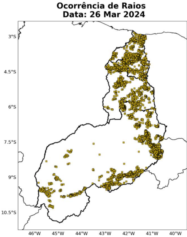
Figura 6: Ocorrências de descargas atmosféricas nuvem-solo detectadas pelo sistema Earth Networks para o dia 26 de março sobre a área de concessão da Equatorial-PI.
