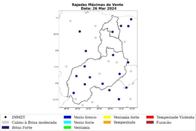
Figura 14: Máxima rajada de vento diária sobre a área de concessão da Equatorial-PI para o dia 26 de março, baseado nas estações meteorológicas do INMET.
