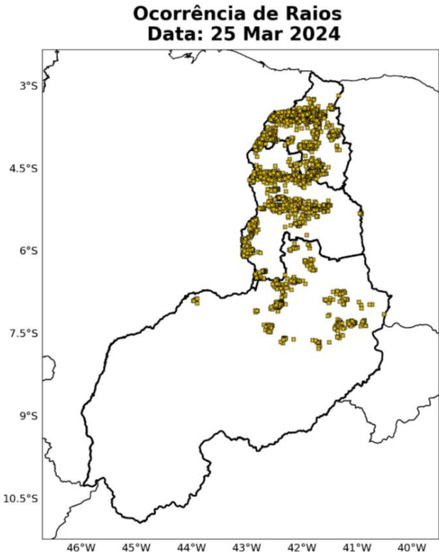
Figura 5: Ocorrências de descargas atmosféricas nuvem-solo detectadas pelo sistema Earth Networks para o dia 25 de março sobre a área de concessão da Equatorial-PI.
