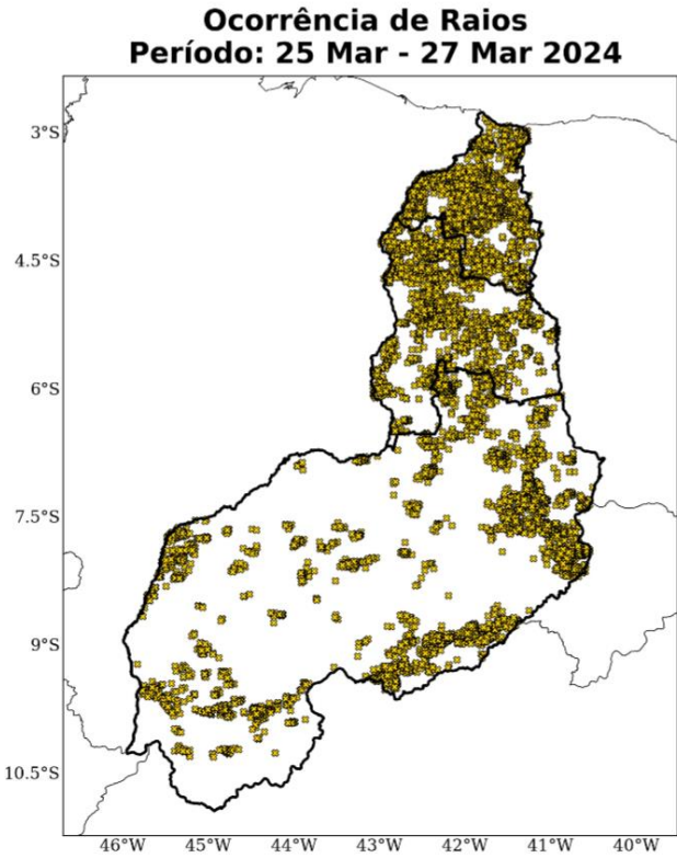
Figura 8: Total de descargas atmosféricas nuvem-solo detectadas pelo sistema Earth Networks durante o período de 25 a 27 de março de 2024 sobre a área de concessão da Equatorial-PI.
