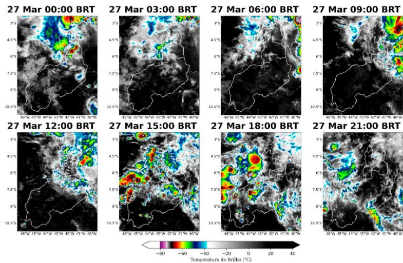
Figura 4: Imagens realçadas do satélite GOES-16 das 00 BRT até 21 BRT (a cada 3 horas) para o dia 27 de março.
