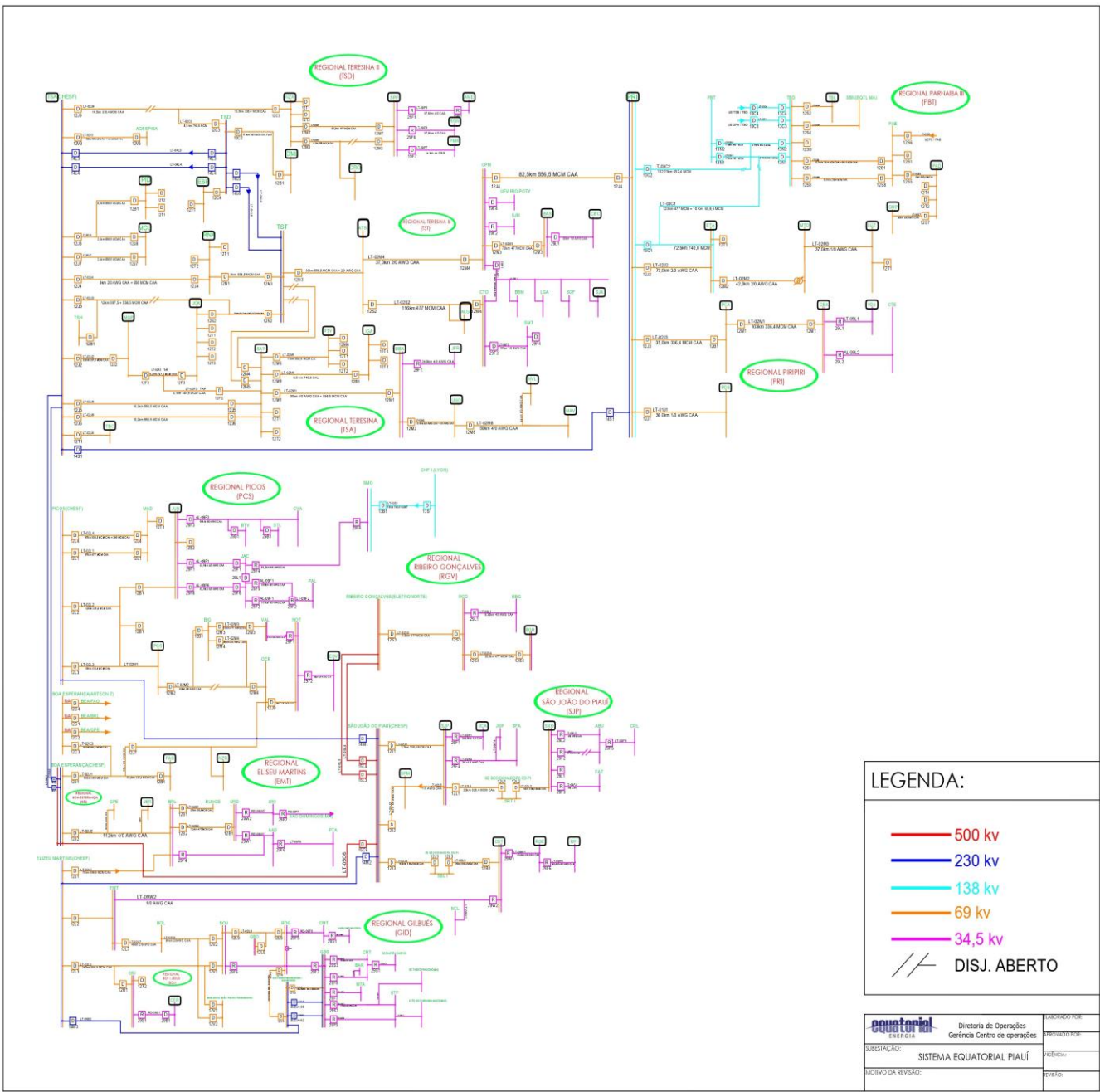
Figura 3 – Diagrama unifilar do sistema de distribuição da Equatorial Piauí
