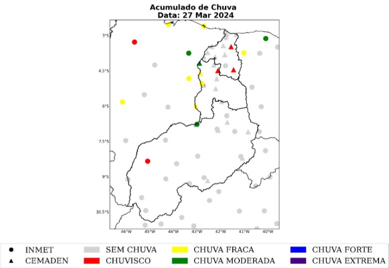
Figura 11: Acumulado diário de precipitação sobre a área de concessão da Equatorial-PI para o dia 27 de março, baseado nas estações meteorológicas do INMET e CEMADEN.
