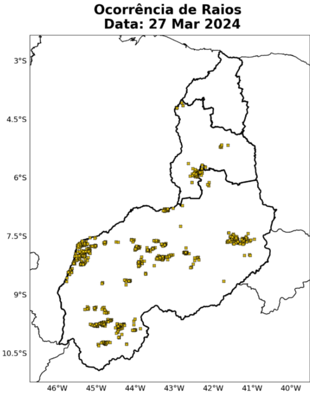
Figura 7: Ocorrências de descargas atmosféricas nuvem-solo detectadas pelo sistema Earth Networks para o dia 27 de março sobre a área de concessão da Equatorial-PI.
