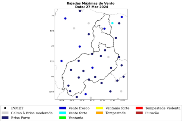
Figura 15: Máxima rajada de vento diária sobre a área de concessão da Equatorial-PI para o dia 27 de março, baseado nas estações meteorológicas do INMET.
