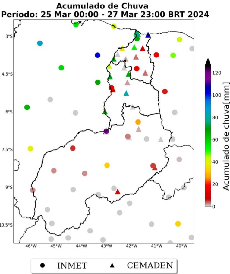
Figura 12: Acumulado de precipitação sobre o estado do Piauí para o período do evento (dias 25 a 27 de março de 2024), baseado nas estações meteorológicas do INMET e CEMADEN.
