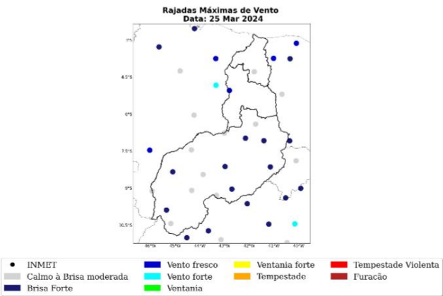
Figura 13: Máxima rajada de vento diária sobre a área de concessão da Equatorial-PI para o dia 25 de março, baseado nas estações meteorológicas do INMET.
