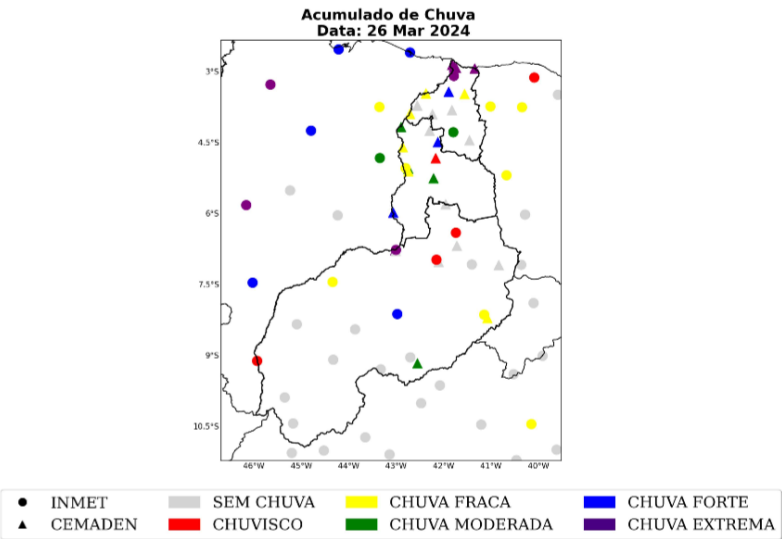
Figura 10: Acumulado diário de precipitação sobre a área de concessão da Equatorial-PI para o dia 26 de março, baseado nas estações meteorológicas do INMET e CEMADEN.
