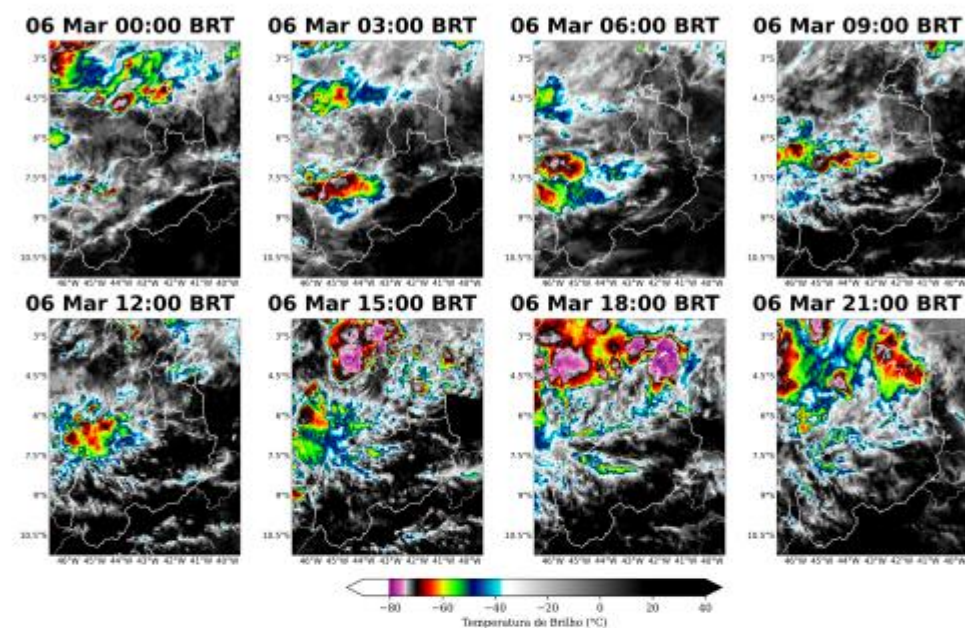
Figura 5: Imagens realçadas do satélite GOES-16 das 00 BRT até 21 BRT (a cada 3 horas) para o dia 06 de Março.
