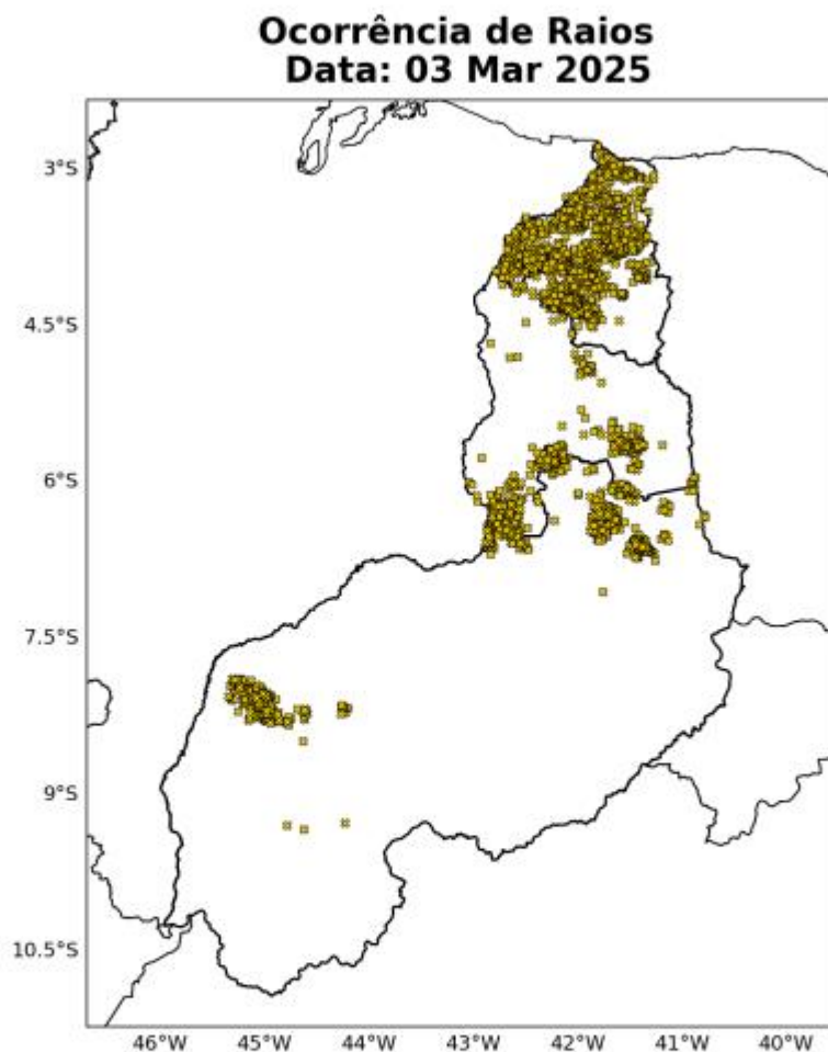
Figura 7: Ocorrências de descargas atmosféricas nuvem-solo detectadas pelo sistema Earth Networks para o dia 03 de Março sobre a área de concessão da Equatorial-PI.
