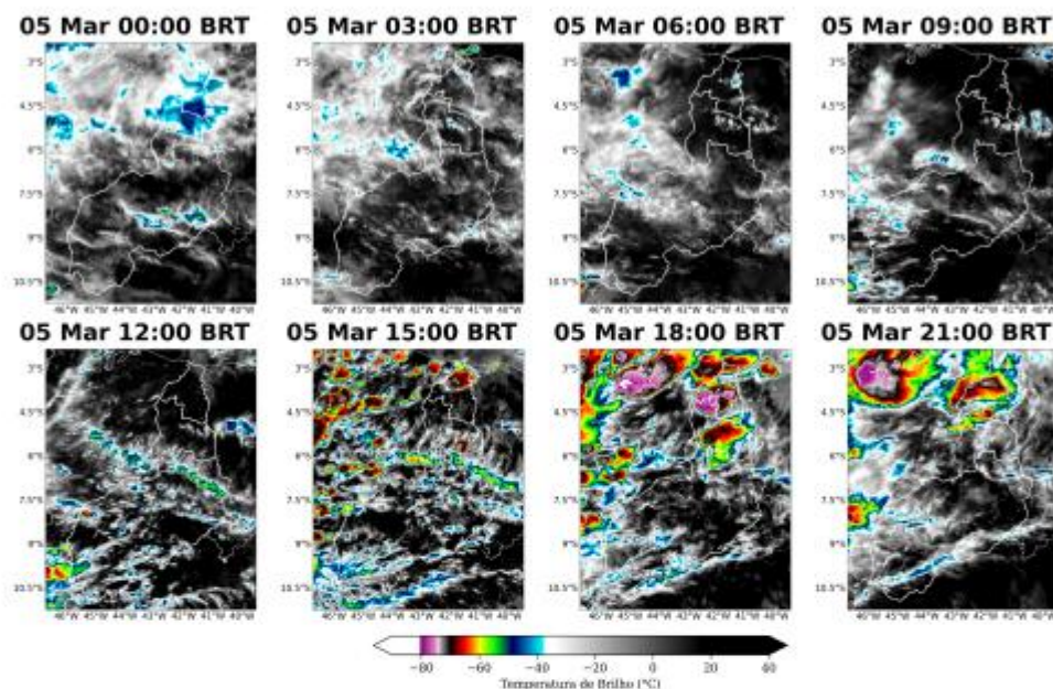
Figura 4: Imagens realçadas do satélite GOES-16 das 00 BRT até 21 BRT (a cada 3 horas) para o dia 05 de Março.
