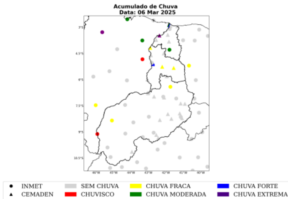
Figura 16: Acumulado diário de precipitação sobre a área de concessão da Equatorial-PI para o dia 06 de Março, baseado nas estações meteorológicas do INMET e CEMADEN.
