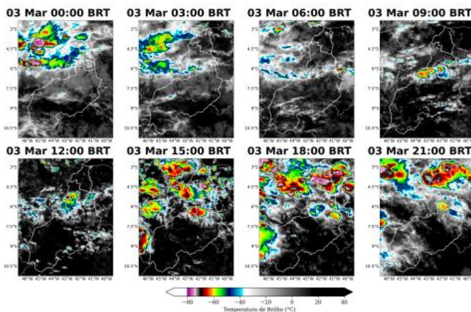
Figura 2: Imagens realçadas do satélite GOES-16 das 00 BRT até 21 BRT (a cada 3 horas) para o dia 03 de Março.
