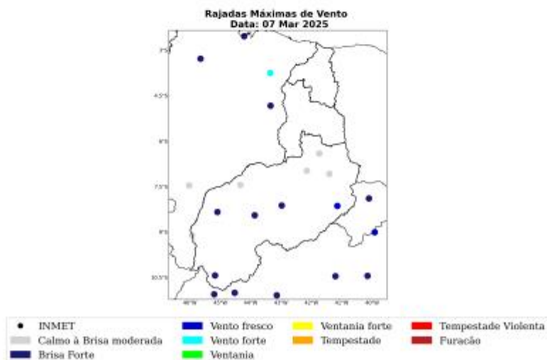
Figura 23: Máxima rajada de vento diária sobre a área de concessão da Equatorial-PI para o dia 07 de Março, baseado nas estações meteorológicas do INMET.
