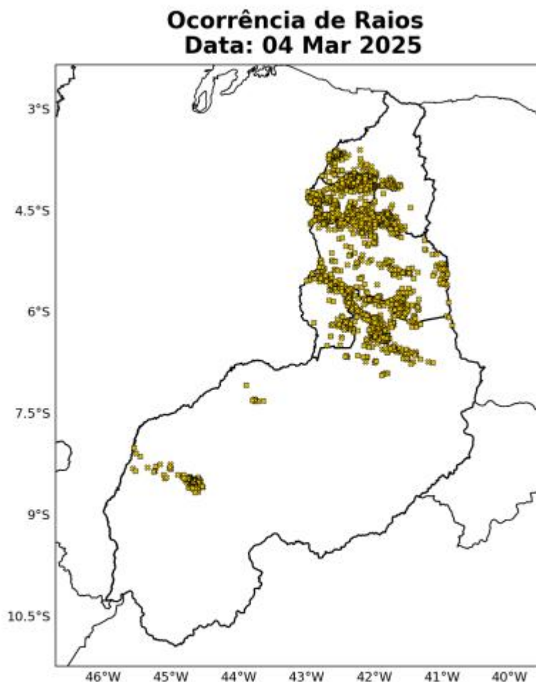
Figura 8: Ocorrências de descargas atmosféricas nuvem-solo detectadas pelo sistema Earth Networks para o dia 04 de Março sobre a área de concessão da Equatorial-PI.
