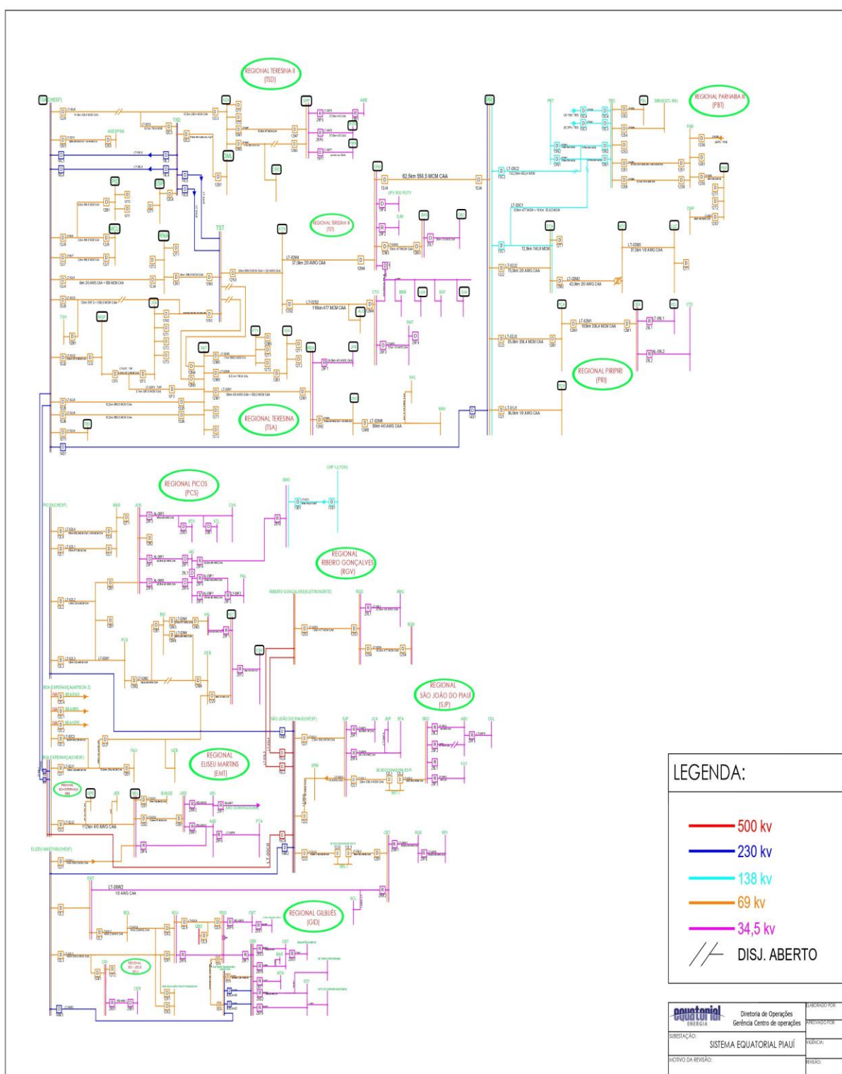
Figura 3 - Diagrama unifilar concessão Piauí
