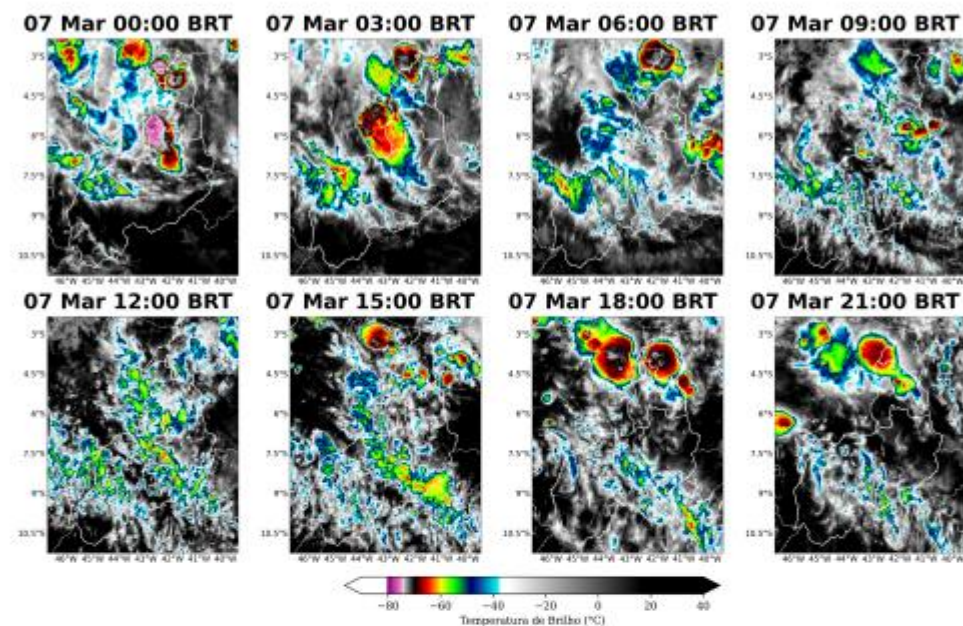
Figura 6: Imagens realizadas do satélite GOES-16 das 00 BRT até 21 BRT (a cada 3 horas) para o dia 07 de Março.
