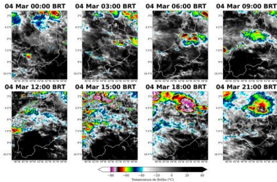
Figura 3: Imagens realçadas do satélite GOES-16 das 00 BRT até 21 BRT (a cada 3 horas) para o dia 04 de Março.
