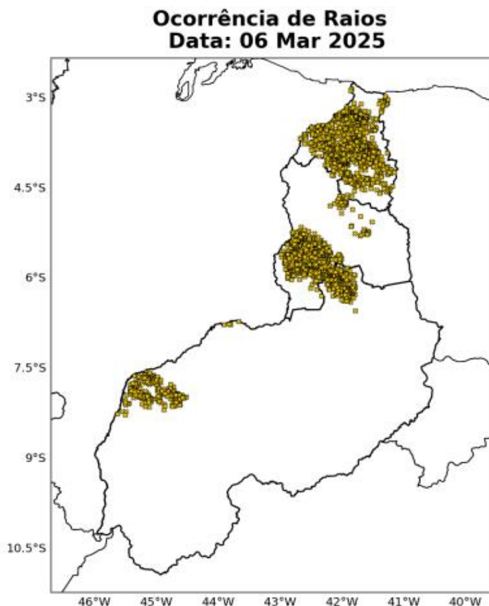
Figura 10: Ocorrências de descargas atmosféricas nuvem-solo detectadas pelo sistema Earth Networks para o dia 06 de Março sobre a área de concessão da Equatorial-PI.
