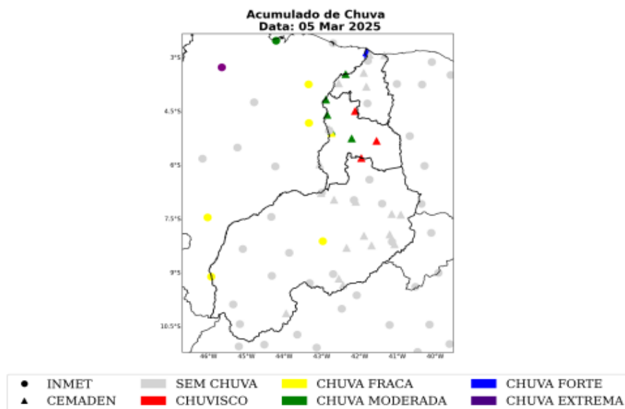
Figura 15: Acumulado diário de precipitação sobre a área de concessão da Equatorial-PI para o dia 05 de Março, baseado nas estações meteorológicas do INMET e CEMADEN.
