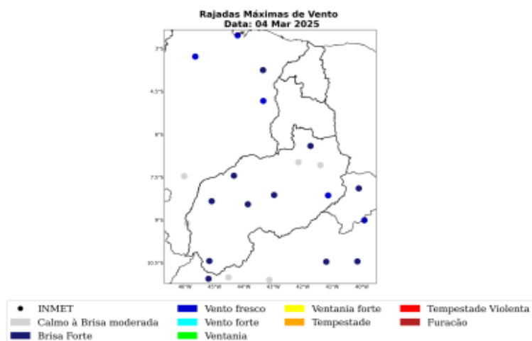
Figura 20: Máxima rajada de vento diária sobre a área de concessão da Equatorial-PI para o dia 04 de Março, baseado nas estações meteorológicas do INMET.
