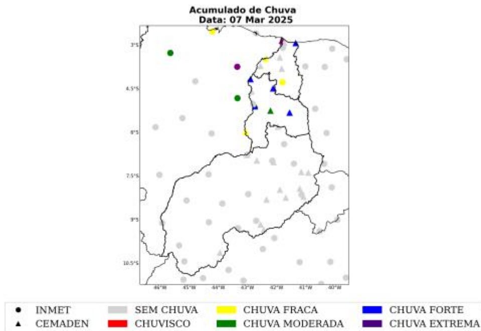
Figura 17: Acumulado diário de precipitação sobre a área de concessão da Equatorial-PI para o dia 07 de Março, baseado nas estações meteorológicas do INMET e CEMADEN.
