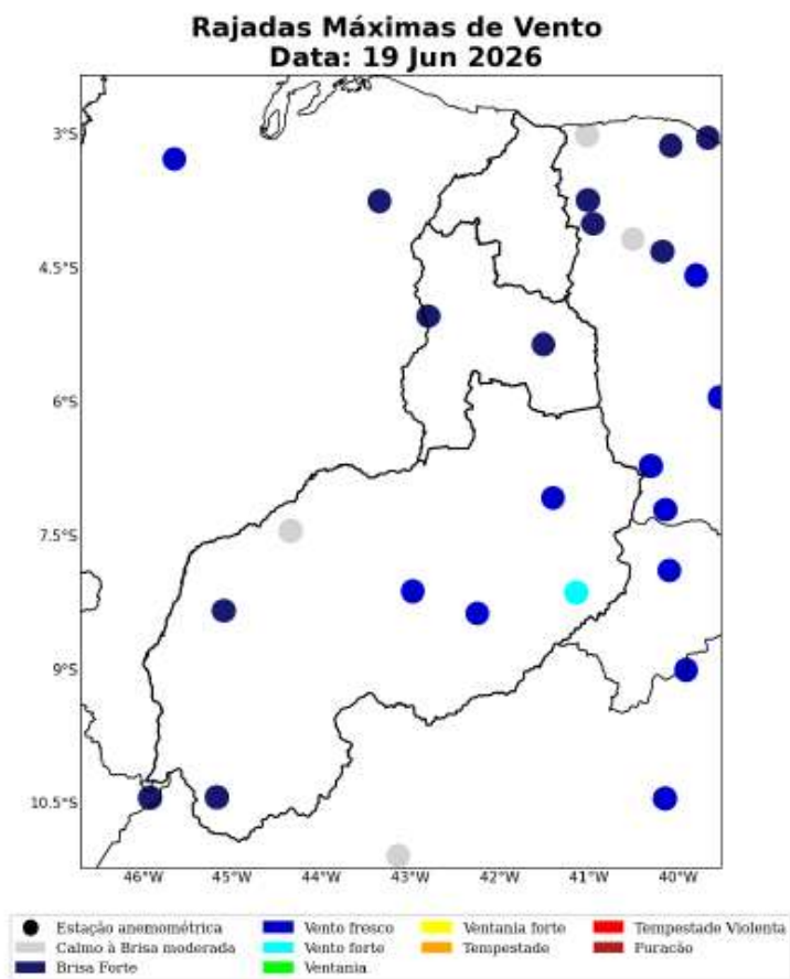
Figura 40: Máxima rajada de vento diária sobre a área de concessão da Equatorial-PI para o dia 19 de Junho, baseado nas estações meteorológicas do INMET.
