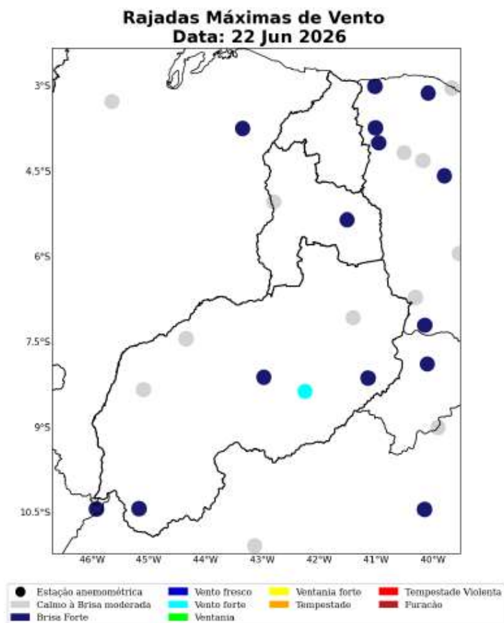
Figura 43: Máxima rajada de vento diária sobre a área de concessão da Equatorial-PI para o dia 22 de Junho, baseado nas estações meteorológicas do INMET.
