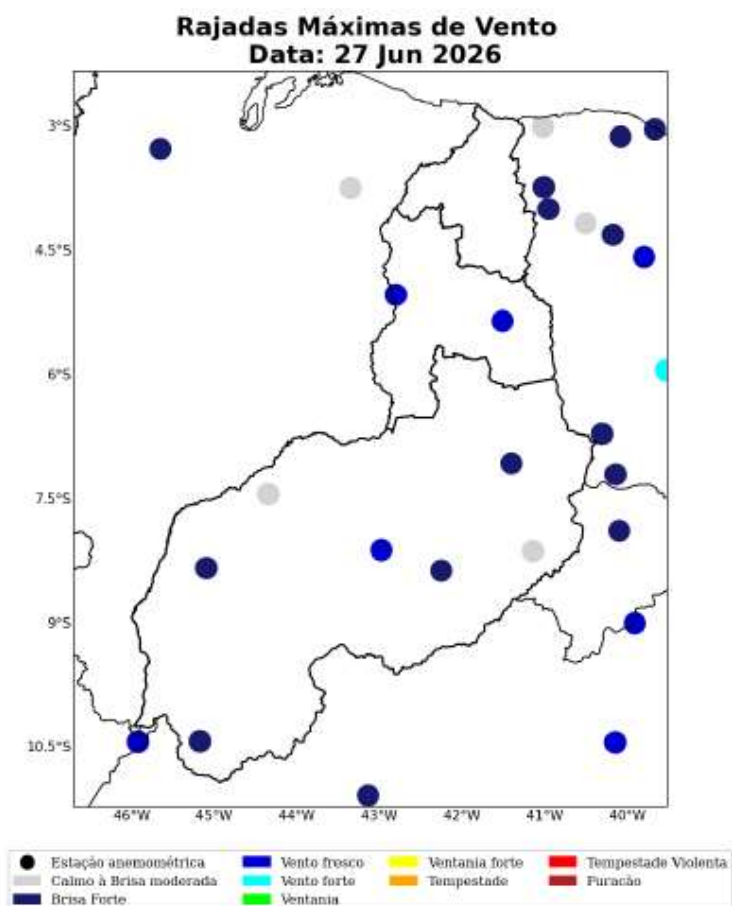
Figura 48: Máxima rajada de vento diária sobre a área de concessão da Equatorial-PI para o dia 27 de Junho, baseado nas estações meteorológicas do INMET.
