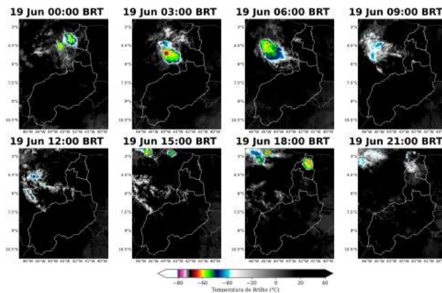
Figura 4: Imagens realçadas do satélite GOES-19 das 00 BRT até 21 BRT (a cada 3 horas) para o dia 19 de Junho.
