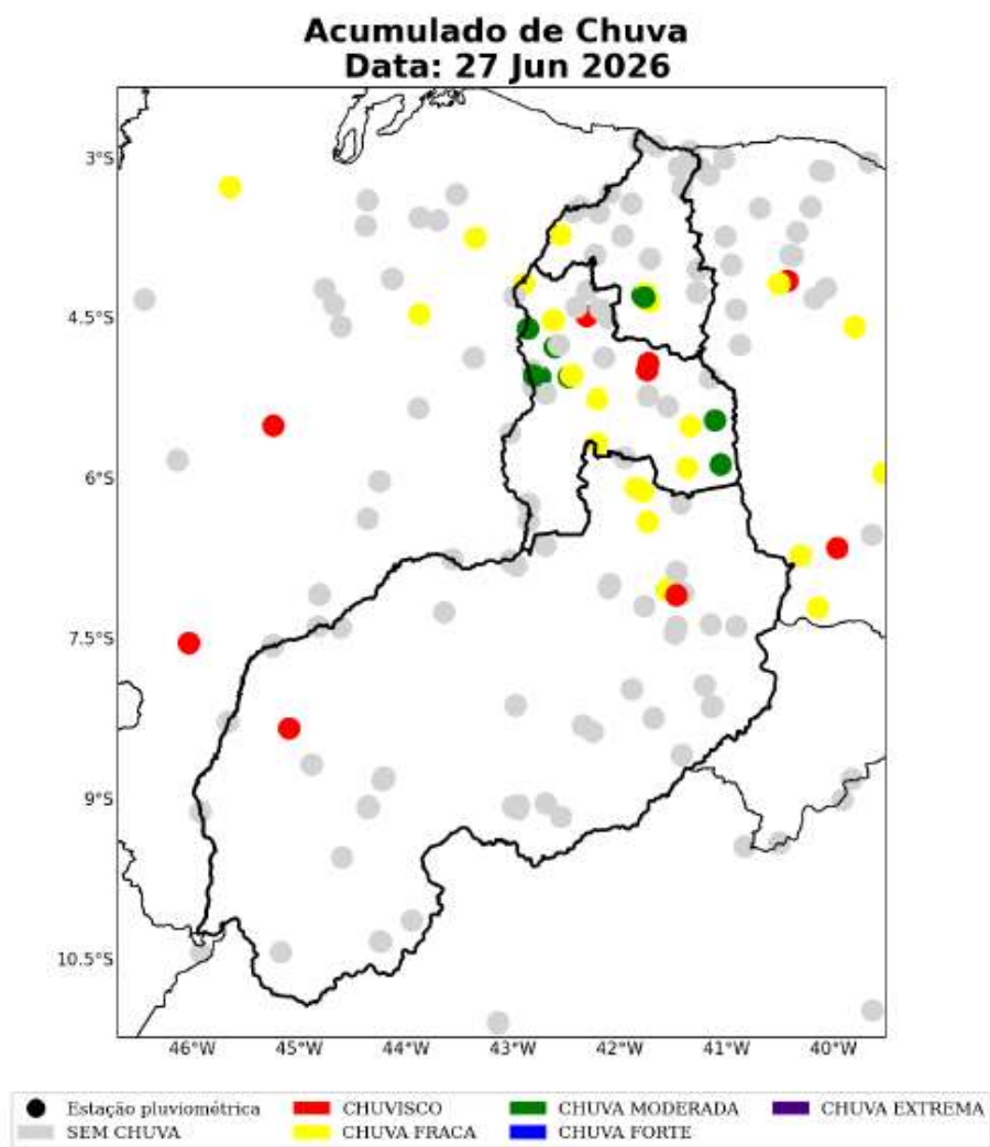
Figura 34: Acumulado diário de precipitação sobre a área de concessão da Equatorial-PI para o dia 27 de Junho, baseado nas estações meteorológicas do INMET e CEMADEN.
