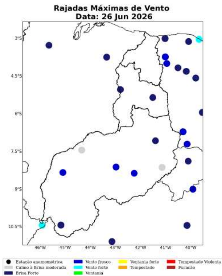
Figura 47: Máxima rajada de vento diária sobre a área de concessão da Equatorial-PI para o dia 26 de Junho, baseado nas estações meteorológicas do INMET.
