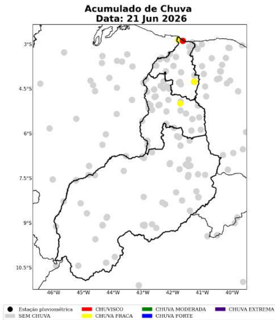
Figura 28: Acumulado diário de precipitação sobre a área de concessão da Equatorial-PI para o dia 21 de Junho, baseado nas estações meteorológicas do INMET e CEMADEN.
