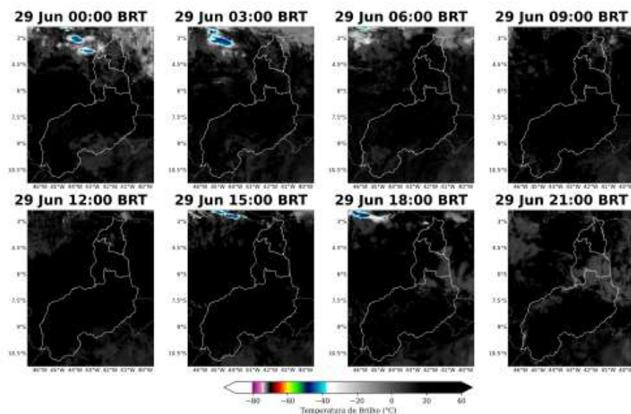
Figura 14: Imagens realçadas do satélite GOES-19 das 00 BRT até 21 BRT (a cada 3 horas) para o dia 29 de Junho.
