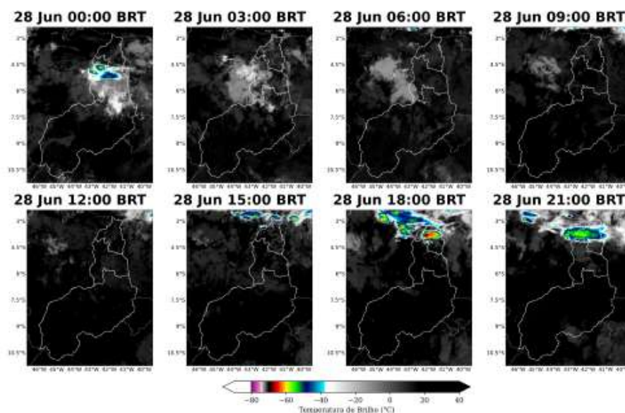
Figura 13: Imagens realçadas do satélite GOES-19 das 00 BRT até 21 BRT (a cada 3 horas) para o dia 28 de Junho.
