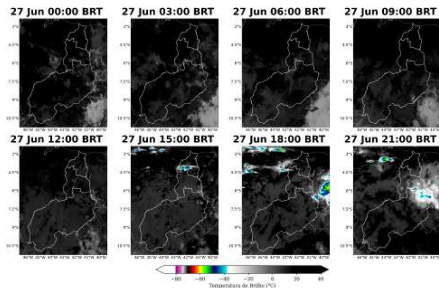
Figura 12: Imagens reagçadas dos satélite GOES-19 das 00 BRT até 21 BRT (a cada 3 horas) para o dia 27 de Junho.
