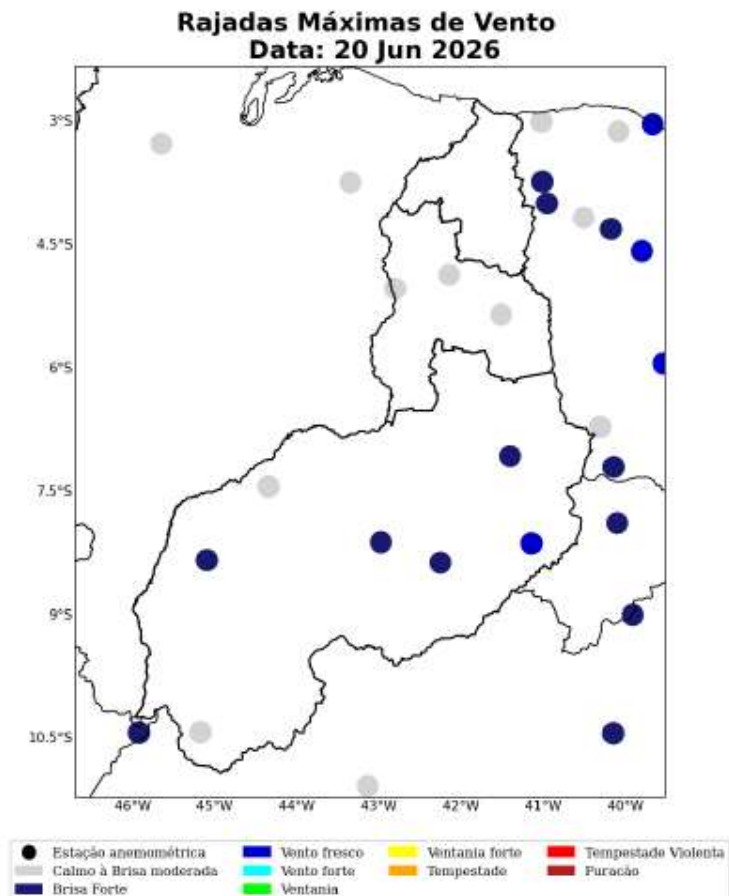
Figura 41: Máxima rajada de vento diária sobre a área de concessão da Equatorial-PI para o dia 20 de Junho, baseado nas estações meteorológicas do INMET.
