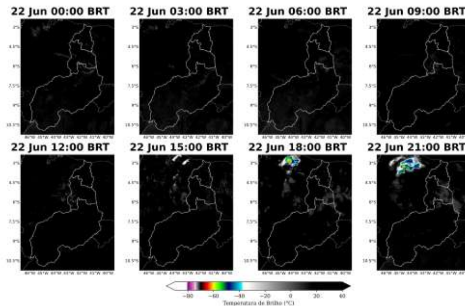
Figura 7: Imagens realçadas do satélite GOES-19 das 00 BRT até 21 BRT (a cada 3 horas) para o dia 22 de Junho.
