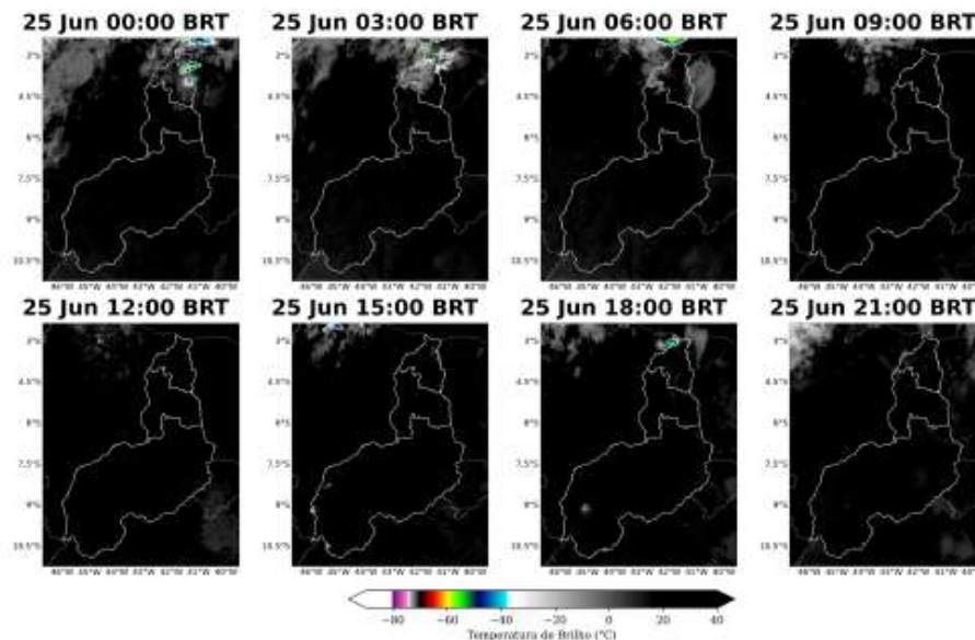
Figura 10: Imagens realçadas do satélite GOES-19 das 00 BRT até 21 BRT (a cada 3 horas) para o dia 25 de Junho.
