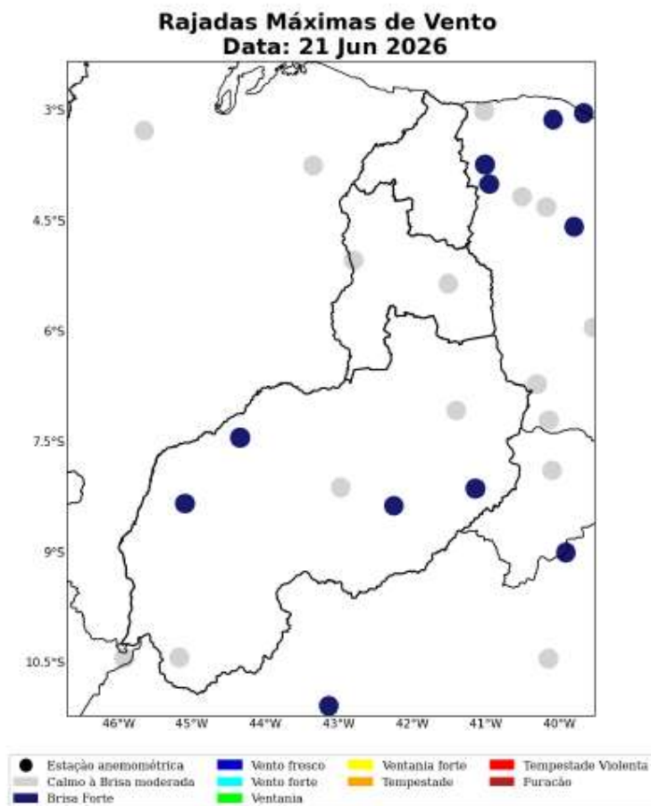
Figura 42: Máxima rajada de vento diária sobre a área de concessão da Equatorial-PI para o dia 21 de Junho, baseado nas estações meteorológicas do INMET.
