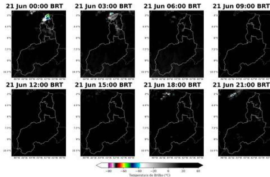
Figura 6: Imagens realçadas do satélite GOES-19 das 00 BRT até 21 BRT (a cada 3 horas) para o dia 21 de Junho.
