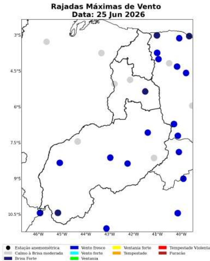
Figura 46: Máxima rajada de vento diária sobre a área de concessão da Equatorial-PI para o dia 25 de Junho, baseado nas estações meteorológicas do INMET.
