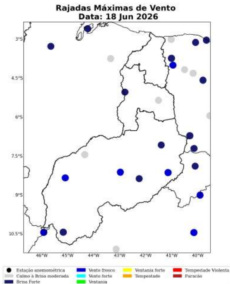
Figura 39: Máxima rajada de vento diária sobre a área de concessão da Equatorial-PI para o dia 18 de Junho, baseado nas estações meteorológicas do INMET.
