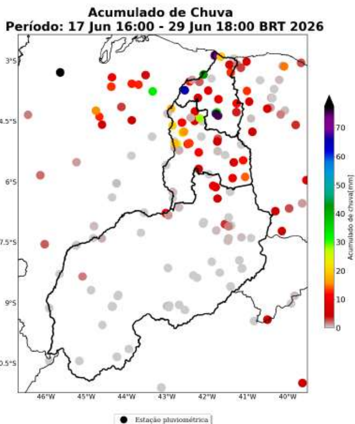
Figura 37: Acumulado de precipitação sobre a área de concessão da Equatorial-PI para o período do evento (dias 17 a 29 de Junho de 2026), baseado nas estações meteorológicas do INMET e CEMADEN.
