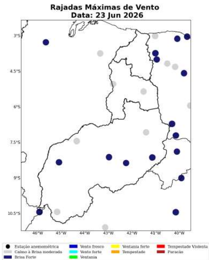
Figura 44: Máxima rajada de vento diária sobre a área de concessão da Equatorial-PI para o dia 23 de Junho, baseado nas estações meteorológicas do INMET.
