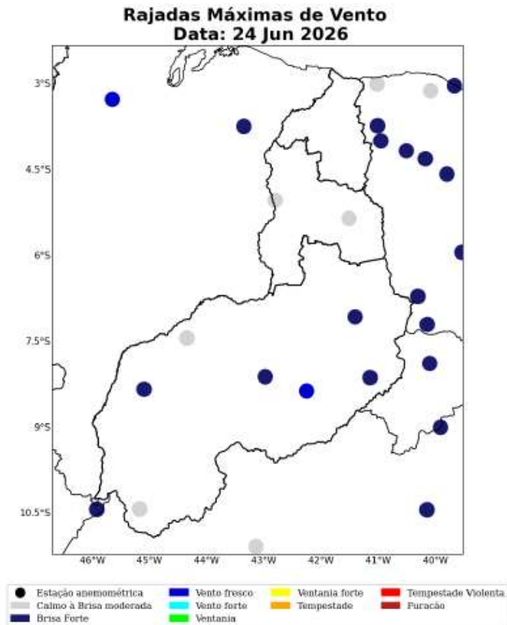
Figura 45: Máxima rajada de vento diária sobre a área de concessão da Equatorial-PI para o dia 24 de Junho, baseado nas estações meteorológicas do INMET.
