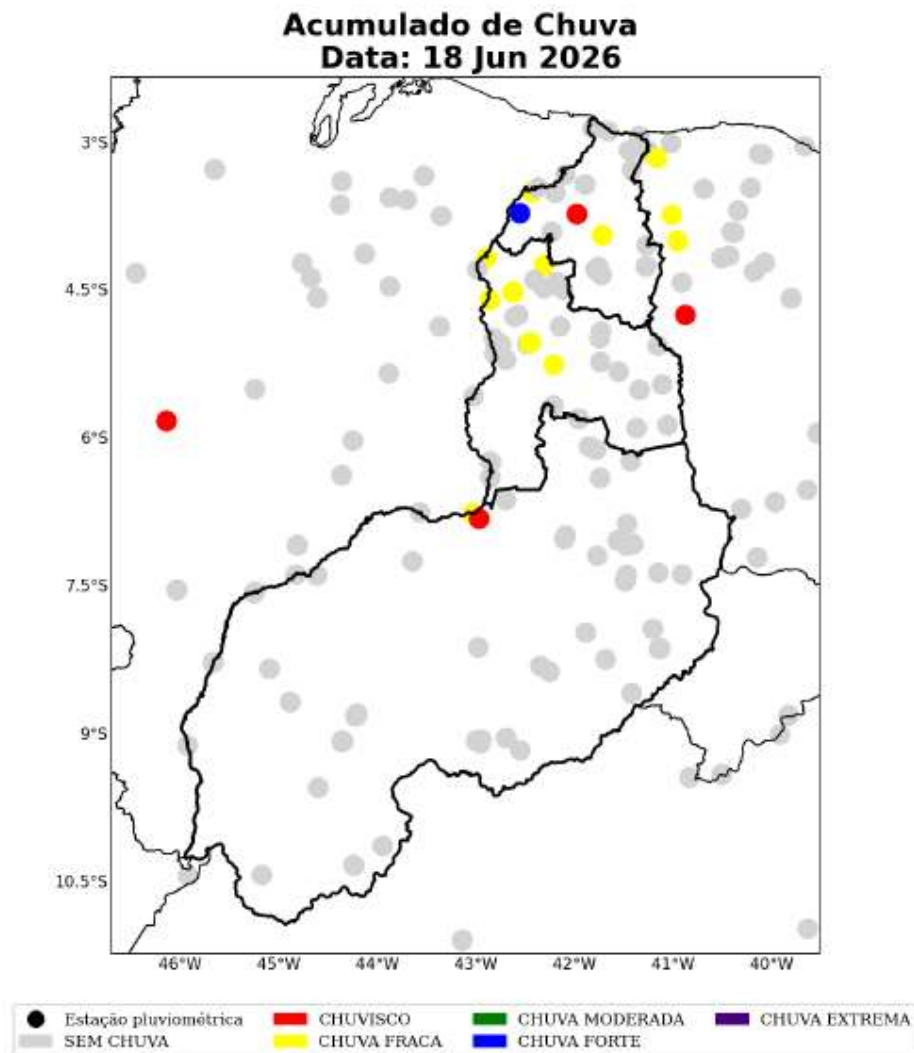
Figura 25: Acumulado diário de precipitação sobre a área de concessão da Equatorial-PI para o dia 18 de Junho, baseado nas estações meteorológicas do INMET e CEMADEN.
