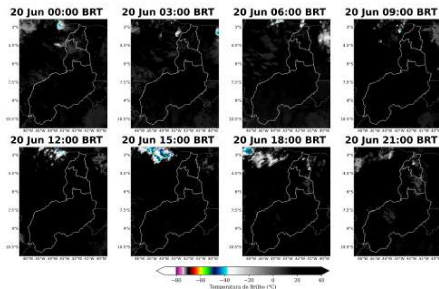
Figura 5: Imagens realçadas do satélite GOES-19 das 00 BRT até 21 BRT (a cada 3 horas) para o dia 20 de Junho.
