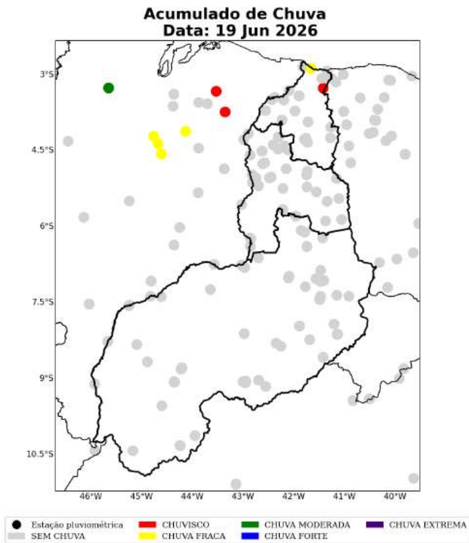
Figura 26: Acumulado diário de precipitação sobre a área de concessão da Equatorial-PI para o dia 19 de Junho, baseado nas estações meteorológicas do INMET e CEMADEN.
