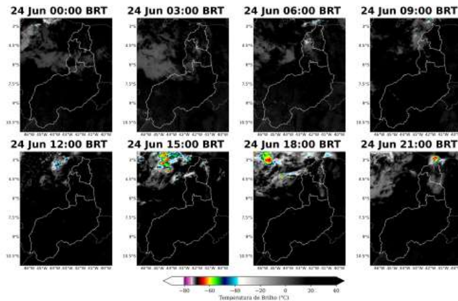
Figura 9: Imagens realçadas do satélite GOES-19 das 00 BRT até 21 BRT (a cada 3 horas) para o dia 24 de Junho.
