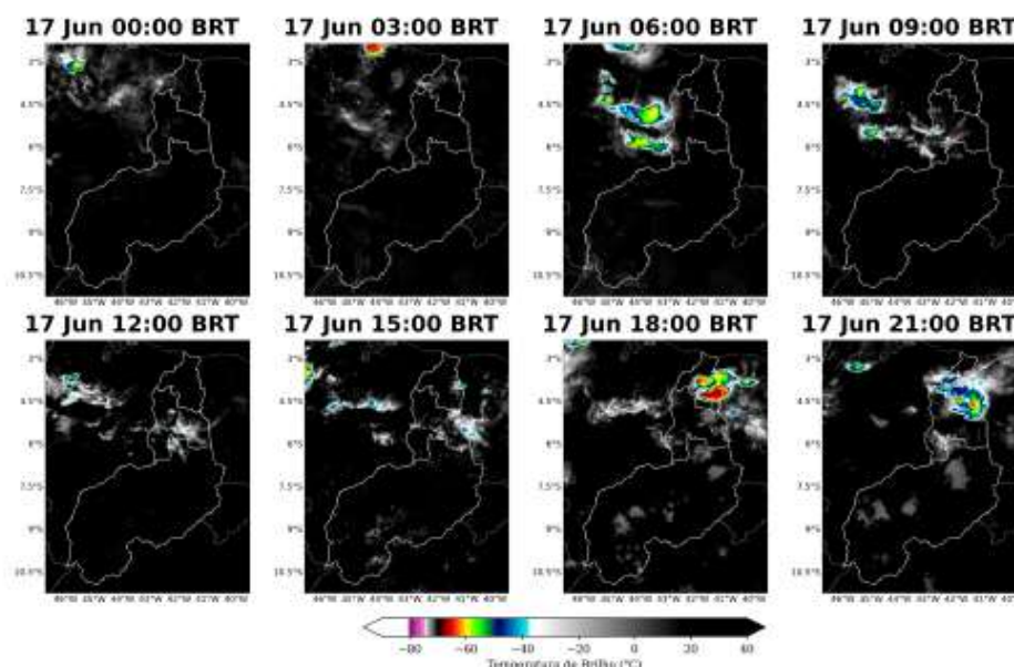
Figura 2: Imagens realçadas do satélite GOES-19 das 00 BRT até 21 BRT (a cada 3 horas) para o dia 17 de Junho.
