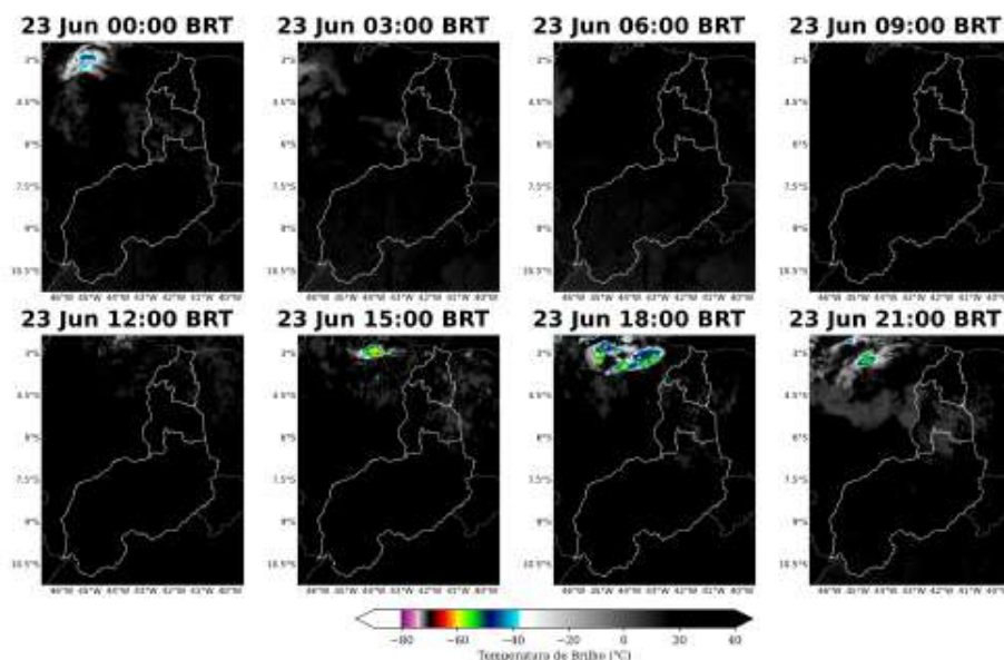
Figura 8: Imagens realçadas do satélite GOES-19 das 00 BRT até 21 BRT (a cada 3 horas) para o dia 23 de Junho.
