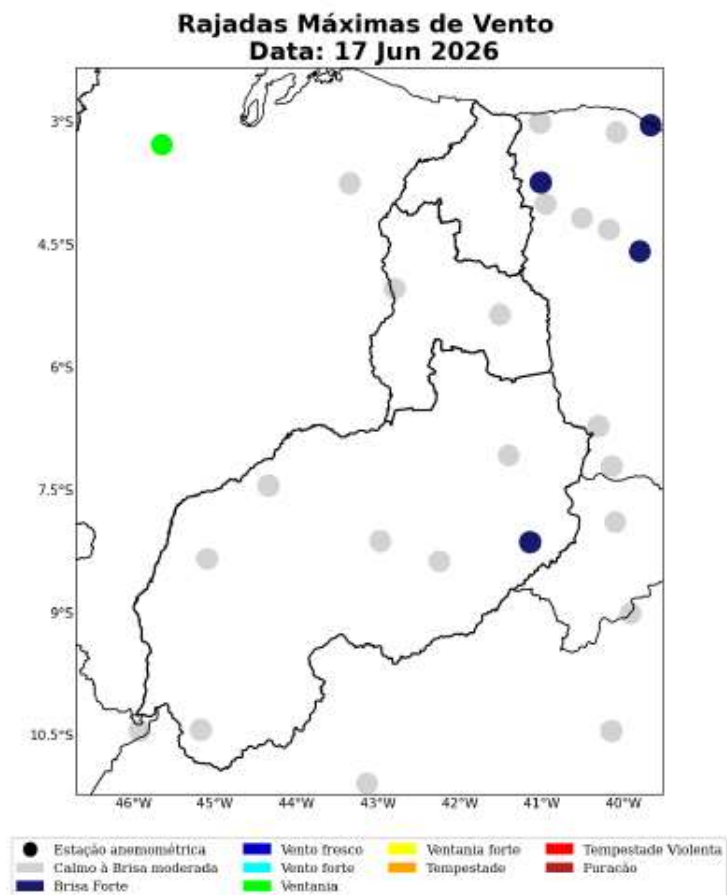
Figura 38: Máxima rajada de vento diária sobre a área de concessão da Equatorial-PI para o dia 17 de Junho, baseado nas estações meteorológicas do INMET.
