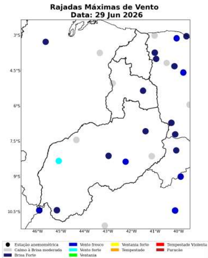
Figura 50: Máxima rajada de vento diária sobre a área de concessão da Equatorial-PI para o dia 29 de Junho, baseado nas estações meteorológicas do INMET.
