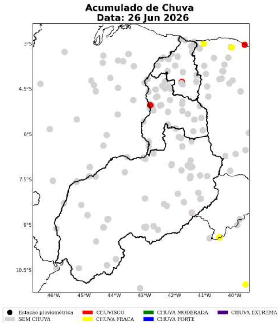
Figura 33: Acumulado diário de precipitação sobre a área de concessão da Equatorial-PI para o dia 26 de Junho, baseado nas estações meteorológicas do INMET e CEMADEN.
