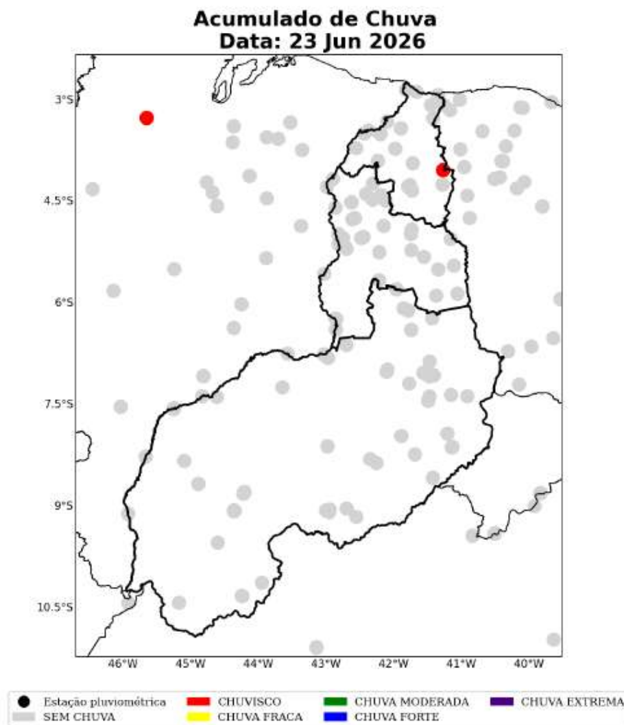
Figura 30: Acumulado diário de precipitação sobre a área de concessão da Equatorial-PI para o dia 23 de Junho, baseado nas estações meteorológicas do INMET e CEMADEN.
