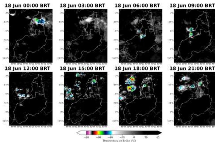
Figura 3: Imagens realçadas do satélite GOES-19 das 00 BRT até 21 BRT (a cada 3 horas) para o dia 18 de Junho.
