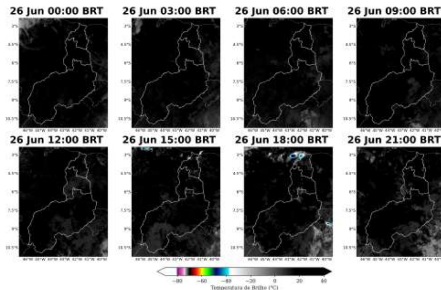
Figura 11: Imagens realçadas do satélite GOES-19 das 00 BRT até 21 BRT (a cada 3 horas) para o dia 26 de Junho.
