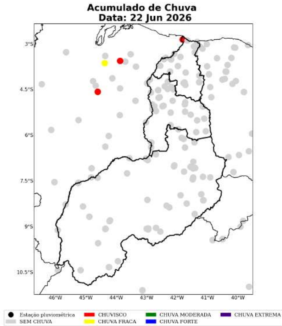
Figura 29: Acumulado diário de precipitação sobre a área de concessão da Equatorial-PI para o dia 22 de Junho, baseado nas estações meteorológicas do INMET e CEMADEN.
