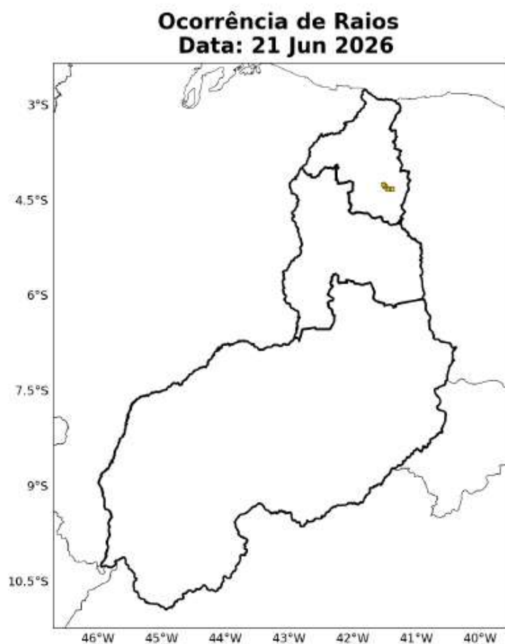
Figura 19: Ocorrências de descargas atmosféricas nuvem-solo detectadas pelo sistema Earth Networks para o dia 21 de Junho sobre a área de concessão da Equatorial-PI.
