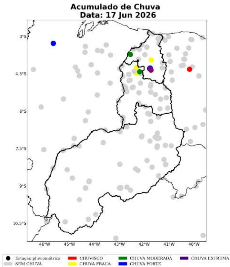
Figura 24: Acumulado diário de precipitação sobre a área de concessão da Equatorial-PI para o dia 17 de Junho, baseado nas estações meteorológicas do INMET e CEMADEN.
