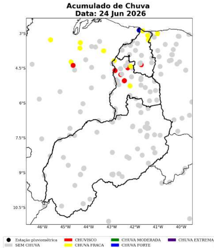
Figura 31: Acumulado diário de precipitação sobre a área de concessão da Equatorial-PI para o dia 24 de Junho, baseado nas estações meteorológicas do INMET e CEMADEN.
