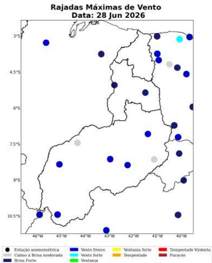
Figura 49: Máxima rajada de vento diária sobre a área de concessão da Equatorial-PI para o dia 28 de Junho, baseado nas estações meteorológicas do INMET.
