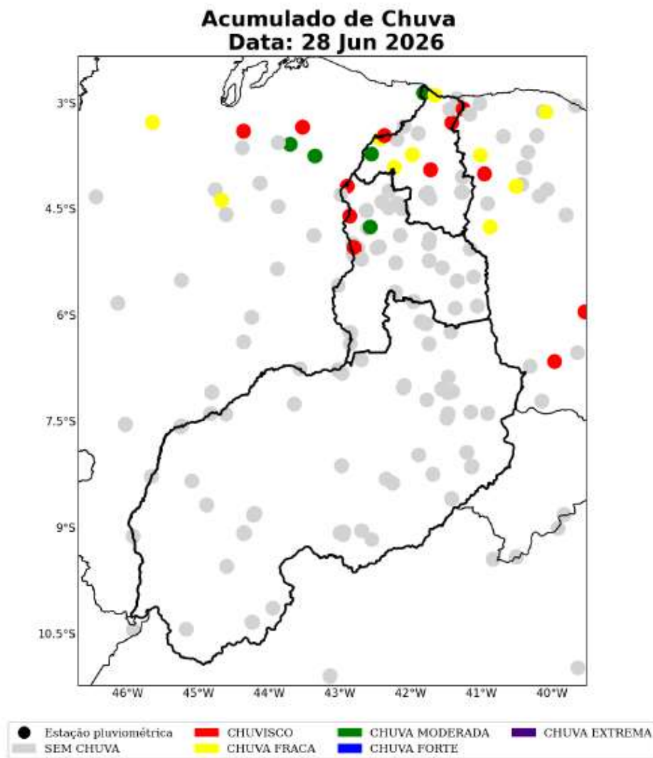
Figura 35: Acumulado diário de precipitação sobre a área de concessão da Equatorial-PI para o dia 28 de Junho, baseado nas estações meteorológicas do INMET e CEMADEN.
