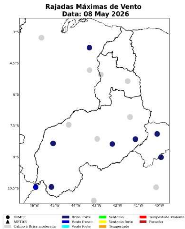
Figura 34: Máxima rajada de vento diária sobre a área de concessão da Equatorial-PI para o dia 08 de Maio, baseado nas estações meteorológicas do INMET.
