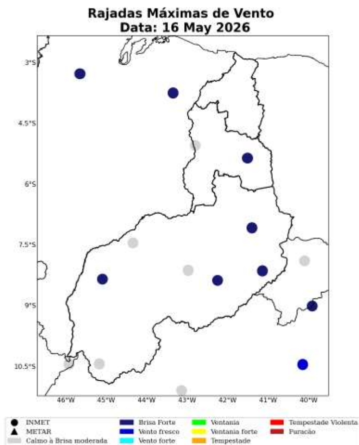
Figura 42: Máxima rajada de vento diária sobre a área de concessão da Equatorial-PI para o dia 16 de Maio, baseado nas estações meteorológicas do INMET.
