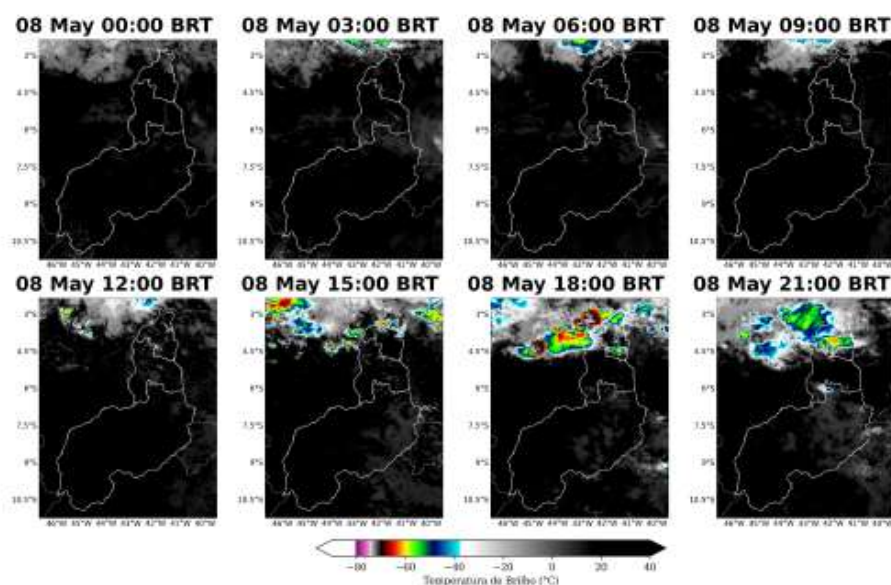
Figura 2: Imagens realçadas do satélite GOES-19 das 00 BRT até 21 BRT (a cada 3 horas) para o dia 08 de Maio.
