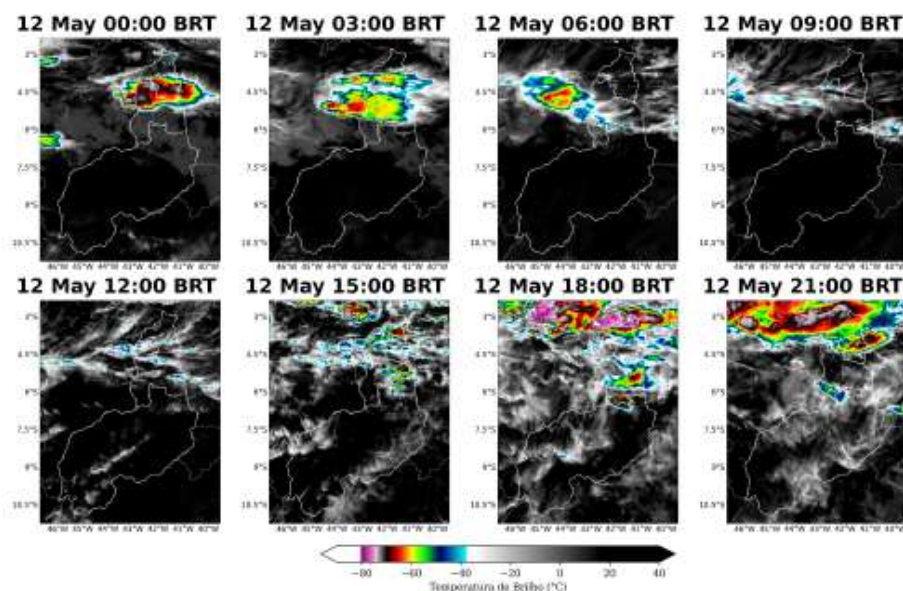
Figura 6: Imagens realizadas do satélite GOES-19 das 00 BRT até 21 BRT (a cada 3 horas) para o dia 12 de Maio.
