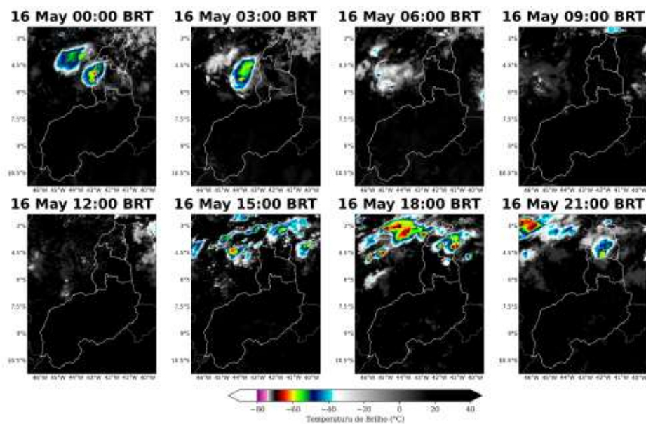
Figura 10: Imagens realçadas do satélite GOES-19 das 00 BRT até 21 BRT (a cada 3 horas) para o dia 16 de Maio.
