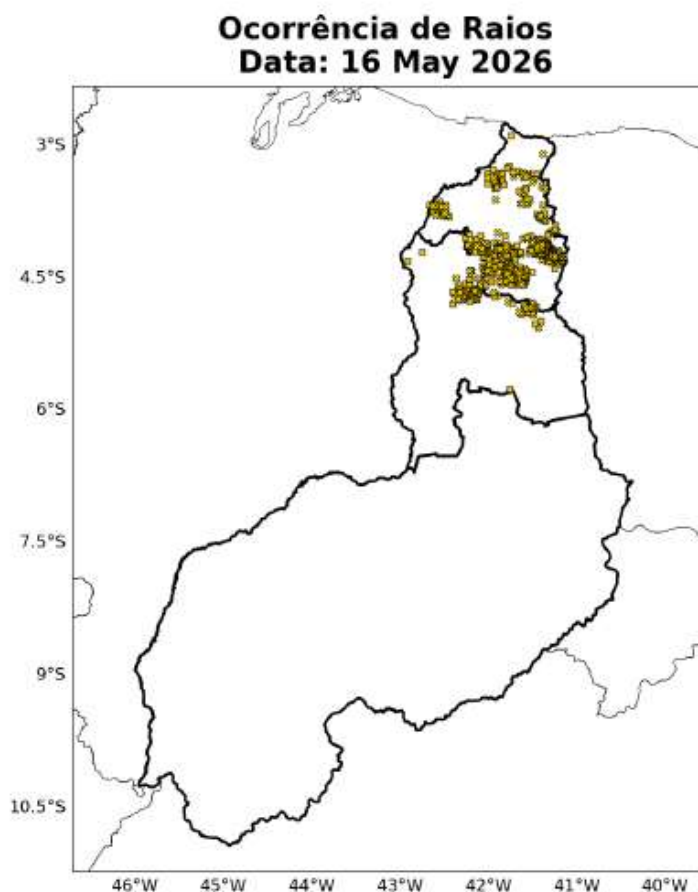
Figura 20: Ocorrências de descargas atmosféricas nuvem-solo detectadas pelo sistema Earth Networks para o dia 16 de Maio sobre a área de concessão da Equatorial-PI.
