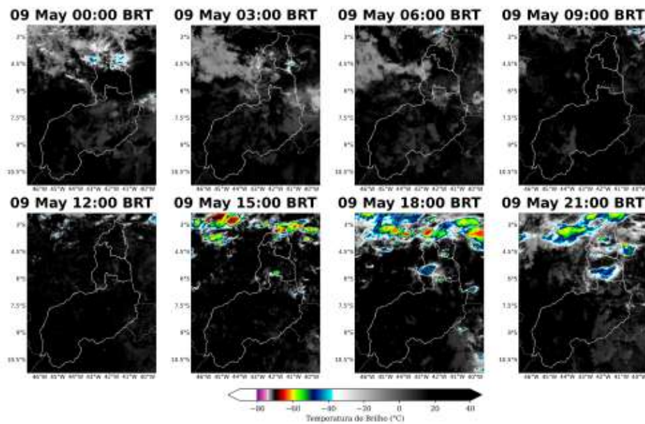
Figura 3: Imagens realçadas do satélite GOES-19 das 00 BRT até 21 BRT (a cada 3 horas) para o dia 09 de Maio.
