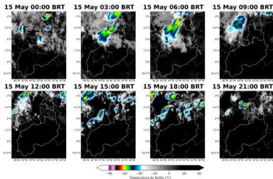
Figura 9: Imagens realizadas do satélite GOES-19 das 00 BRT até 21 BRT (a cada 3 horas) para o dia 15 de Maio.
