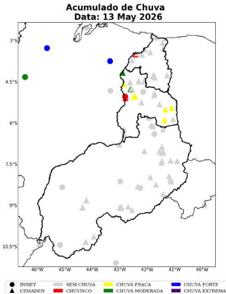
Figura 28: Acumulado diário de precipitação sobre a área de concessão da Equatorial-PI para o dia 13 de Maio, baseado nas estações meteorológicas do INMET e CEMADEN.
