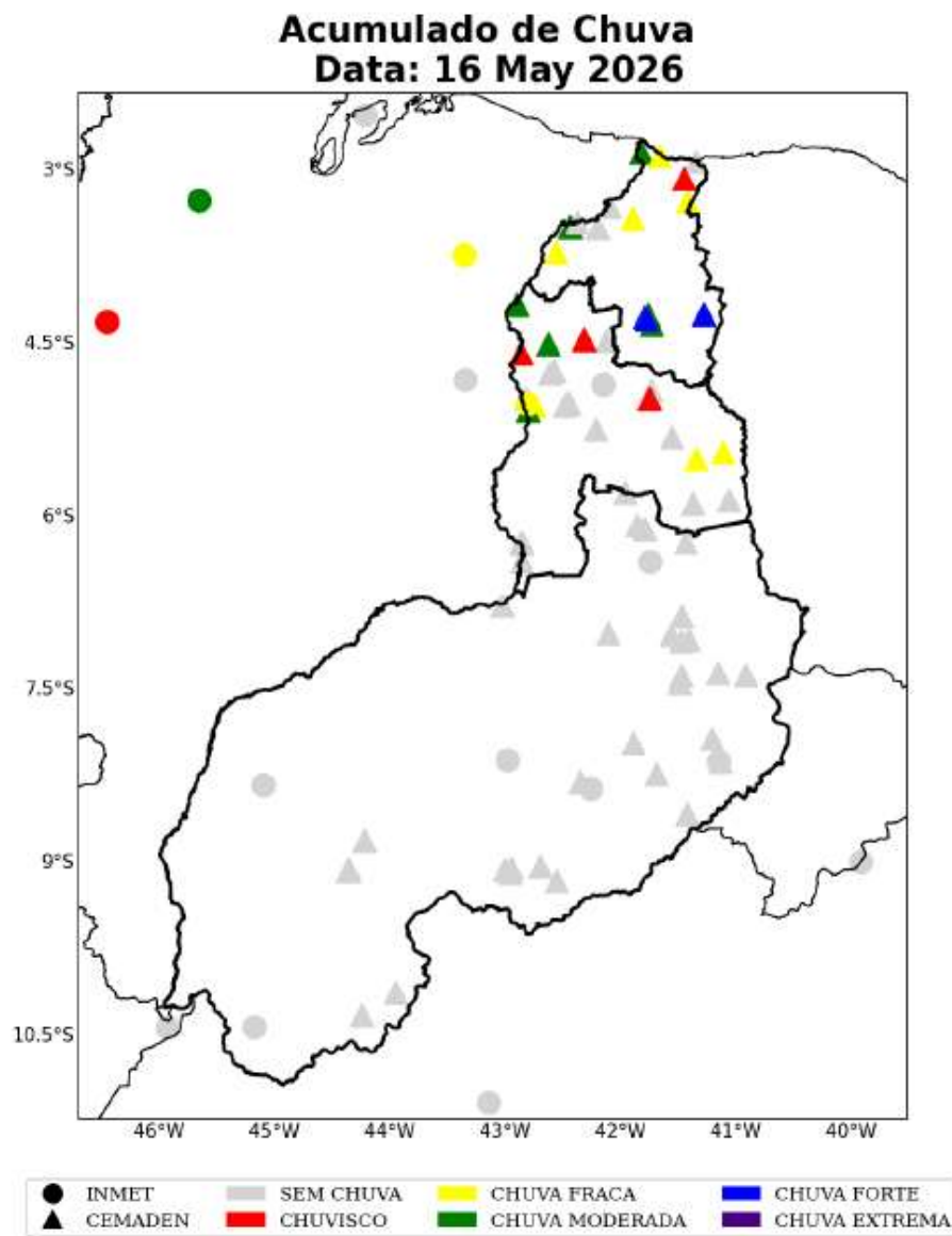
Figura 31: Acumulado diário de precipitação sobre a área de concessão da Equatorial-PI para o dia 16 de Maio, baseado nas estações meteorológicas do INMET e CEMADEN.
