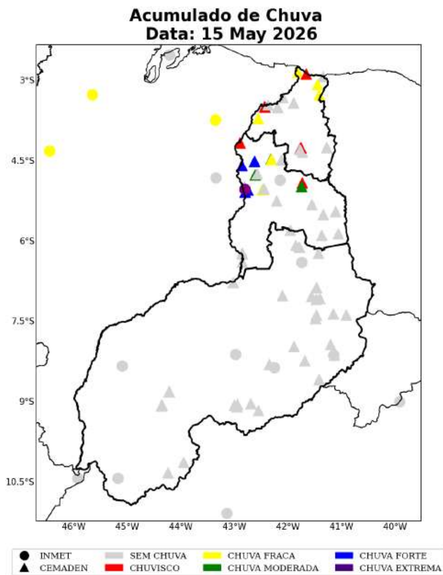
Figura 30: Acumulado diário de precipitação sobre a área de concessão da Equatorial-PI para o dia 15 de Maio, baseado nas estações meteorológicas do INMET e CEMADEN.
