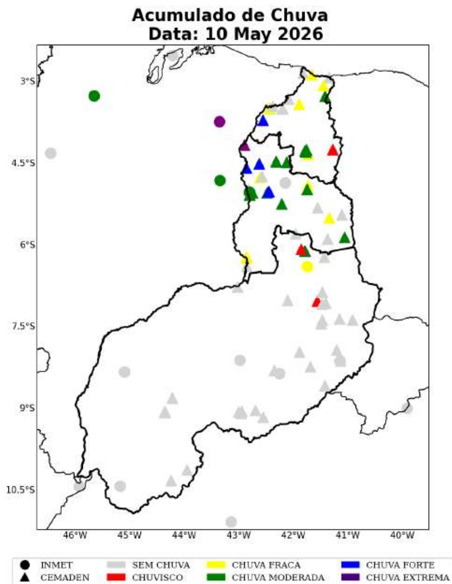
Figura 25: Acumulado diário de precipitação sobre a área de concessão da Equatorial-PI para o dia 10 de Maio, baseado nas estações meteorológicas do INMET e CEMADEN.
