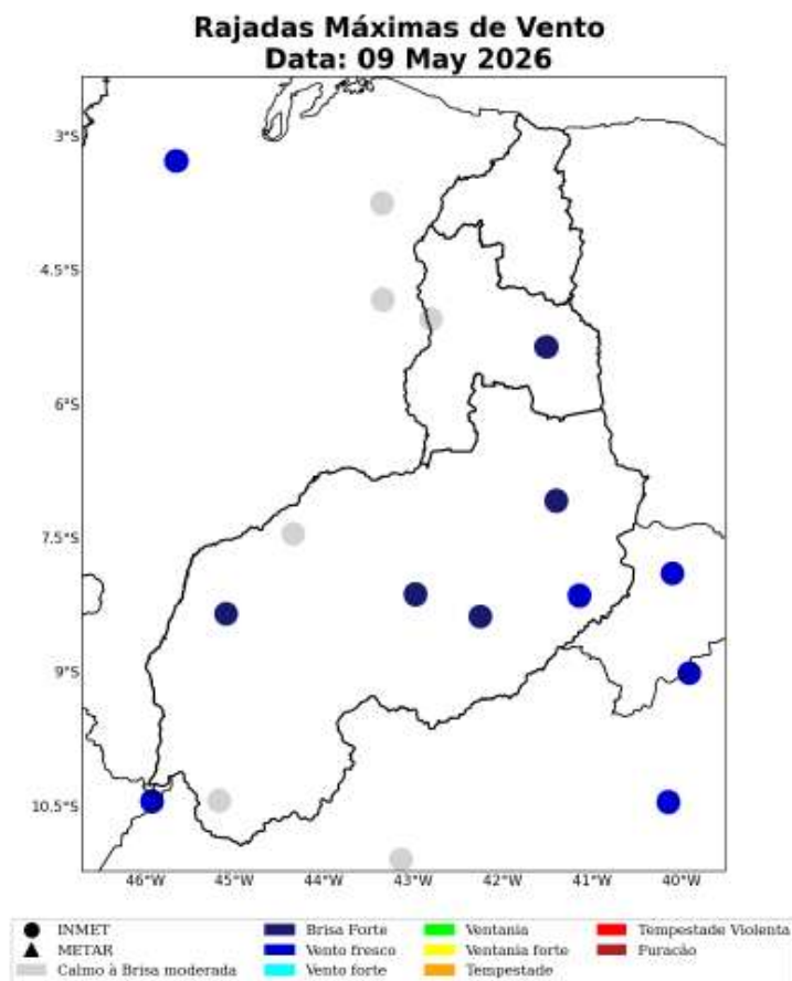
Figura 35: Máxima rajada de vento diária sobre a área de concessão da Equatorial-PI para o dia 09 de Maio, baseado nas estações meteorológicas do INMET.
