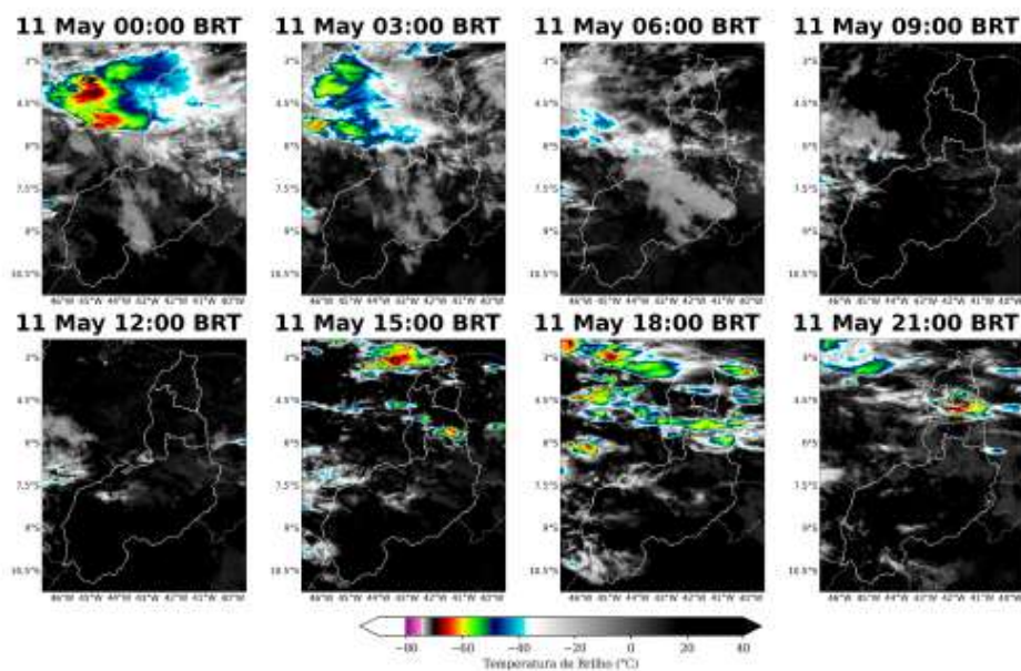
Figura 5: Imagens realçadas do satélite GOES-19 das 00 BRT até 21 BRT (a cada 3 horas) para o dia 11 de Maio.
