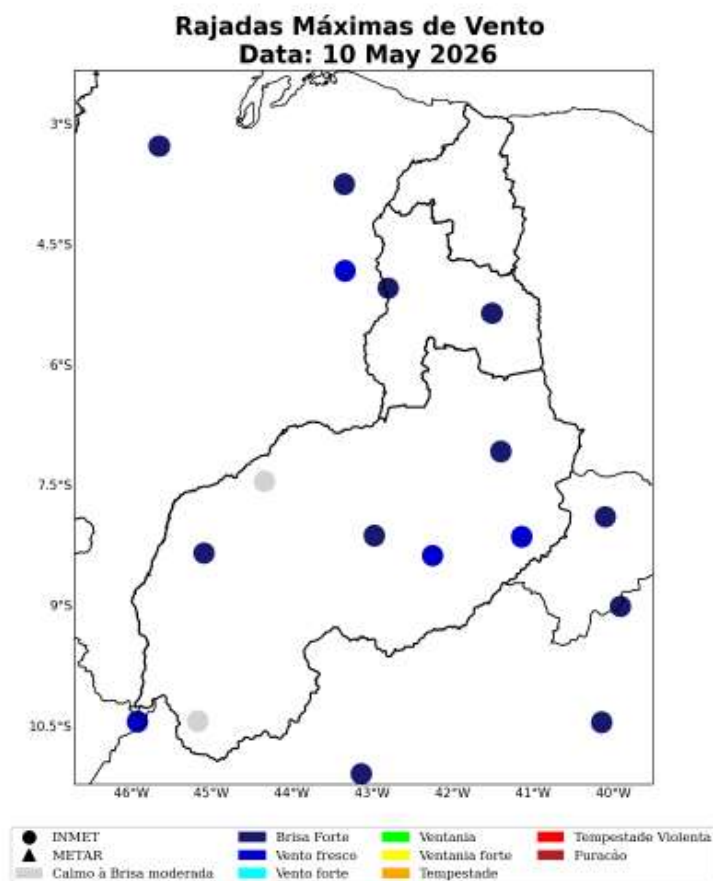
Figura 36: Máxima rajada de vento diária sobre a área de concessão da Equatorial-PI para o dia 10 de Maio, baseado nas estações meteorológicas do INMET.
