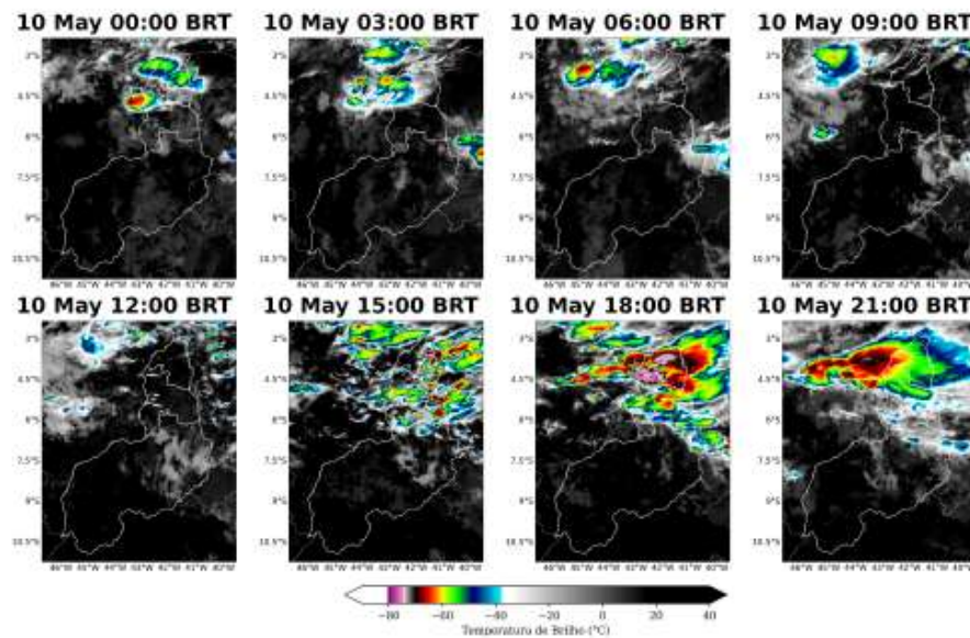
Figura 4: Imagens realçadas do satélite GOES-19 das 00 BRT até 21 BRT (a cada 3 horas) para o dia 10 de Maio.
