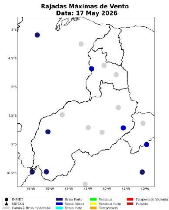
Figura 43: Máxima rajada de vento diária sobre a área de concessão da Equatorial-PI para o dia 17 de Maio, baseado nas estações meteorológicas do INMET.
