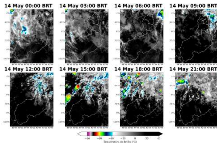
Figura 8: Imagens realçadas do satélite GOES-19 das 00 BRT até 21 BRT (a cada 3 horas) para o dia 14 de Maio.
