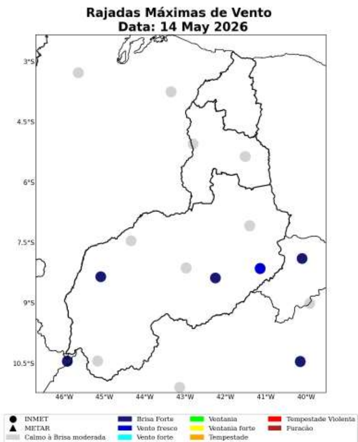
Figura 40: Máxima rajada de vento diária sobre a área de concessão da Equatorial-PI para o dia 14 de Maio, baseado nas estações meteorológicas do INMET.
