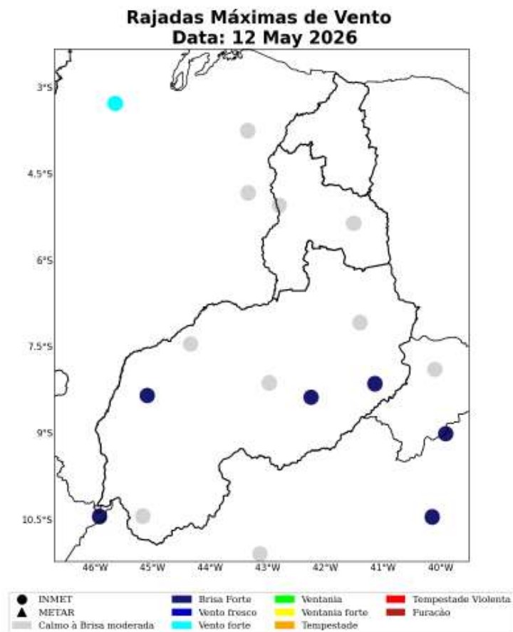
Figura 38: Máxima rajada de vento diária sobre a área de concessão da Equatorial-PI para o dia 12 de Maio, baseado nas estações meteorológicas do INMET.
