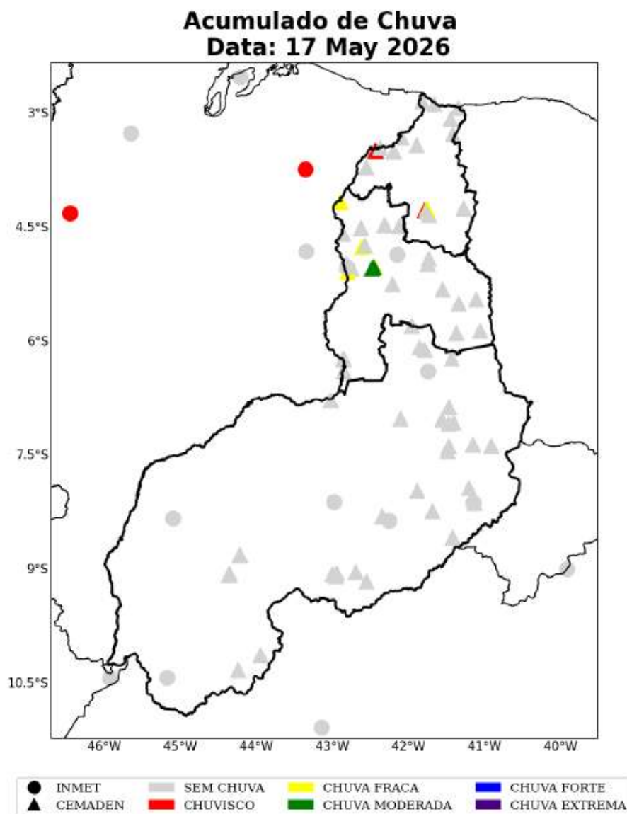
Figura 32: Acumulado diário de precipitação sobre a área de concessão da Equatorial-PI para o dia 17 de Maio, baseado nas estações meteorológicas do INMET e CEMADEN.
