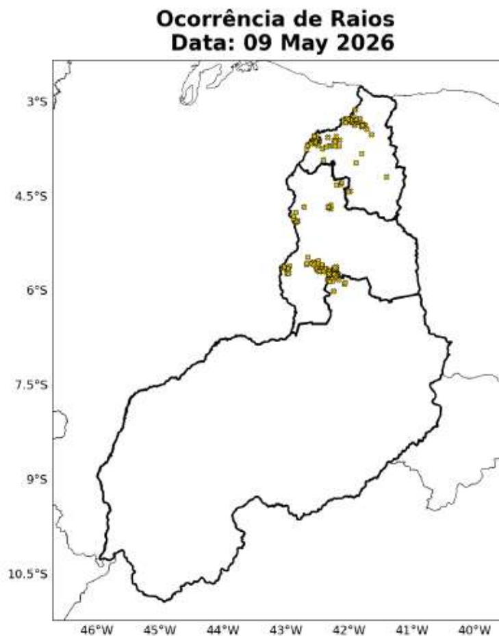
Figura 13: Ocorrências de descargas atmosféricas nuvem-solo detectadas pelo sistema Earth Networks para o dia 09 de Maio sobre a área de concessão da Equatorial-PI.
