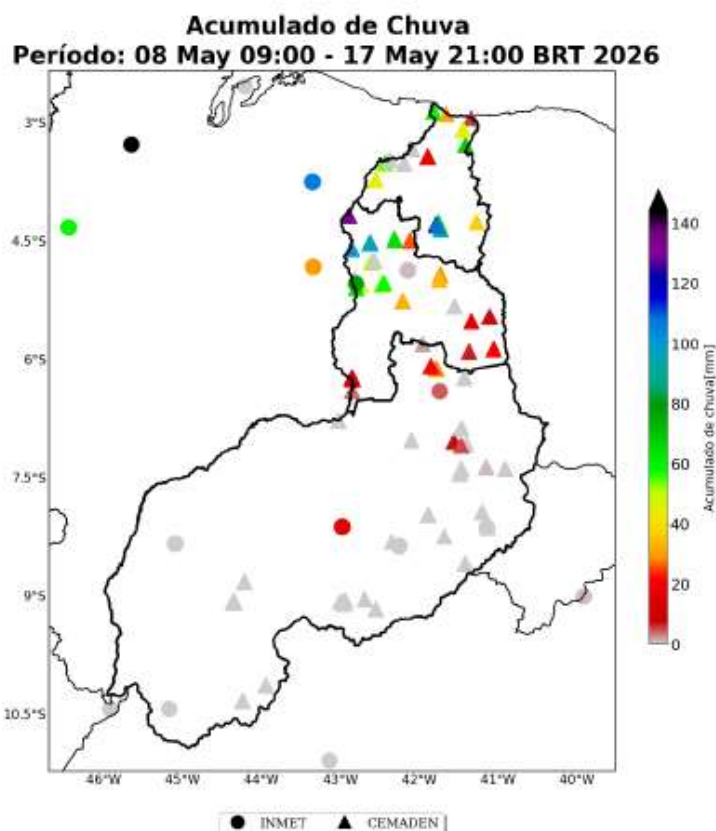
Figura 33: Acumulado de precipitação sobre a área de concessão da Equatorial-PI para o período do evento (dias 08 a 17 de Maio de 2026), baseado nas estações meteorológicas do INMET e CEMADEN.
