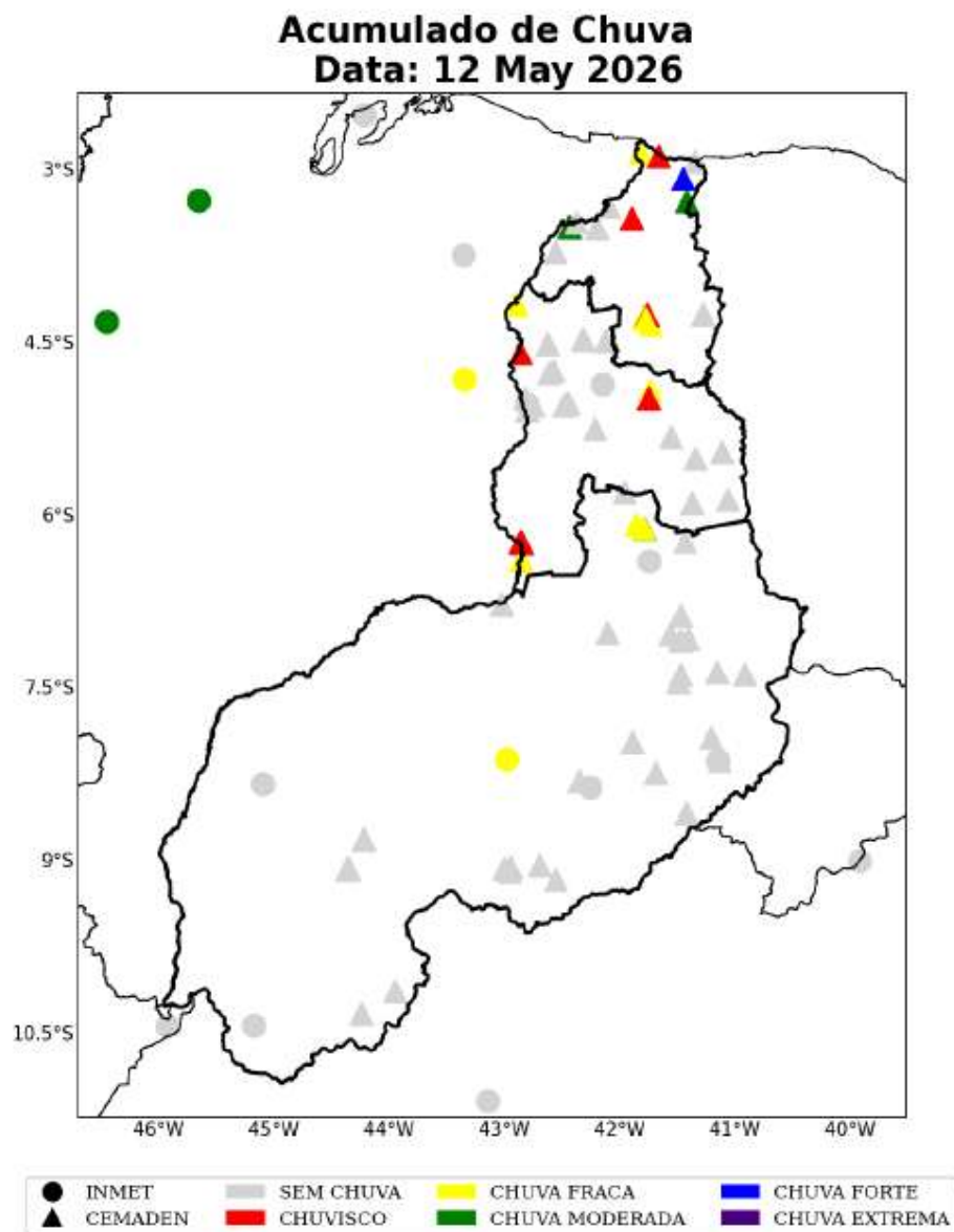
Figura 27: Acumulado diário de precipitação sobre a área de concessão da Equatorial-PI para o dia 12 de Maio, baseado nas estações meteorológicas do INMET e CEMADEN.
