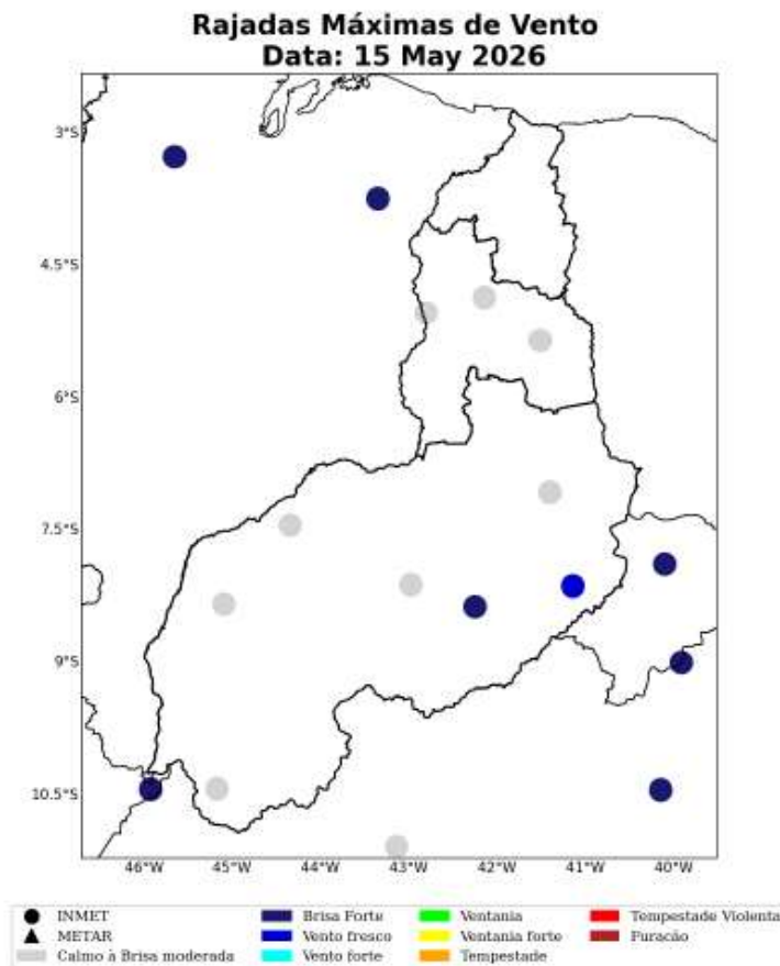
Figura 41: Máxima rajada de vento diária sobre a área de concessão da Equatorial-PI para o dia 15 de Maio, baseado nas estações meteorológicas do INMET.
