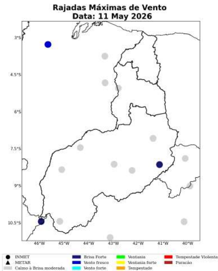
Figura 37: Máxima rajada de vento diária sobre a área de concessão da Equatorial-PI para o dia 11 de Maio, baseado nas estações meteorológicas do INMET.
