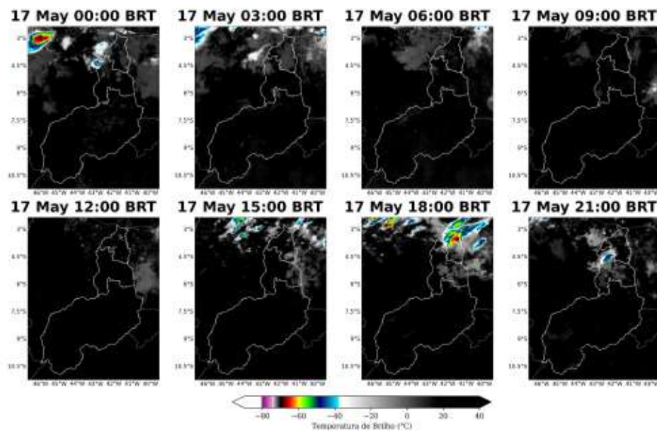
Figura 11: Imagens reagçadas do satélite GOES-19 das 00 BRT até 21 BRT (a cada 3 horas) para o dia 17 de Maio.
