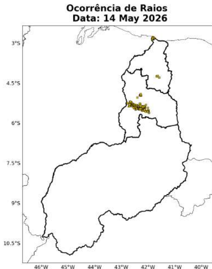
Figura 18: Ocorrências de descargas atmosféricas nuvem-solo detectadas pelo sistema Earth Networks para o dia 14 de Maio sobre a área de concessão da Equatorial-PI.
