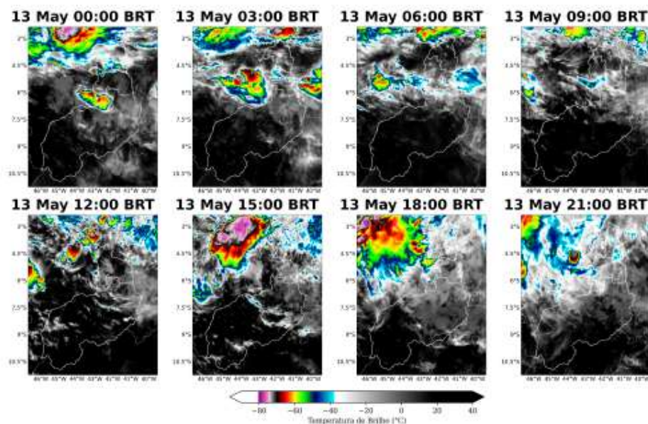
Figura 7: Imagens realçadas do satélite GOES-19 das 00 BRT até 21 BRT (a cada 3 horas) para o dia 13 de Maio.
