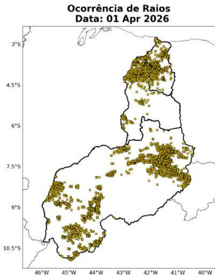
Figura 5: Ocorrências de descargas atmosféricas nuvem-solo detectadas pelo sistema Earth Networks para o dia 01 de Abril sobre a área de concessão da Equatorial-PI.
