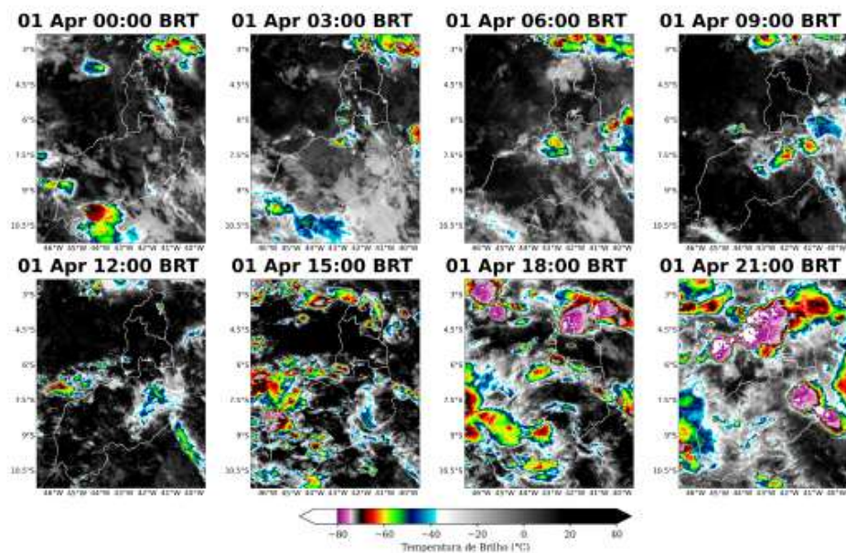
Figura 2: Imagens realçadas do satélite GOES-19 das 00 BRT até 21 BRT (a cada 3 horas) para o dia 01 de Abril.
