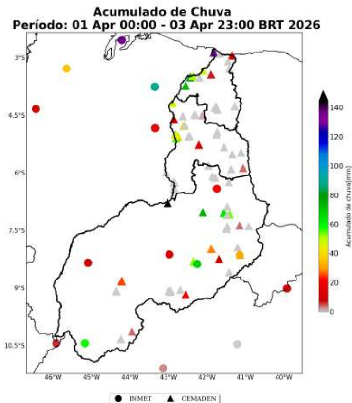
Figura 12: Acumulado de precipitação sobre a área de concessão da Equatorial-PI para o período do evento (dias 01 a 03 de Abril de 2026), baseado nas estações meteorológicas do INMET e CEMADEN.
