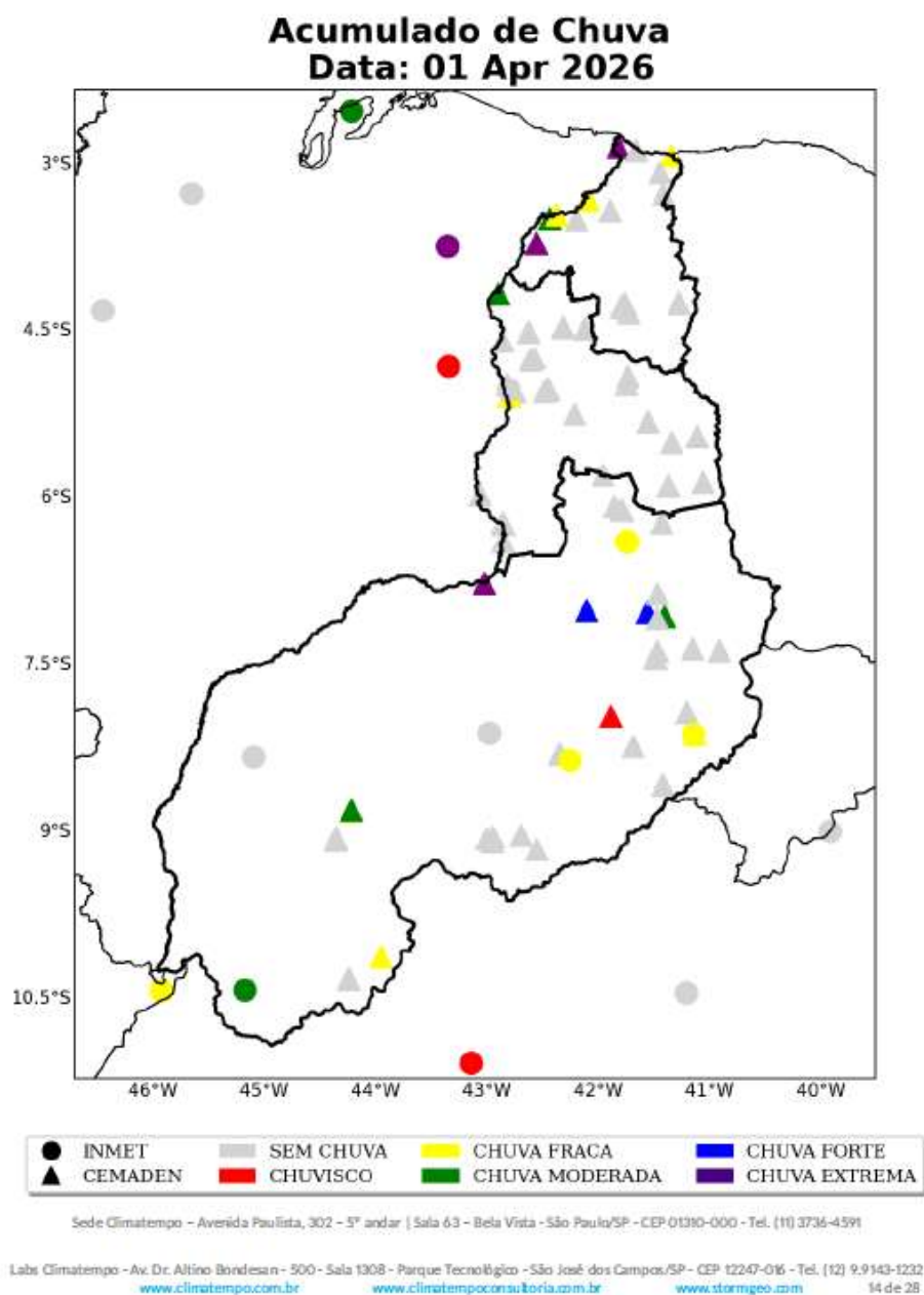
Figura 9: Acumulado diário de precipitação sobre a área de concessão da Equatorial-PI para o dia 01 de Abril, baseado nas estações meteorológicas do INMET e CEMADEN.
