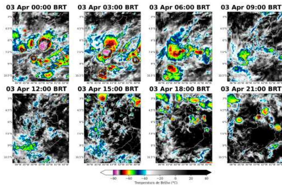
Figura 4: Imagens realçadas do satélite GOES-19 das 00 BRT até 21 BRT (a cada 3 horas) para o dia 03 de Abril.
