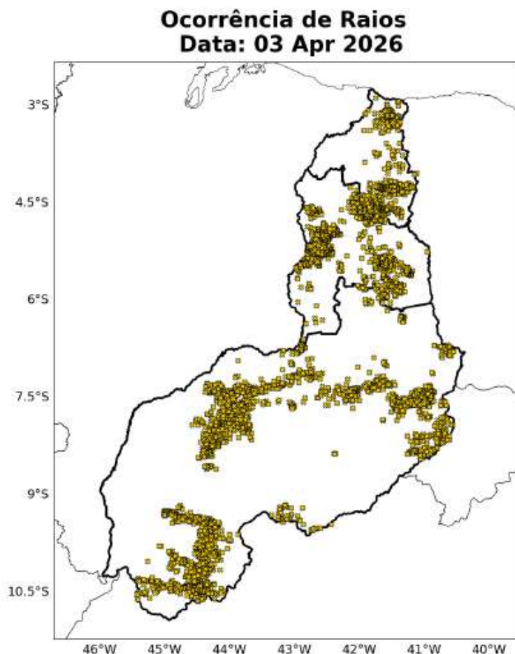
Figura 7: Ocorrências de descargas atmosféricas nuvem-solo detectadas pelo sistema Earth Networks para o dia 03 de Abril sobre a área de concessão da Equatorial-PI.
