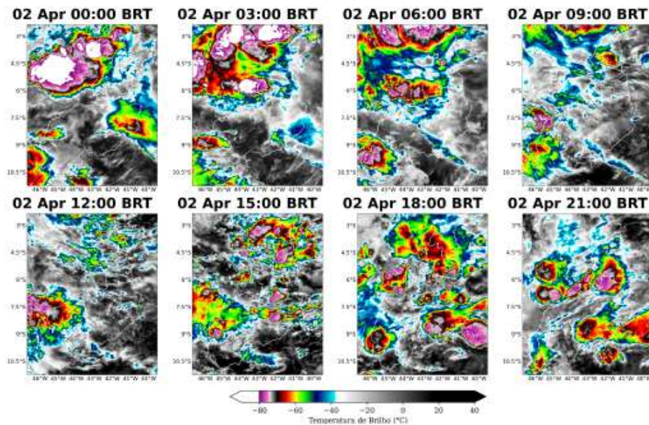
Figura 3: Imagens realçadas do satélite GOES-19 das 00 BRT até 21 BRT (a cada 3 horas) para o dia 02 de Abril.
