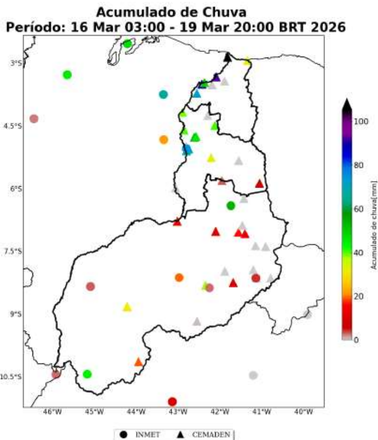
Figura 15: Acumulado de precipitação sobre o estado do Piauí para o período do evento (dias 16 a 19 de Março de 2026), baseado nas estações meteorológicas do INMET e CEMADEN.
