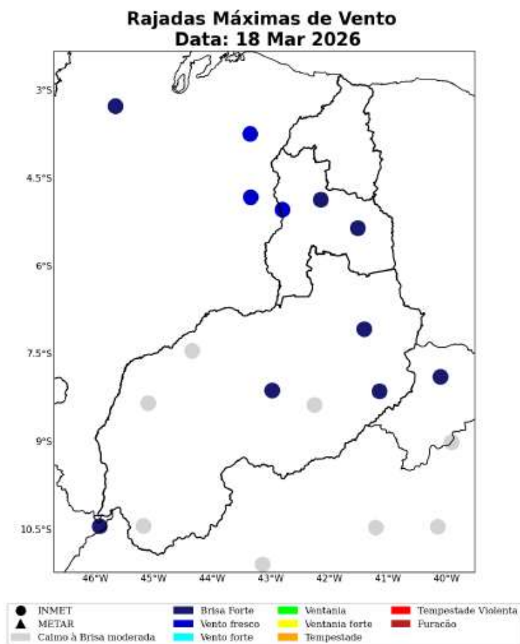
Figura 18: Máxima rajada de vento diária sobre a área de concessão da Equatorial-PI para o dia 18 de Março, baseado nas estações meteorológicas do INMET.
