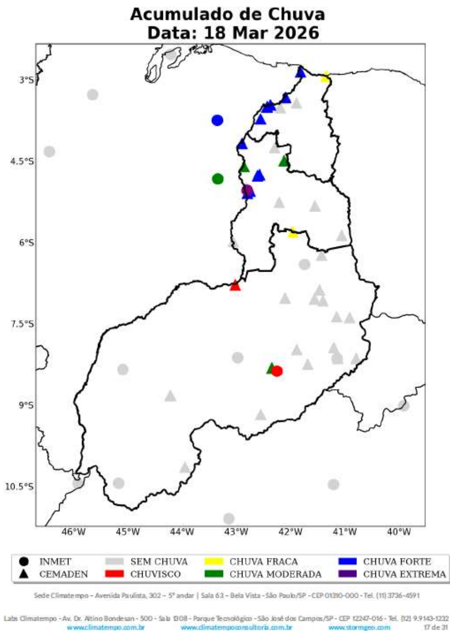
Figura 13: Acumulado diário de precipitação sobre a área de concessão da Equatorial-PI para o dia 18 de Março, baseado nas estações meteorológicas do INMET e CEMADEN.
