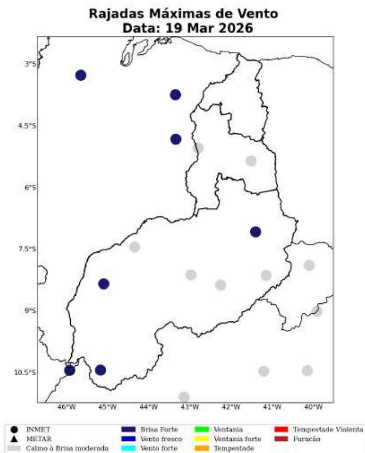
Figura 19: Máxima rajada de vento diária sobre a área de concessão da Equatorial-PI para o dia 19 de Março, baseado nas estações meteorológicas do INMET.
