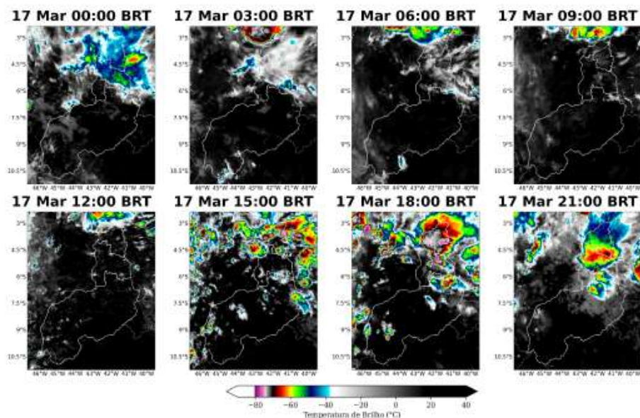
Figura 3: Imagens realizadas do satélite GOES-19 das 00 BRT até 21 BRT (a cada 3 horas) para o dia 17 de Março.
