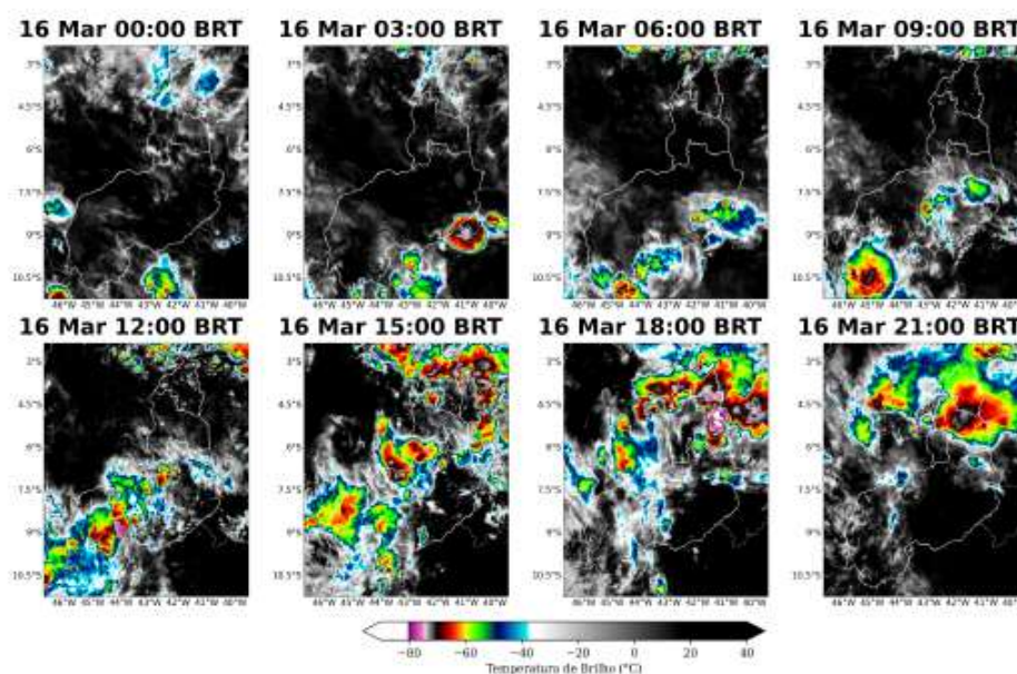
Figura 2: Imagens realizadas do satélite GOES-19 das 00 BRT até 21 BRT (a cada 3 horas) para o dia 16 de Março.
