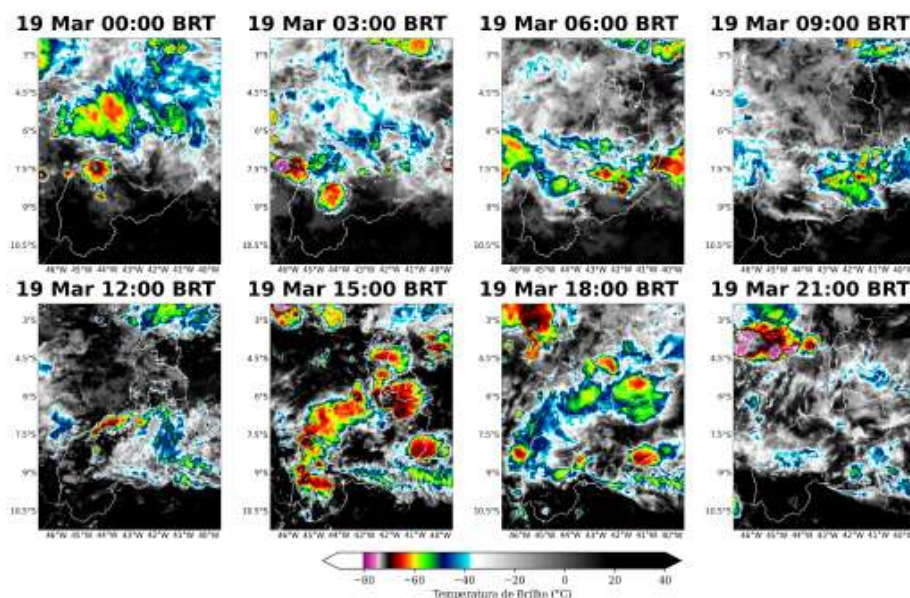
Figura 5: Imagens realizadas do satélite GOES-19 das 00 BRT até 21 BRT (a cada 3 horas) para o dia 19 de Março.
