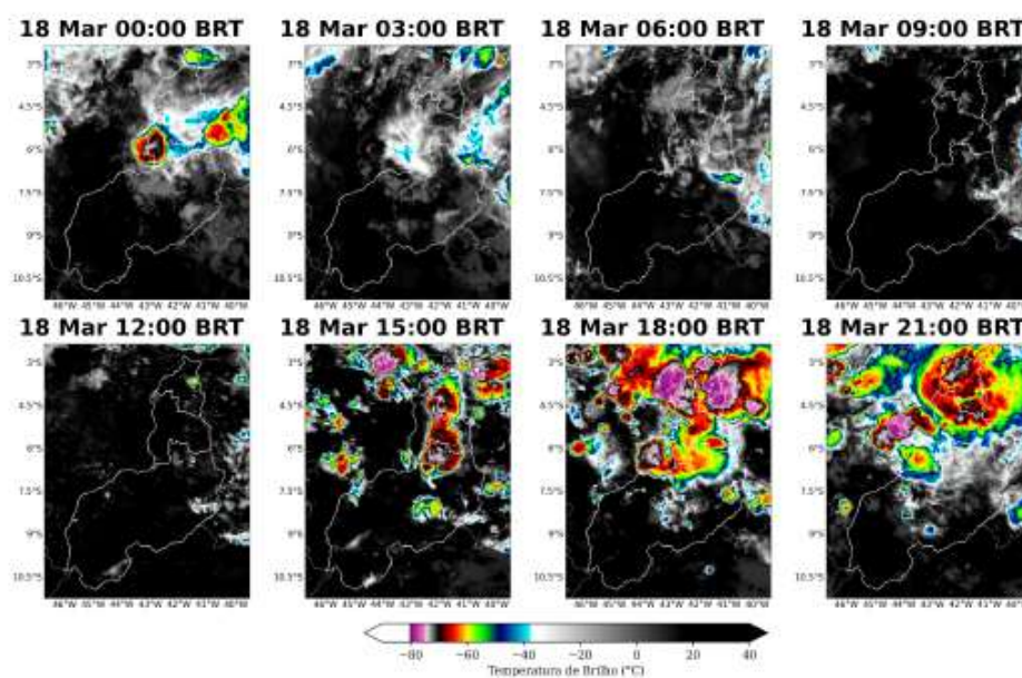
Figura 4: Imagens realçadas do satélite GOES-19 das 00 BRT até 21 BRT (a cada 3 horas) para o dia 18 de Março.
