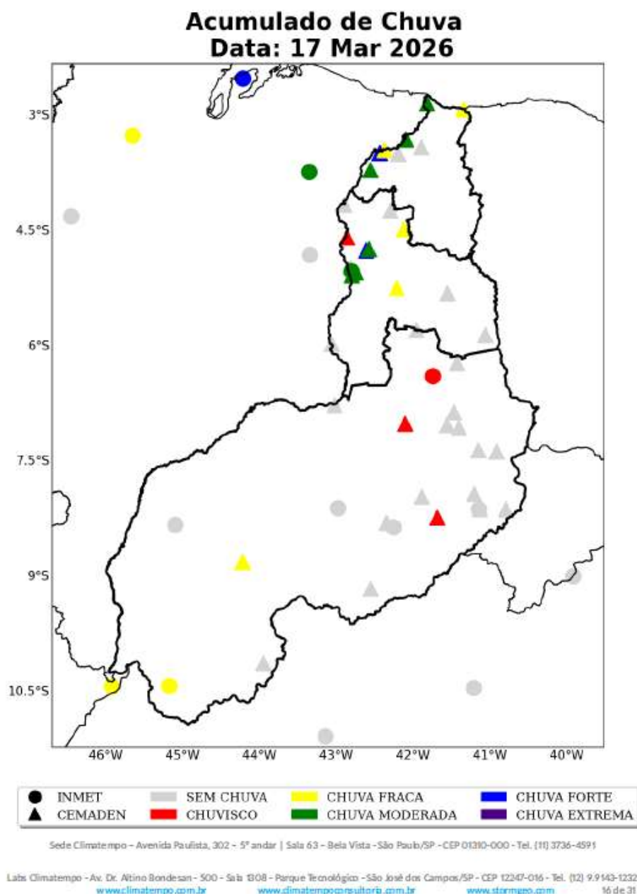
Figura 12: Acumulado diário de precipitação sobre a área de concessão da Equatorial-PI para o dia 17 de Março, baseado nas estações meteorológicas do INMET e CEMADEN.
