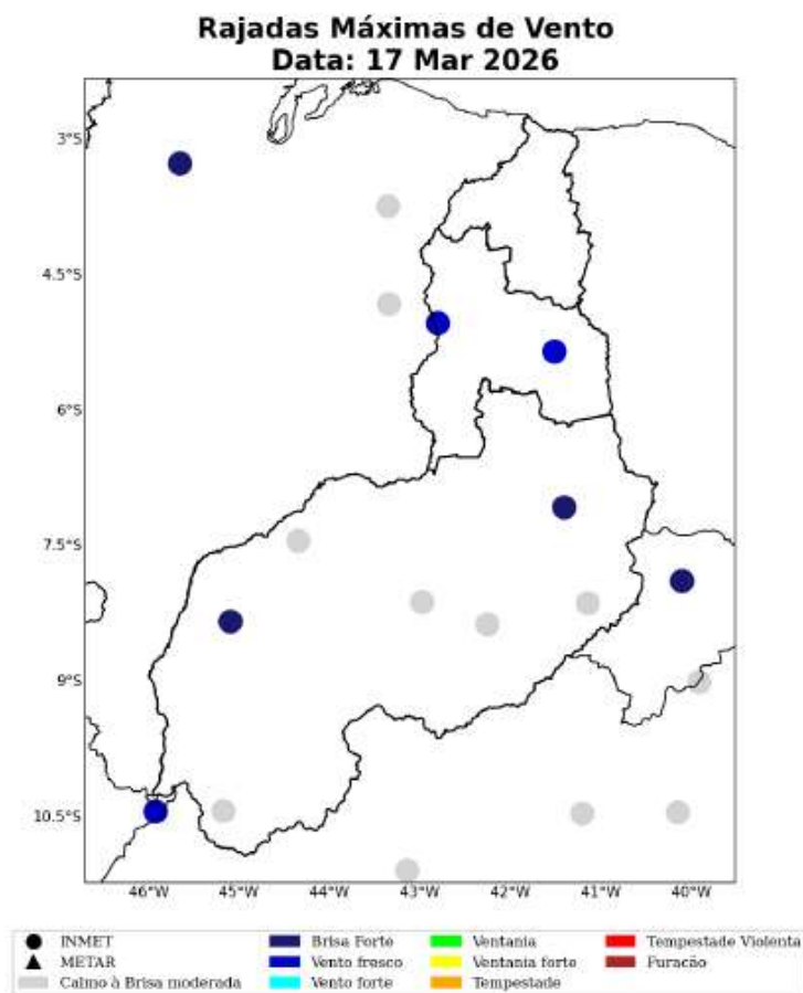
Figura 17: Máxima rajada de vento diária sobre a área de concessão da Equatorial-PI para o dia 17 de Março, baseado nas estações meteorológicas do INMET.
