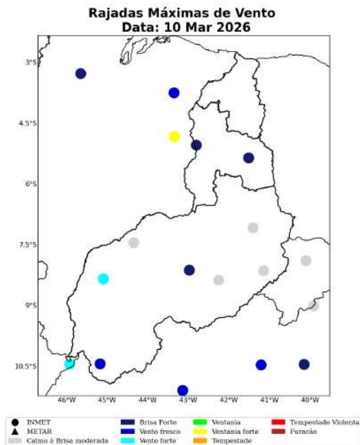
Figura 11: Máxima rajada de vento diária sobre a área de concessão da Equatorial-PI para o dia 10 de Março, baseado nas estações meteorológicas do INMET.
