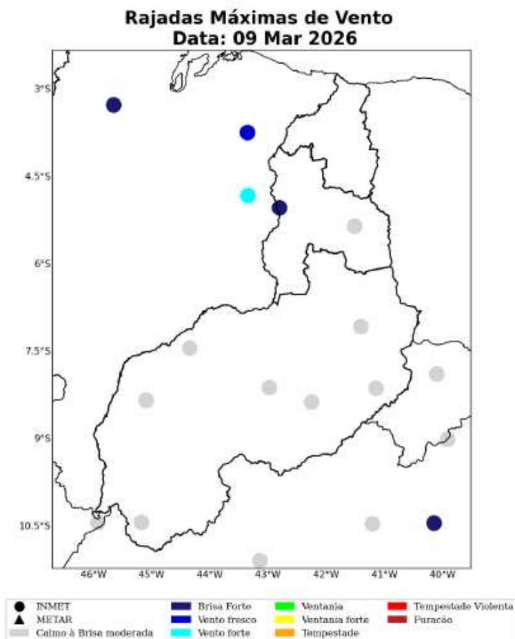
Figura 10: Máxima rajada de vento diária sobre a área de concessão da Equatorial-PI para o dia 09 de Março, baseado nas estações meteorológicas do INMET.
