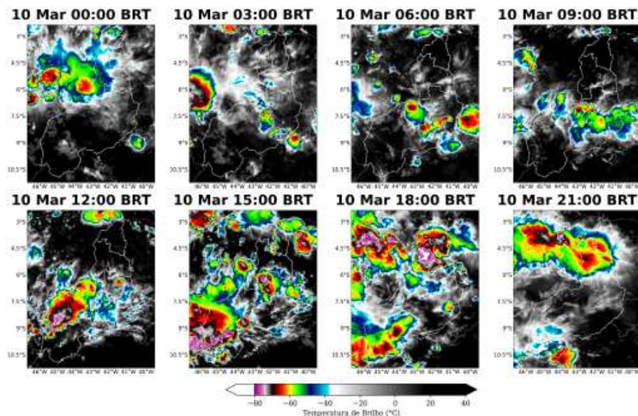
Figura 3: Imagens realçadas do satélite GOES-19 das 00 BRT até 21 BRT (a cada 3 horas) para o dia 10 de Março.
