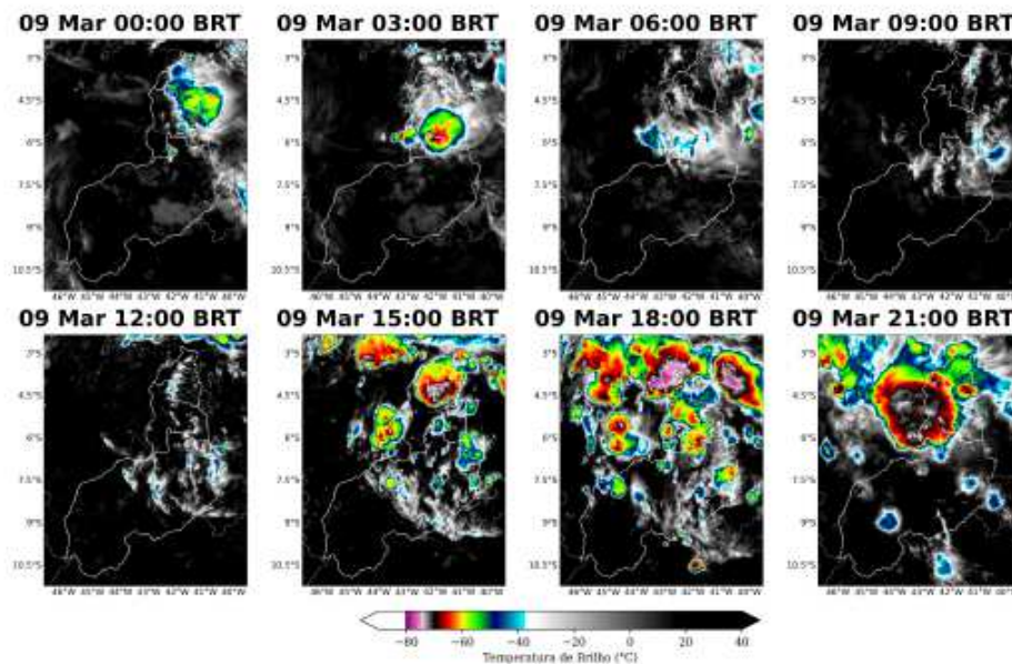
Figura 2: Imagens realçadas do satélite GOES-19 das 00 BRT até 21 BRT (a cada 3 horas) para o dia 09 de Março.
