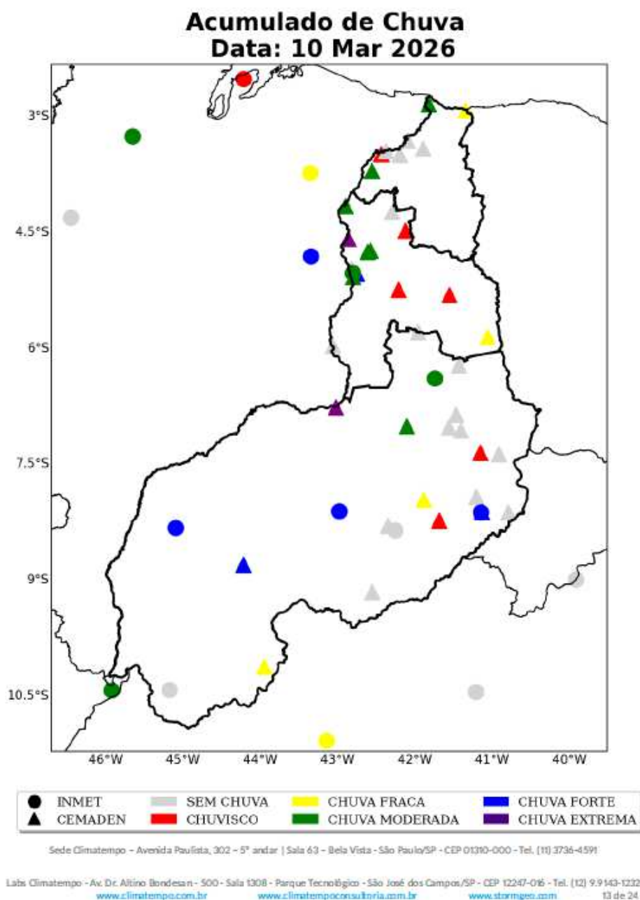
Figura 8: Acumulado diário de precipitação sobre a área de concessão da Equatorial-PI para o dia 10 de Março, baseado nas estações meteorológicas do INMET e CEMADEN.
