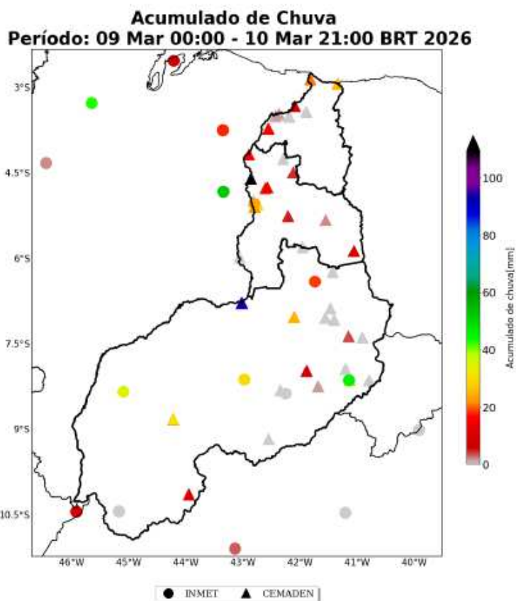
Figura 9: Acumulado de precipitação sobre a área de concessão da Equatorial-PI para o período do evento (dias 09 a 10 de Março de 2026), baseado nas estações meteorológicas do INMET e CEMADEN.
