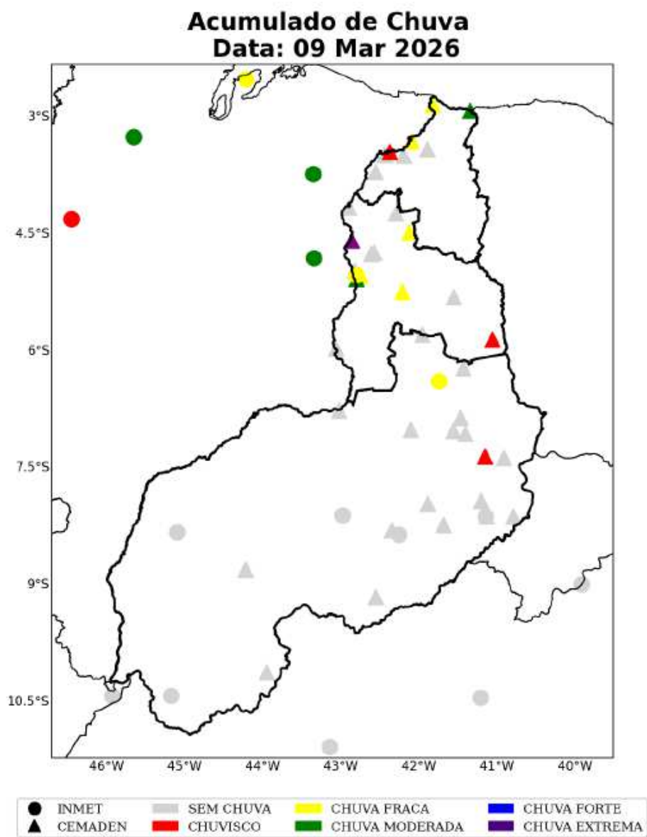
Figura 7: Acumulado diário de precipitação sobre a área de concessão da Equatorial-PI para o dia 09 de Março, baseado nas estações meteorológicas do INMET e CEMADEN.
