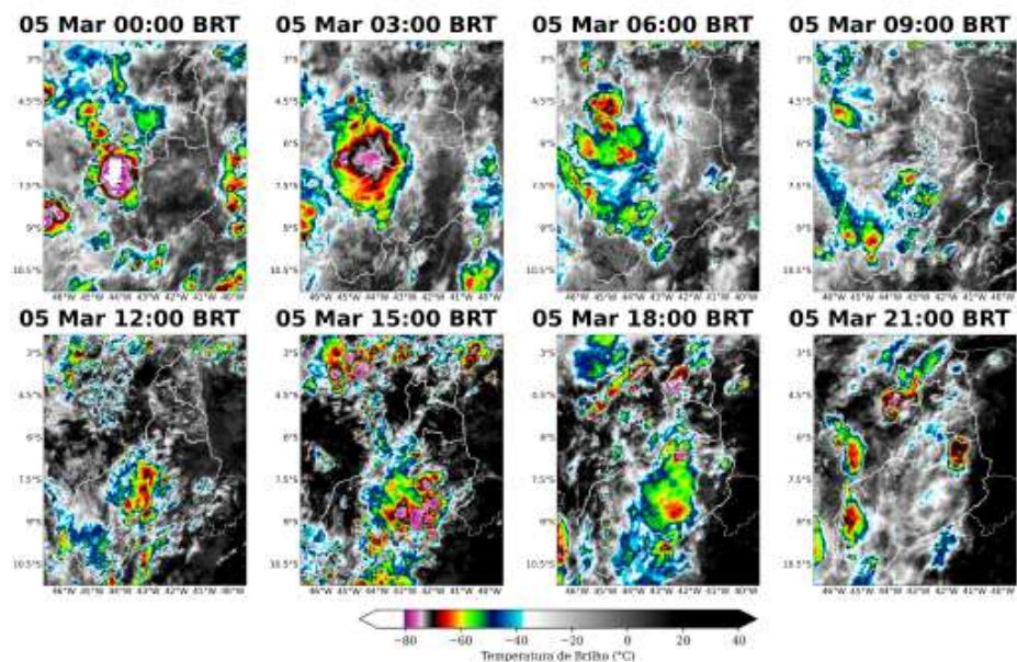
Figura 5: Imagens realçadas do satélite GOES-19 das 00 BRT até 21 BRT (a cada 3 horas) para o dia 05 de Março.
