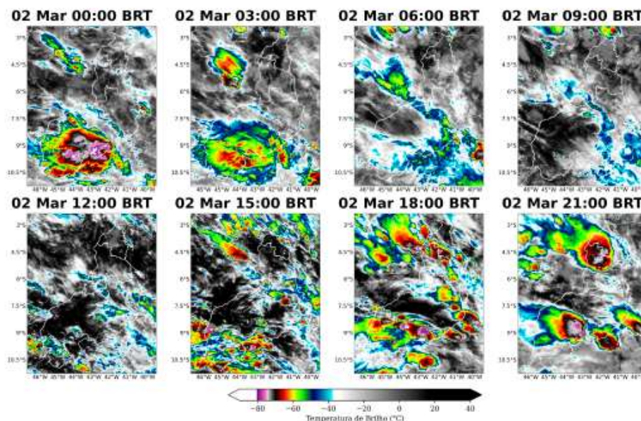
Figura 2: Imagens realçadas do satélite GOES-19 das 00 BRT até 21 BRT (a cada 3 horas) para o dia 02 de Março.
