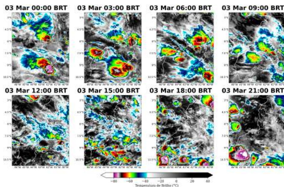
Figura 3: Imagens realçadas do satélite GOES-19 das 00BRT até 21BRT (a cada 3 horas) para o dia 03 de Março.
