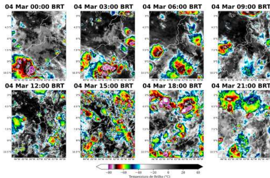
Figura 4: Imagens realçadas do satélite GOES-19 das 00 BRT até 21 BRT (a cada 3 horas) para o dia 04 de Março.
