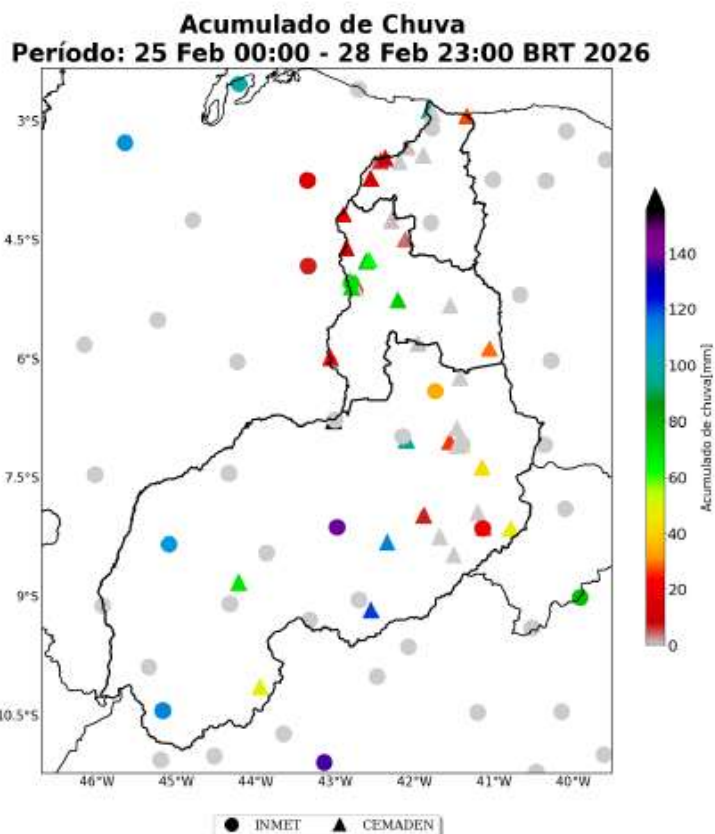
Figura 15: Acumulado de precipitação sobre o estado do Piauí para o período do evento (dias 25 a 28 de Fevereiro de 2026), baseado nas estações meteorológicas do INMET e CEMADEN.
