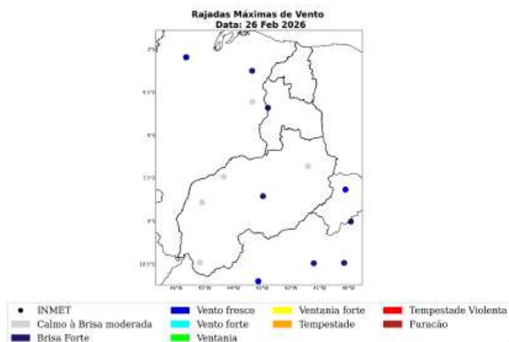
Figura 17: Máxima rajada de vento diária sobre a área de concessão da Equatorial-PI para o dia 26 de Fevereiro, baseado nas estações meteorológicas do INMET.
