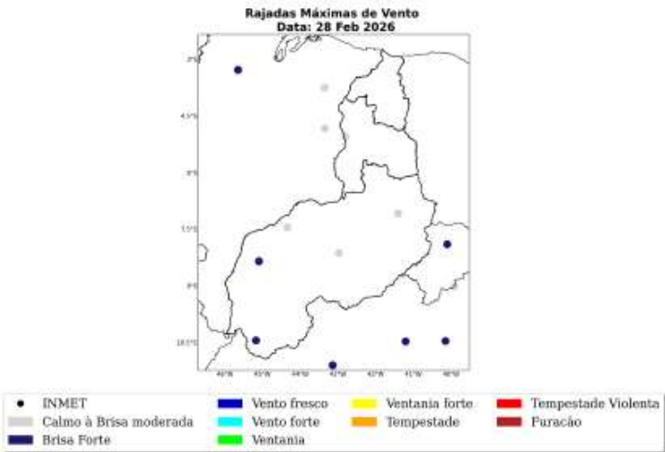
Figura 19: Máxima rajada de vento diária sobre a área de concessão da Equatorial-PI para o dia 28 de Fevereiro, baseado nas estações meteorológicas do INMET.
