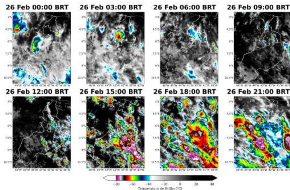
Figura 3: Imagens realçadas do satélite GOES-16 das 00 BRT até 21 BRT (a cada 3 horas) para o dia 26 de Fevereiro.
