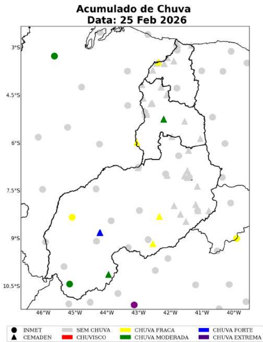
Figura 11: Acumulado diário de precipitação sobre a área de concessão da Equatorial-PI para o dia 25 de Fevereiro, baseado nas estações meteorológicas do INMET e CEMADEN.
