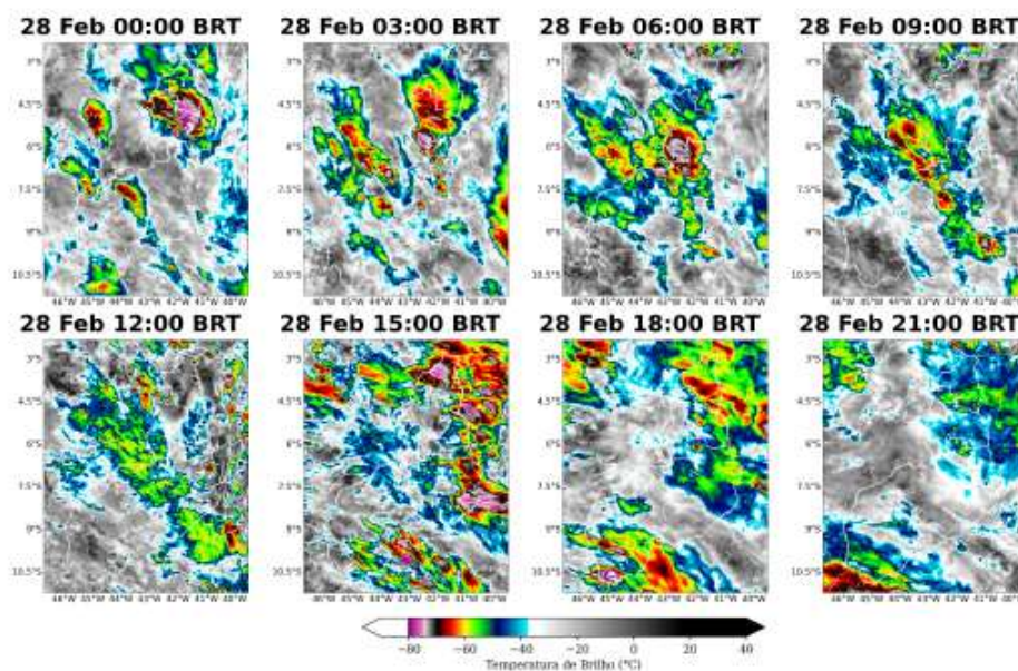
Figura 5: Imagens realçadas do satélite GOES-16 das 00 BRT até 21 BRT (a cada 3 horas) para o dia 28 de Fevereiro.
