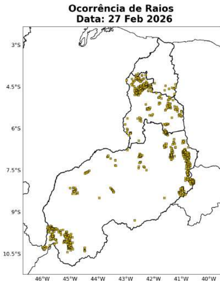
Figura 8: Ocorrências de descargas atmosféricas nuvem-solo detectadas pelo sistema Earth Networks para o dia 27 de Fevereiro sobre a área de concessão da Equatorial-PI.
