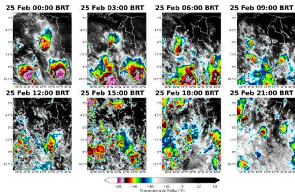
Figura 2: Imagens realçadas do satélite GOES-16 das 00 BRT até 21 BRT (a cada 3 horas) para o dia 25 de Fevereiro.
