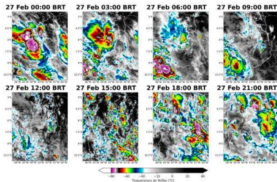
Figura 4: Imagens realçadas do satélite GOES-16 das 00 BRT até 21 BRT (a cada 3 horas) para o dia 27 de Fevereiro.
