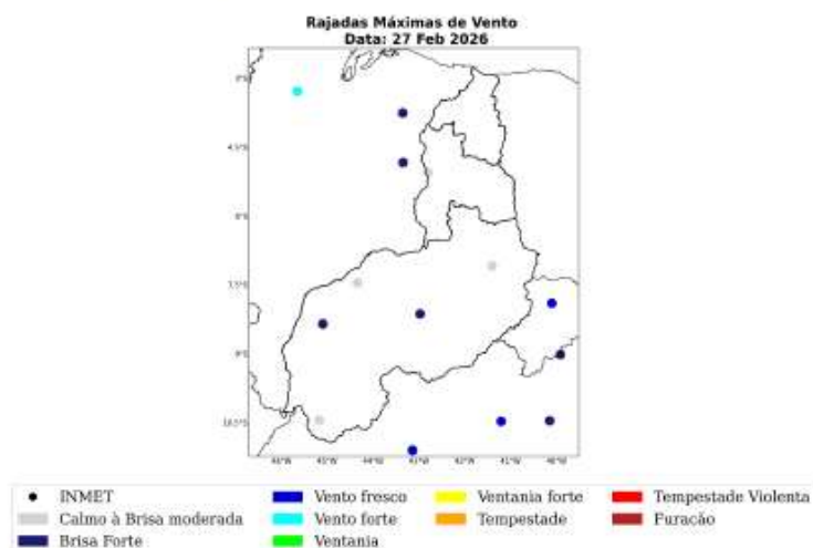
Figura 18: Máxima rajada de vento diária sobre a área de concessão da Equatorial-PI para o dia 27 de Fevereiro, baseado nas estações meteorológicas do INMET.
