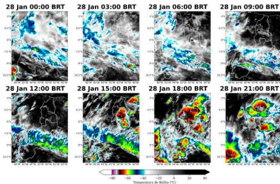
Figura 4: Imagens realçadas do satélite GOES-19 das 00 BRT até 21 BRT (a cada 3 horas) para o dia 28 de Janeiro.
