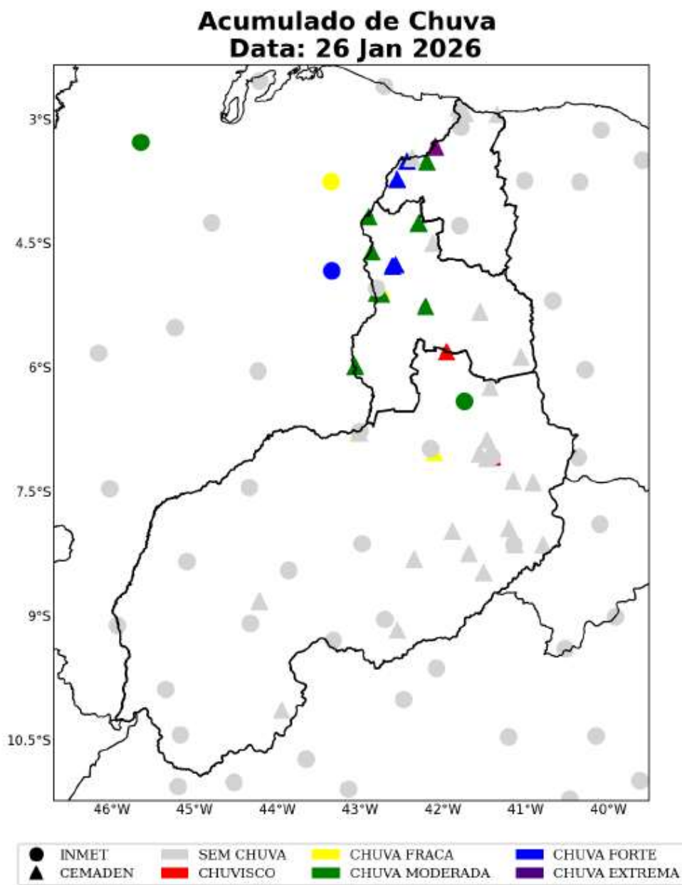
Figura 9: Acumulado diário de precipitação sobre a área de concessão da Equatorial-PI para o dia 26 de Janeiro, baseado nas estações meteorológicas do INMET e CEMADEN.
