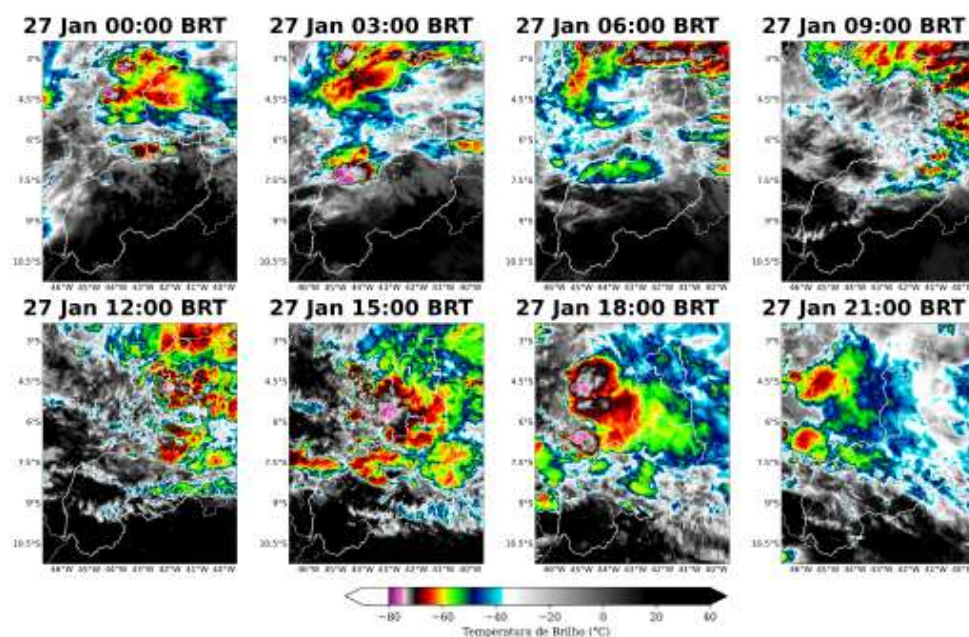
Figura 3: Imagens realçadas do satélite GOES-19 das 00 BRT até 21 BRT (a cada 3 horas) para o dia 27 de Janeiro.
