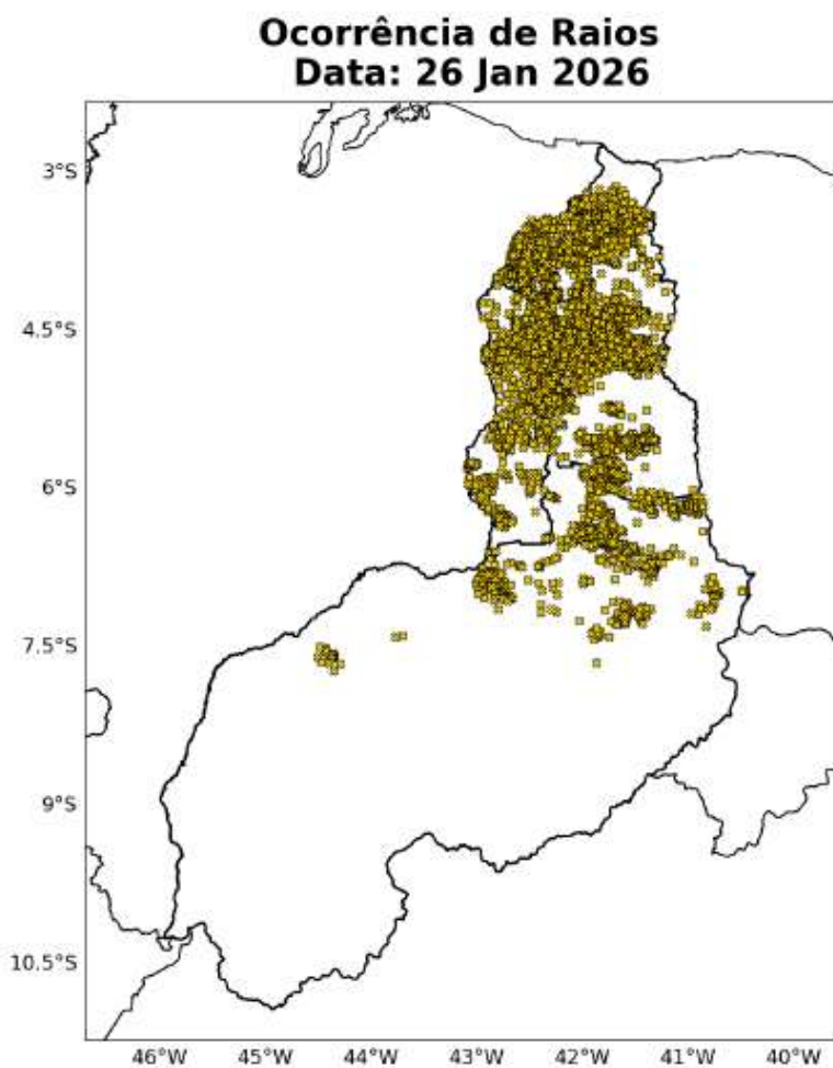
Figura 5: Ocorrências de descargas atmosféricas nuvem-solo detectadas pelo sistema Earth Networks para o dia 26 de Janeiro sobre a área de concessão da Equatorial-PI.
