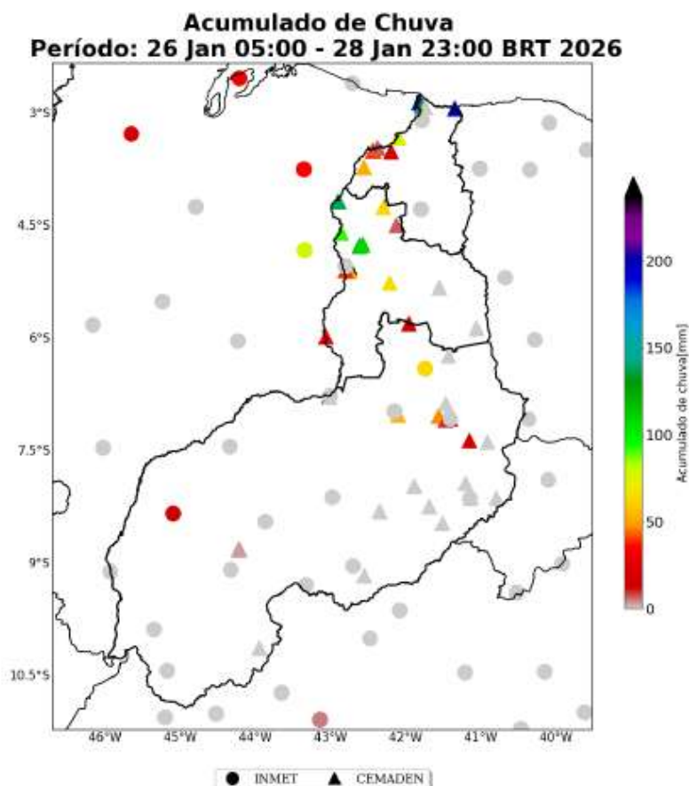
Figura 12: Acumulado de precipitação sobre a área de concessão da Equatorial-PI para o período do evento (dias 26 a 28 de Janeiro de 2026), baseado nas estações meteorológicas do INMET e CEMADEN.
