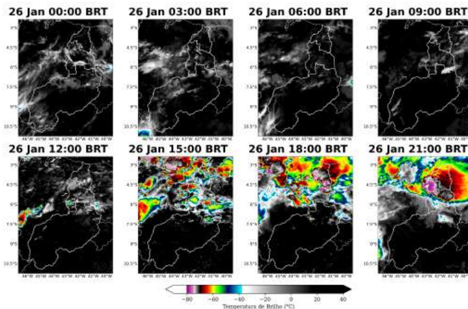
Figura 2: Imagens realçadas do satélite GOES-19 das 00 BRT até 21 BRT (a cada 3 horas) para o dia 26 de Janeiro.
