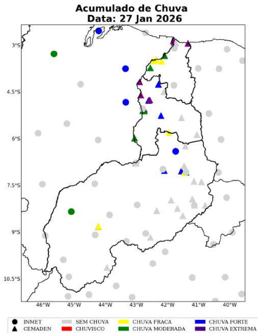
Figura 10: Acumulado do diário de precipitação sobre a área de concessão da Equatorial-PI para o dia 27 de Janeiro, baseado nas estações meteorológicas do INMET e CEMADEN.
