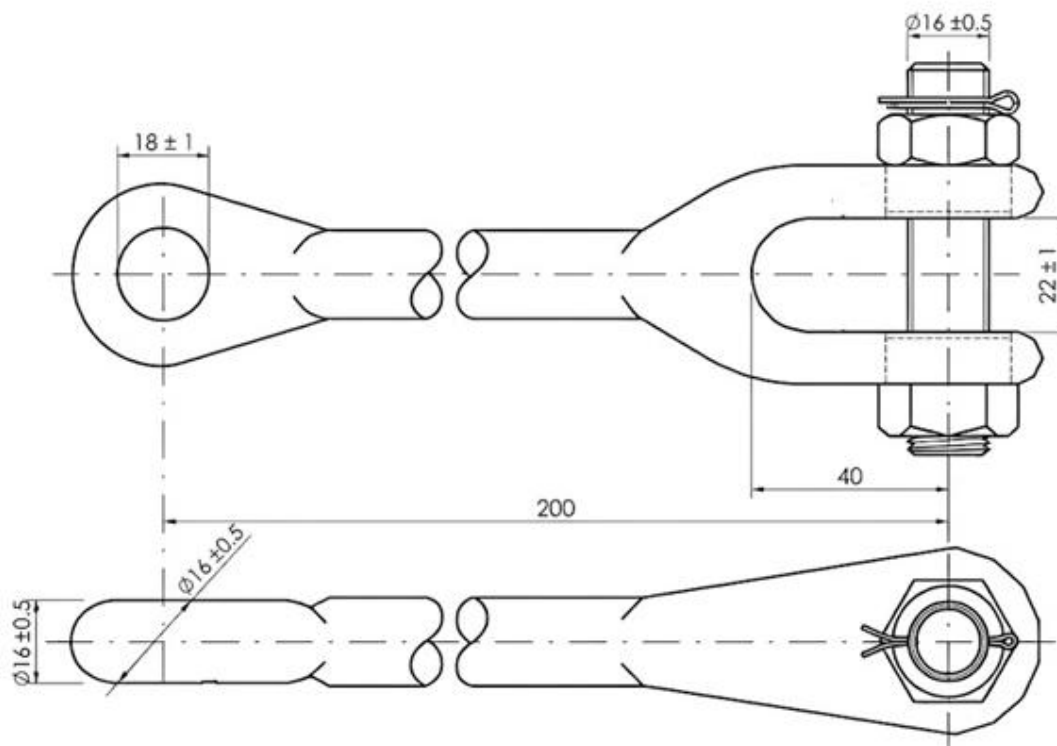
Desenho 1 – Prolongador Garfo Olhal 90° – Detalhes Construtivos
