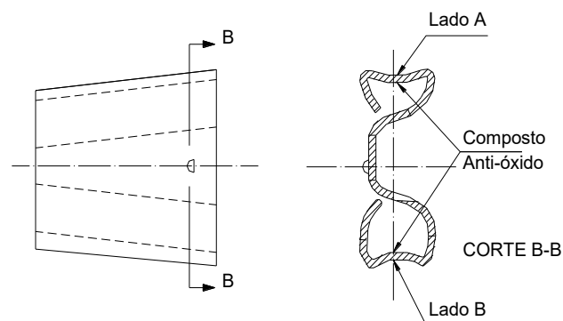
FIGURA 2 - COMPONENTE "CUNHA"
