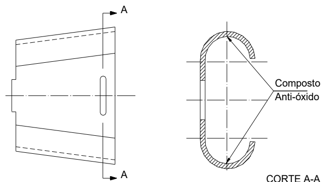
FIGURA 1 - COMPONENTE "C"
