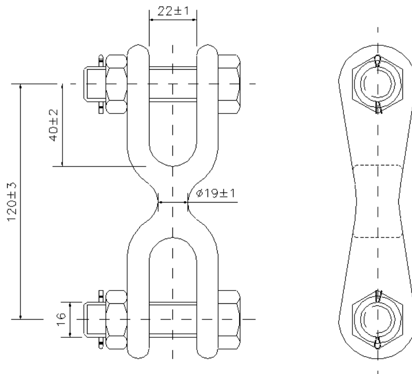
Desenho 1 – Engate Garfo-Garfo – Detalhes Construtivos
