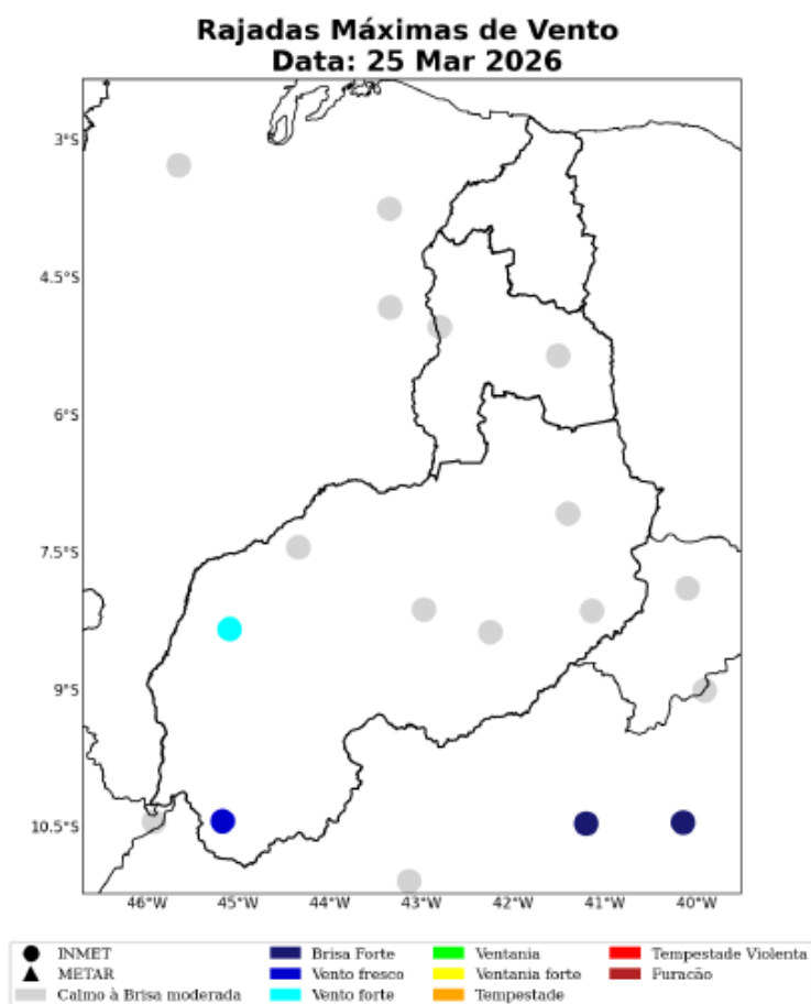
Figura 15: Máxima rajada de vento diária sobre a área de concessão da Equatorial-PI para o dia 25 de Março, baseado nas estações meteorológicas do INMET.
