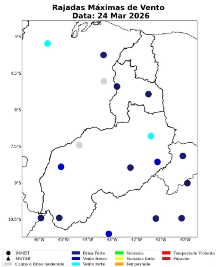
Figura 14: Máxima rajada de vento diária sobre a área de concessão da Equatorial-PI para o dia 24 de Março, baseado nas estações meteorológicas do INMET.
