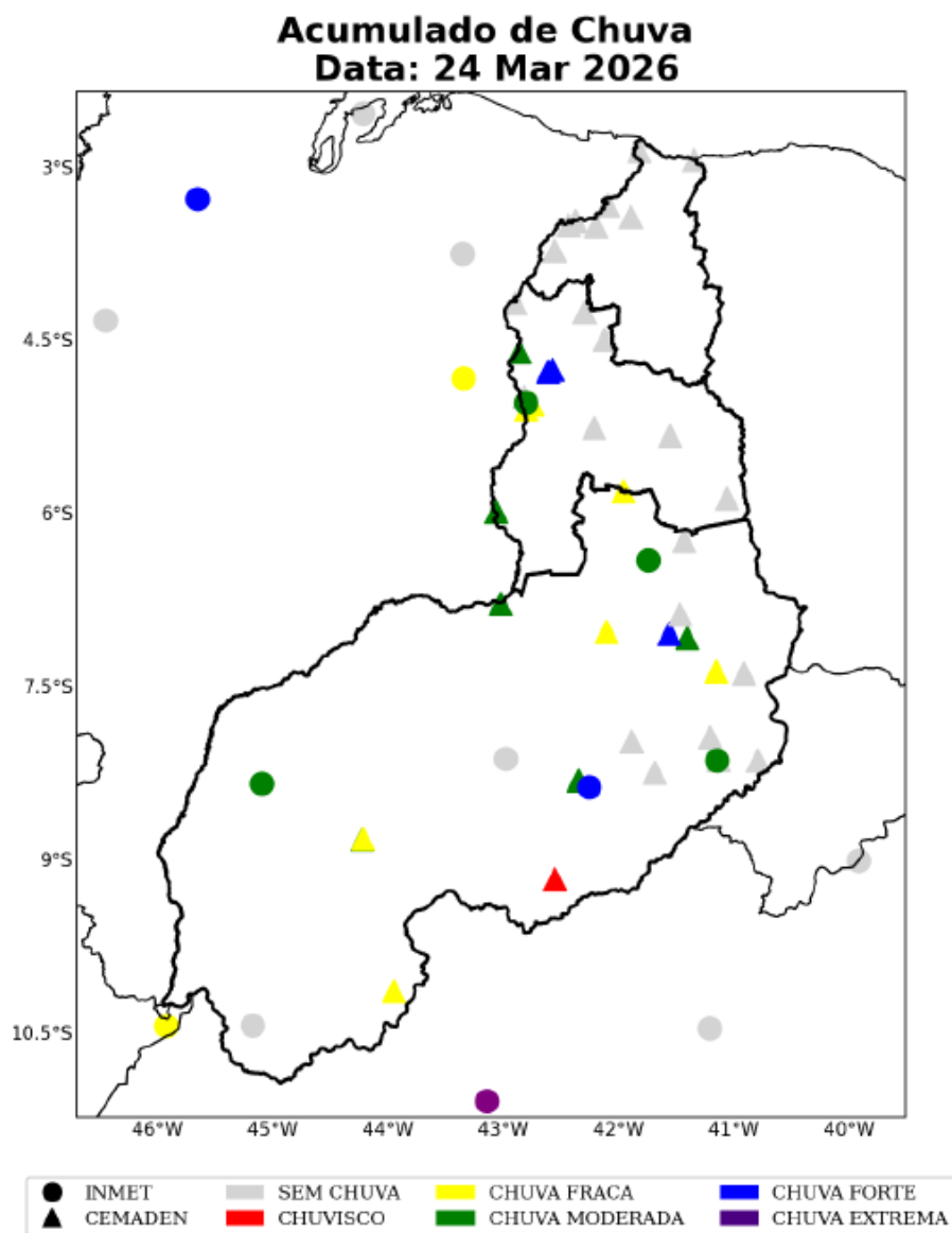
Figura 10: Acumulado diário de precipitação sobre a área de concessão da Equatorial-PI para o dia 24 de Março, baseado nas estações meteorológicas do INMET e CEMADEN.
