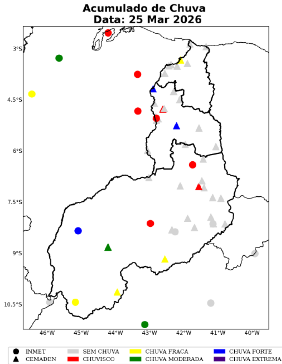
Figura 11: Acumulado diário de precipitação sobre a área de concessão da Equatorial-PI para o dia 25 de Março, baseado nas estações meteorológicas do INMET e CEMADEN.
