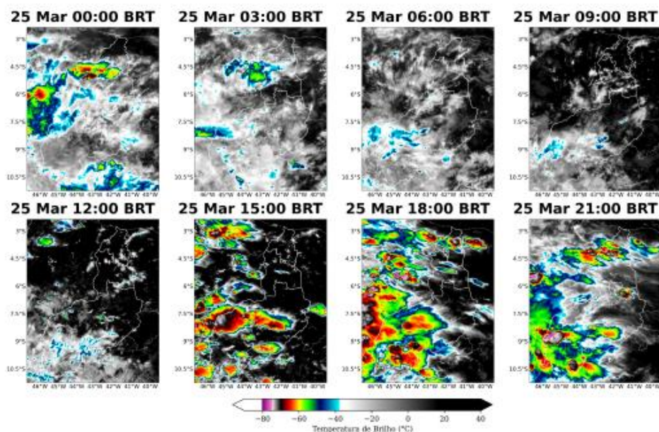
Figura 4: Imagens realçadas do satélite GOES-19 das 00 BRT até 21 BRT (a cada 3 horas) para o dia 25 de Março.
