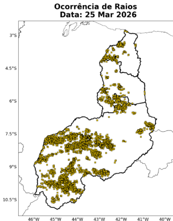
Figura 7: Ocorrências de descargas atmosféricas nuvem-solo detectadas pelo sistema Earth Networks para o dia 25 de Março sobre a área de concessão da Equatorial-PI.
