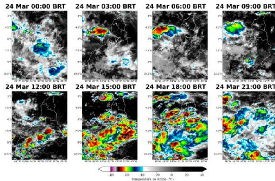
Figura 3: Imagens realçadas do satélite GOES-19 das 00 BRT até 21 BRT (a cada 3 horas) para o dia 24 de Março.
