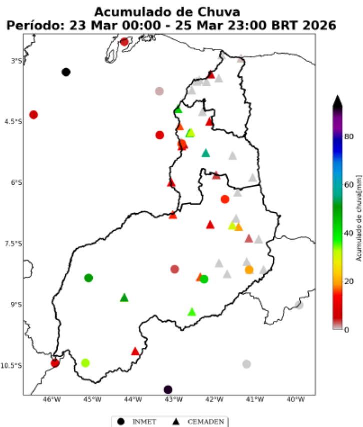
Figura 12: Acumulado de precipitação sobre a área de concessão da Equatorial-PI para o período do evento (dias 23 a 25 de Março de 2026), baseado nas estações meteorológicas do INMET e CEMADEN.
