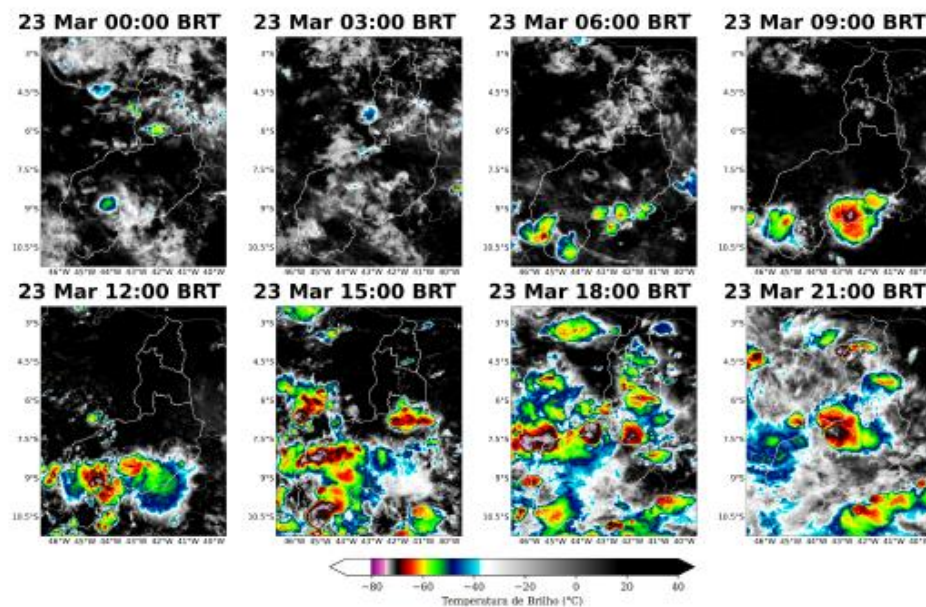
Figura 2: Imagens realçadas do satélite GOES-19 das 00 BRT até 21 BRT (a cada 3 horas) para o dia 23 de Março.
