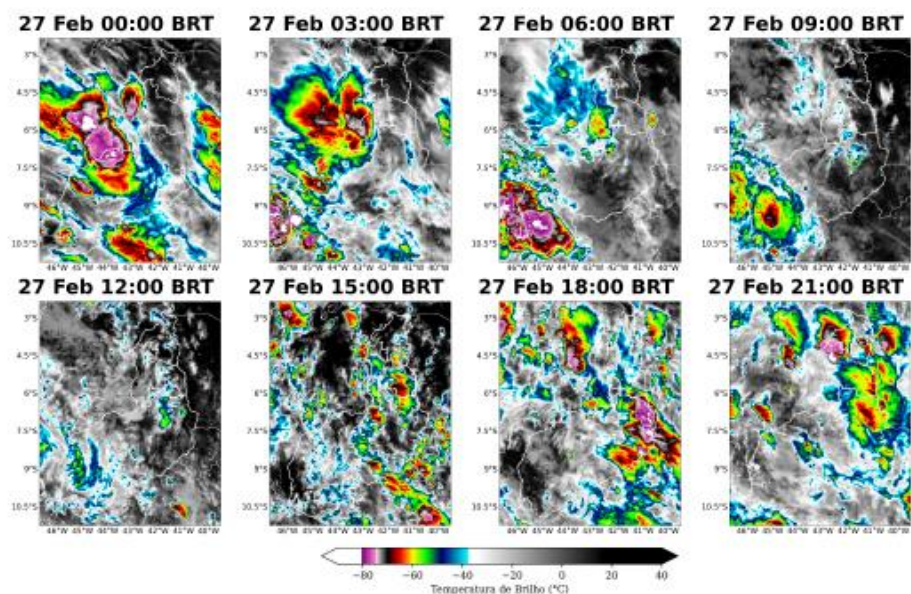
Figura 4: Imagens realçadas do satélite GOES-16 das 00 BRT até 21 BRT (a cada 3 horas) para o dia 27 de Fevereiro.
