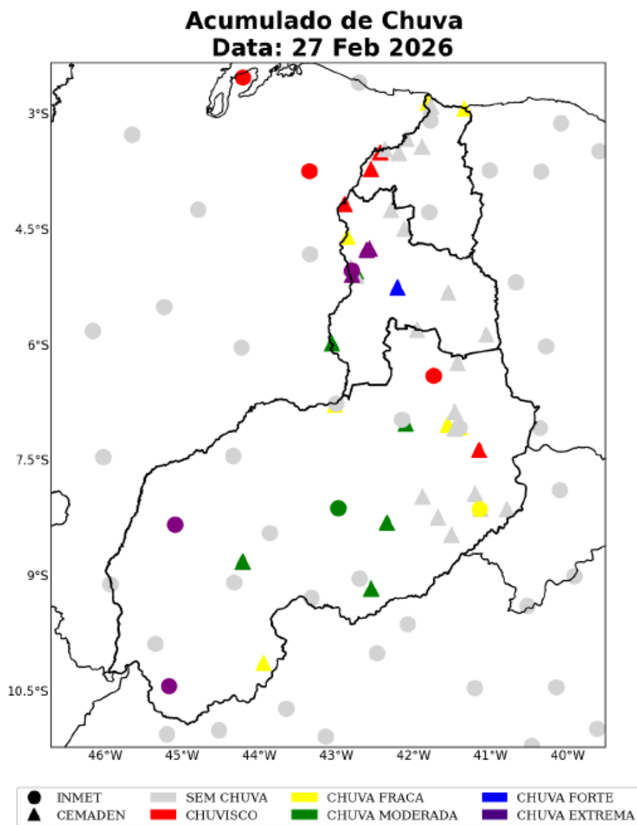
Figura 13: Acumulado diário de precipitação sobre a área de concessão da Equatorial-PI para o dia 27 de Fevereiro, baseado nas estações meteorológicas do INMET e CEMADEN.
