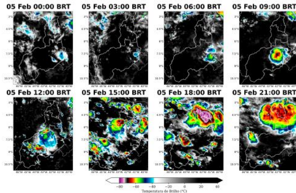
Figura 2: Imagens realçadas do satélite GOES-19 das 00 BRT até 21 BRT (a cada 3 horas) para o dia 05 de Fevereiro.
