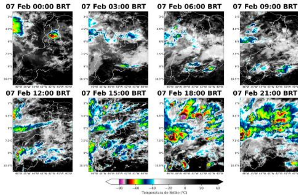
Figura 4: Imagens realçadas do satélite GOES-19 das 00 BRT até 21 BRT (a cada 3 horas) para o dia 07 de Fevereiro.
