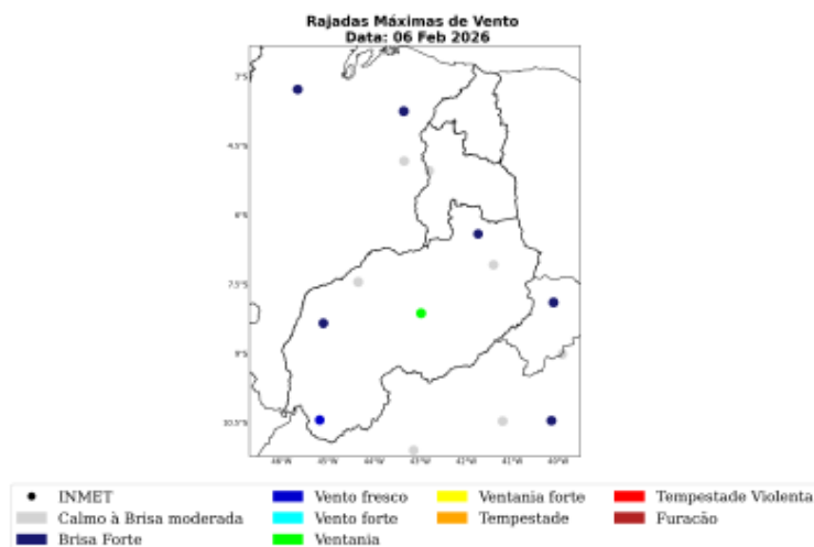
Figura 17: Máxima rajada de vento diária sobre a área de concessão da Equatorial-PI para o dia 06 de Fevereiro, baseado nas estações meteorológicas do INMET.
