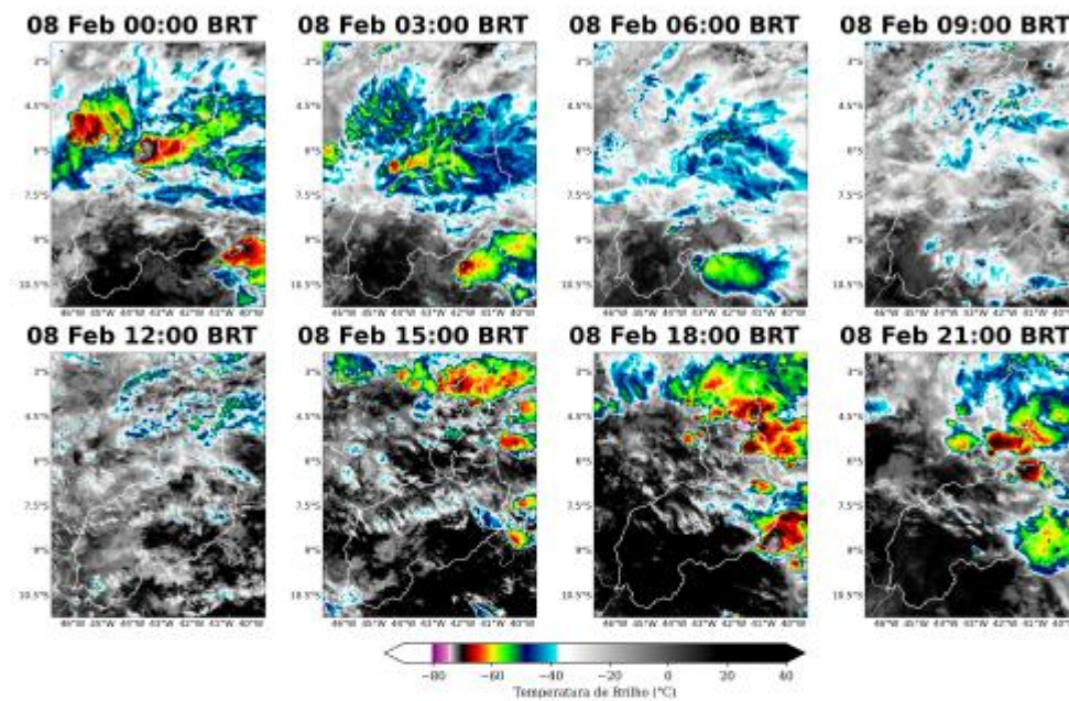
Figura 5: Imagens realçadas do satélite GOES-19 das 00 BRT até 21 BRT (a cada 3 horas) para o dia 08 de Fevereiro.
