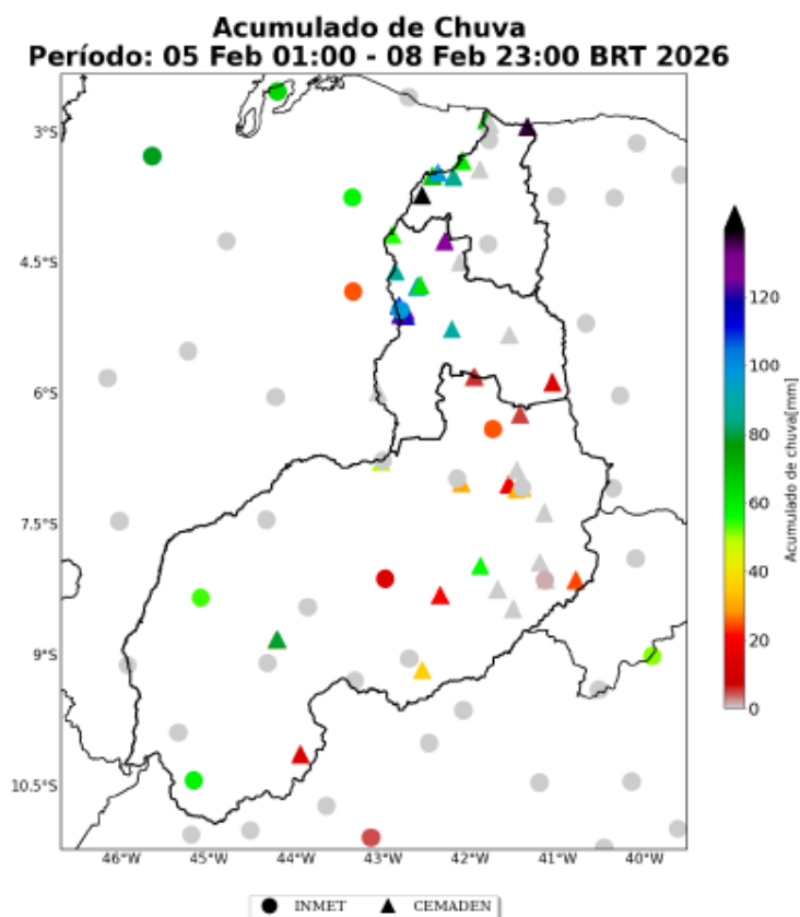
Figura 15: Acumulado de precipitação sobre a área de concessão da Equatorial-PI para o período do evento (dias 05 a 08 de Fevereiro de 2026), baseado nas estações meteorológicas do INMET e CEMADEN.
