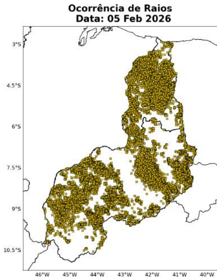
Figura 6: Ocorrências de descargas atmosféricas nuvem-solo detectadas pelo sistema Earth Networks para o dia 05 de Fevereiro sobre a área de concessão da Equatorial-PI.
