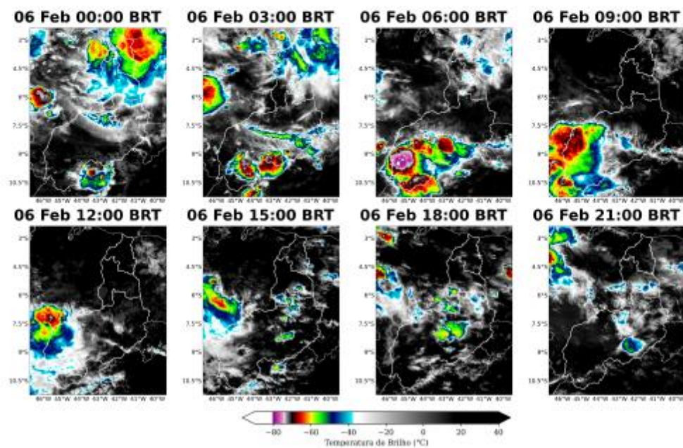
Figura 3: Imagens realizadas do satélite GOES-19 das 00 BRT até 21 BRT (a cada 3 horas) para o dia 06 de Fevereiro.
