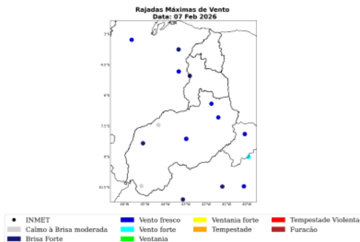
Figura 18: Máxima rajada de vento diária sobre a área de concessão da Equatorial-PI para o dia 07 de Fevereiro, baseado nas estações meteorológicas do INMET.
