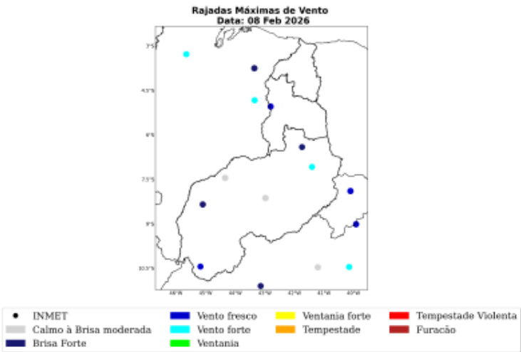
Figura 19: Máxima rajada de vento diária sobre a área de concessão da Equatorial-PI para o dia 08 de Fevereiro, baseado nas estações meteorológicas do INMET.
