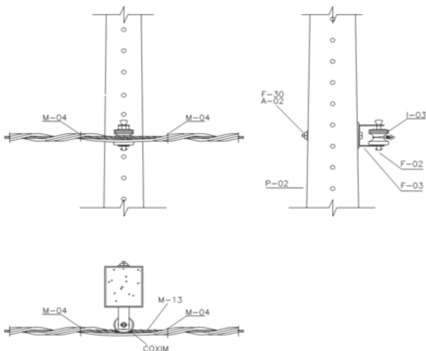
Desenho 29 - Rede de Baixa Tensão (Secundária Multiplexada) – Estrutura de passagem S1I
