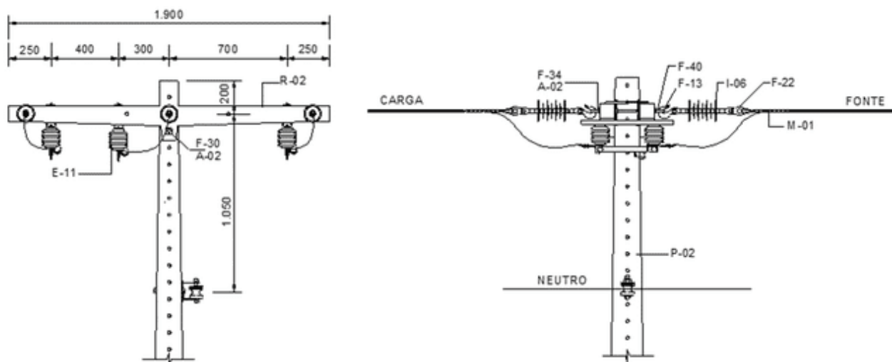
Quadro 128 - Lista de Materiais referente ao Desenho 115 – Chave faca em alinhamento
