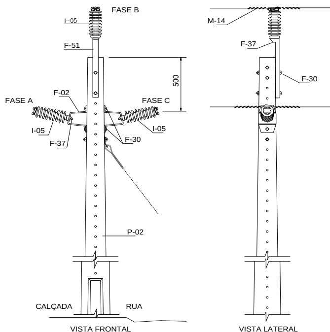
Quadro 98 - Lista de Materiais referente ao Desenho 93 – Estrutura PTA1
