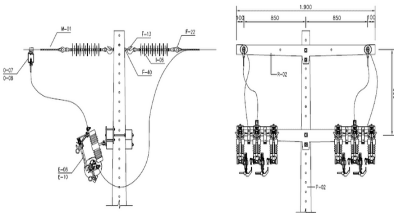
Desenho 123 - Chaves e equipamentos – Estrutura N4B-NS CR.
