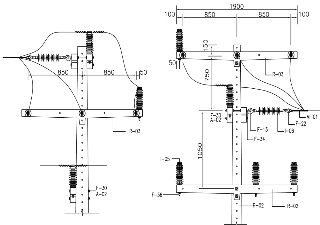
Quadro 78 - Lista de Materiais referente ao Desenho 82 – Estrutura N3-N3-N1
