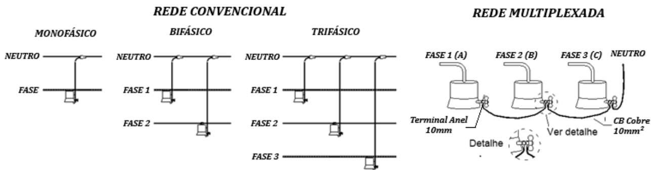
Desenho 135 Chaves e equipamentos - Baixa Tensão - PRBT - Detalhes da Ligações - MRT
