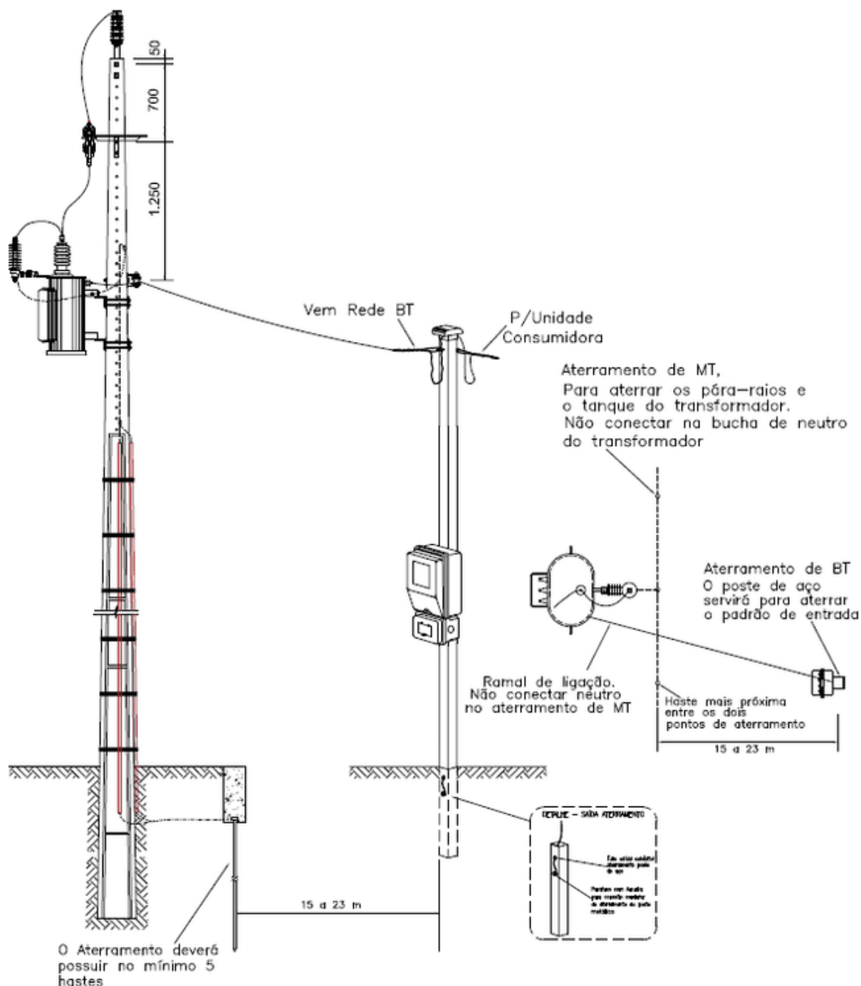
Desenho 160 - Detalhe da entrada de serviço. Posto de Transformação em Tangência - MRT
