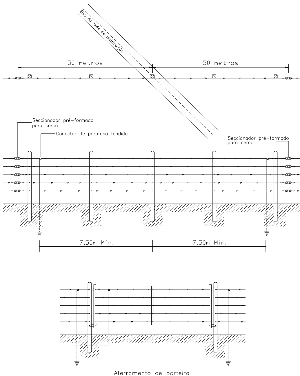
Desenho 158 - Aterramento de cerca – Cerca transversal
