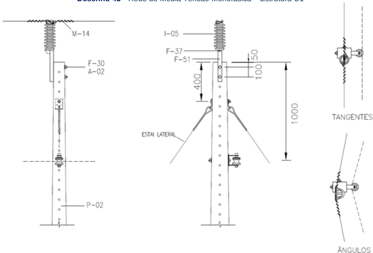
Desenho 43 - Rede de Média Tensão Monofásica – Estrutura U1
