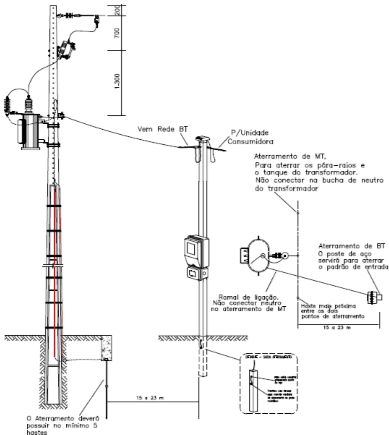
Desenho 161 - Detalhe da entrada de serviço. Posto de Transformação em fim de linha - MRT
