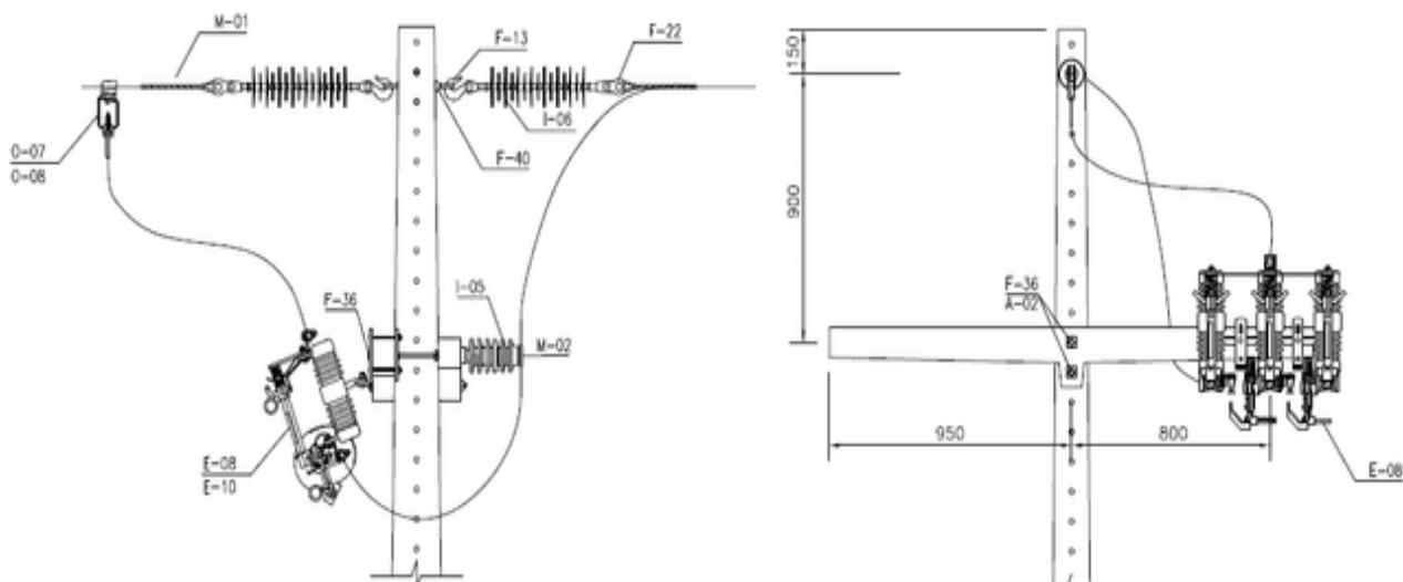
Quadro 134 - Lista de Materiais referente ao Desenho 122 – Estrutura UP4-CR
