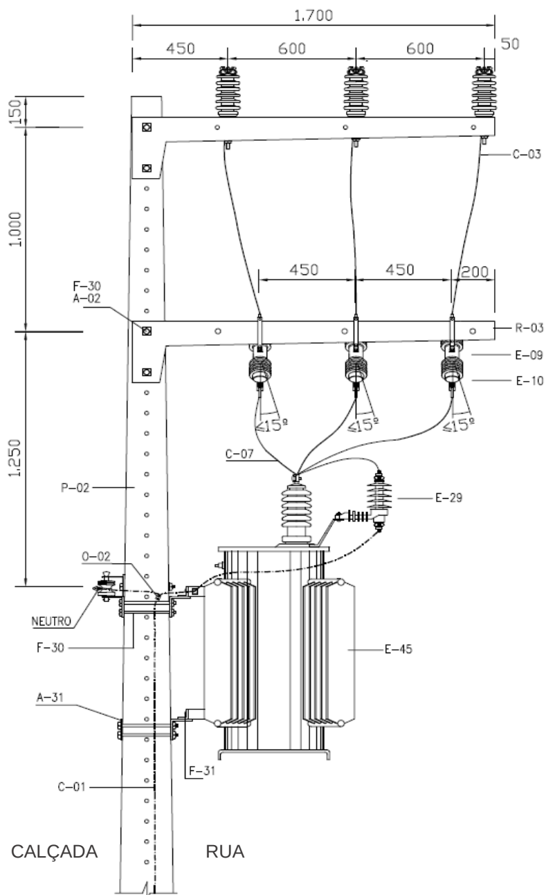
Desenho 118 - Chaves e equipamentos – Transformador trifásico – Estrutura beco B1-BS.
