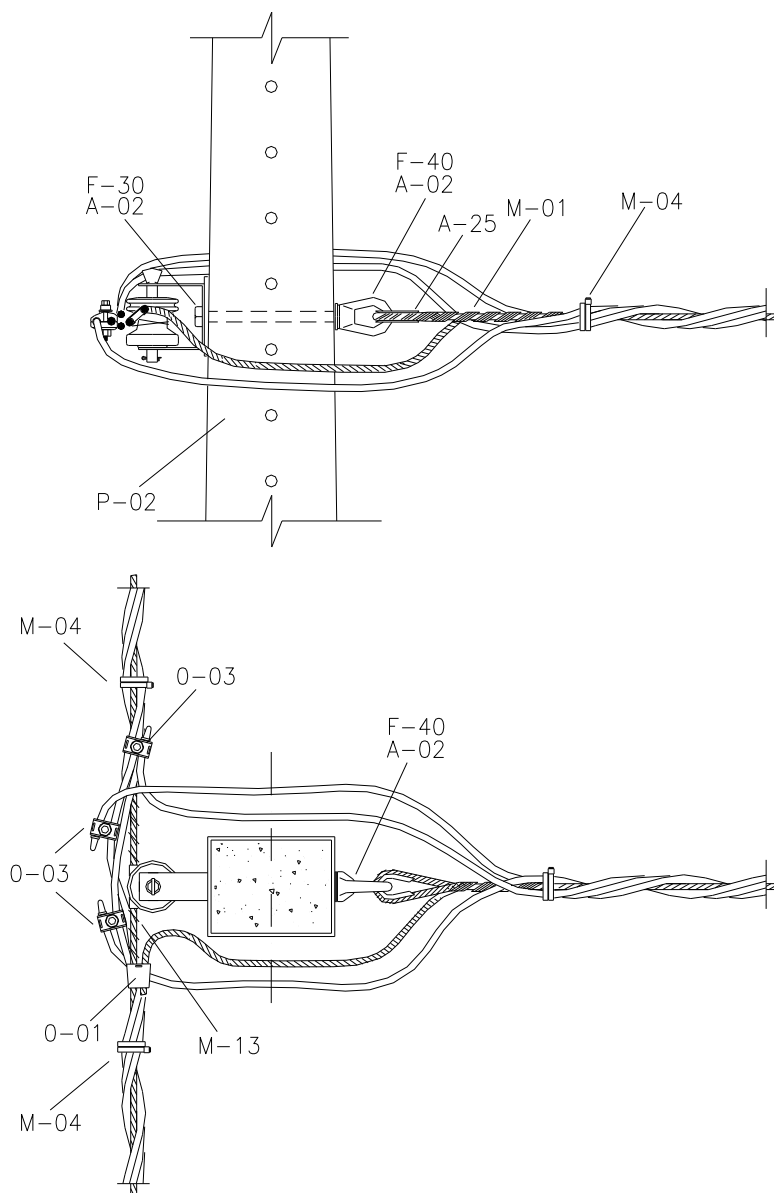
Desenho 33- Rede de Baixa Tensão (Secundária Multiplexada) – Estrutura de derivação tangente oposta (S1I-S3I OP).
