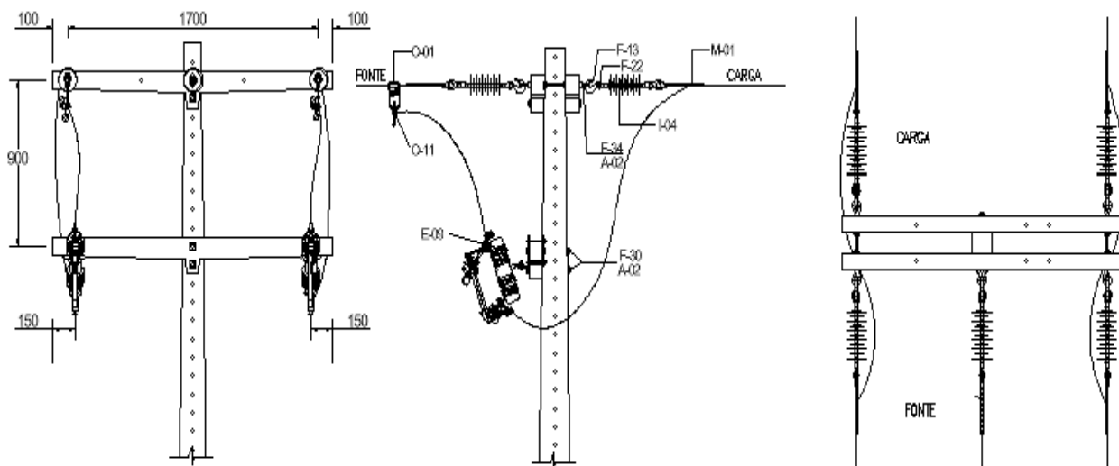
Quadro 51 - Lista de Materiais referente ao Desenho 67 – Estrutura N4T-B.
