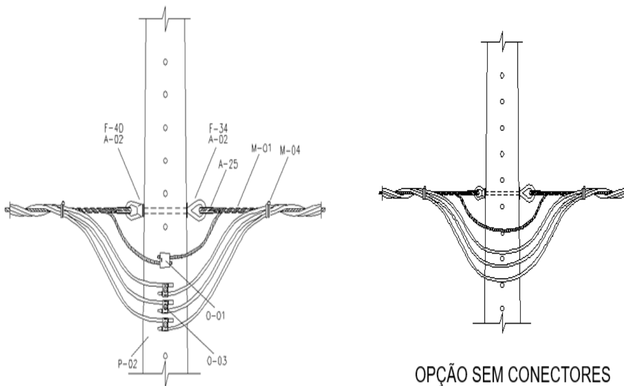
Desenho 36 - Rede de Baixa Tensão (Secundária Multiplexada) – Estrutura de amarração sem seccionamento S4I
