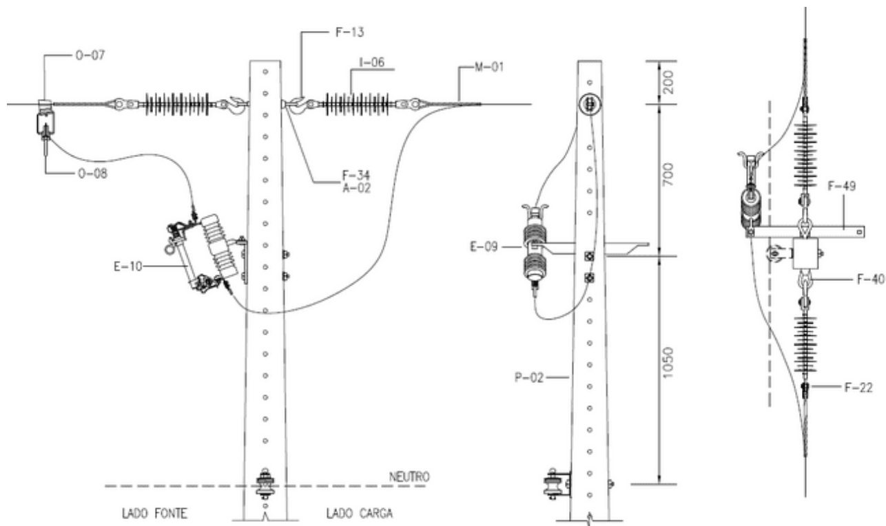
Quadro 124 - Lista de Materiais referente ao Desenho 110 – Chave Fusível Derivação Monofásica U4
