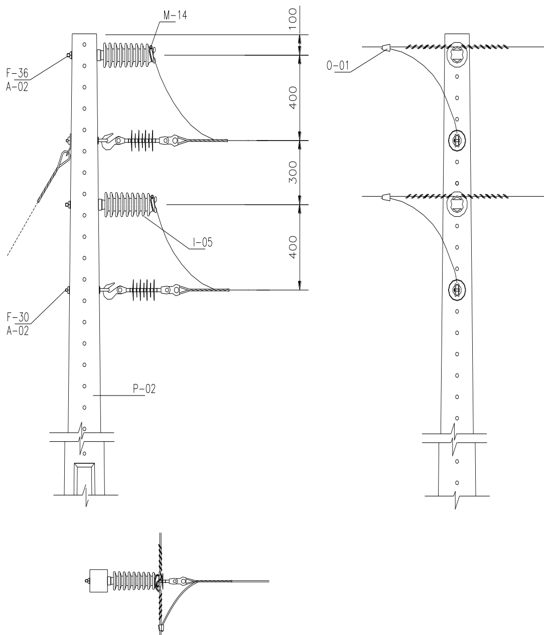
Desenho 60 - Rede de Média Tensão Bifásica – Estrutura BP1-BP3
