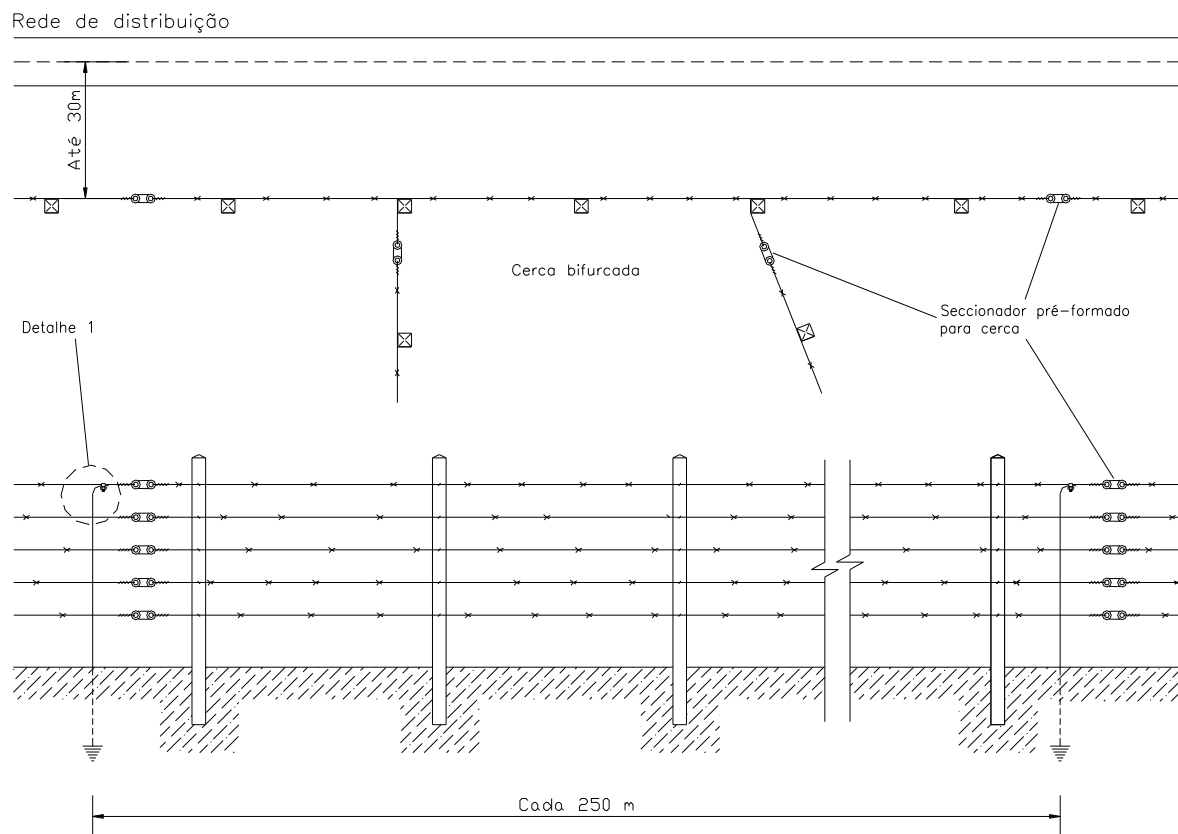
Desenho 159 - Aterramento e seccionamento de cerca – Cerca paralela
