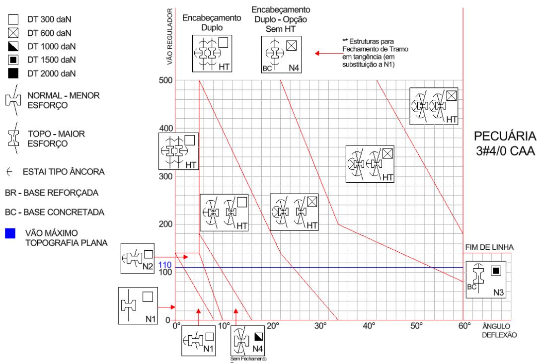
Desenho 168 - Ábaco para estruturas trifásicas tipo Normal cabo 4/0 CAA em áreas de Pecuária
