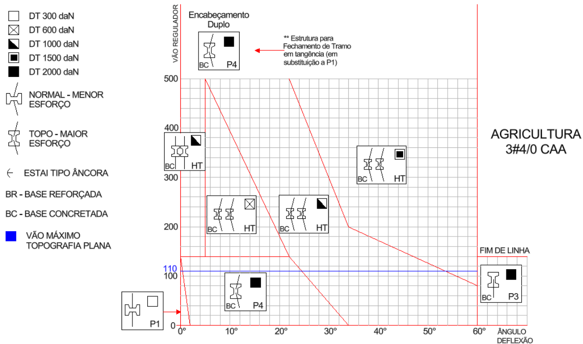
Desenho 174 - Ábaco para aplicação de estruturas trifásicas tipo Pilar no Poste (P) cabo 4/0 CAA em áreas de Agricultura
