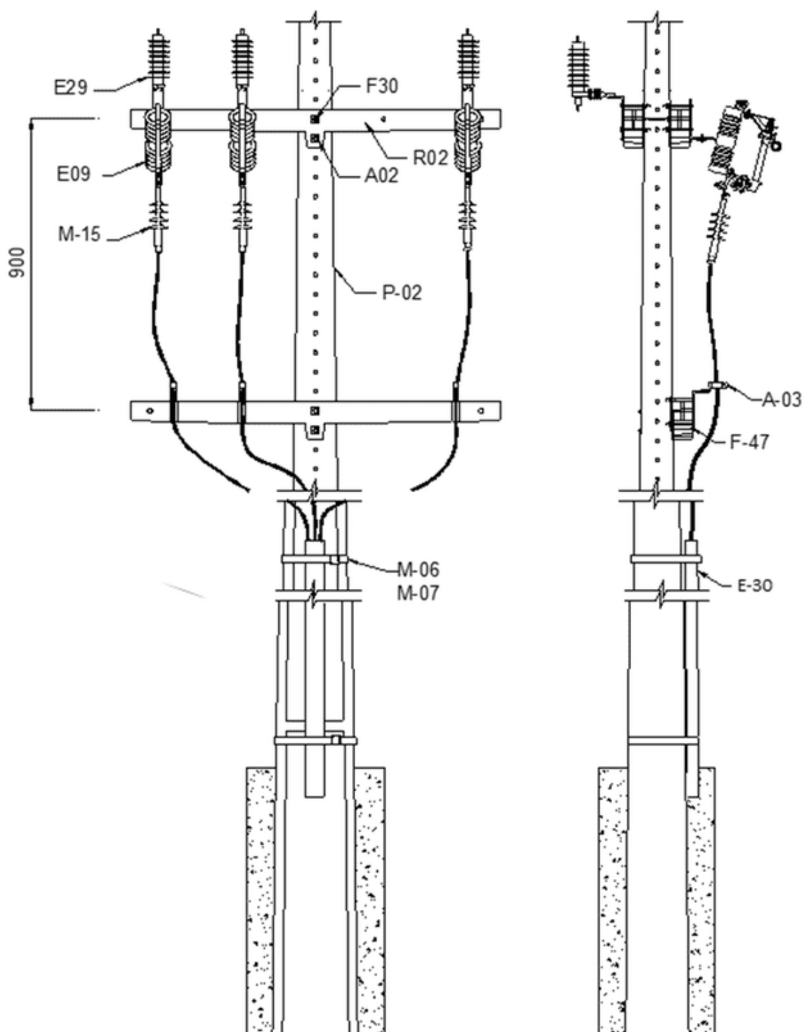
Desenho 131 - Chaves e equipamentos - Estrutura para mufla com chave fusível - Padrão existente (manutenção)
