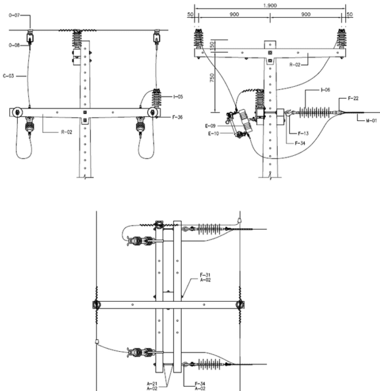
Desenho 127 - Chaves e equipamentos – Estrutura de derivação com chave fusível- N1B- N3B-CF
