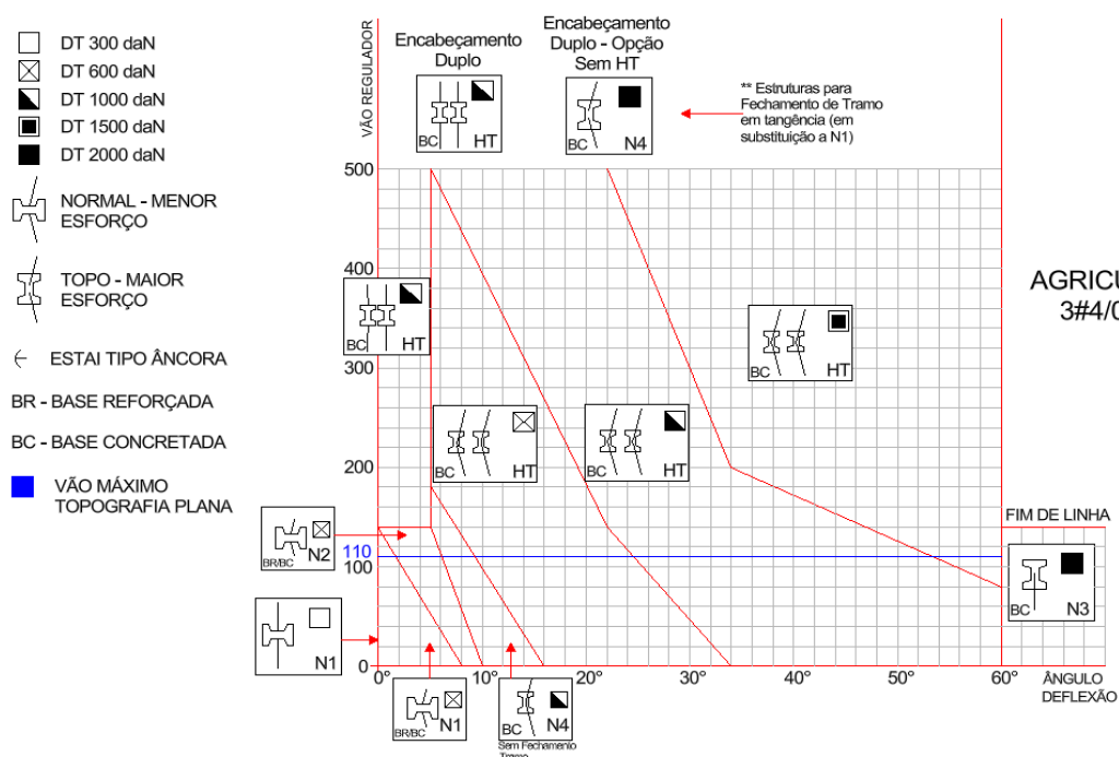
Desenho 167 - Ábaco para estruturas trifásicas tipo Normal cabo 4/0 CAA em áreas de Agricultura
