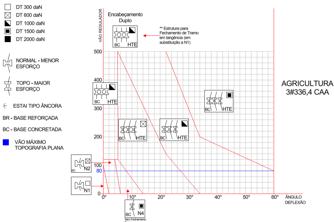
Desenho 169 - Ábaco para estruturas trifásicas tipo Normal cabo 336,4 MCM CAA em áreas de Agricultura
