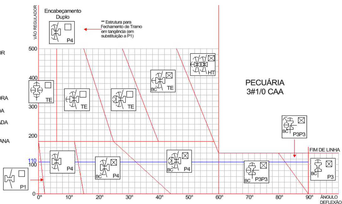
Desenho 171 - Ábaco para estruturas trifásicas tipo Pilar no Poste (P) cabo 1/0 CAA em áreas de Pecuária
