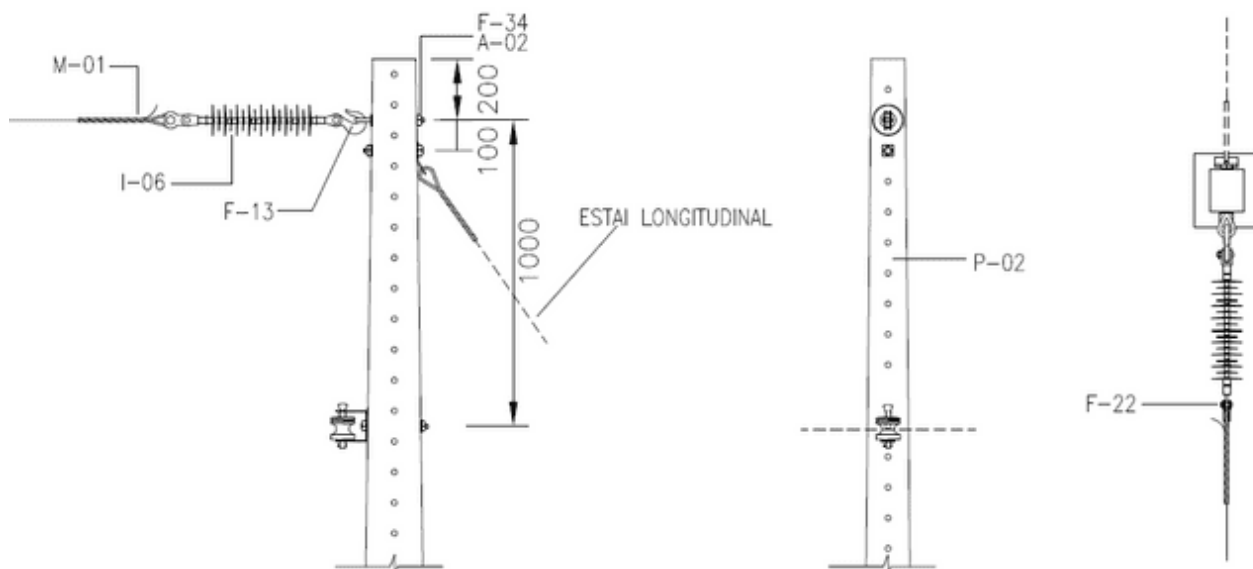
Quadro 22 - Lista de Materiais referente ao Desenho 50 – Estrutura UP3
