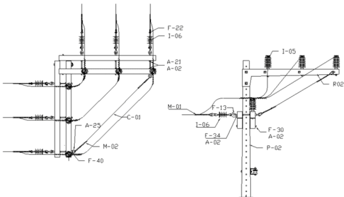
Desenho 75 - Rede de Média Tensão Trifásica – Estrutura B3-B3
