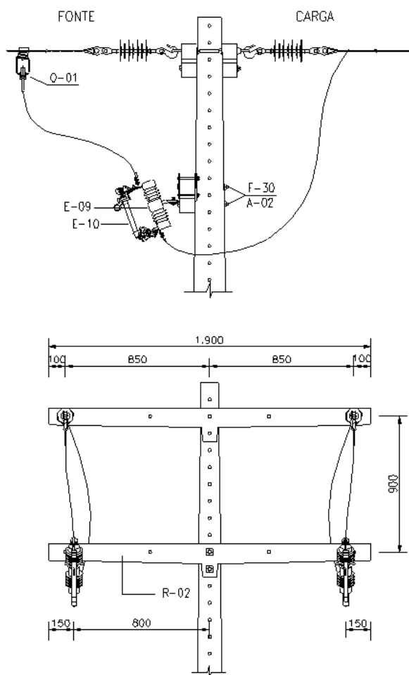
Desenho 125 - Chaves e equipamentos – Estrutura com chave fusível - N4B-NSCF
