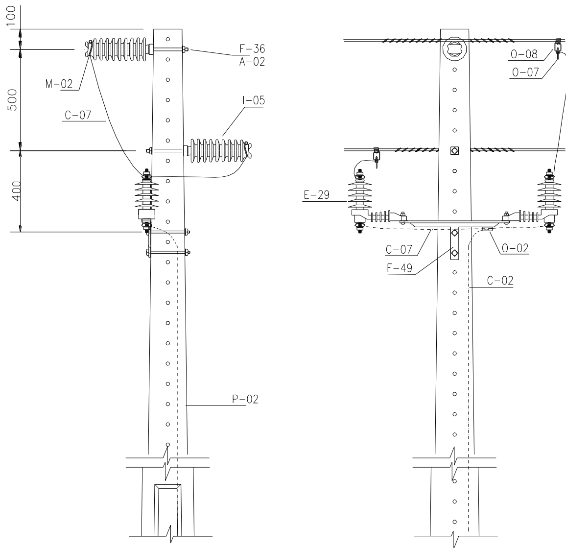
Desenho 61 - Rede de Média Tensão Bifásica – Estrutura com para-raios- BP1A-PR
