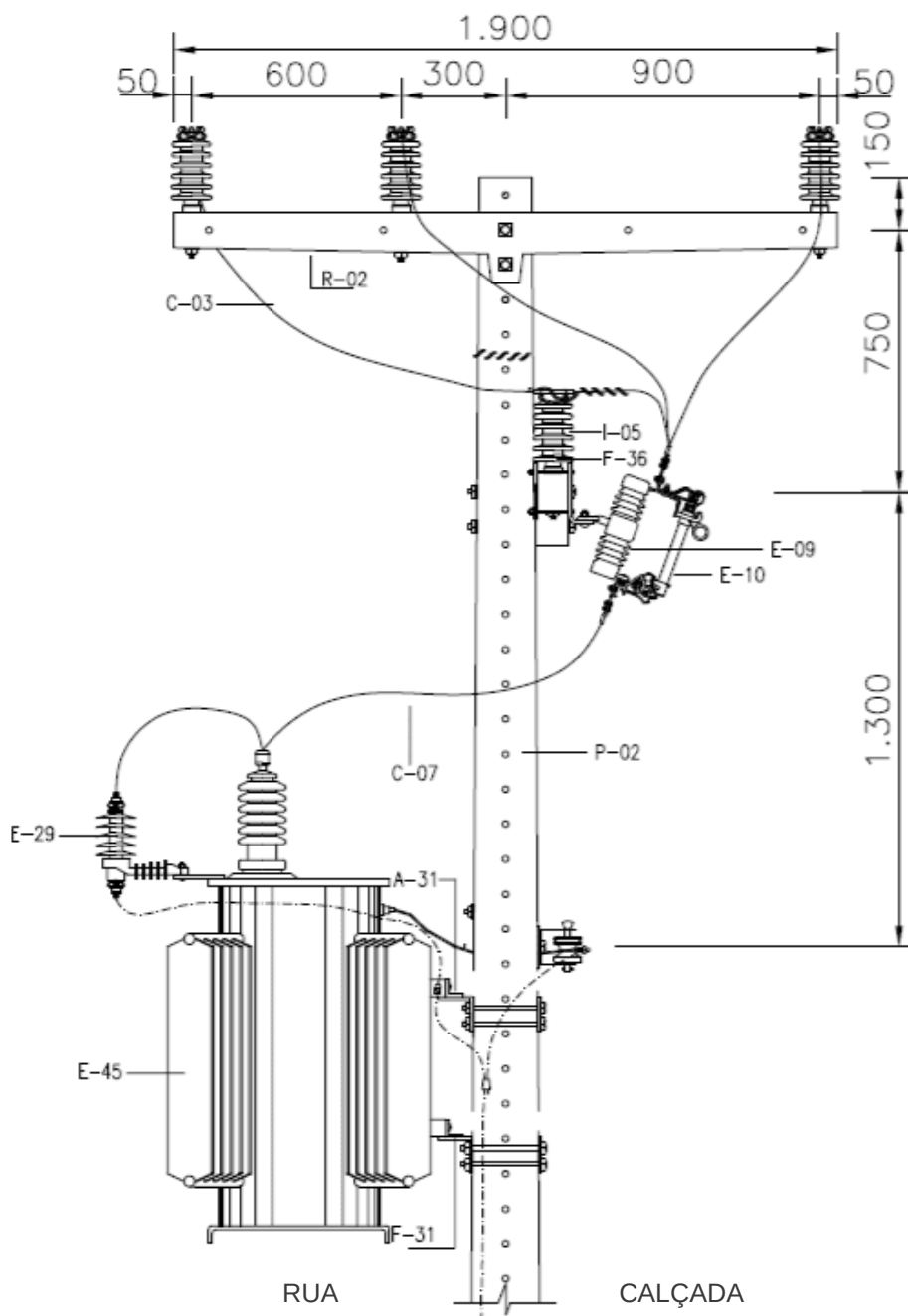
Desenho 119 - Chaves e equipamentos – Transformador trifásico – Estrutura normal N1-NS.
