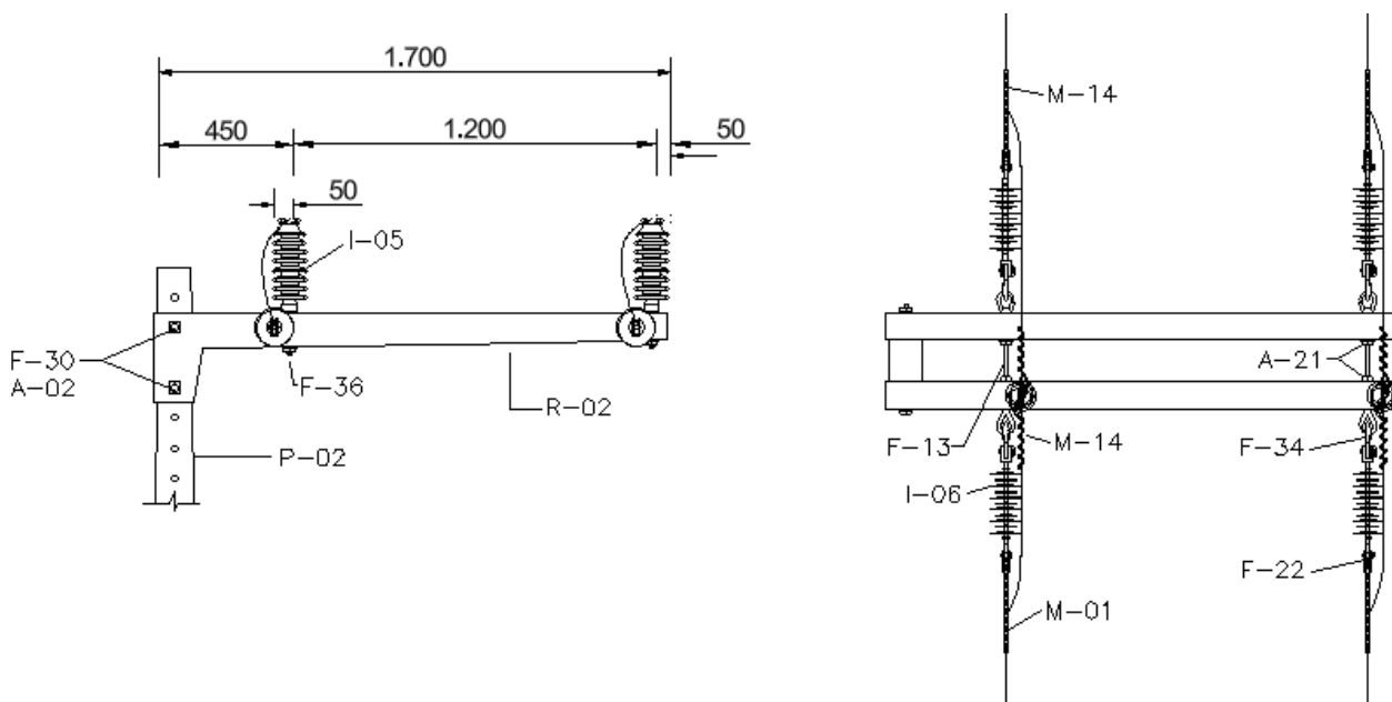
Desenho 65- Rede de Média Tensão Bifásica – Estrutura Beco Bifásica – B4B
