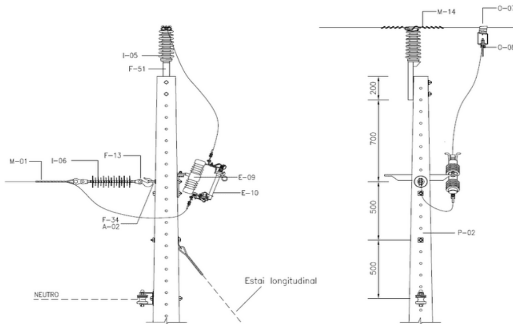
Quadro 123 - Lista de Materiais referente ao Desenho 109 – Chave Fusível Derivação Monofásica U1-U3
