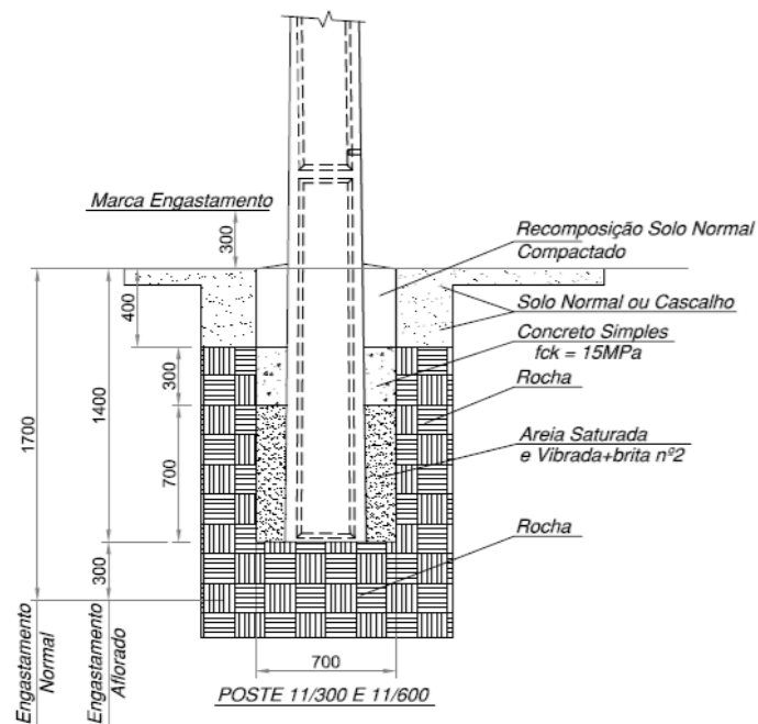
Desenho 23 - Detalhe Engastamento em Rocha com Concreto de 1 Camada – Tipo 2
