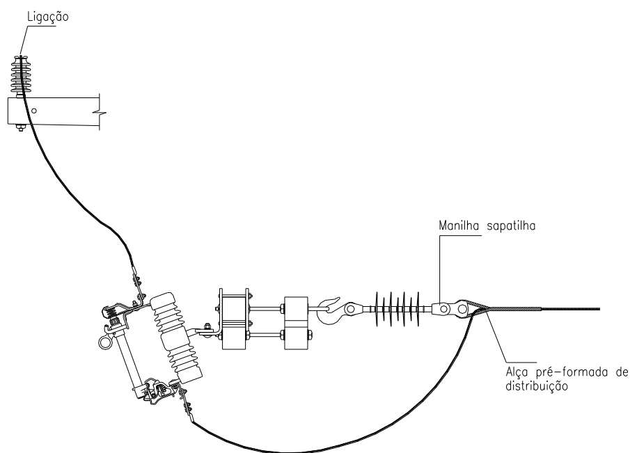
Desenho 142 - Amarrações e ligações – Primário – Chave-fusível e chave faca em derivação
