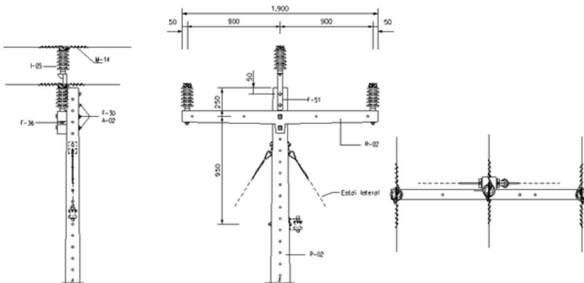
Quadro 79 - Lista de Materiais referente ao Desenho 83 – Estrutura T1
