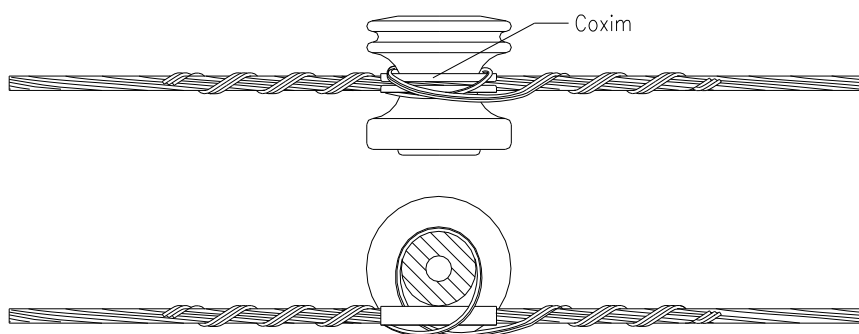
Desenho 149 - Amarrações e ligações – Secundário – ligação de baixa tensão do transformador
