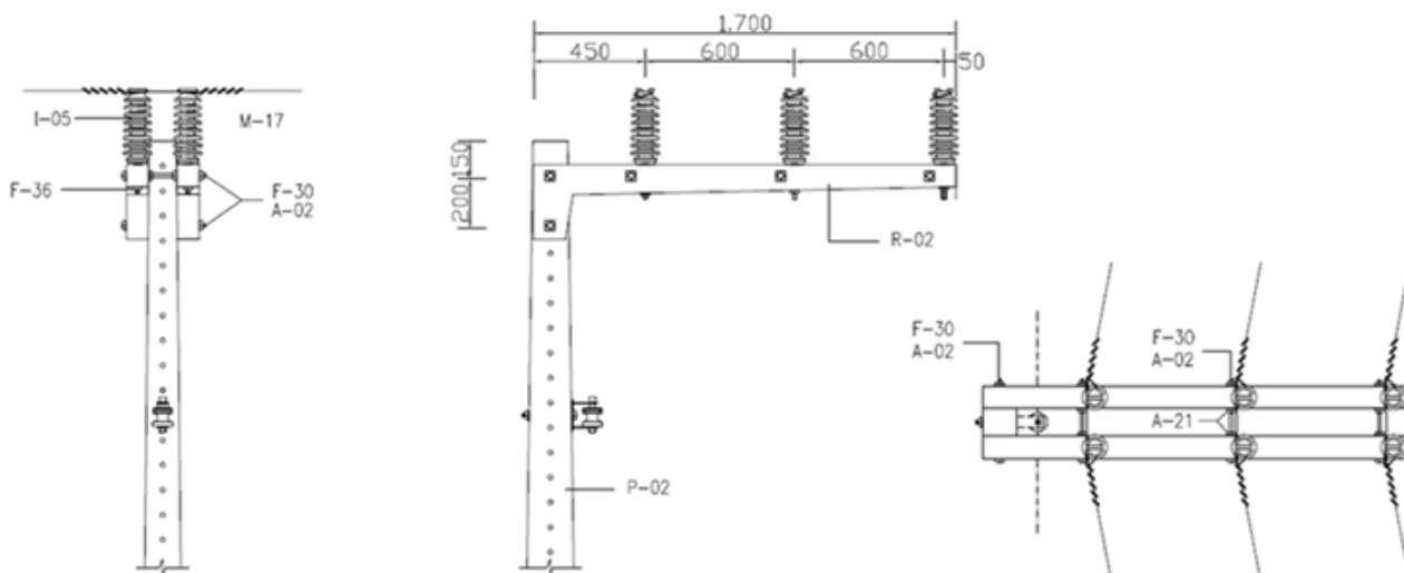
Quadro 62 - Lista de Materiais referente ao Desenho 73 – Estrutura B2
