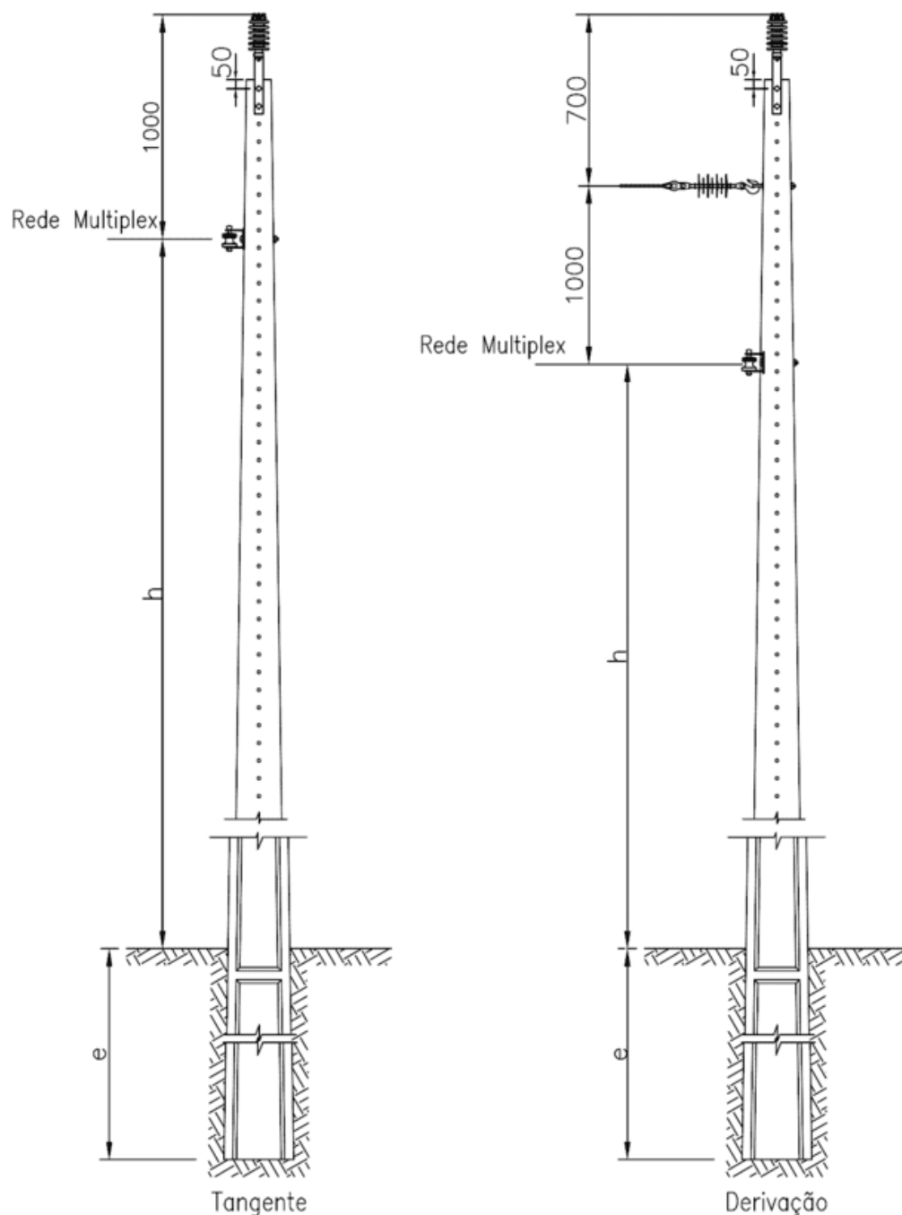
Desenho 15 - Afastamentos mínimos – Estrutura monofásica tangente e derivação
