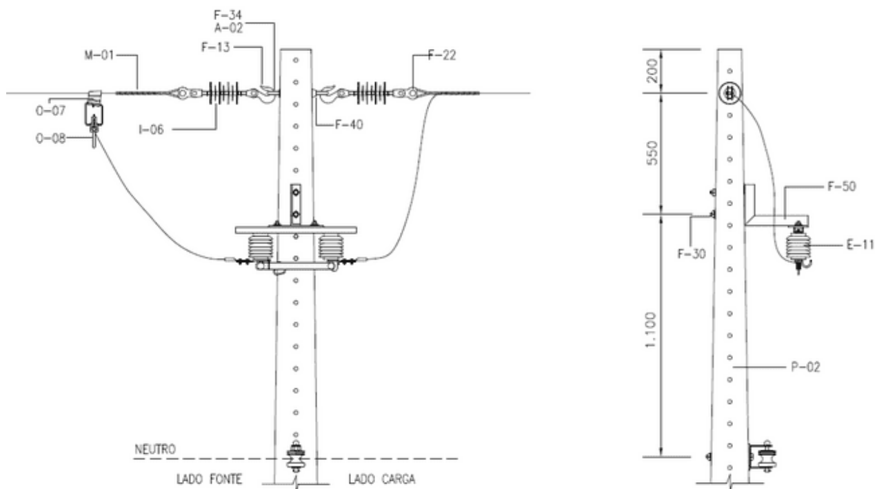
Quadro 121 - Lista de Materiais referente ao Desenho 107 – Chave Faca Unipolar Monofásica
