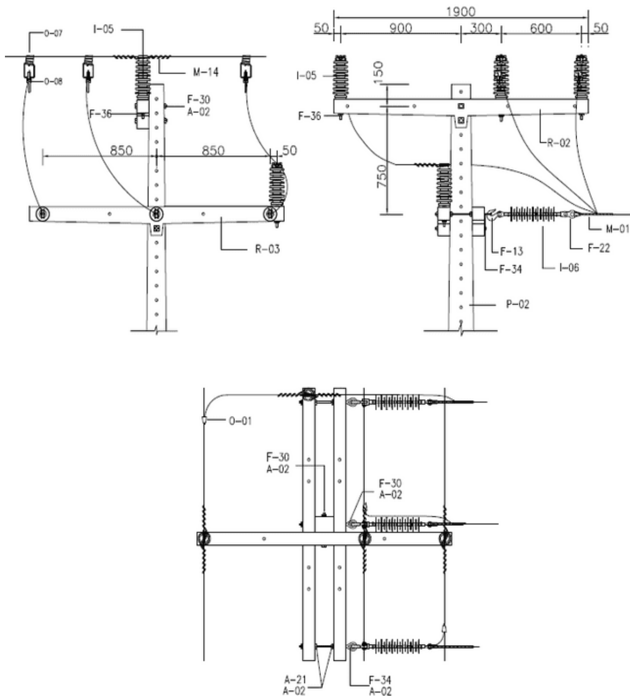
Desenho 78- Rede de Média Tensão Trifásica – Estrutura N1-DN3
