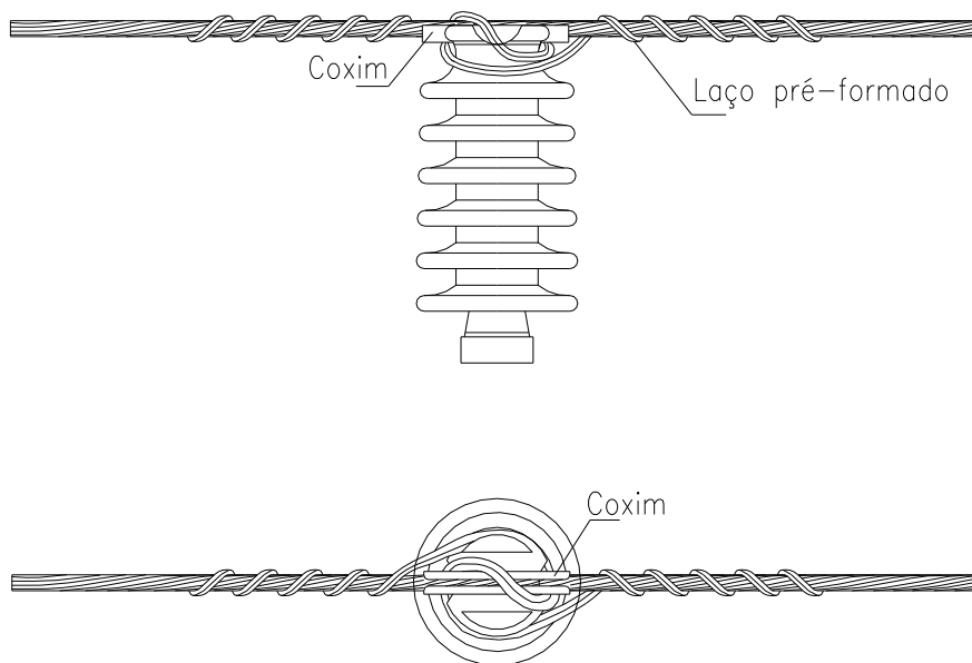
Desenho 136 - Amarrações e ligações – Primário – Amarração simples de topo
