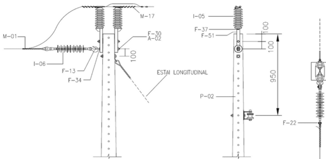
Quadro 18 - Lista de Materiais referente ao Desenho 47 – Estrutura U3.2
