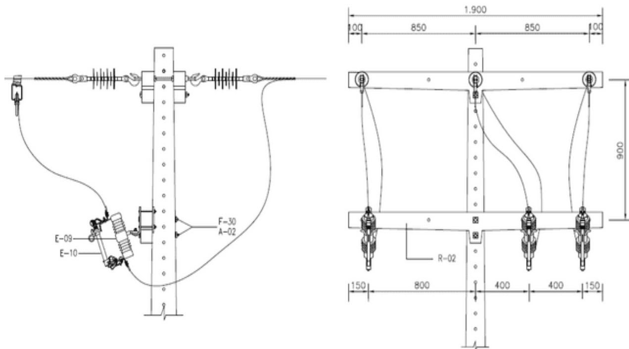
Quadro 125 - Lista de Materiais referente ao Desenho 111 – Chave Fusível em alinhamento N4
