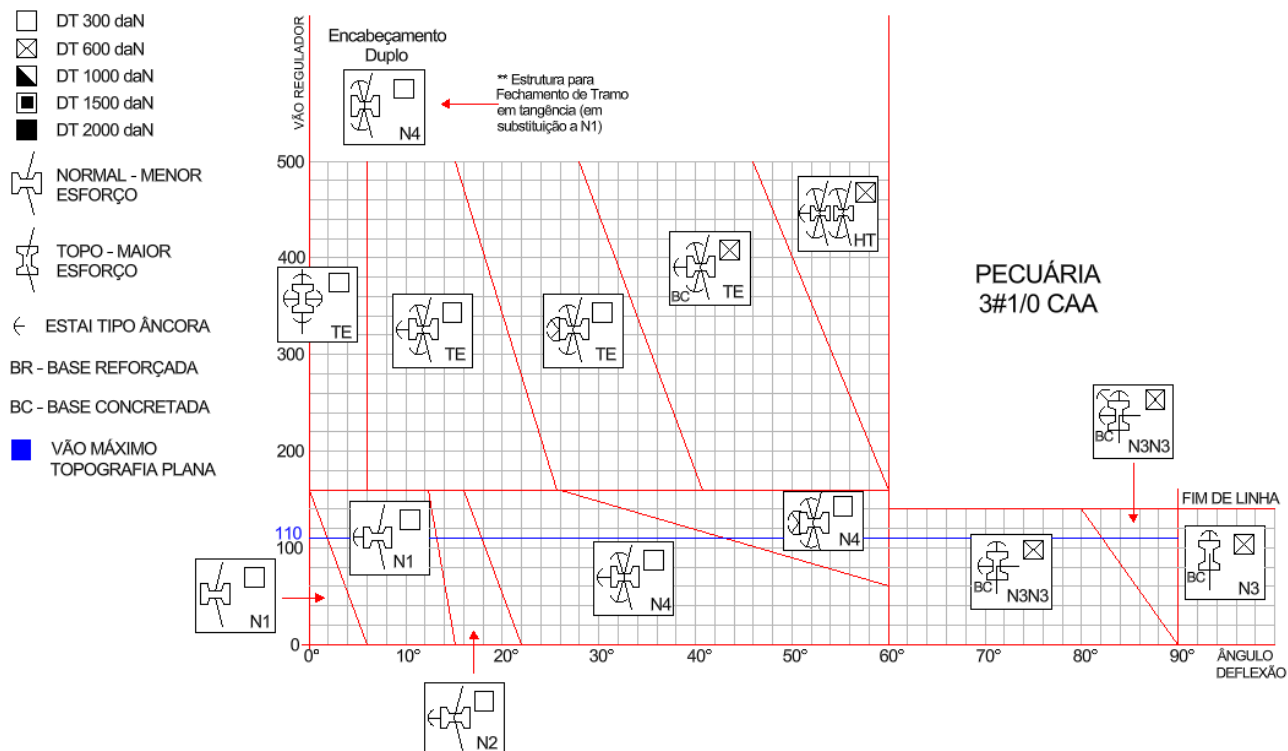
Desenho 166 - Ábaco para estruturas trifásicas tipo Normal cabo 1/0 CAA em áreas de Pecuária
