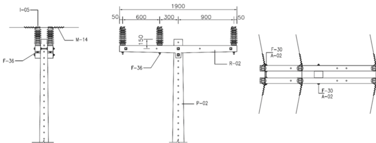
Quadro 54 - Lista de Materiais referente ao Desenho 69 – Estrutura N2
