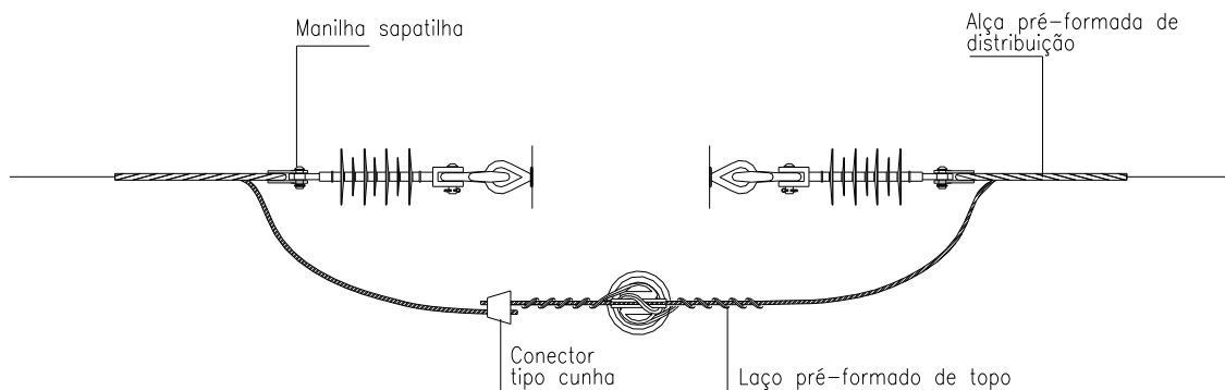
Desenho 139 - Amarrações e ligações – Primário – Ancoragem dupla
