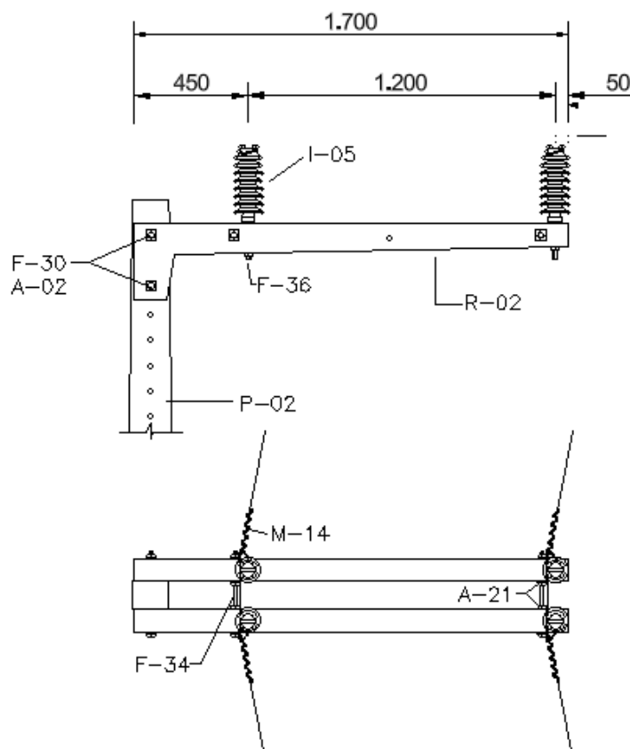
Quadro 47 - Lista de Materiais referente ao Desenho 63 – Estrutura B2B
