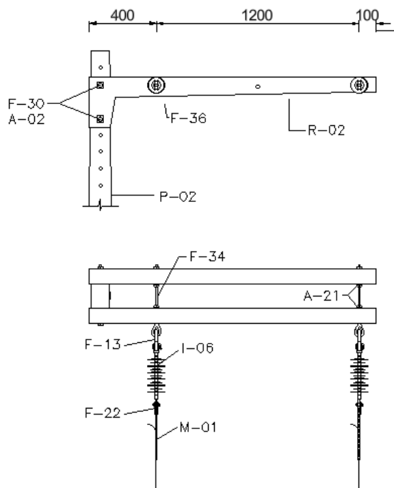
Quadro 48 - Lista de Materiais referente ao Desenho 64 – Estrutura B3B
