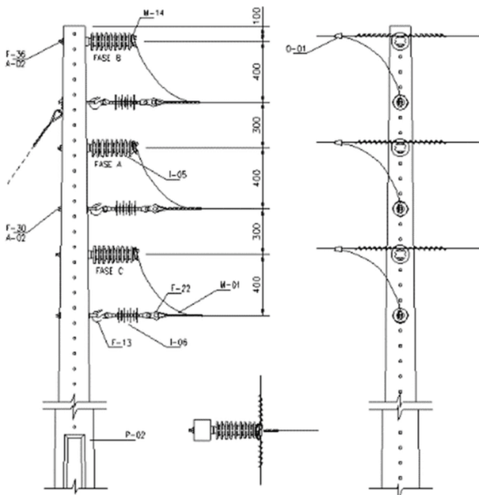
Desenho 97 - Rede de Média Tensão Trifásica – Estrutura P1.P3
