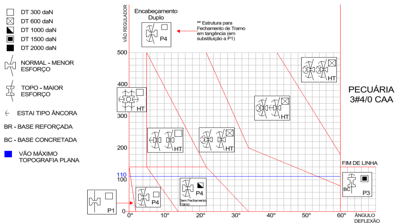
Desenho 173 - Ábaco para aplicação de estruturas trifásicas tipo Pilar no Poste (P) cabo 4/0 CAA em áreas de Pecuária
