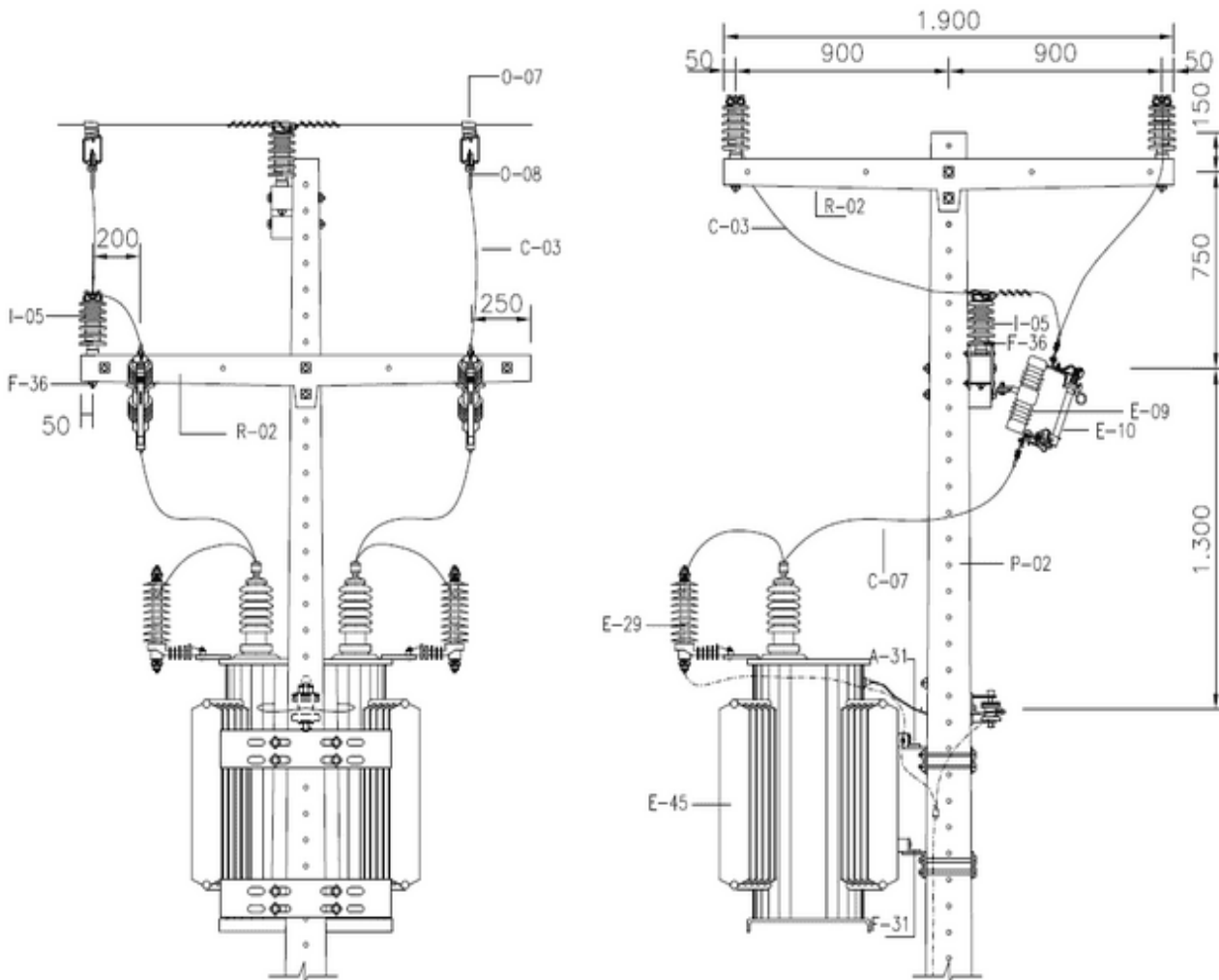
Desenho 128 - Chaves e equipamentos – Estrutura com transformador FF - N1B- NSCF-TM
