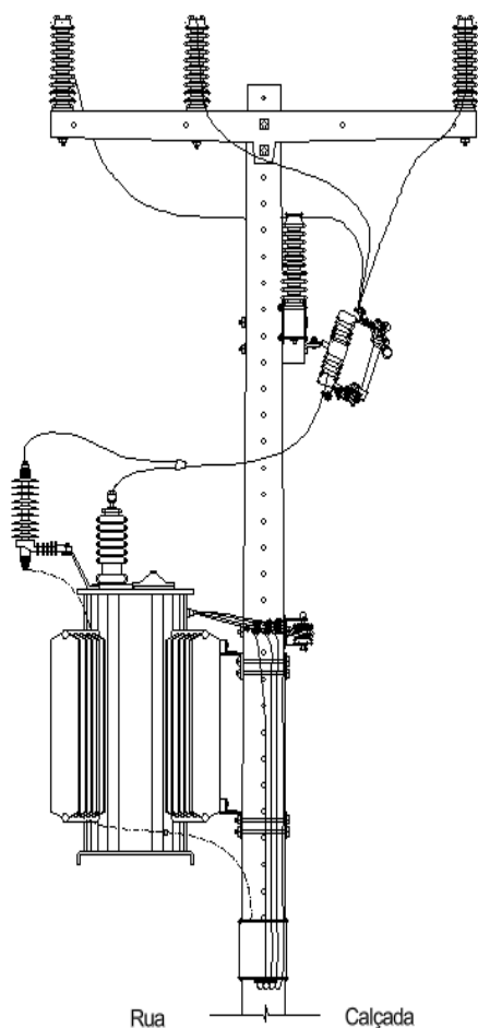
Desenho 120 - Chaves e equipamentos – Detalhe instalação Medição Totalizadora
