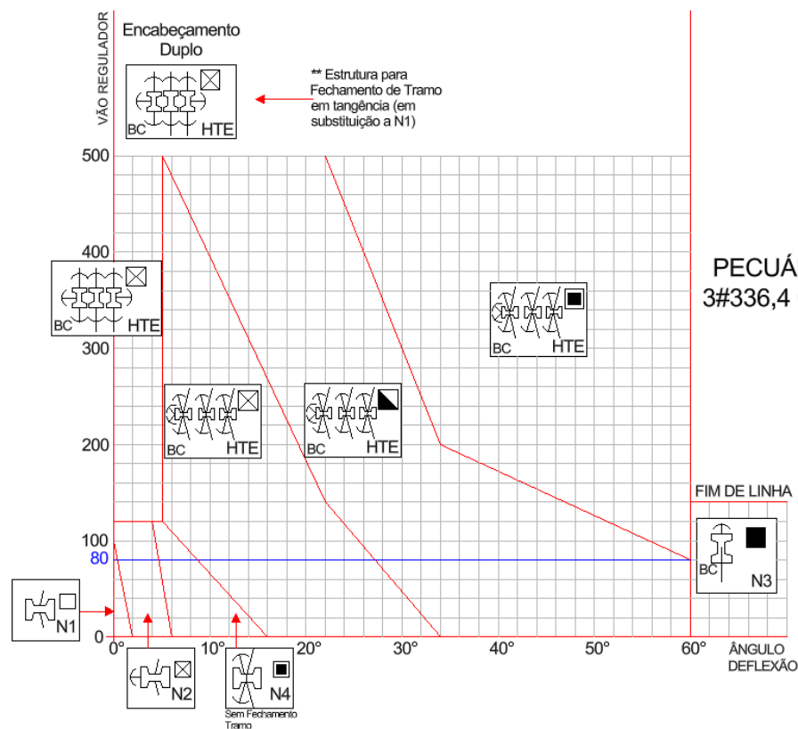
Desenho 170 - Ábaco para estruturas trifásicas tipo Normal cabo 336,4 MCM CAA em áreas de Pecuária
