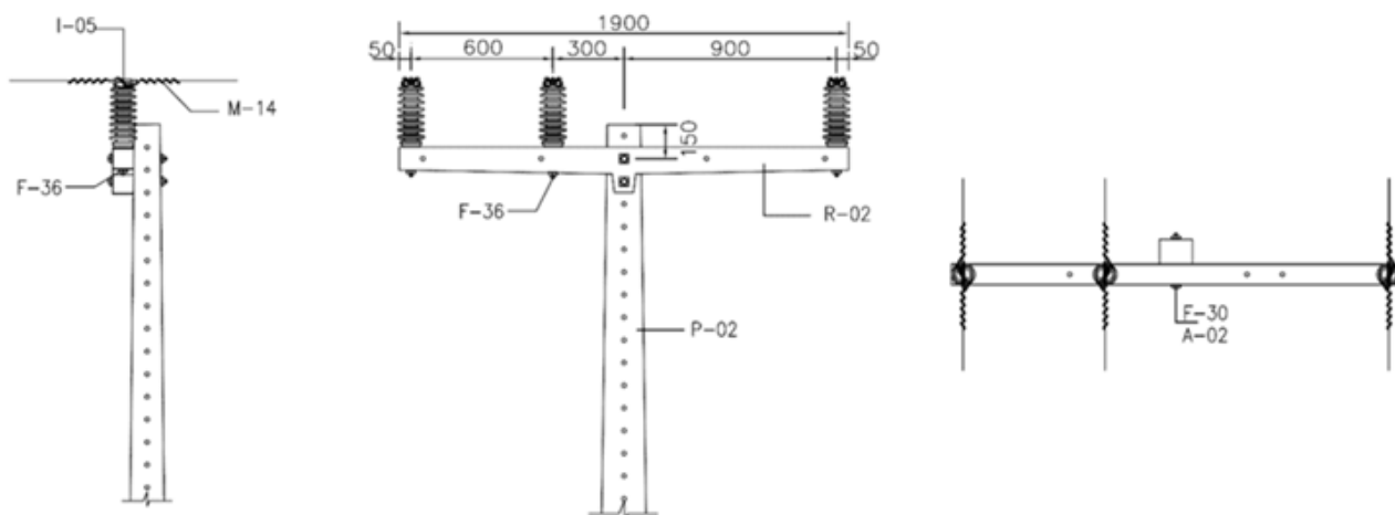
Desenho 68 - Rede de Média Tensão Trifásica – Estrutura N1
