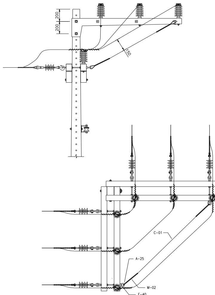
Quadro 120 - Lista de Materiais referente ao Desenho 105 – Detalhe Estai de cruzeta a cruzeta
