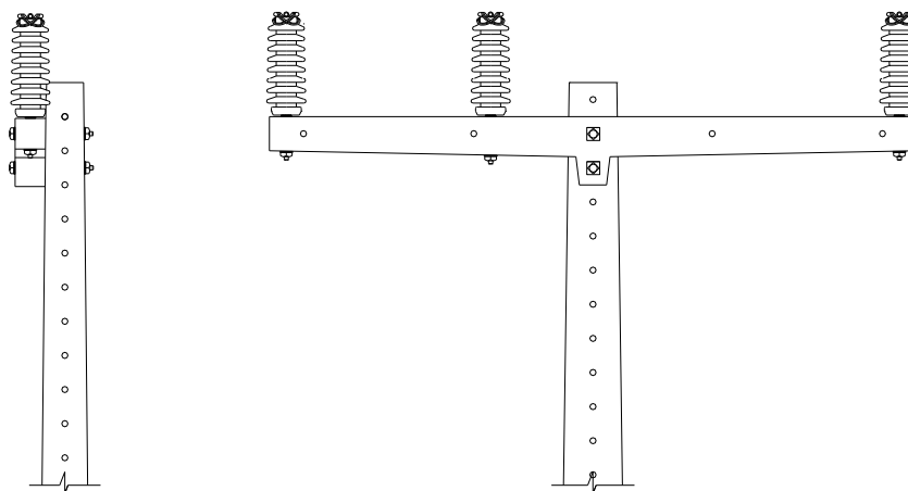
Desenho 3 - Estrutura de alinhamento com cruzeta tipo T 1.900mm
