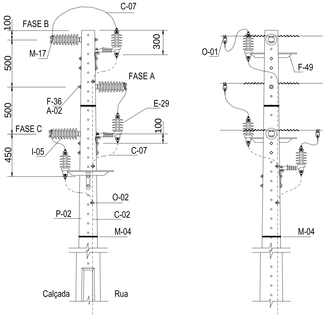
Desenho 100 - Rede de Média Tensão Trifásica – Estrutura P1A-PR
