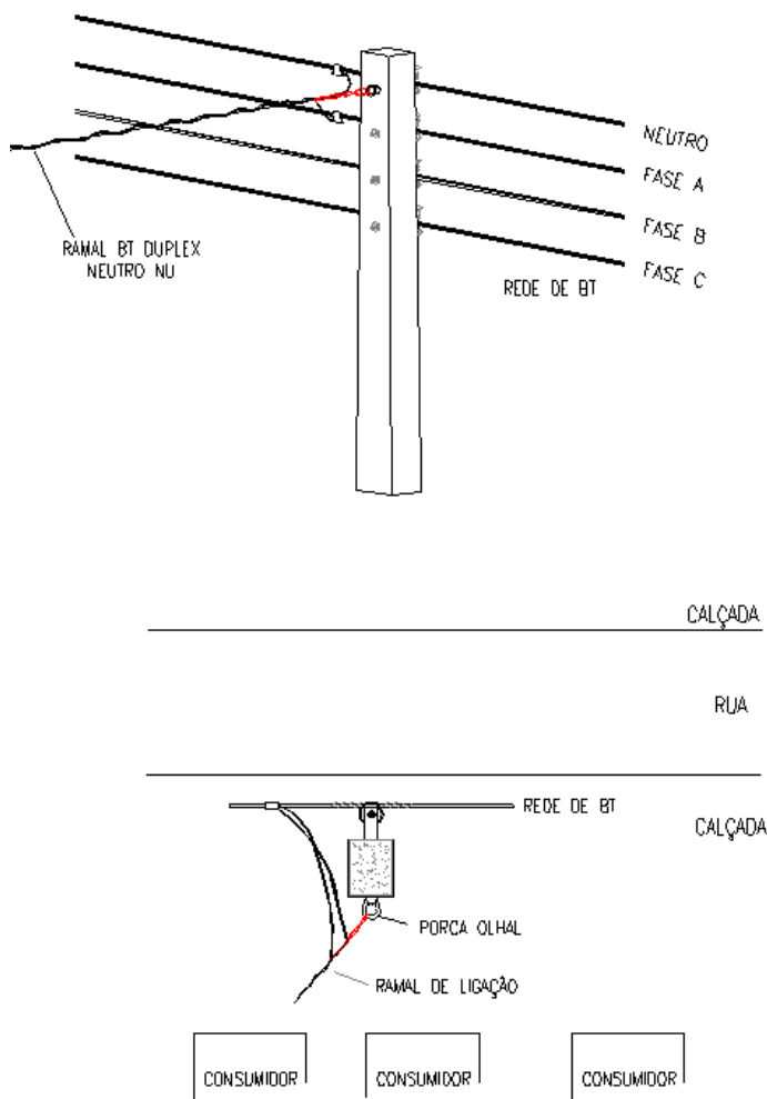
Desenho 151 - Amarrações – Ramal de ligação com o consumidor no mesmo lado da rede de BT.
