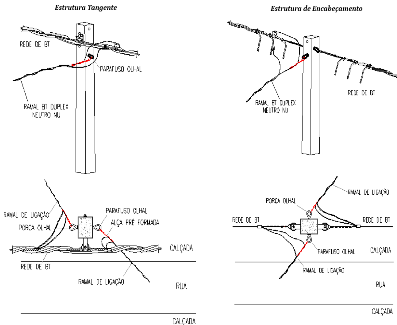
Desenho 153 - Amarrações – Ramal de ligação em rede de BT multiplexada.
