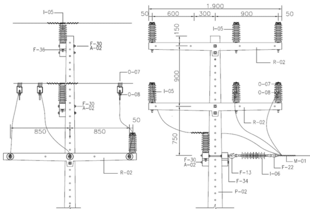
Quadro 77 - Lista de Materiais referente ao Desenho 81 – Estrutura N1-N1-DN3
