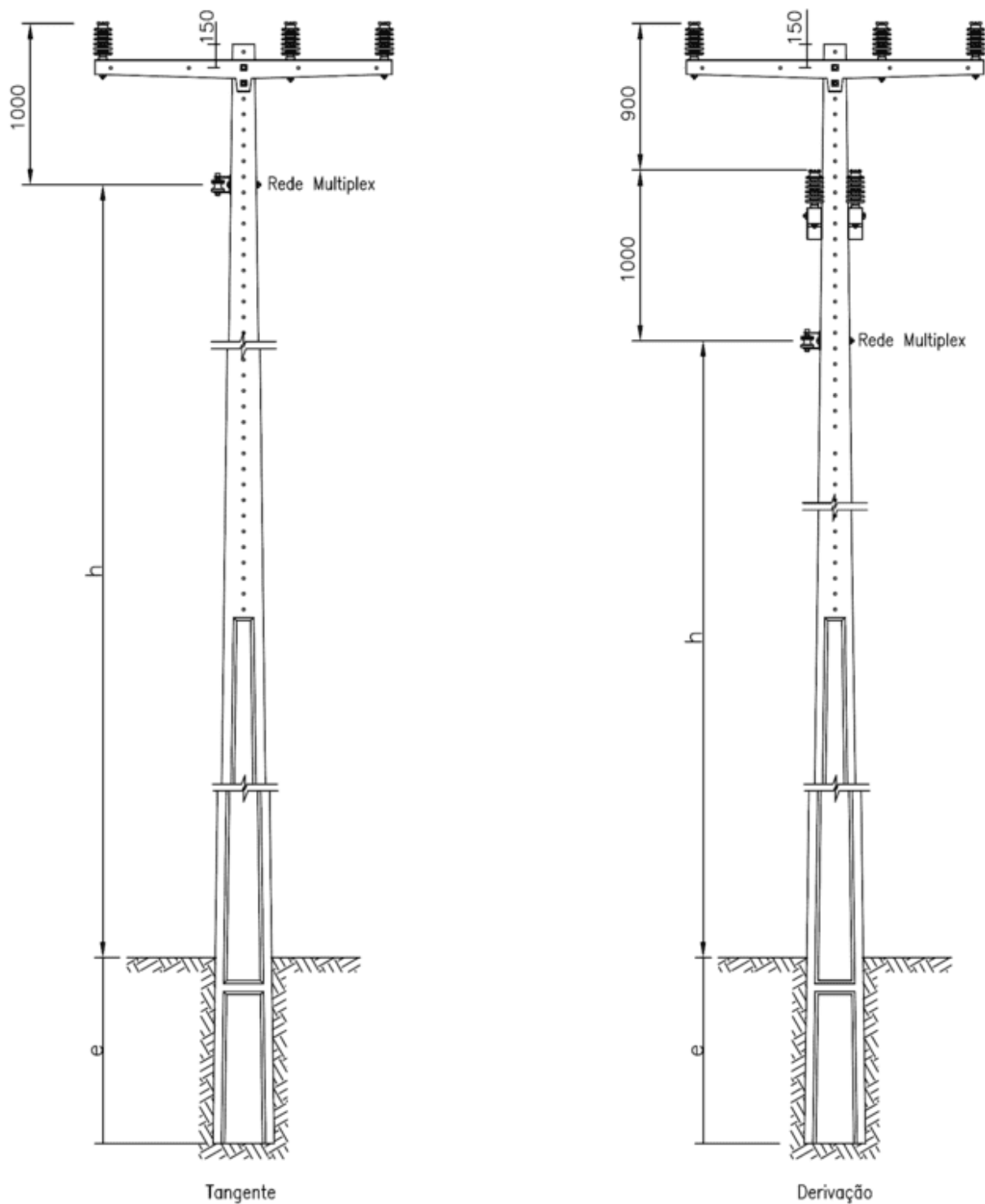
Desenho 16 - Afastamentos mínimos – Estrutura trifásica tangente e derivação
