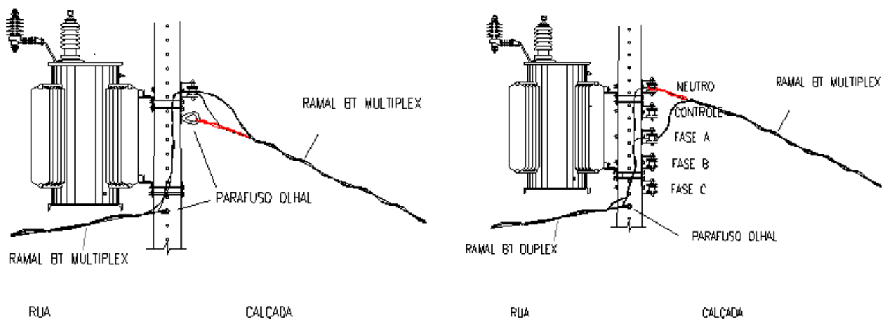
Desenho 155 - Amarrações e ligações – Secundário – Seccionamento aéreo
