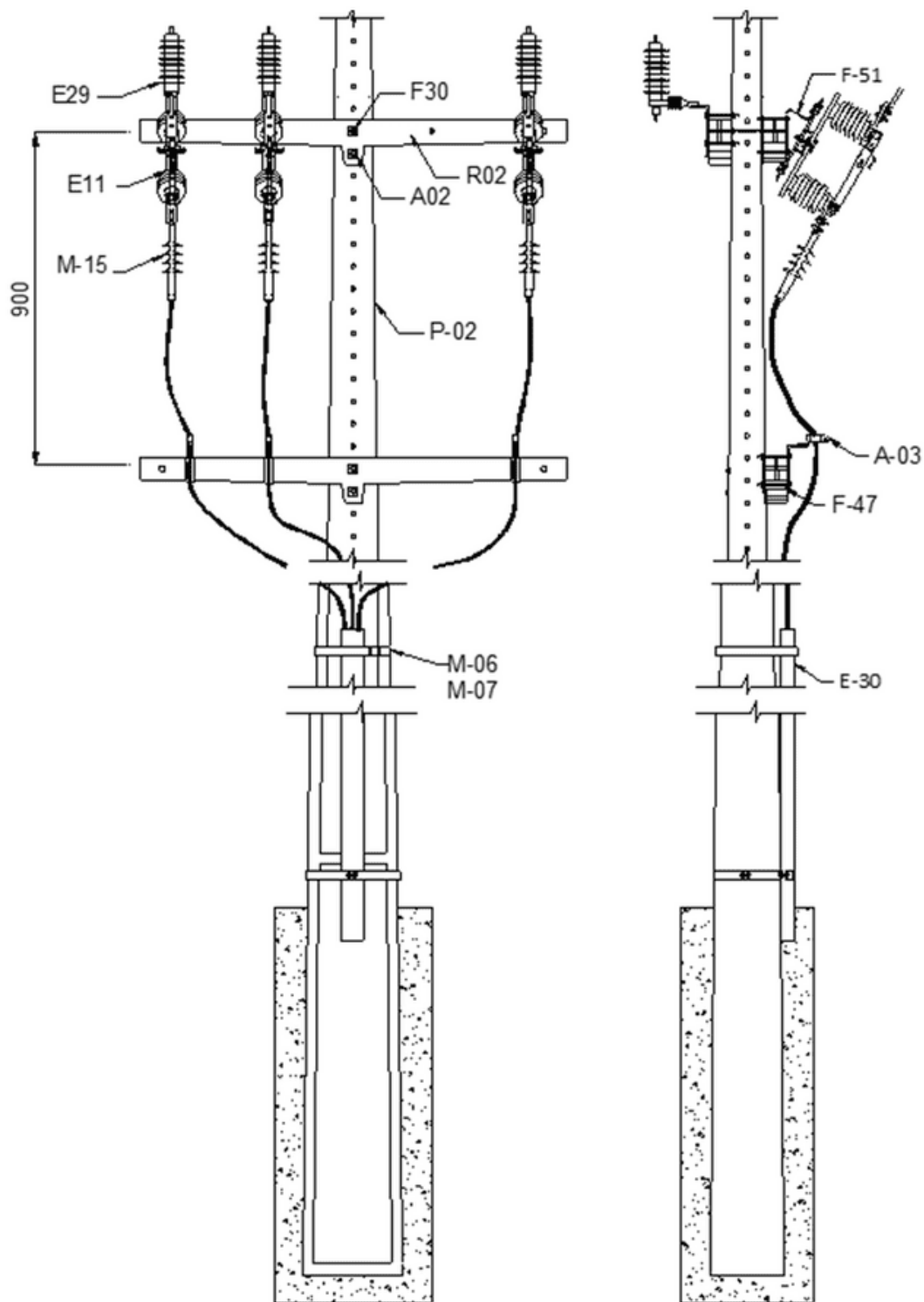
Desenho 132 - Chaves e equipamentos - Estrutura para mufla com chave faca - Padrão existente (manutenção)
