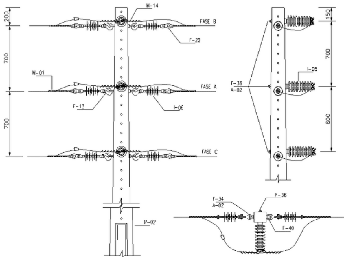
Quadro 104 - Lista de Materiais referente ao Desenho 96 – Estrutura P4
