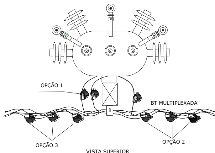
Desenho 133 - Chaves e equipamentos - Para-raios de Baixa Tensão - Opções de Instalação
