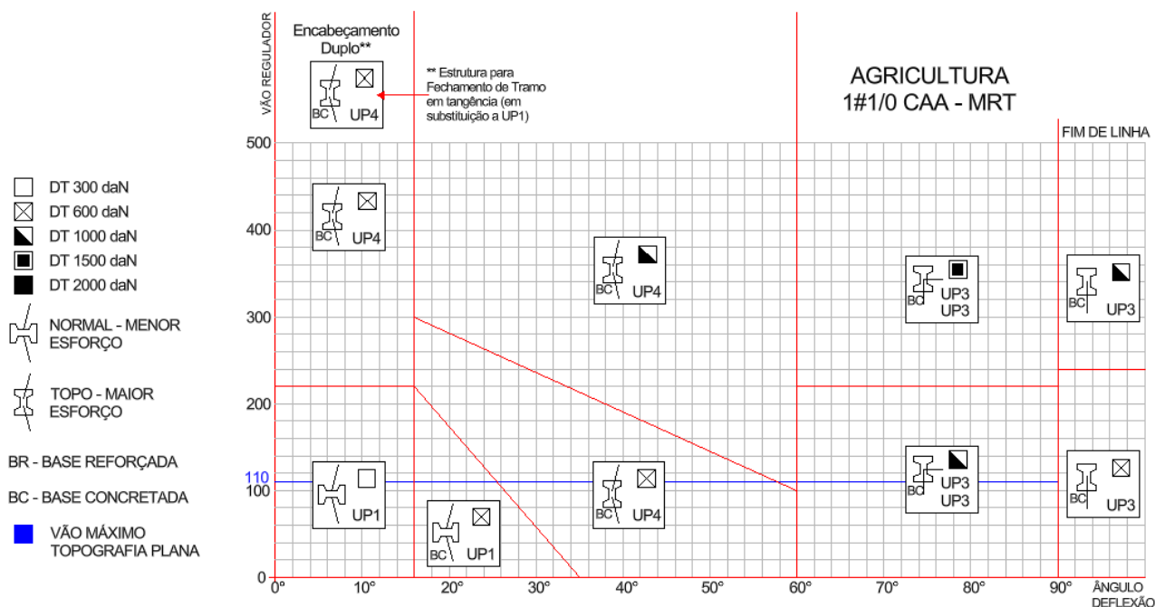
Desenho 163 - Ábaco para aplicação de estruturas monofásicas MRT cabo 1/0 CAA em áreas de Agricultura
