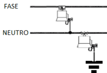
Desenho 135 Chaves e equipamentos - Baixa Tensão - PRBT - Detalhes da Ligações - MRT
