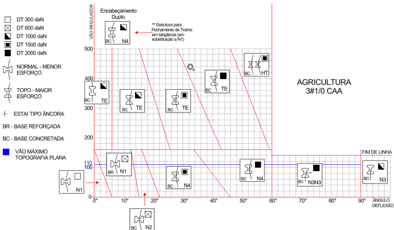
Desenho 165 - Ábaco para estruturas trifásicas tipo Normal cabo 1/0 CAA em áreas de Agricultura
