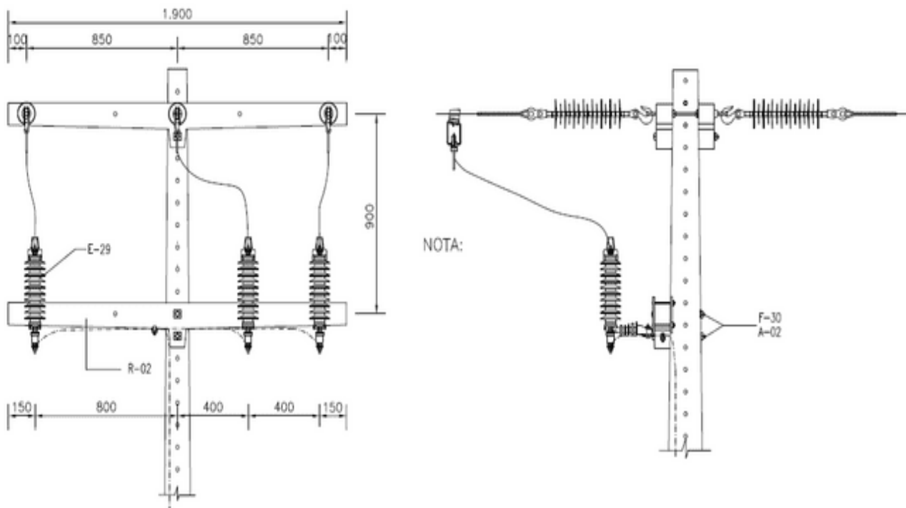
Quadro 126 - Lista de Materiais referente ao Desenho 113 – Para-raios em alinhamento N4
