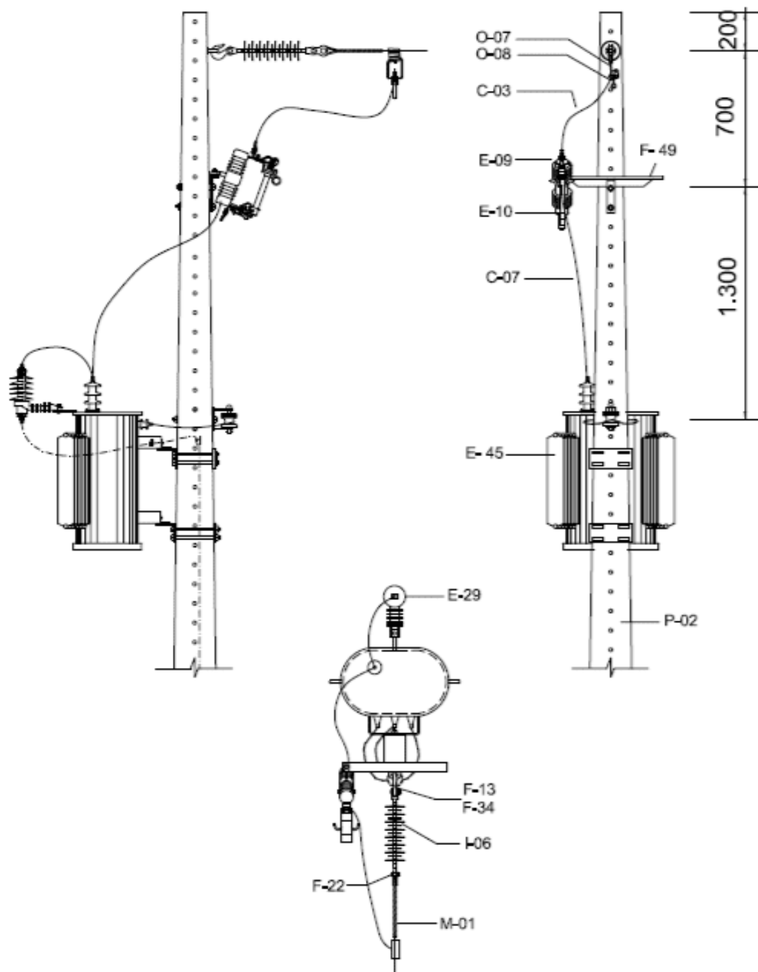
Desenho 116 - Chaves e equipamentos – Transformador Monofásico Fim de Rede
