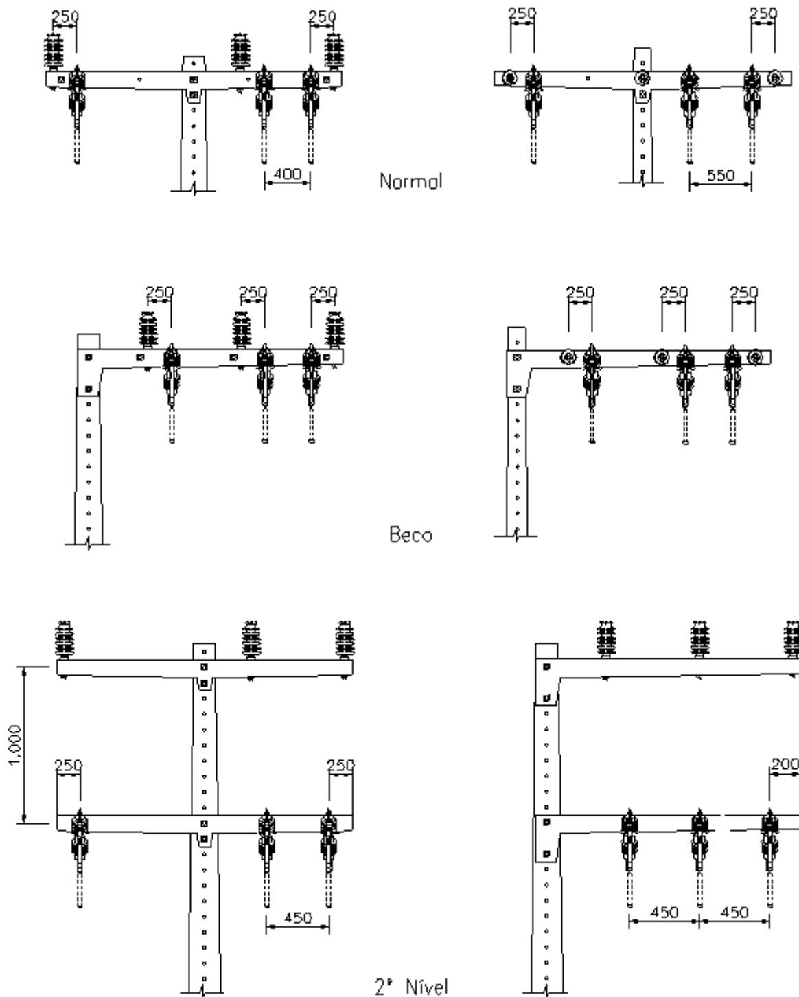
Desenho 42 - Rede de Média Tensão – Afastamentos de chaves e para-raios
