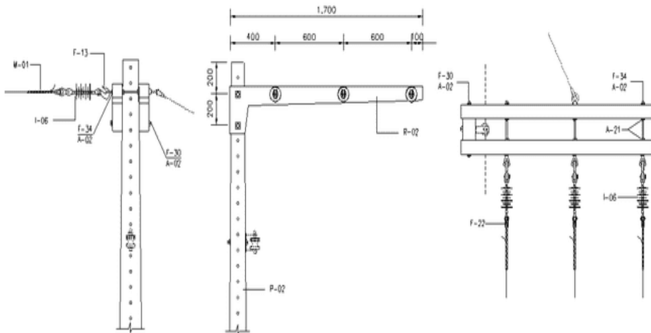
Quadro 64 - Lista de Materiais referente ao Desenho 74 – Estrutura B3
