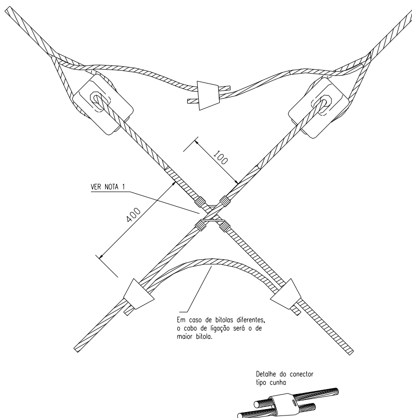
Desenho 155 - Amarrações e ligações – Secundário – Seccionamento aéreo
