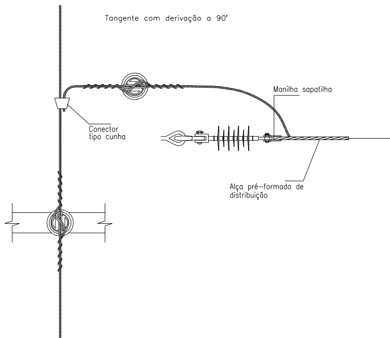
Desenho 141 - Amarrações e ligações – Primário – Ancoragem e derivação
