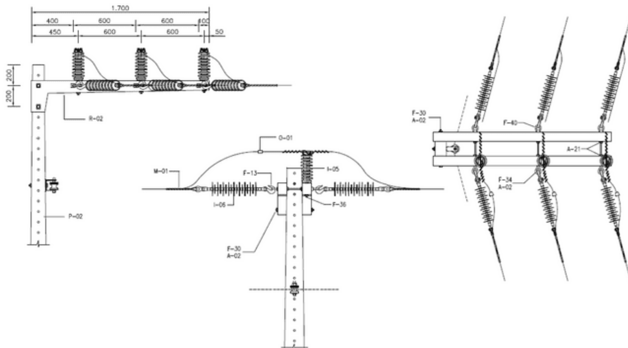
Quadro 68 - Lista de Materiais referente ao Desenho 76 – Estrutura B4
