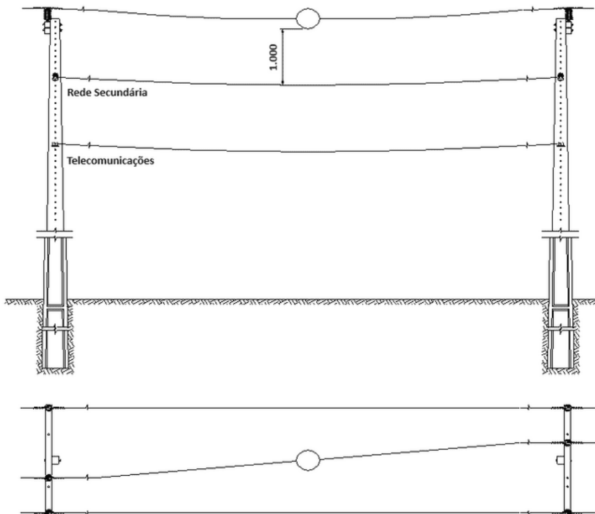
Desenho 7 - Montagem de esferas de sinalização diurna em redes aéreas com condutores nus.
