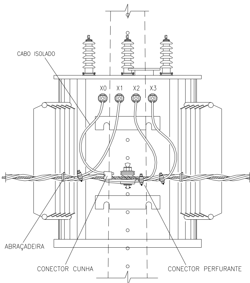
Desenho 149 - Amarrações e ligações – Secundário – ligação de baixa tensão do transformador
