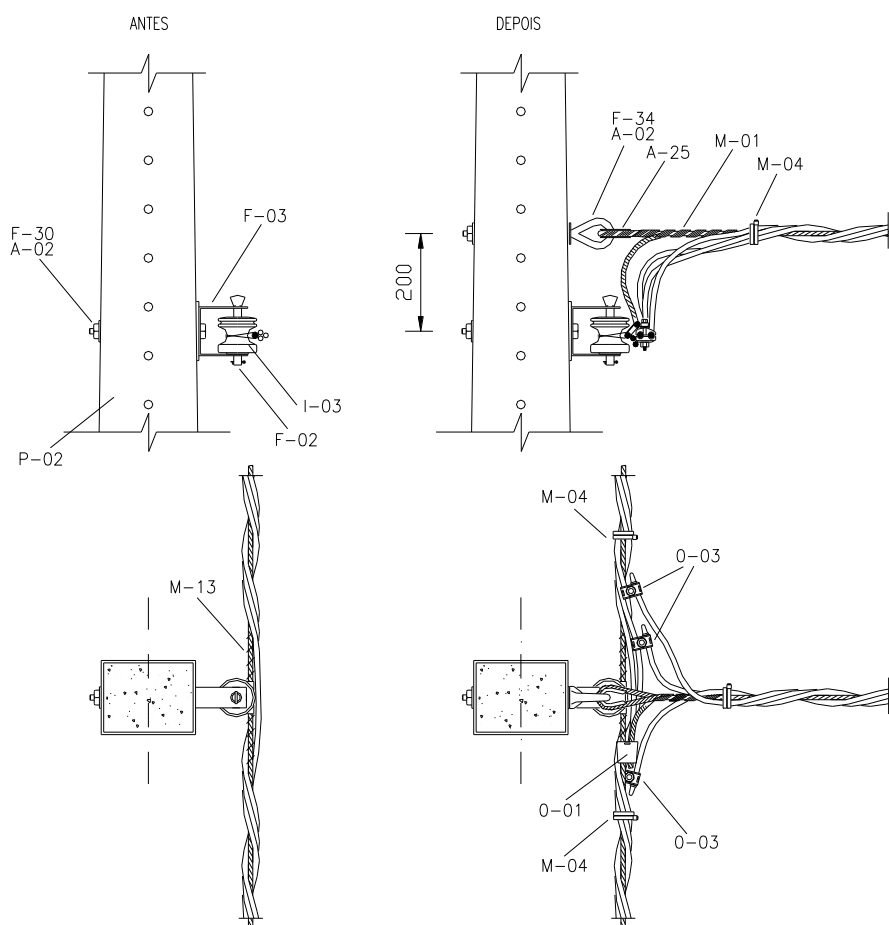
Desenho 32 - Rede de Baixa Tensão (Secundária Multiplexada) – Estrutura de derivação de rede tangente (S1I-S3I TAN)
