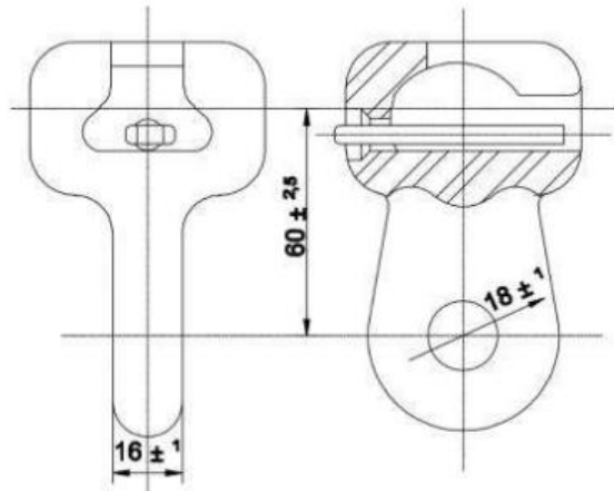
Desenho 1 – Engate Concha Olhal – Detalhes Construtivos
