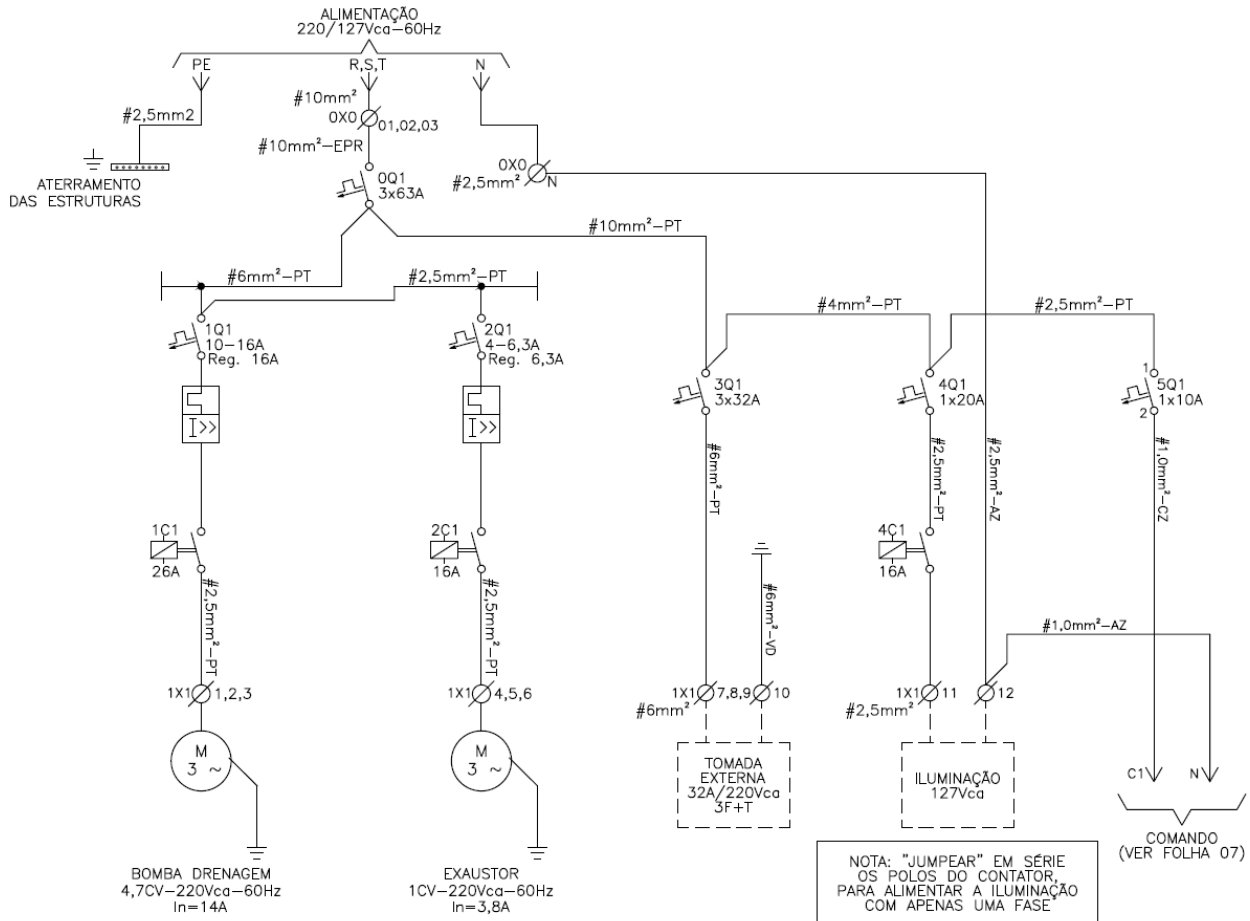
Desenho 3 – Diagrama Unifilar do Circuito de Comando
