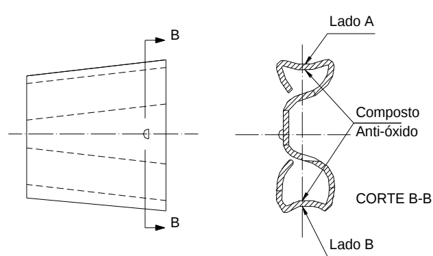
FIGURA 2 - COMPONENTE "CUNHA"
