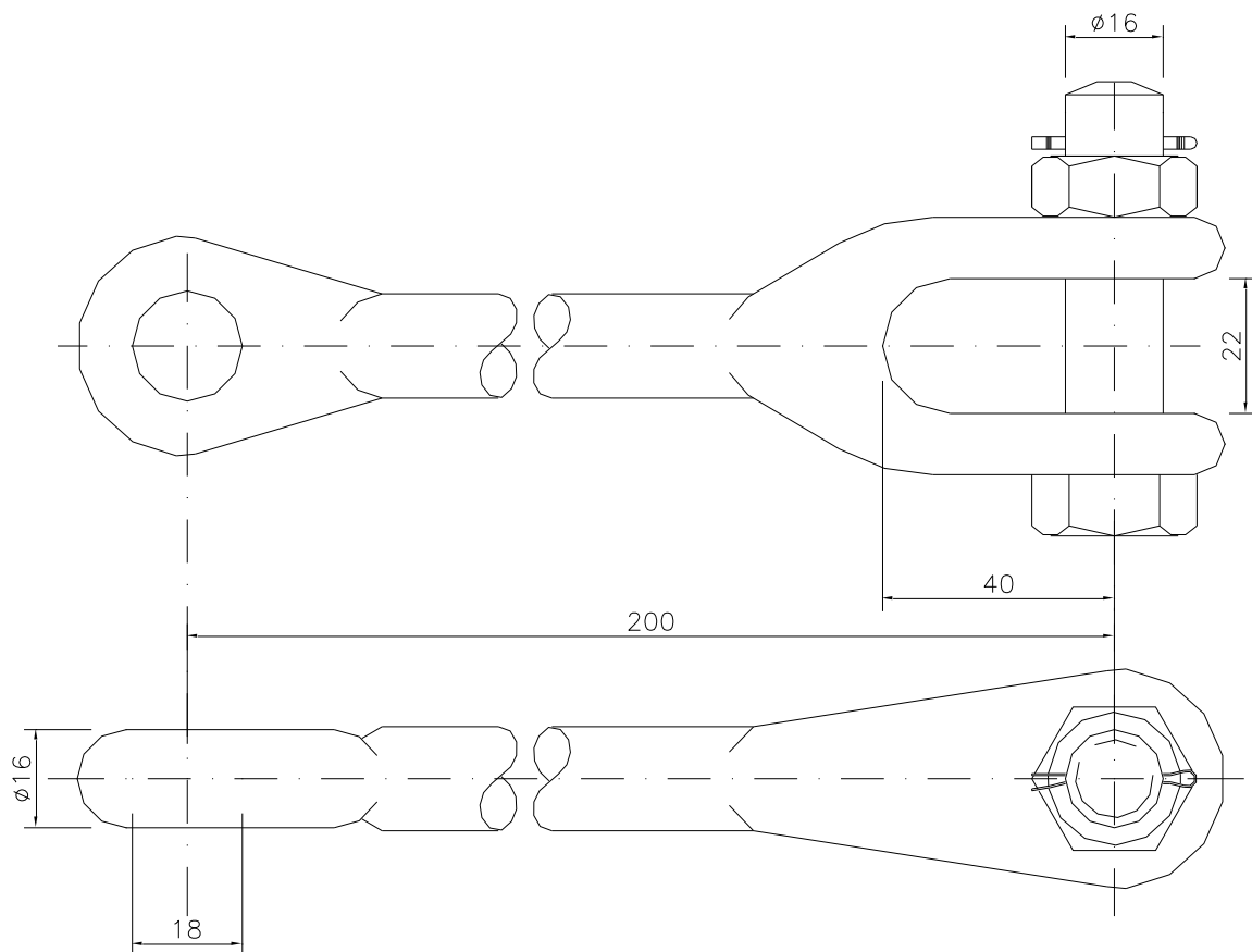
Desenho 1 – Prolongador Garfo Olhal 90° - Detalhes Construtivos.
