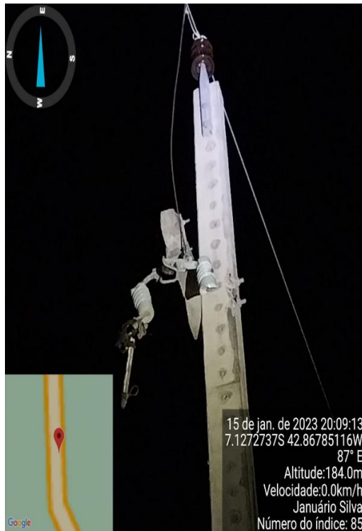
oto – Cruzeta e Isolador quebrado
