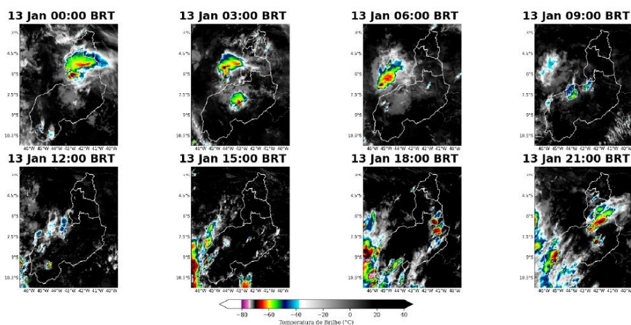
Figura 2: Imagens realizadas do satélite GOES-16 das 00 BRT até 21 BRT (a cada 3 horas) para o dia 13 de janeiro.
