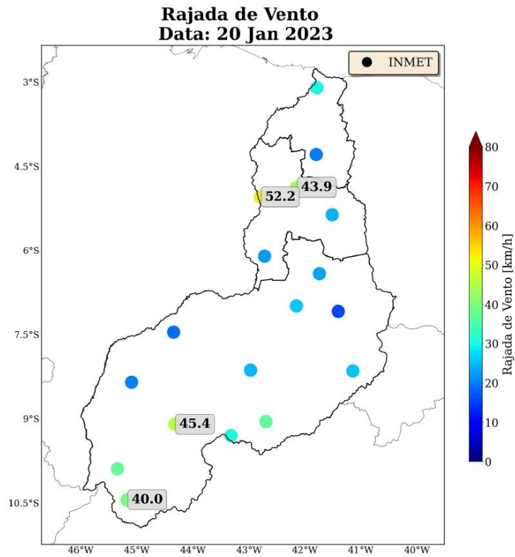
Figura 35: Máxima rajada de vento diária sobre a área de concessão da Equatorial-PI para o dia 20 de janeiro, baseado nas estações meteorológicas do INMET.
