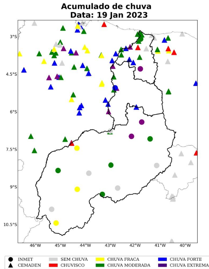
Figura 25: Acumulado diário de precipitação sobre a área de concessão da Equatorial-PI para o dia 19 de janeiro, baseado nas estações meteorológicas do INMET e CEMADEN.
