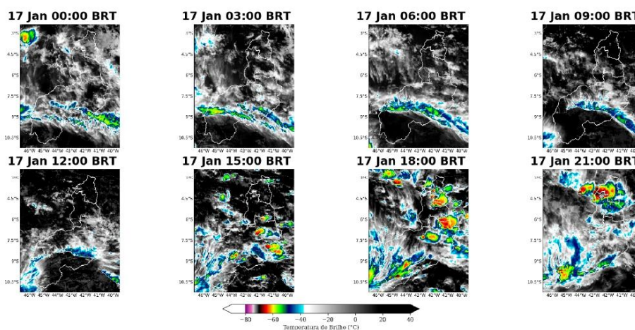
Figura 6: Imagens realizadas do satélite GOES-16 das 00 BRT até 21 BRT (a cada 3 horas) para o dia 17 de janeiro.
