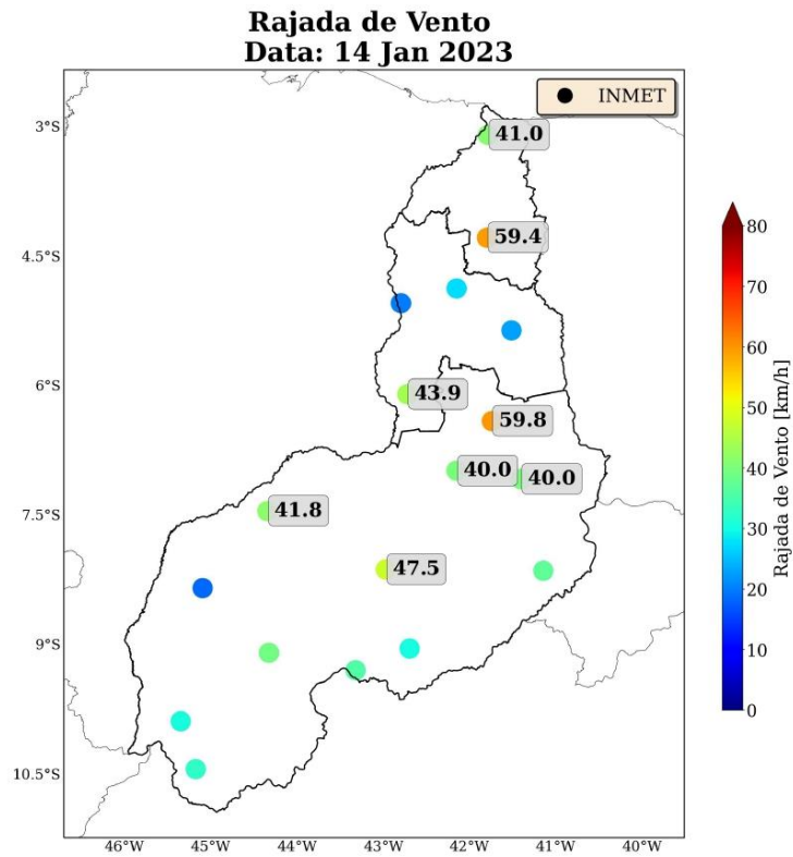
Figura 29: Máxima rajada de vento diária sobre a área de concessão da Equatorial-PI para o dia 14 de janeiro, baseado nas estações meteorológicas do INMET.
