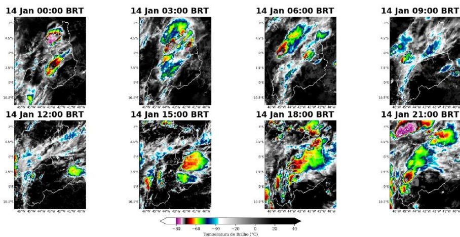
Figura 3: Imagens realizadas do satélite GOES-16 das 00 BRT até 21 BRT (a cada 3 horas) para o dia 14 de janeiro.
