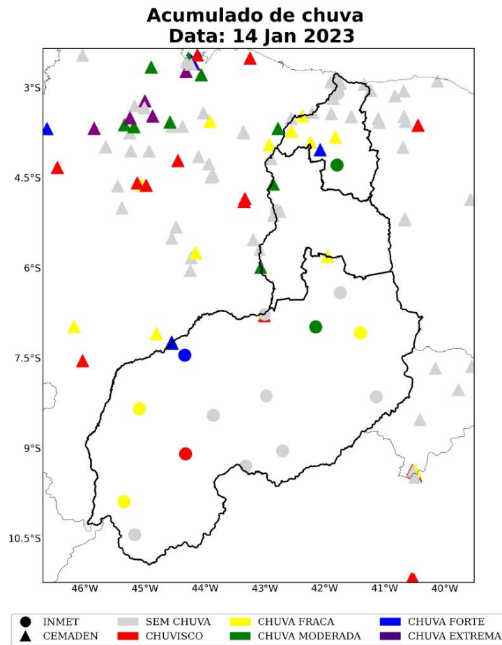
Figura 20: Acumulado diário de precipitação sobre a área de concessão da Equatorial-PI para o dia 14 de janeiro, baseado nas estações meteorológicas do INMET e CEMADEN.
