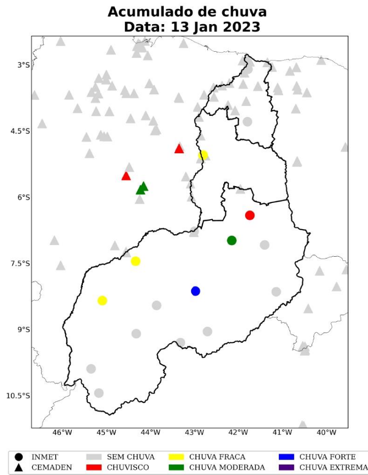
Figura 19: Acumulado diário de precipitação sobre a área de concessão da Equatorial-PI para o dia 13 de janeiro, baseado nas estações meteorológicas do INMET e CEMADEN.
