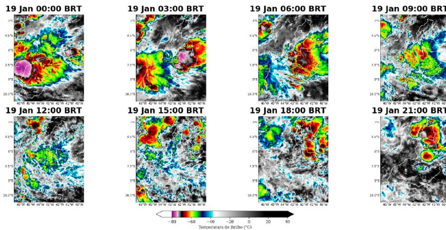
Figura 8: Imagens realizadas do satélite GOES-16 das 00 BRT até 21 BRT (a cada 3 horas) para o dia 19 de janeiro.
