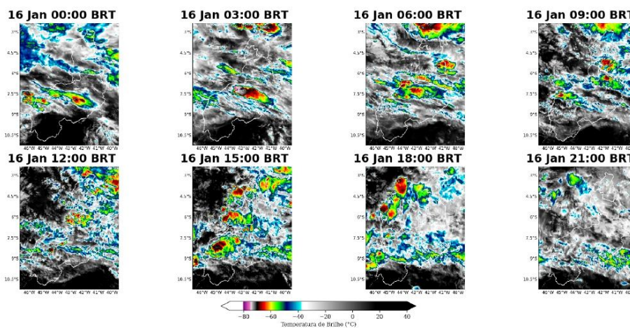
Figura 5: Imagens realizadas do satélite GOES-16 das 00 BRT até 21 BRT (a cada 3 horas) para o dia 16 de janeiro.
