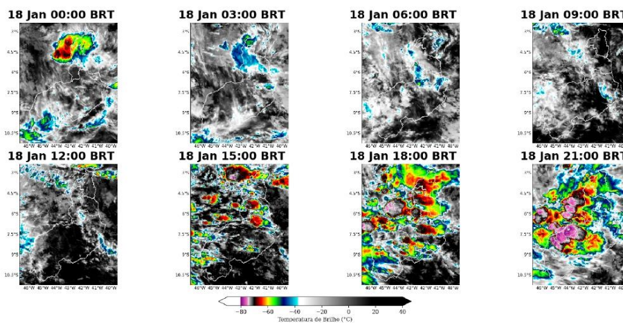
Figura 7: Imagens realizadas do satélite GOES-16 das 00 BRT até 21 BRT (a cada 3 horas) para o dia 18 de janeiro.
