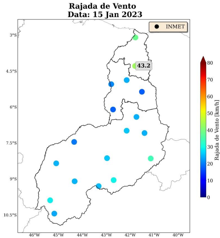
Figura 30: Máxima rajada de vento diária sobre a área de concessão da Equatorial-PI para o dia 15 de janeiro, baseado nas estações meteorológicas do INMET.
