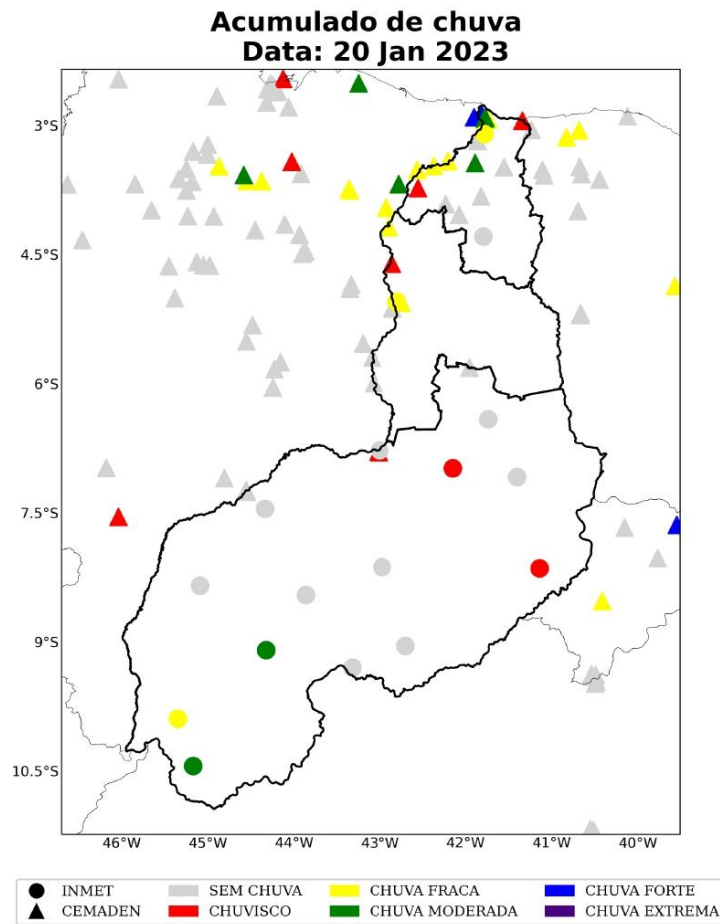
Figura 26: Acumulado diário de precipitação sobre a área de concessão da Equatorial-PI para o dia 20 de janeiro, baseado nas estações meteorológicas do INMET e CEMADEN.
