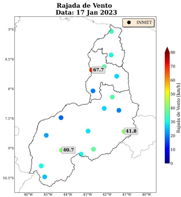
Figura 32: Máxima rajada de vento diária sobre a área de concessão da Equatorial-PI para o dia 17 de janeiro, baseado nas estações meteorológicas do INMET.
