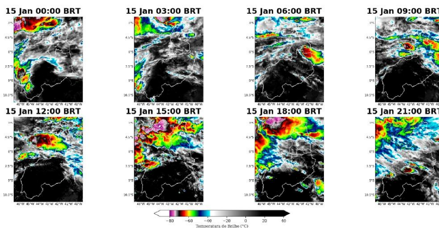
Figura 4: Imagens realizadas do satélite GOES-16 das 00 BRT até 21 BRT (a cada 3 horas) para o dia 15 de janeiro.
