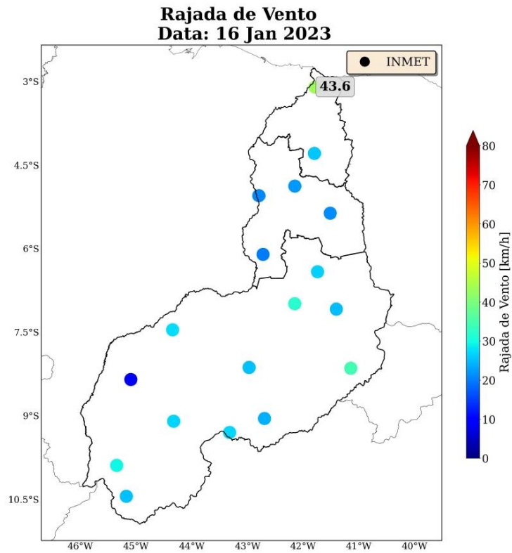
Figura 31: Máxima rajada de vento diária sobre a área de concessão da Equatorial-PI para o dia 16 de janeiro, baseado nas estações meteorológicas do INMET.
