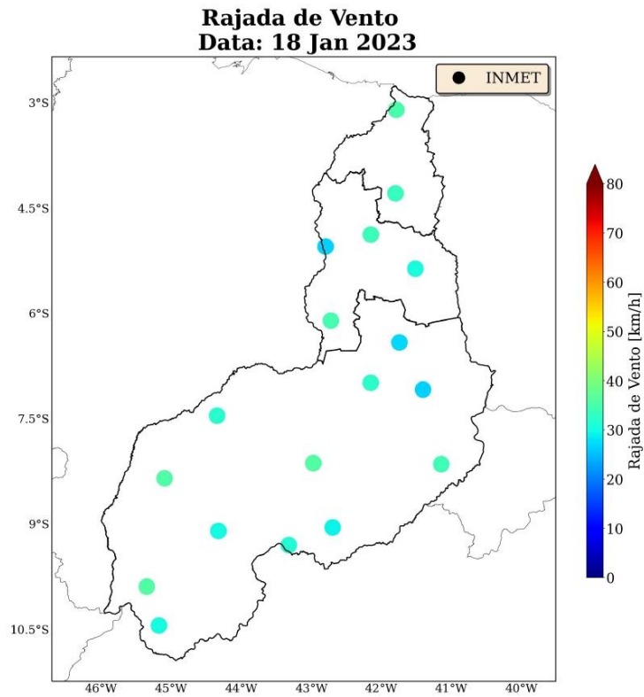
Figura 33: Máxima rajada de vento diária sobre a área de concessão da Equatorial-PI para o dia 18 de janeiro, baseado nas estações meteorológicas do INMET.
