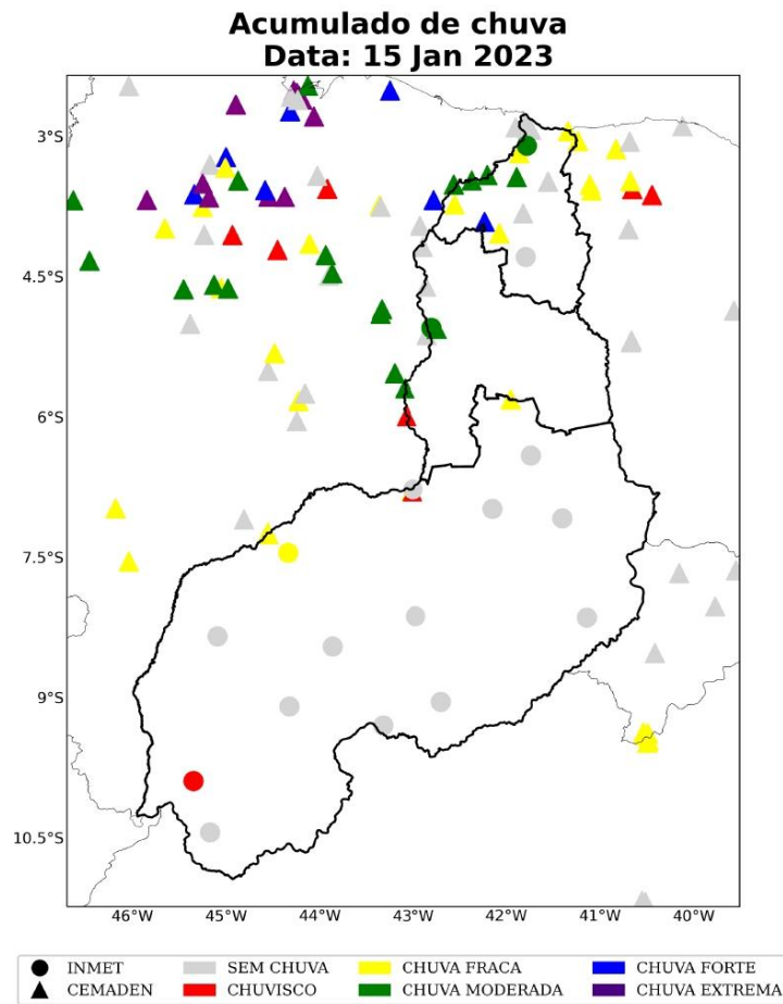
Figura 21: Acumulado diário de precipitação sobre a área de concessão da Equatorial-PI para o dia 15 de janeiro, baseado nas estações meteorológicas do INMET e CEMADEN.
