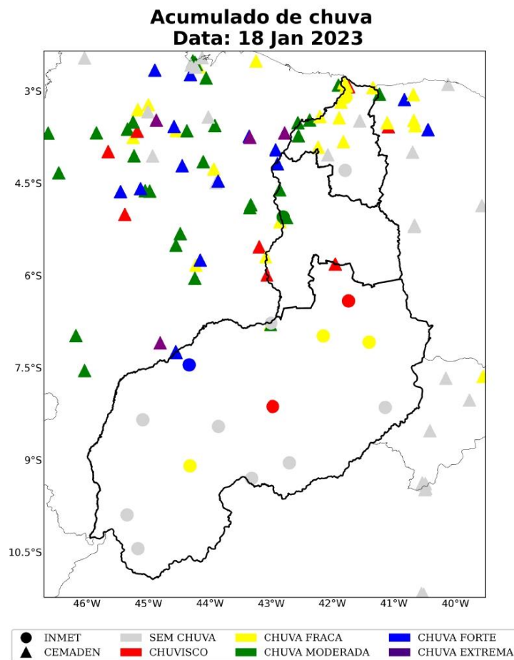
Figura 24: Acumulado diário de precipitação sobre a área de concessão da Equatorial-PI para o dia 18 de janeiro, baseado nas estações meteorológicas do INMET e CEMADEN.
