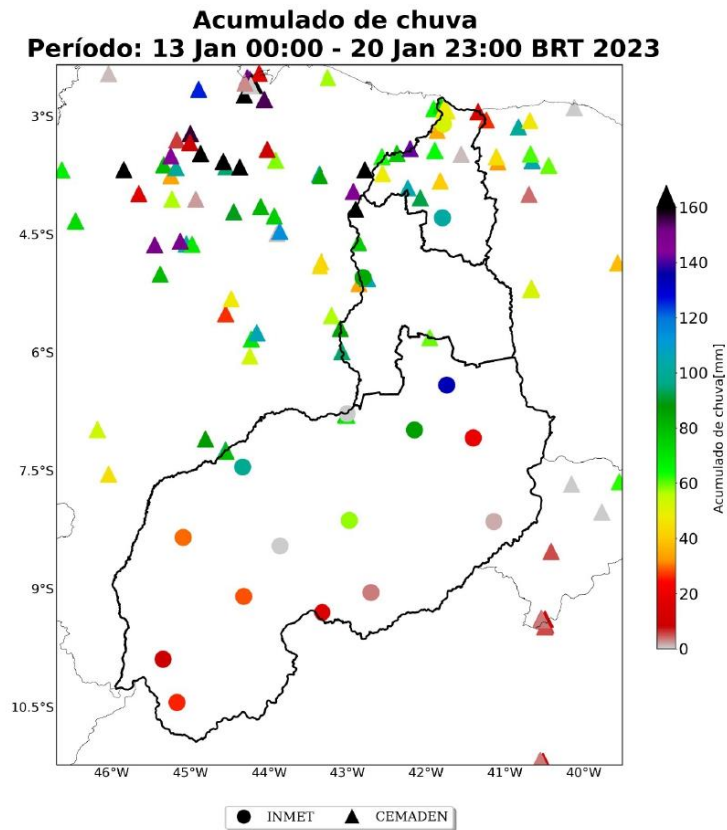
Figura 27: Acumulado de precipitação para o período 13 a 20 de janeiro de 2023 sobre a área de concessão da Equatorial-PI, baseado nas estações meteorológicas do INMET e CEMADEN.
