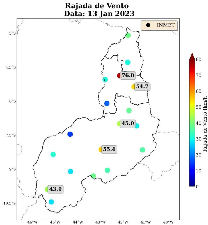
Figura 28: Máxima rajada de vento diária sobre a área de concessão da Equatorial-PI para o dia 13 de janeiro, baseado nas estações meteorológicas do INMET.
