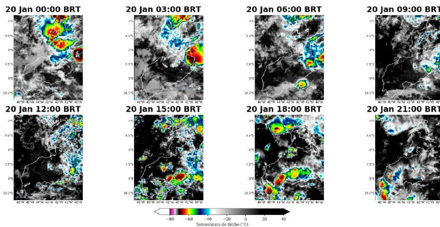
Figura 9: Imagens realizadas do satélite GOES-16 das 00 BRT até 21 BRT (a cada 3 horas) para o dia 20 de janeiro.
