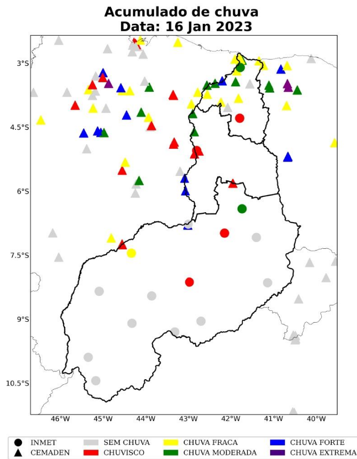
Figura 22: Acumulado diário de precipitação sobre a área de concessão da Equatorial-PI para o dia 16 de janeiro, baseado nas estações meteorológicas do INMET e CEMADEN.
