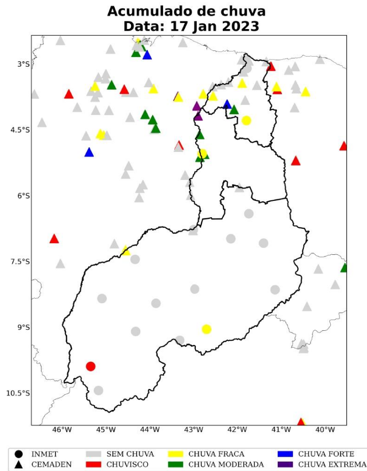
Figura 23: Acumulado diário de precipitação sobre a área de concessão da Equatorial-PI para o dia 17 de janeiro, baseado nas estações meteorológicas do INMET e CEMADEN.
