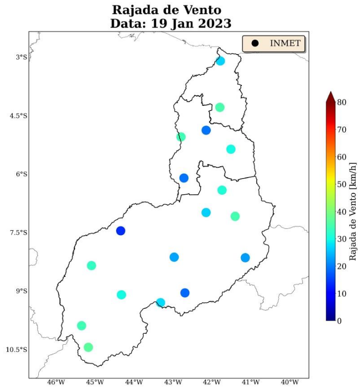
Figura 34: Máxima rajada de vento diária sobre a área de concessão da Equatorial-PI para o dia 19 de janeiro, baseado nas estações meteorológicas do INMET.
