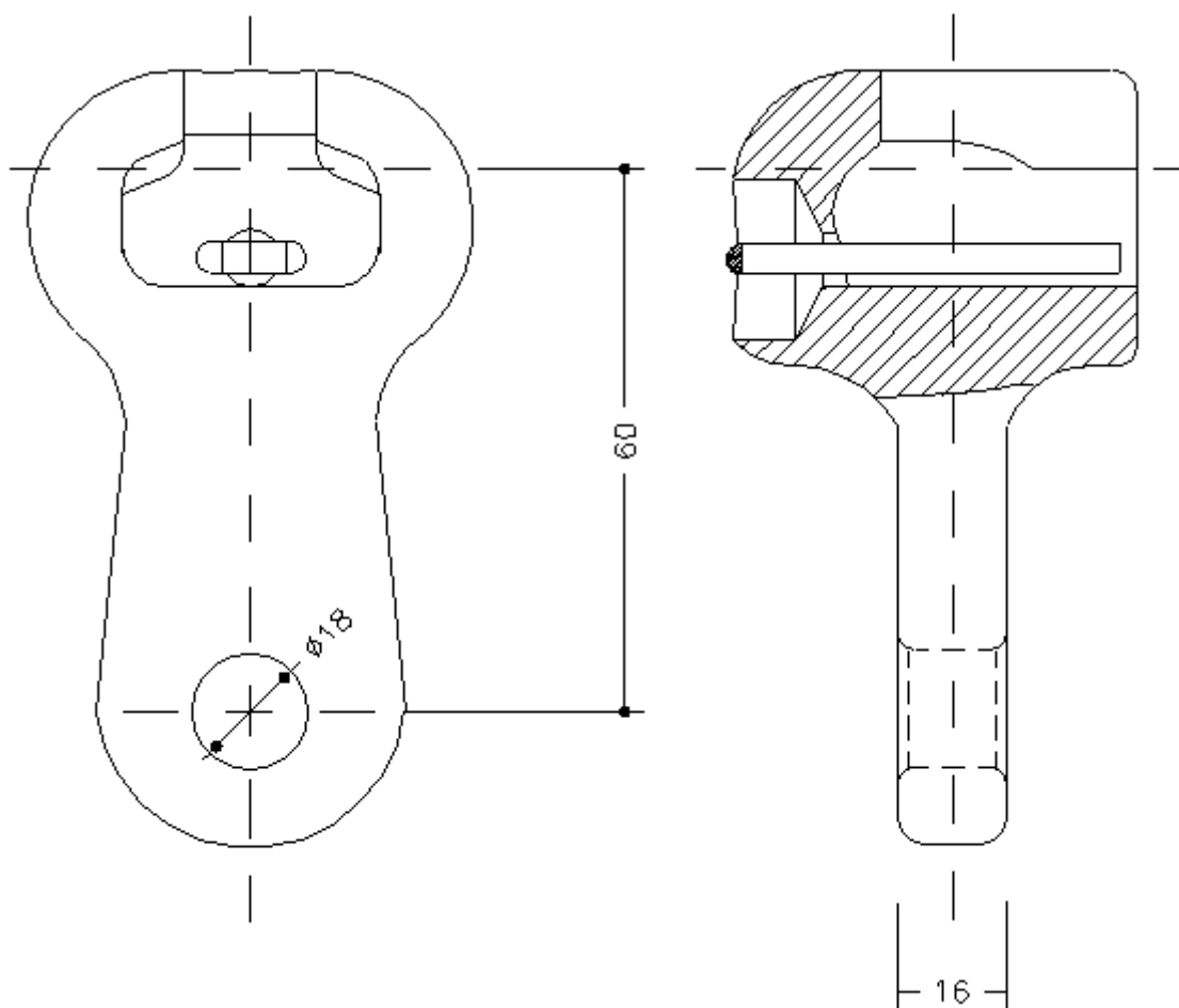
Desenho 1 – Engate Concha Olhal 90° - Detalhes Construtivos.
