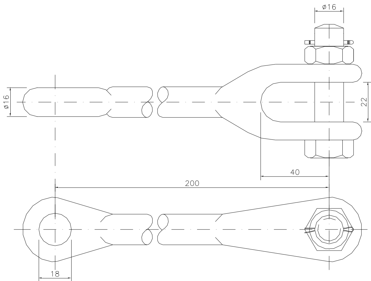
Desenho 1 – Prolongador Garfo Olhal - Detalhes Construtivos.
