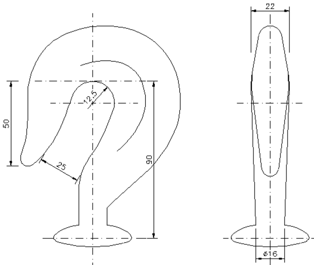
Desenho 1 – Engate Gancho Bola - Detalhes Construtivos.
