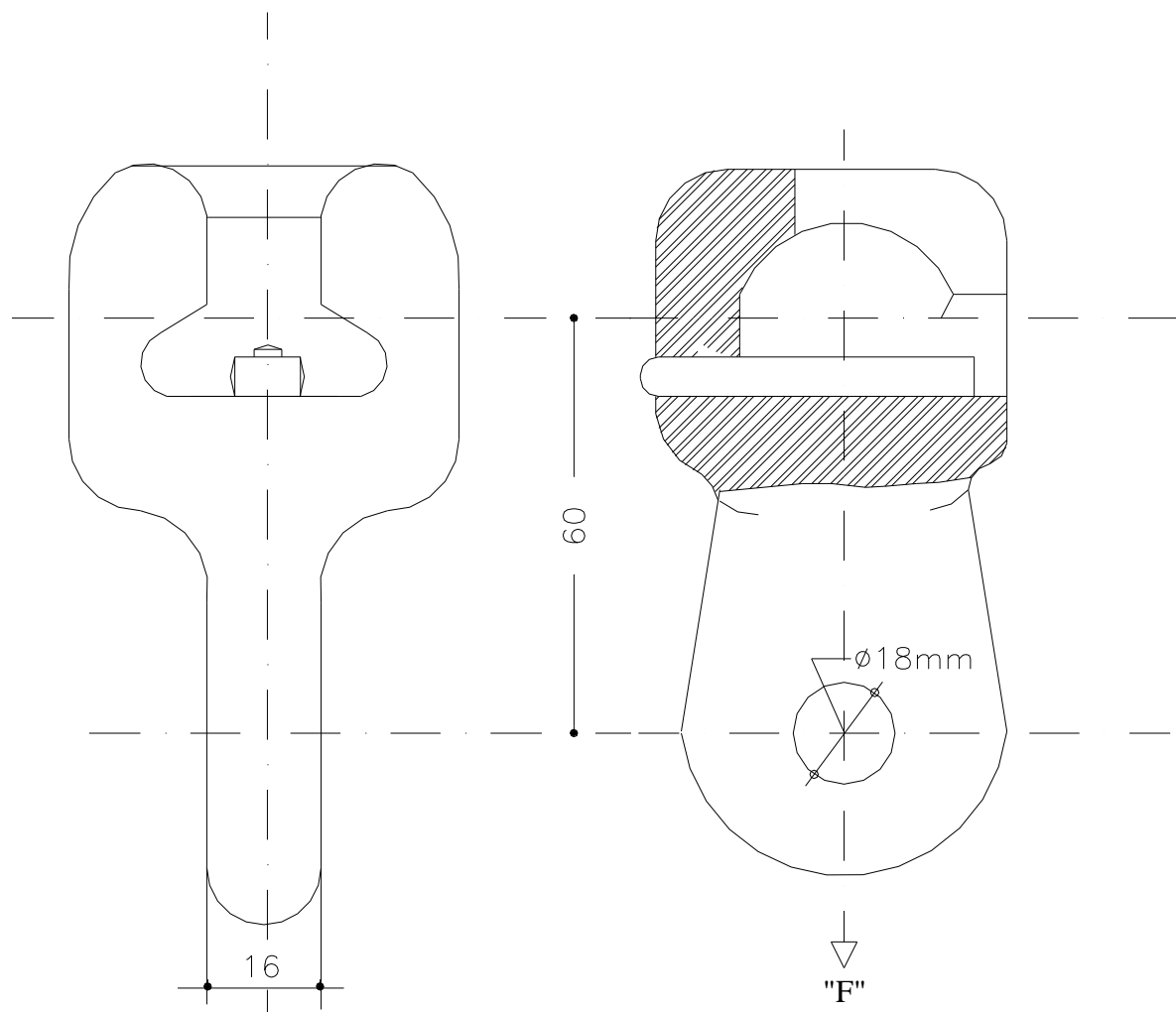
Desenho 1 – Engate Concha Olhal - Detalhes Construtivos.
