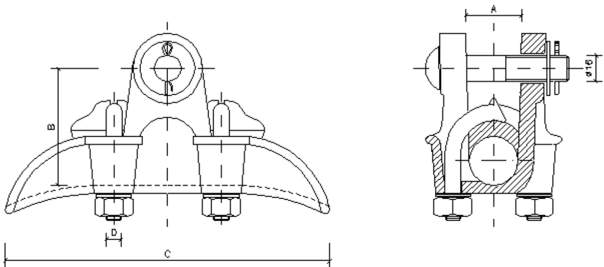
Desenho 1 – Grampo de suspensão monoarticulado - Detalhes Construtivos.
