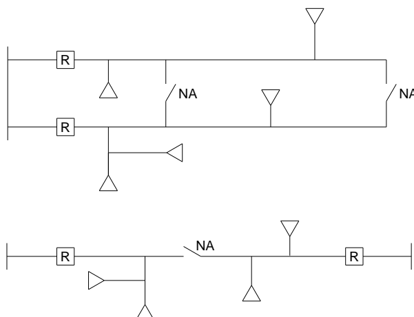
Figura 2 – Sistema Radial com Recursos
