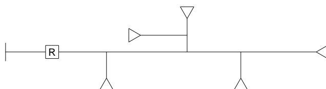
Figura 1 – Sistema Radial Simples
