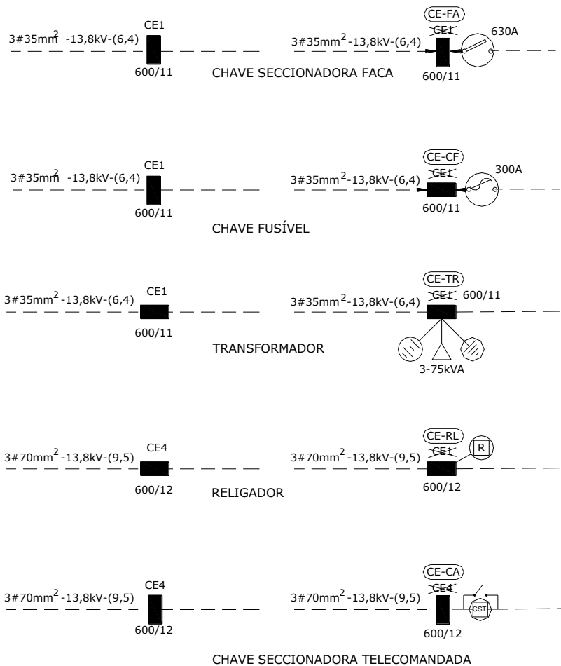
Figura 13 – Instalação de Equipamentos
