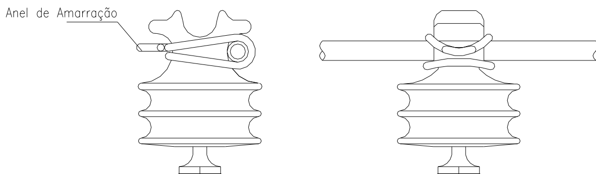
Figura 20 – Amarração Lateral das Fases nos Isoladores de Pino com Anel de Amarração
