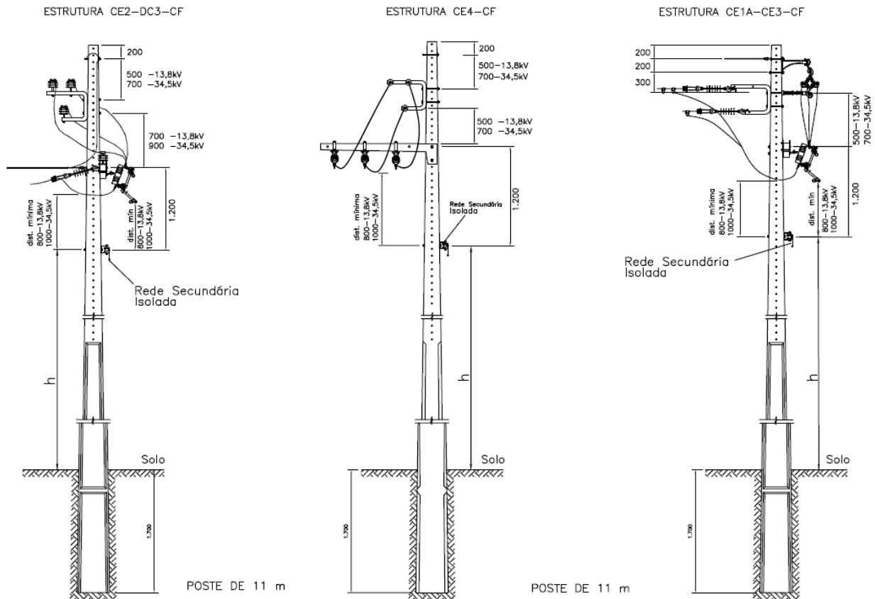
Figura 15-b – Afastamentos Mínimos – os afastamentos mínimos são iguais para 23,1 e 34,5kV
