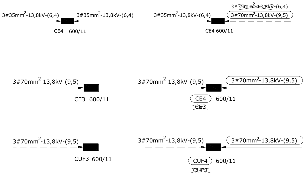
Figura 12 – Substituição da Rede
