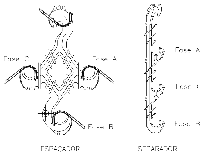
Figura 8 – Faseamento do Espaçador Losangular e Separador Vertical
