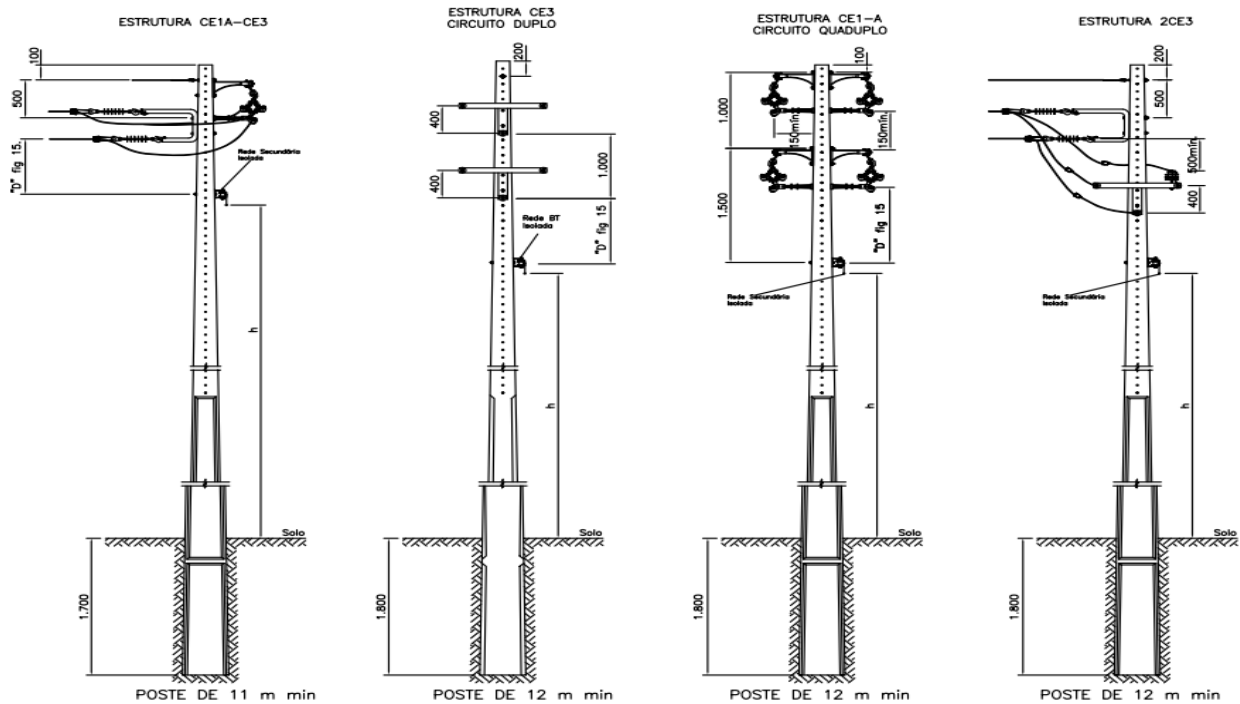
Figura 15-a – Afastamentos Mínimos
