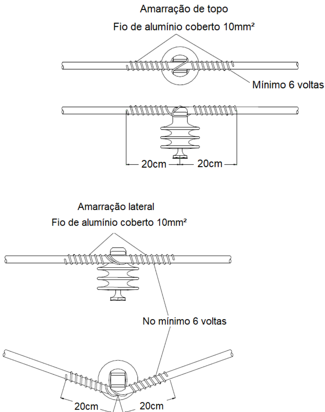
Figura 21.1 – Amarração utilizando fio de alumínio coberto
