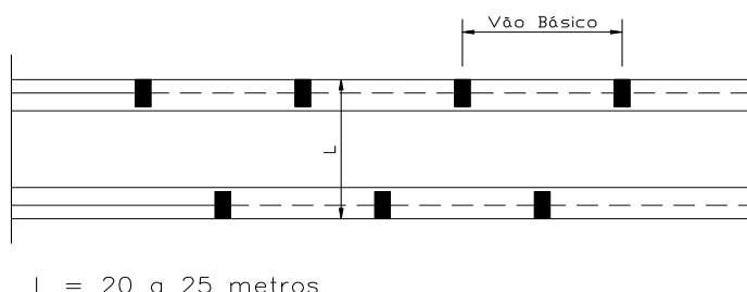
Figura 5 – Posteação Bilateral Alternada
