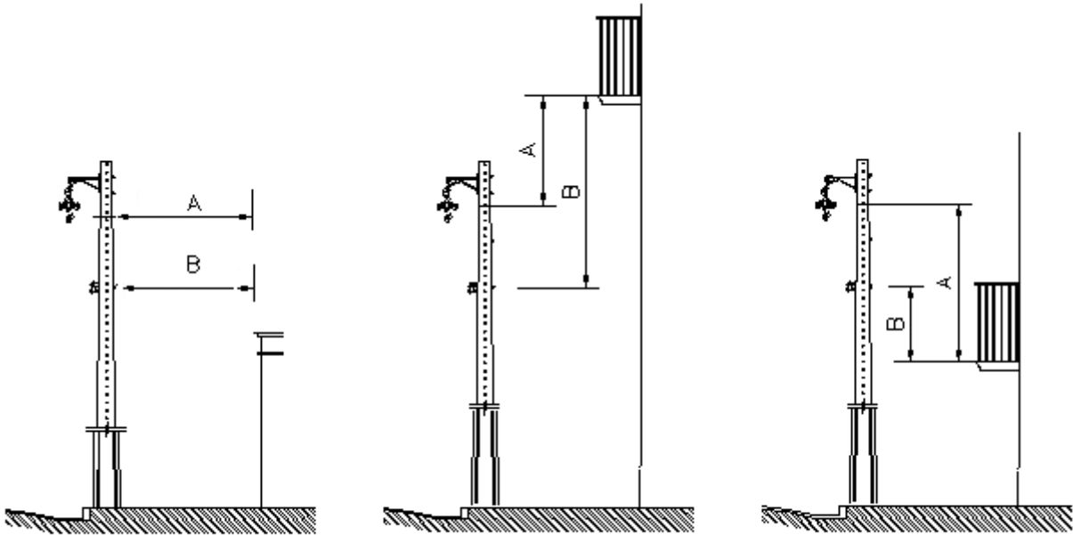
FIGURA 1 Afastamento horizontal entre os condutores e a cimalha e o telhado das edificações
