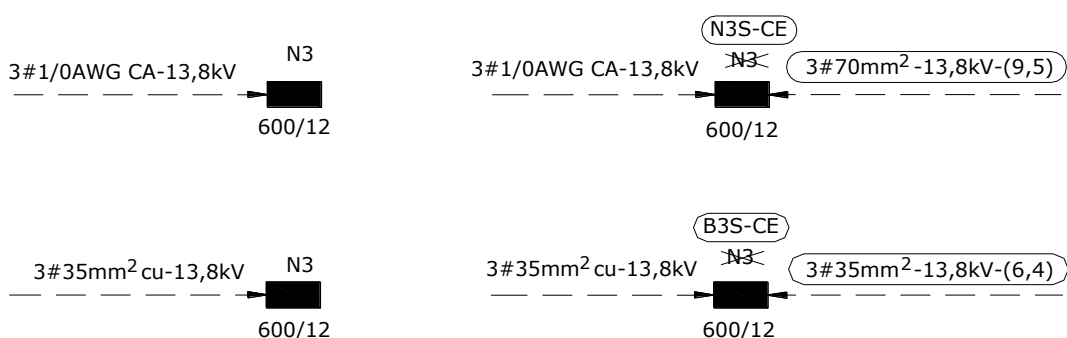
Figura 9 – Transição de Rede Convencional para Compacta
