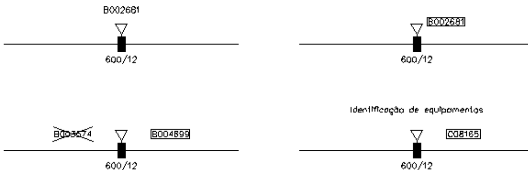
Figura 14 – Numeração de poste e equipamentos
