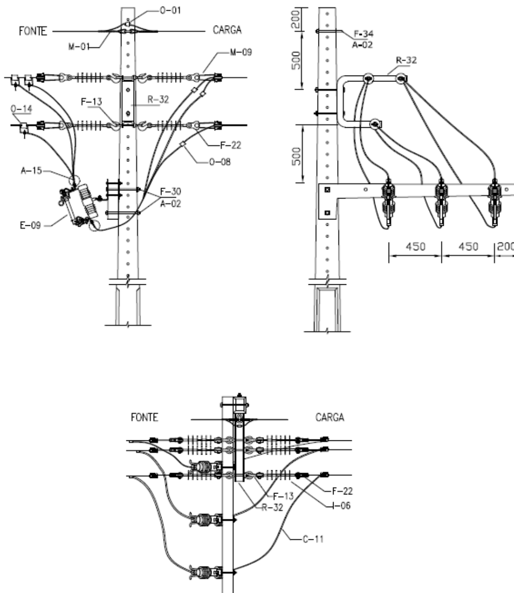
DESENHO 23.1 – ESTRUTURAS PADRONIZADAS - ESTRUTURA CE4-CF
