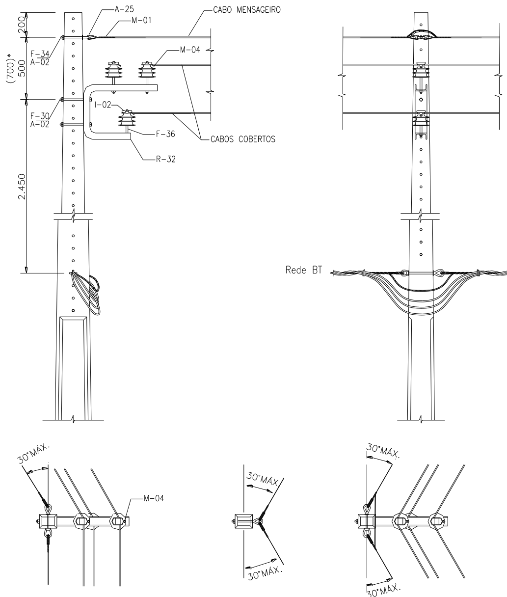
Alternativas de fixação do cabo mensageiro
