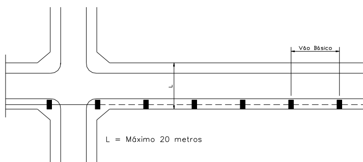
Figura 4 – Posteação Unilateral
