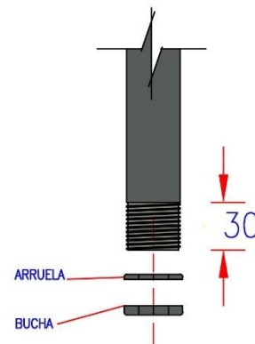
DETALHE DA ROSCA
